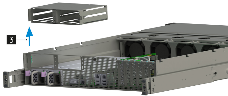
Рис. 22. Снятие каркаса НИКА.301233.012
