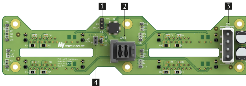
Рис. 13. Плата расширения 4SFF (НИКА.469535.063)
