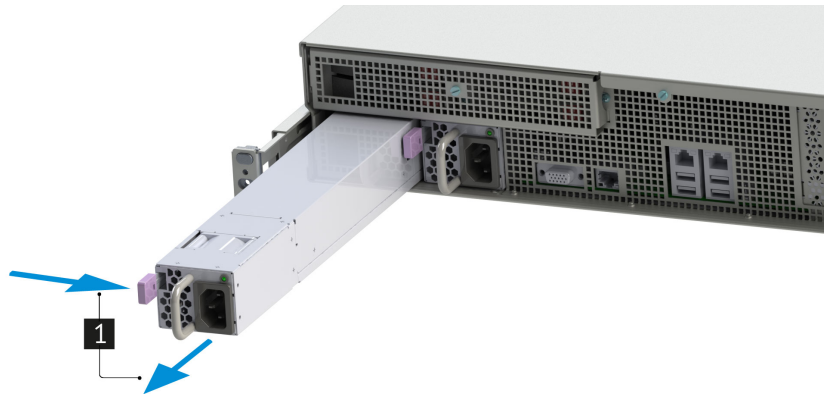
Рис. 50. Извлечение блока питания
