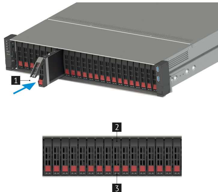
Рис. 42. Установка дисков
