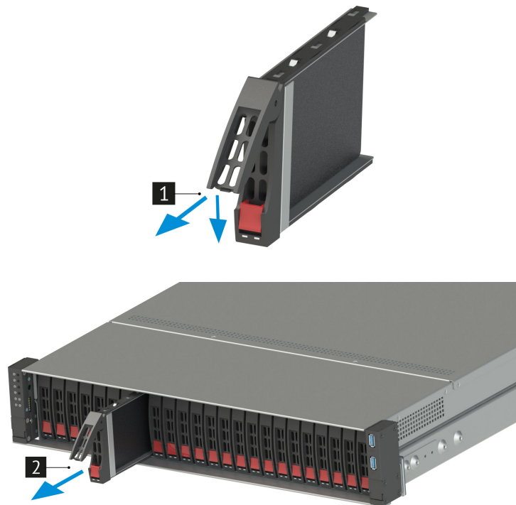
Рис. 41. Извлечение дисков
