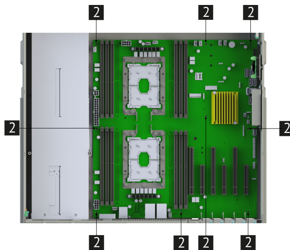
Рис. 40. Установка материнской платы
