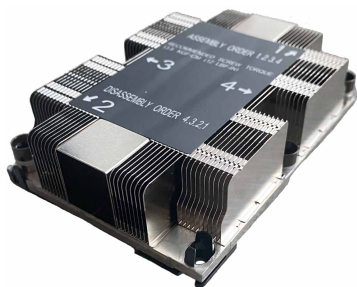
Рис. 32. 1U радиатор
