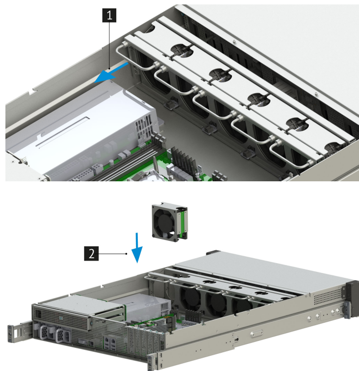
Рис. 27. Подключение вентилятора
