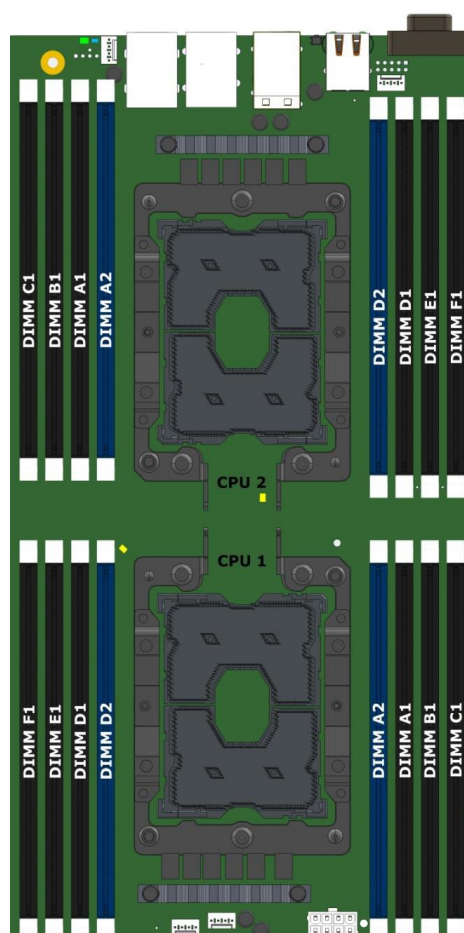
Рис. 29. Расположение разъемов
