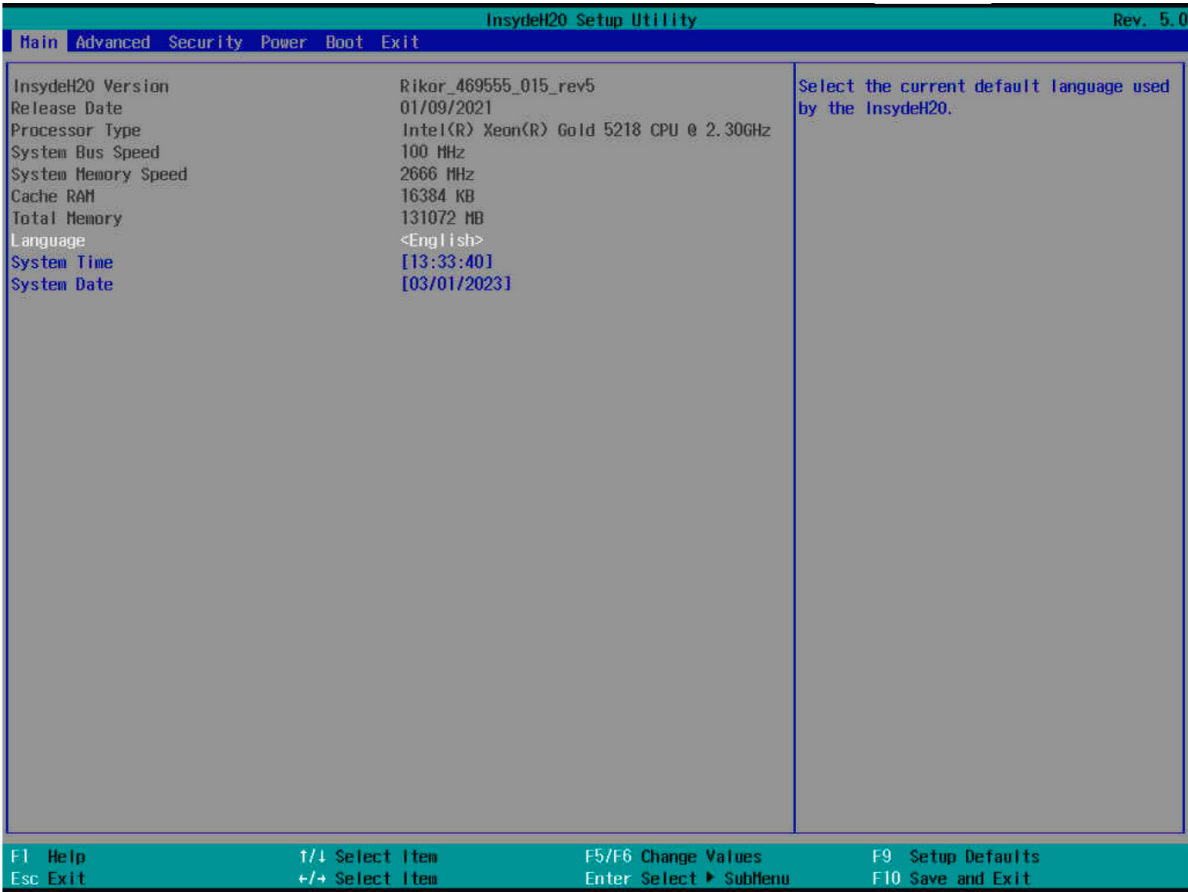
Рис. 60. Разделы меню «Main»
