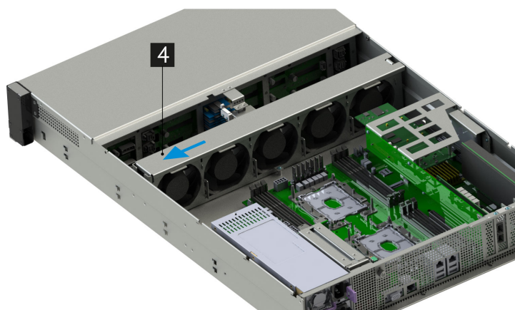
Рис. 28. Подключение вентилятора
