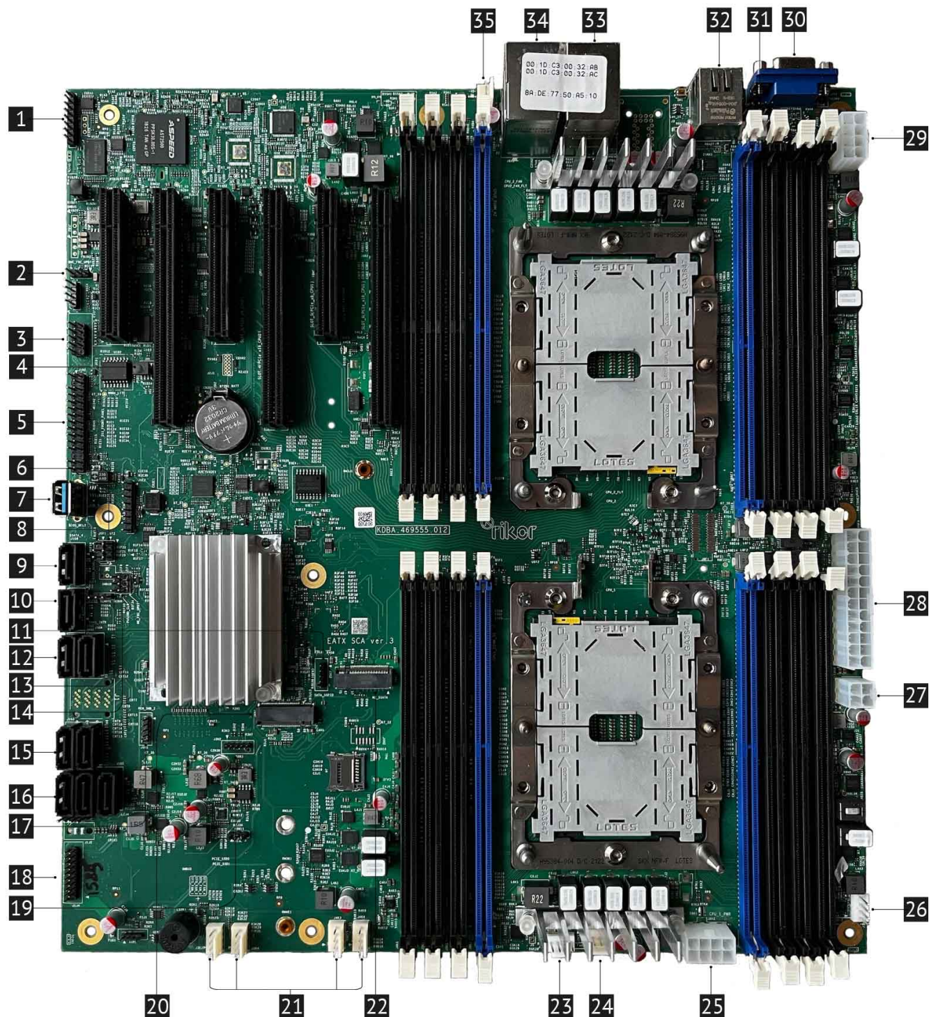
Рис. 10. Соединители и переключатели материнской платы
