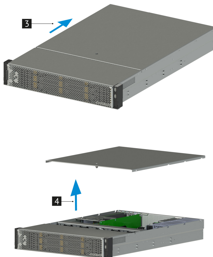
Рис. 21. Снятие верхней крышки сервера
