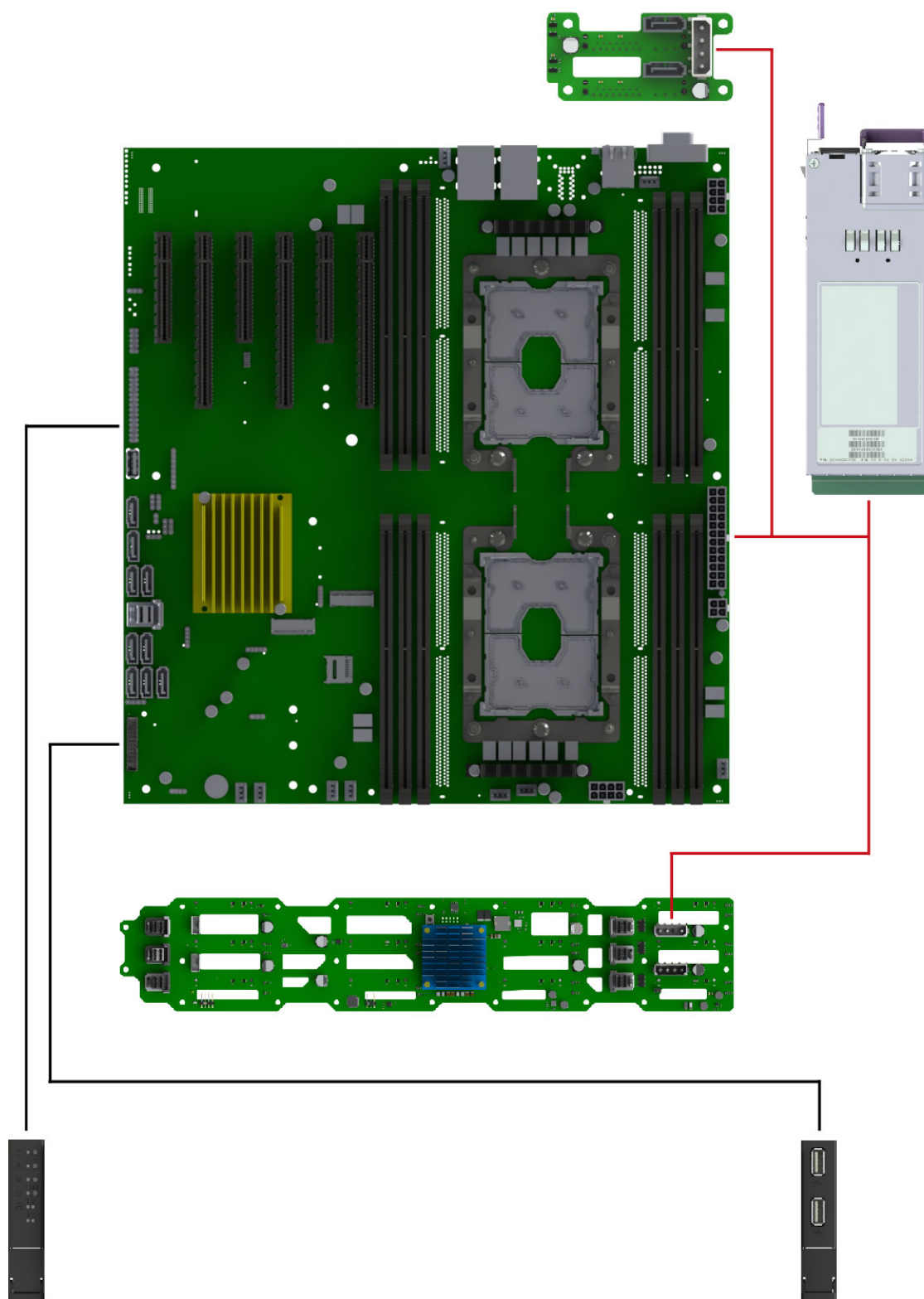
Рис. 24. Схема прокладки системных кабелей и кабелей питания
