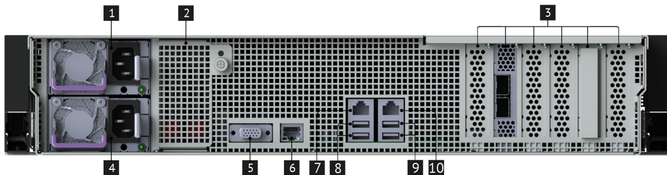
Рис. 5. Вид сервера сзади
