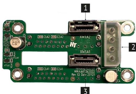
Рис. 12. Плата расширения 2SFF SATA (НИКА.469535.131)
