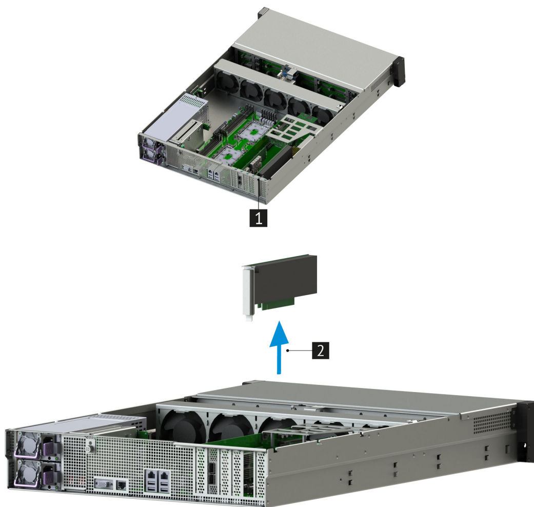
Рис. 50. Извлечение карты расширения
