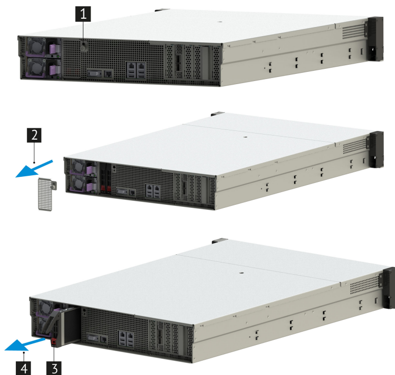
Рис. 44. Извлечение тыльных дисков
