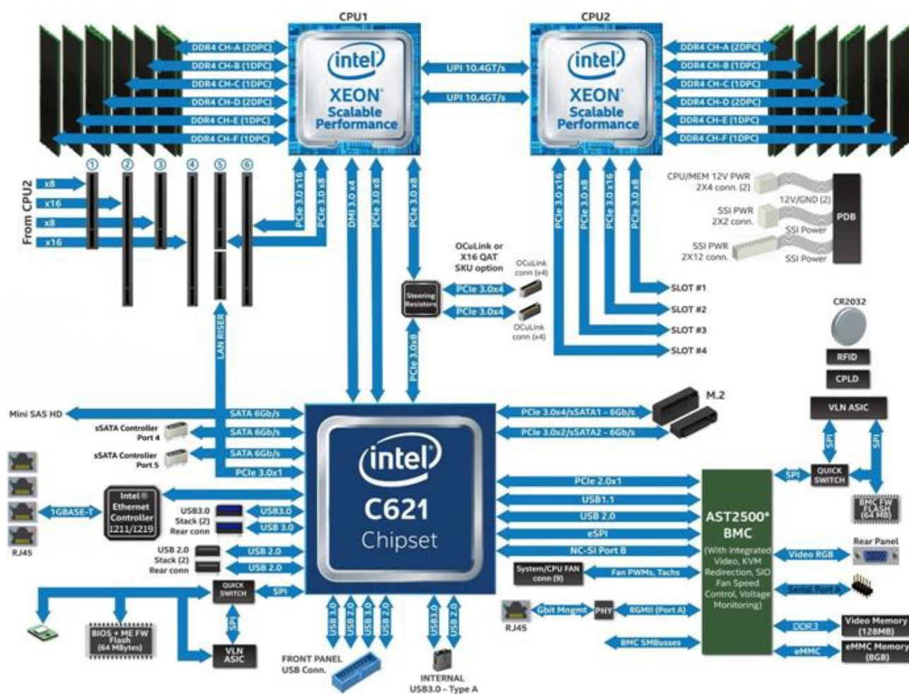
Рис. 1. Структурная схема материнской платы Rikor® R-BD-SXRM-XS16.EA.V6.0
