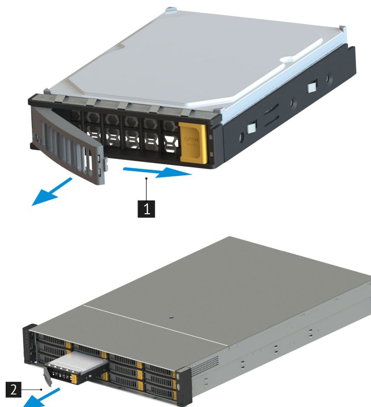
Рис. 42. Извлечение дисков
