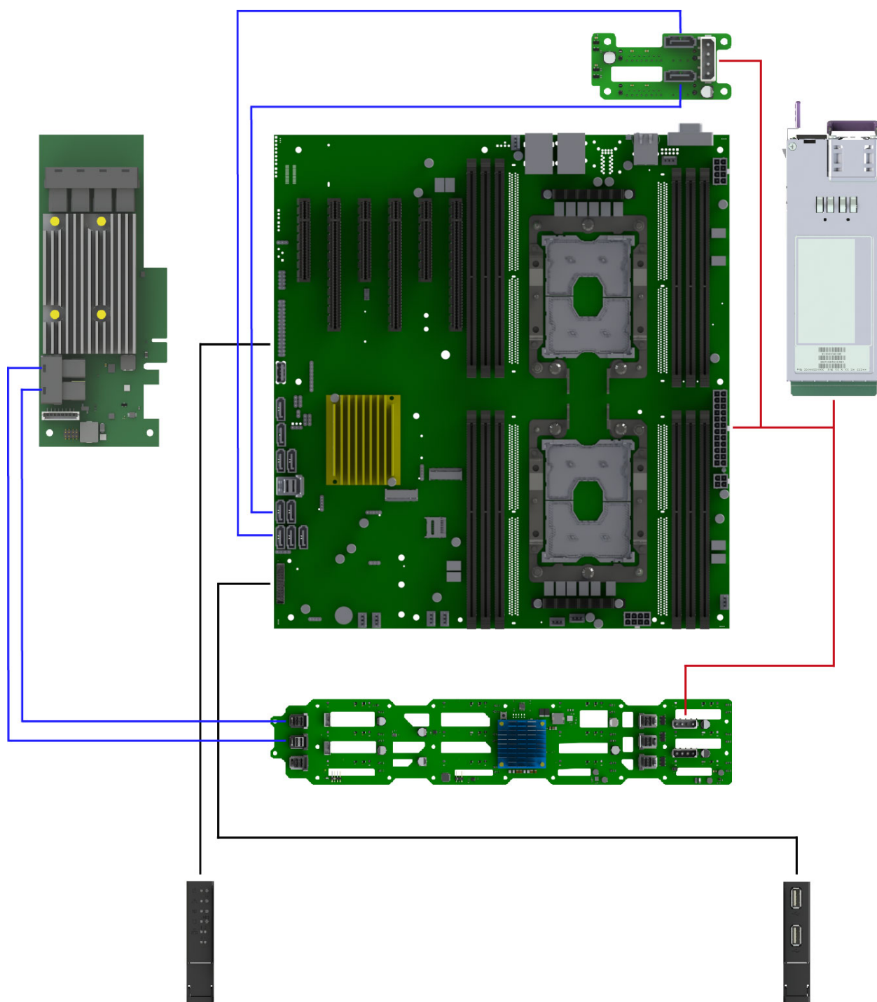
Рис. 25. Схема прокладки системных кабелей и кабелей питания с подключением PCIe RAID при использовании платы расширения 2SFF SATA (НИКА.469535.131)
