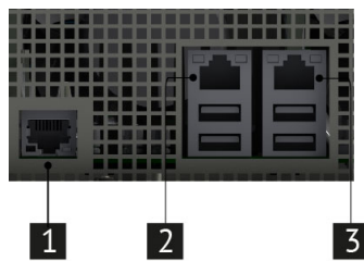
Рис. 7. Сетевые интерфейсы
