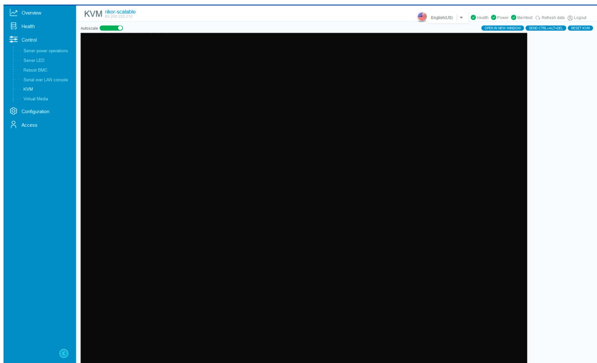
Рис. 76. Окно «KVM»
