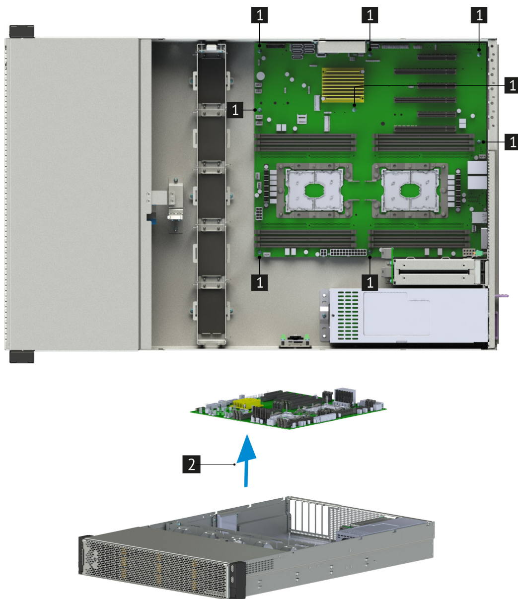
Рис. 40. Извлечение материнской платы из сервера
