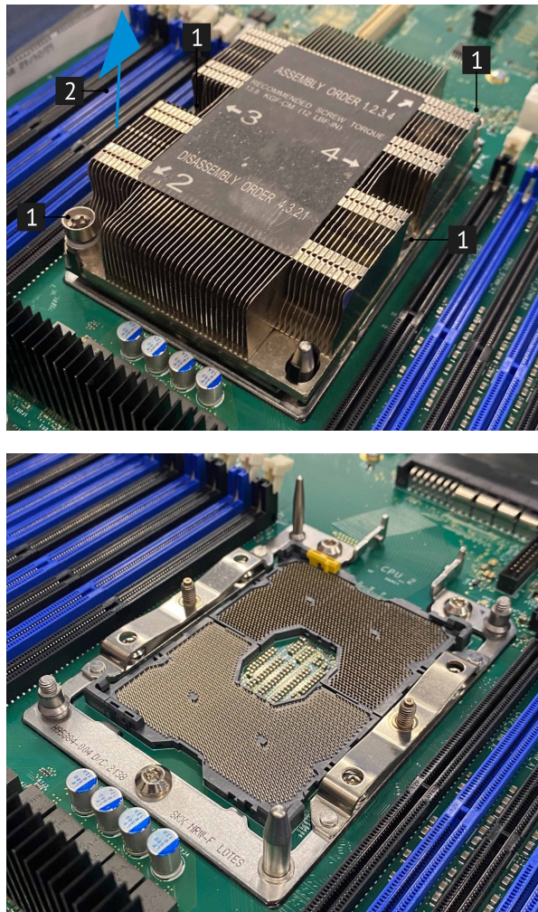
Рис. 35. Снятие модуля процессора с радиатором
