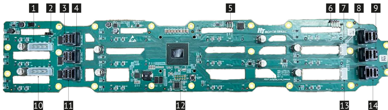
Рис. 11. Плата объединительная 12LFF активная (НИКА.469535.124)
