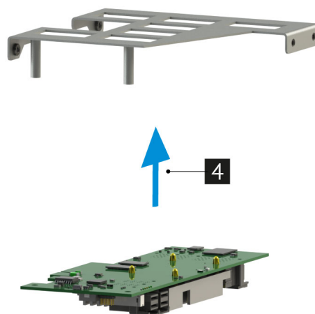
Рис. 48. Извлечение контроллера дискового SAS-3 RAID-24i
