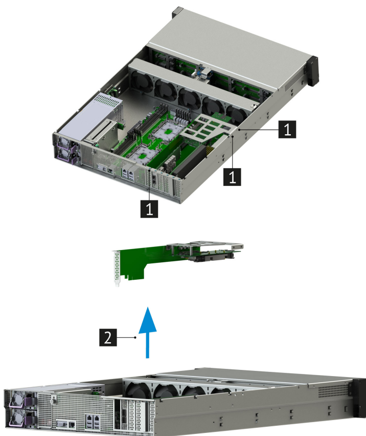
Рис. 46. Извлечение адаптера поворотного PCIe
