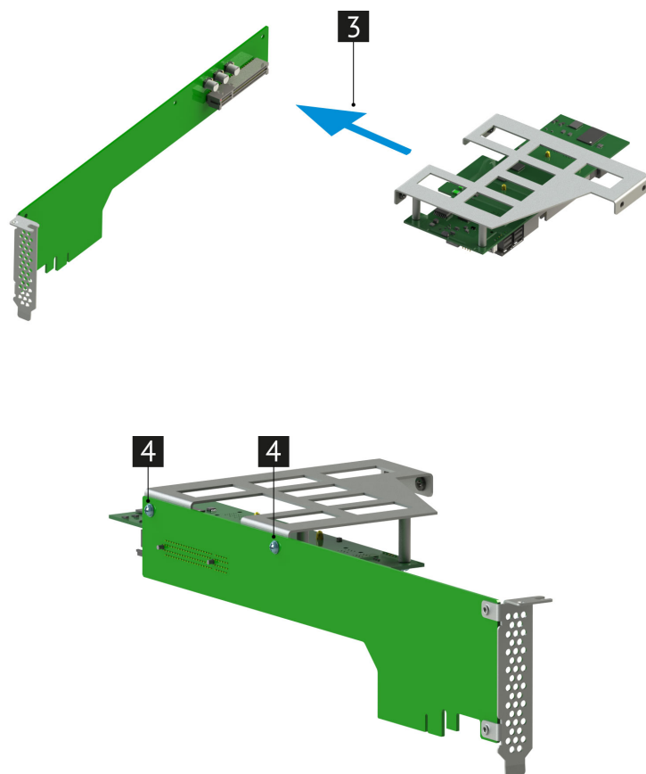
Рис. 49. Установка контроллера дискового SAS-3 RAID-24i
