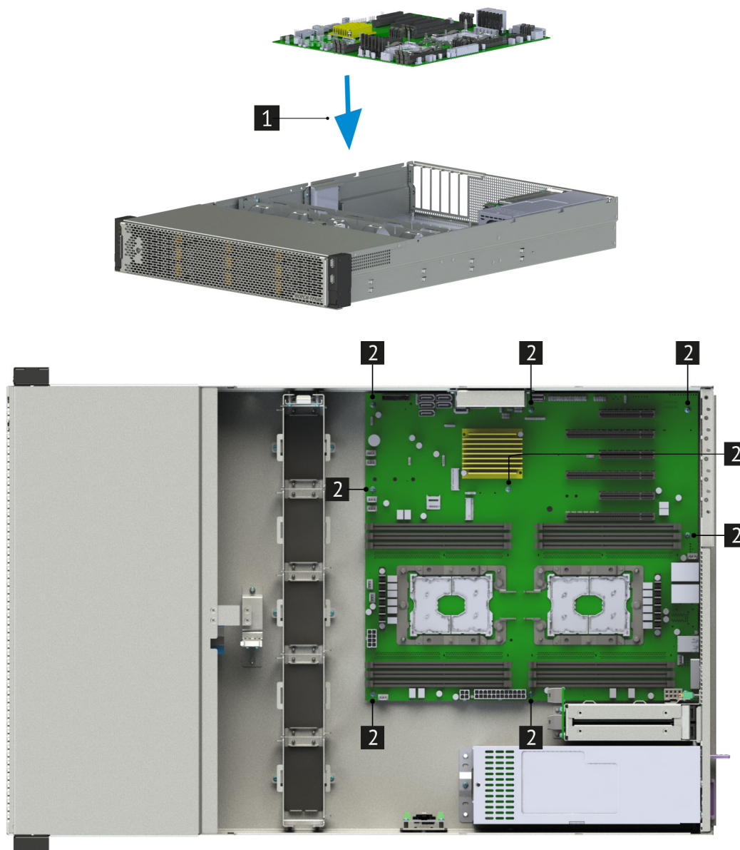
Рис. 41. Установка материнской платы в сервер
