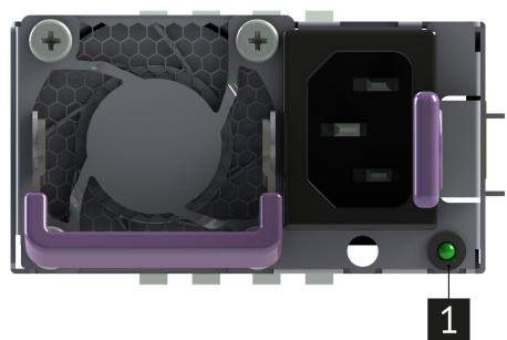
Рис. 52. Светодиодная индикация состояния блока питания
