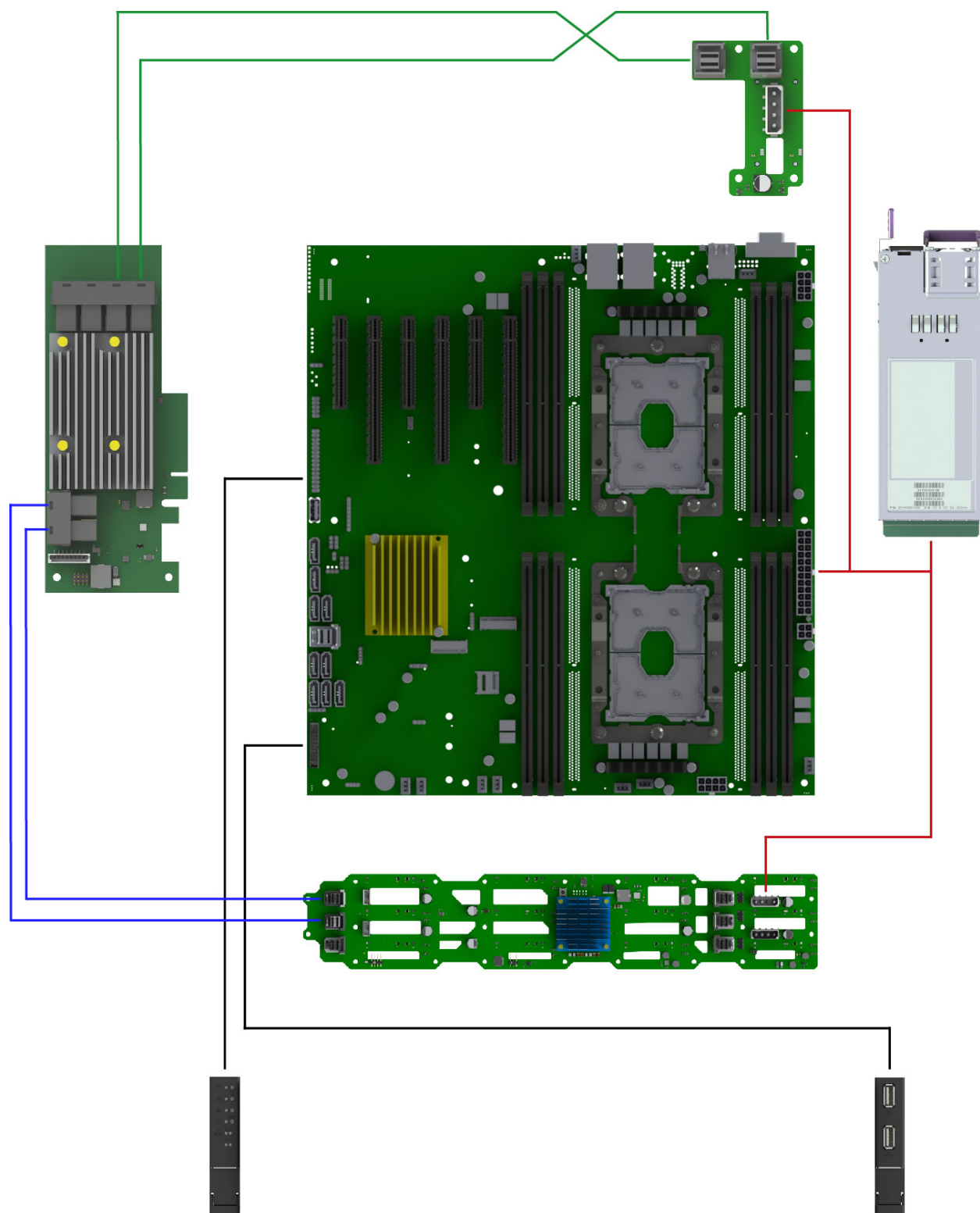
Рис. 26. Схема прокладки системных кабелей и кабелей CBL-SAST-0658 с подключением PCIe RAID при использовании платы расширения 2SFF NVMe (НИКА.469535.220)
