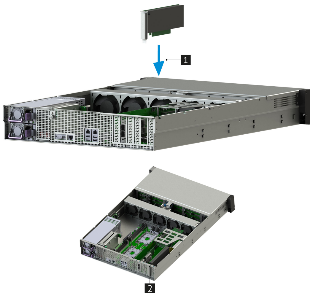
Рис. 51. Установка карты расширения
