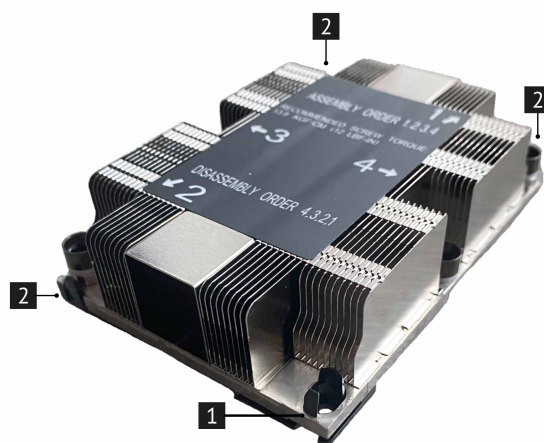
Рис. 36. Снятие процессора с 1U радиатора
