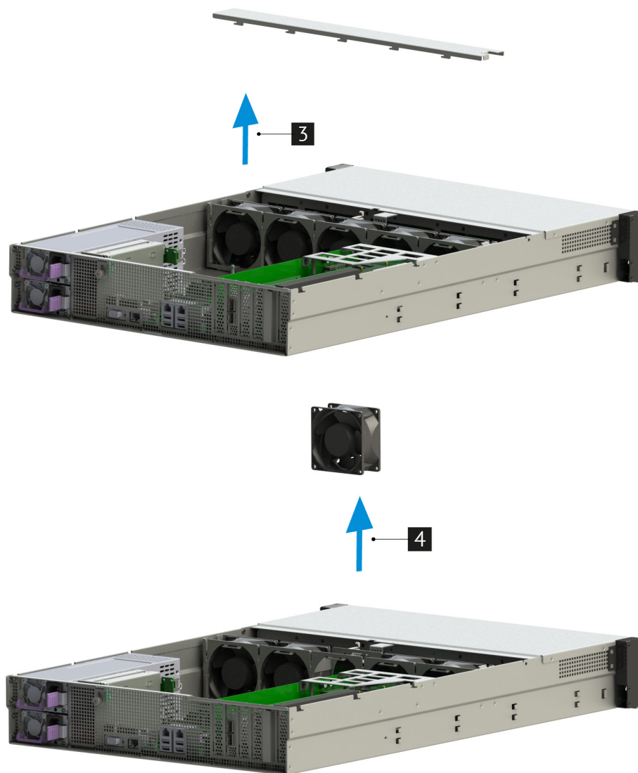
Рис. 27. Извлечение вентилятора из сервера
