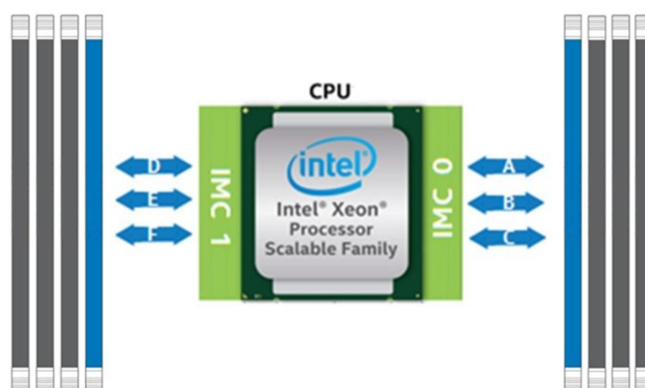
Рис. 30. Каналы памяти
