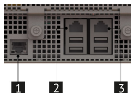
Рис. 7. Сетевые интерфейсы
