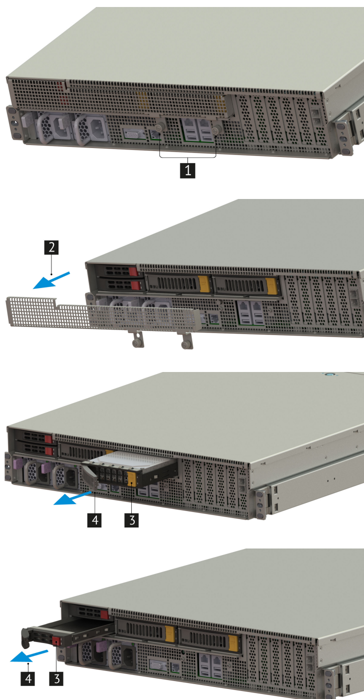
Рис. 47. Извлечение дисков
