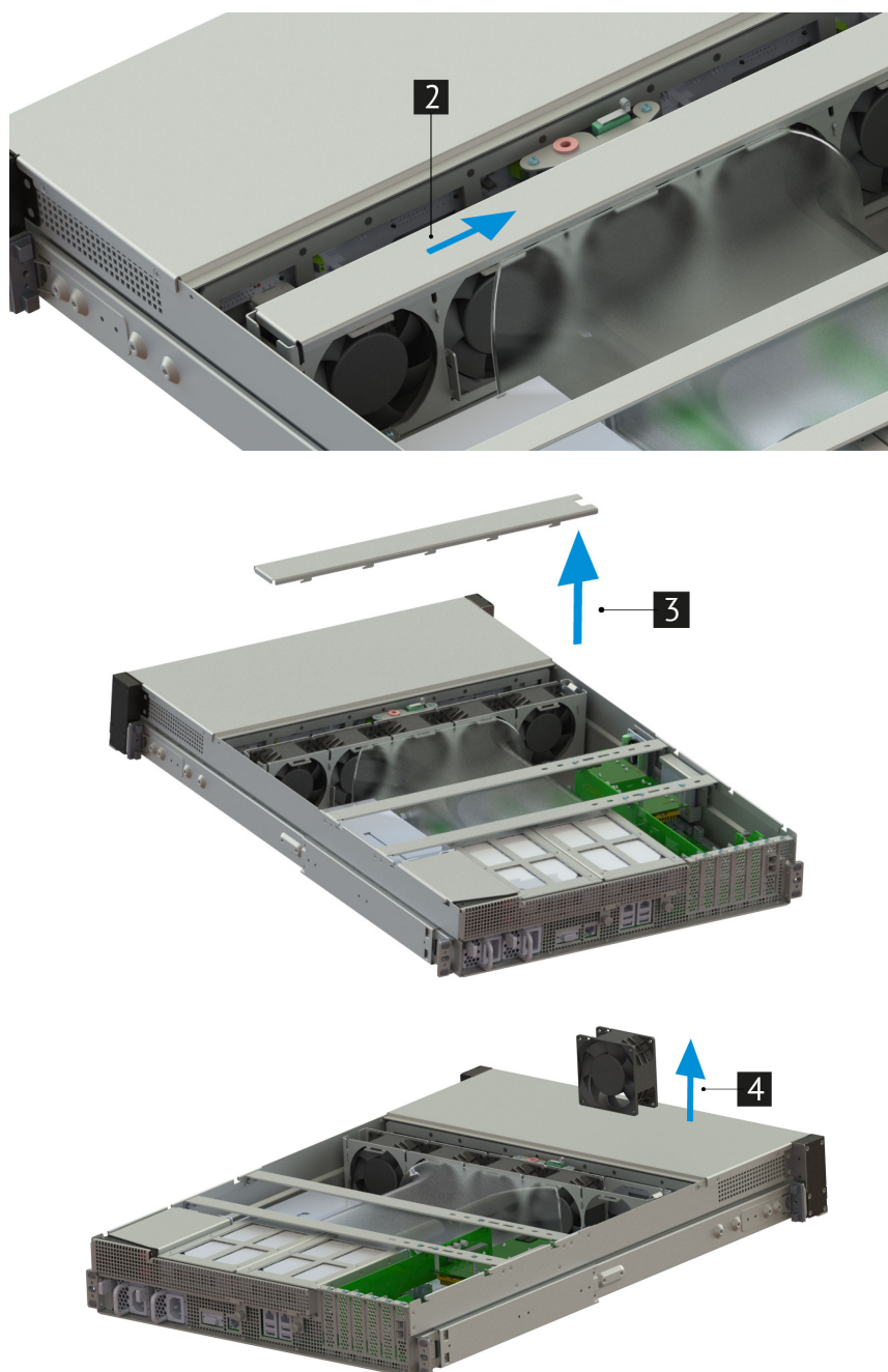
Рис. 30. Извлечение вентилятора
