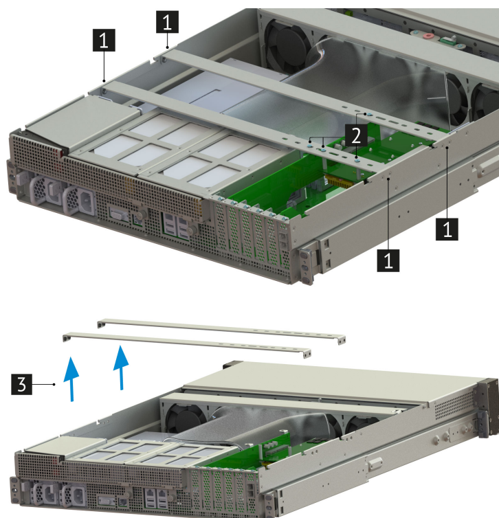
Рис. 22. Снятие скоб
