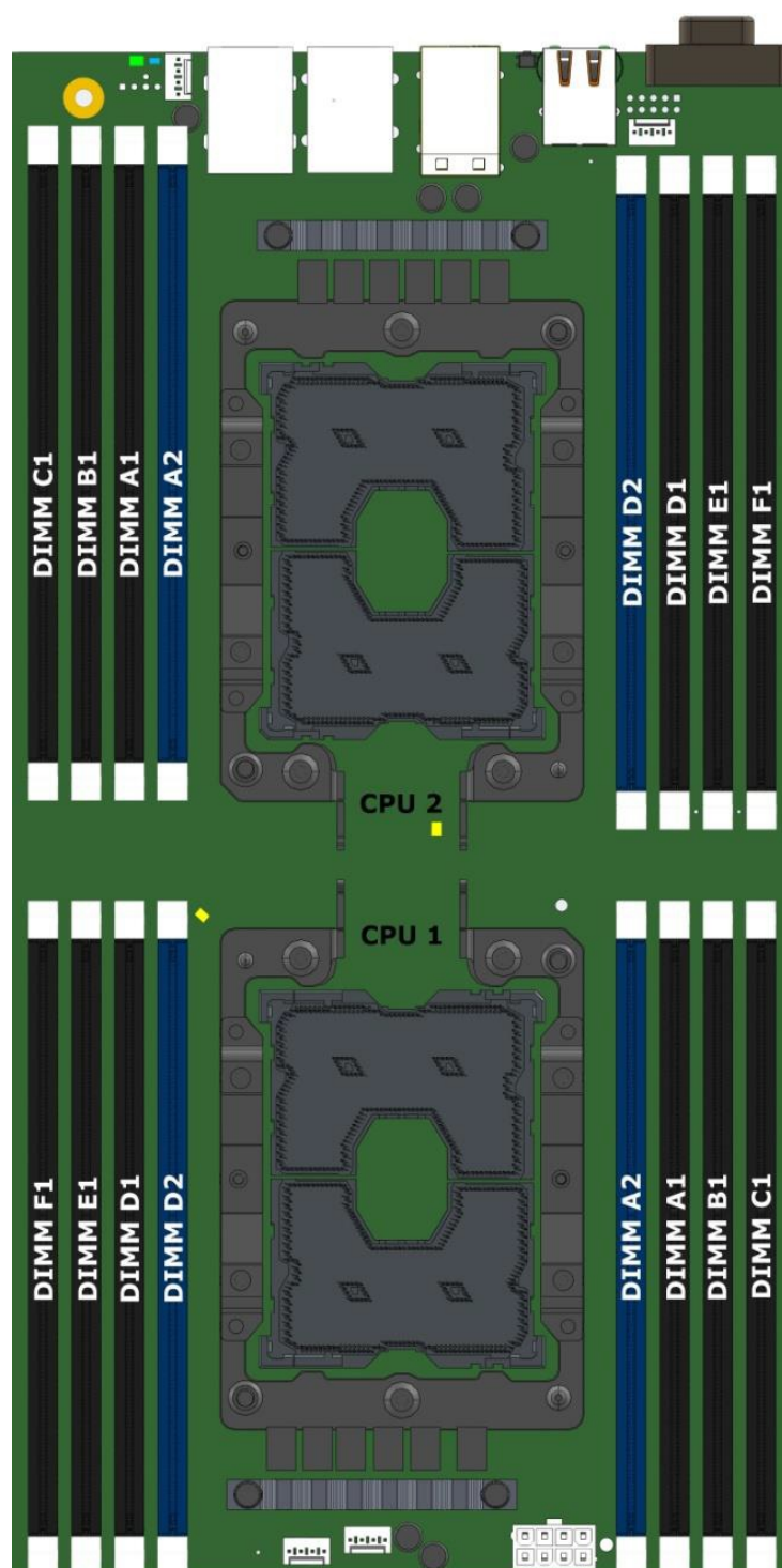
Рис. 32. Расположение разъемов
