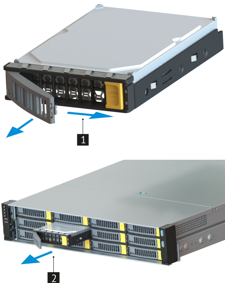
Рис. 45. Извлечение дисков
