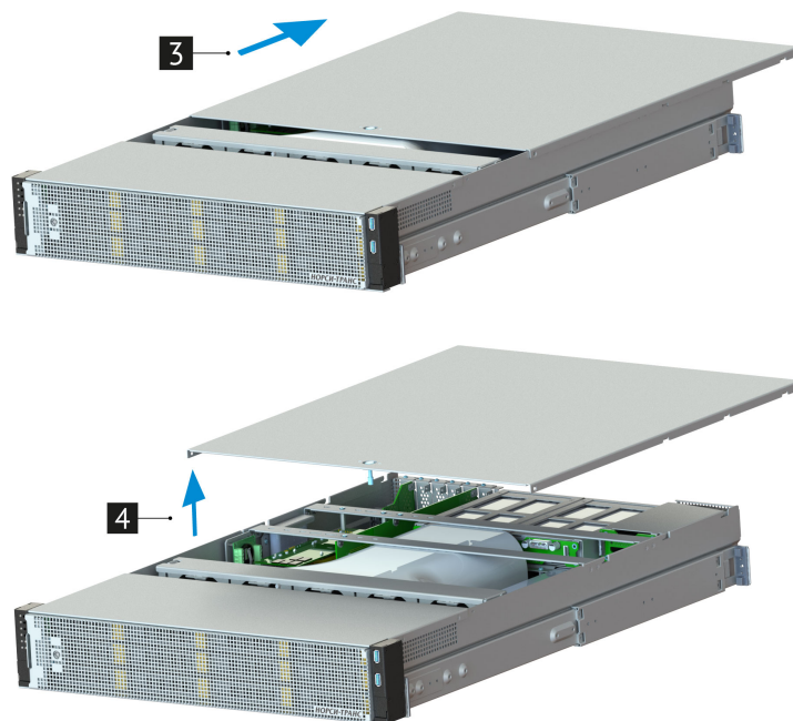
Рис. 20. Снятие верхней крышки платформы
