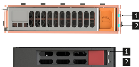
Рис. 9. Индикация дисков
