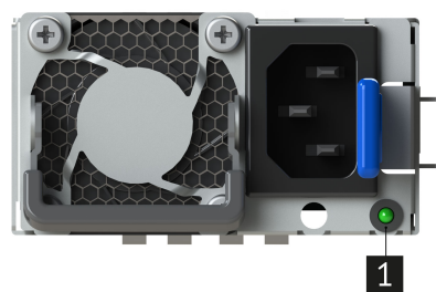
Рис. 60. Светодиодная индикация состояния блока питания
