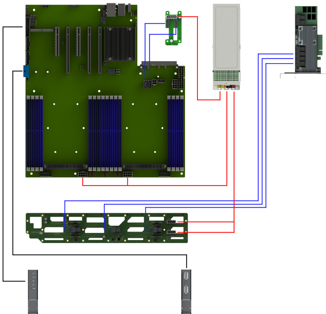
Рис. 30. Схема прокладки системных кабелей и кабелей питания с подключением PCIe RAID при использовании платы расширения 2SFF SATA (НИКА.469535.131)
