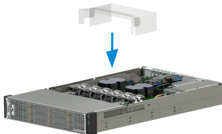
Рис. 25. Установка воздушного кожуха
