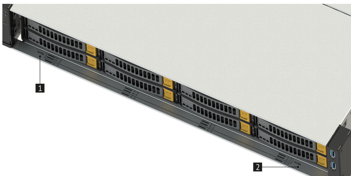
Рис. 51. Место установки NVMe-дисков в сервер
