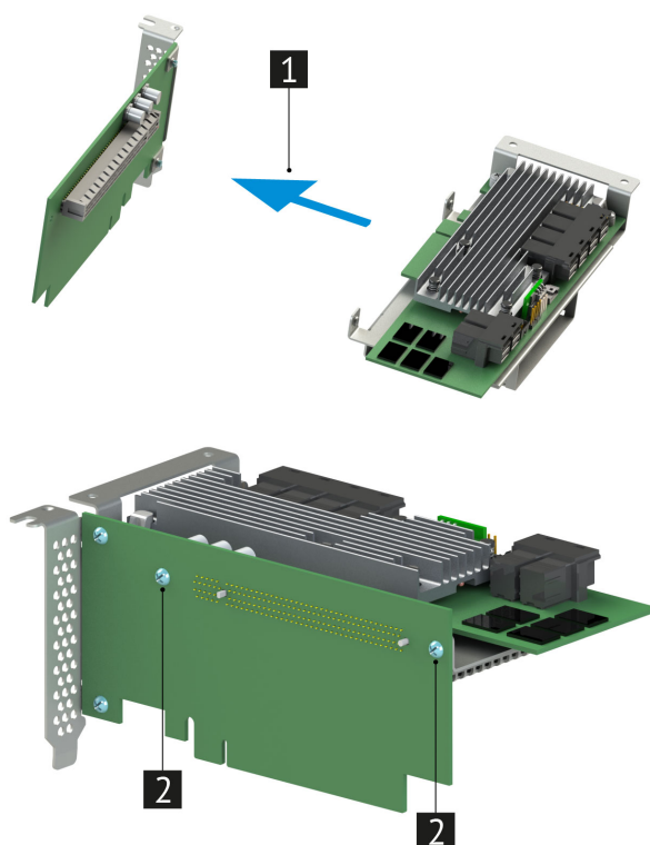
Рис. 57. Установка контроллера дискового MegaRAID 9361-24i
