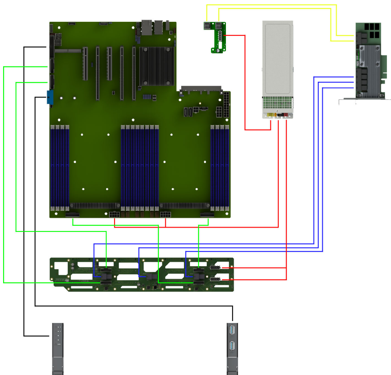
Рис. 33. Схема прокладки системных кабелей и кабелей Oculink-SLIMline X8-X8 с подключением PCIe RAID при использовании платы расширения 2SFF NVMe (НИКА.469535.220)
