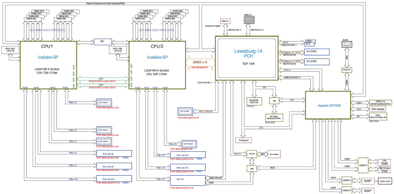
Рис. 1. Структурная схема материнской платы МП2хІХS3G «Арктур»
