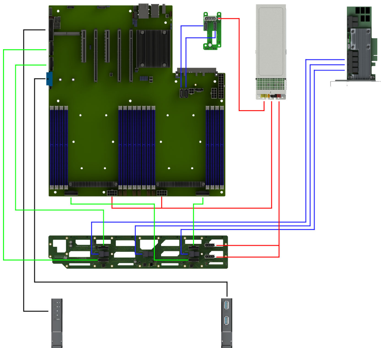
Рис. 34. Схема прокладки системных кабелей и кабелей Oculink-SLIMline X8-X8 с подключением PCIe RAID при использовании платы расширения 2SFF SATA (НИКА.469535.131)
