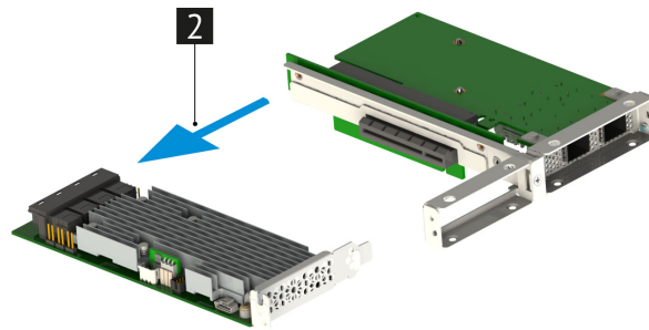
Рис. 52. Извлечение контроллера дискового MegaRAID 9361-16i
