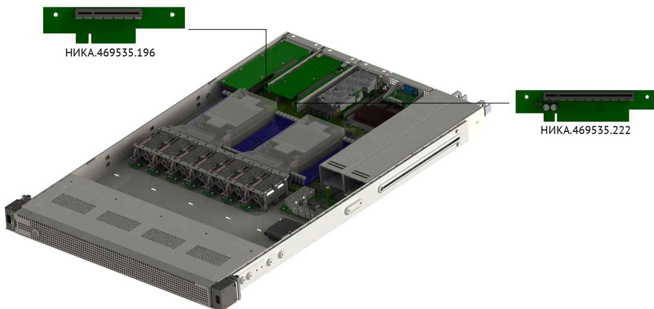
Рис. 12. Расположение PCIe-райзеров в сервере
