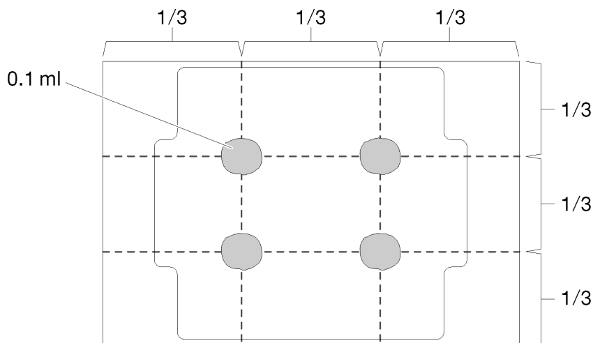
Рис. 40. Нанесение термопасты
