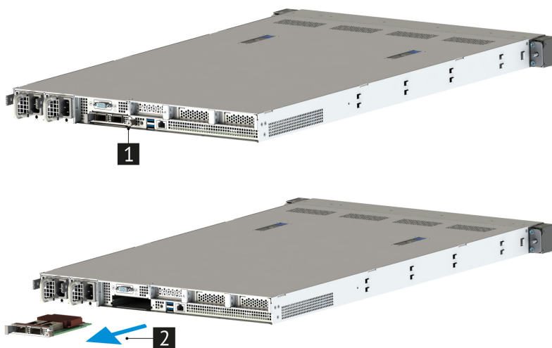
Рис. 60. Извлечение карты OCP 3.0 PCIe x16
