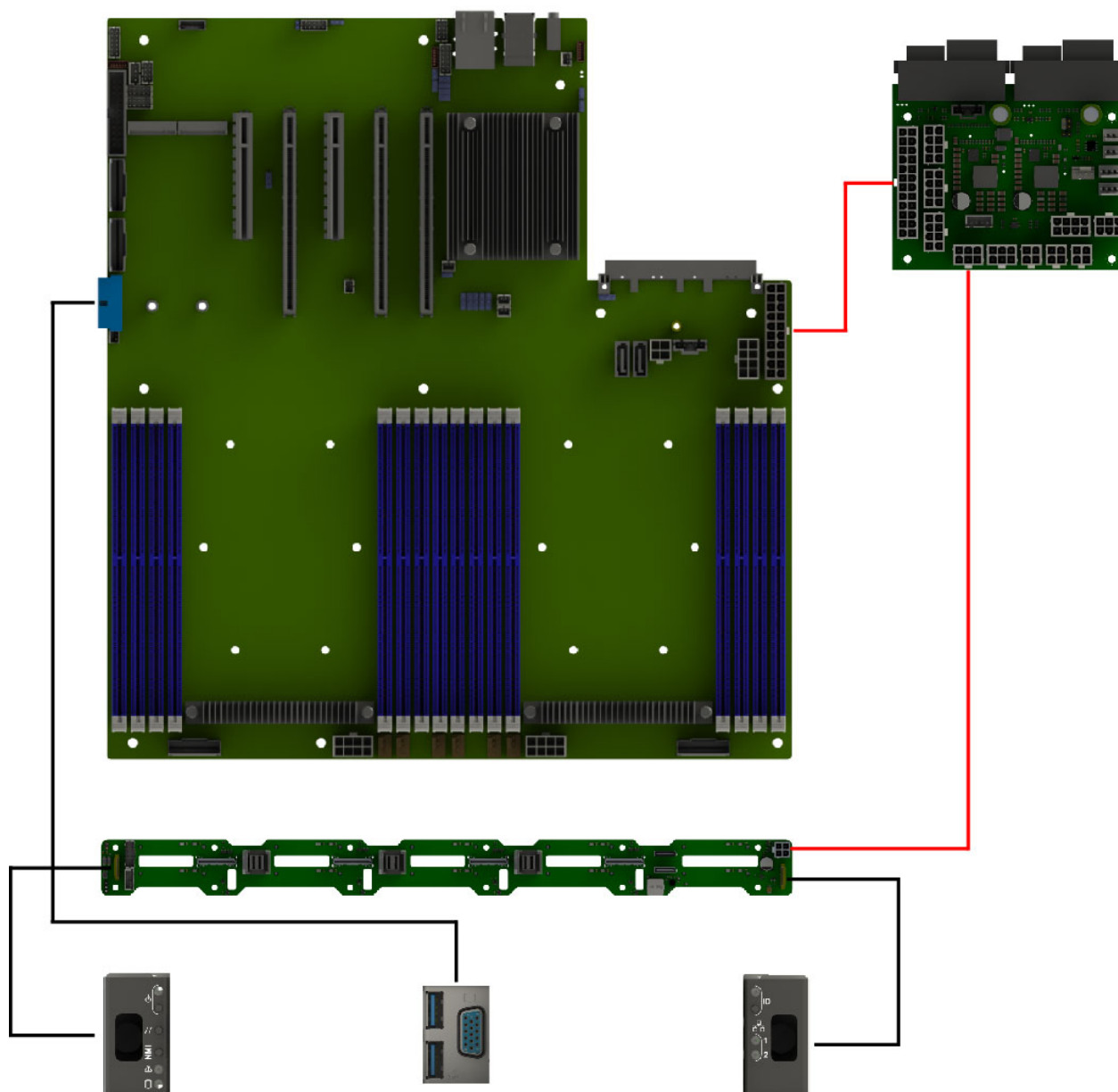
Рис. 27. Схема прокладки системных кабелей и кабелей питания
