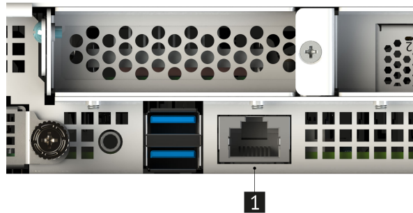
Рис. 7. Сетевые интерфейсы
