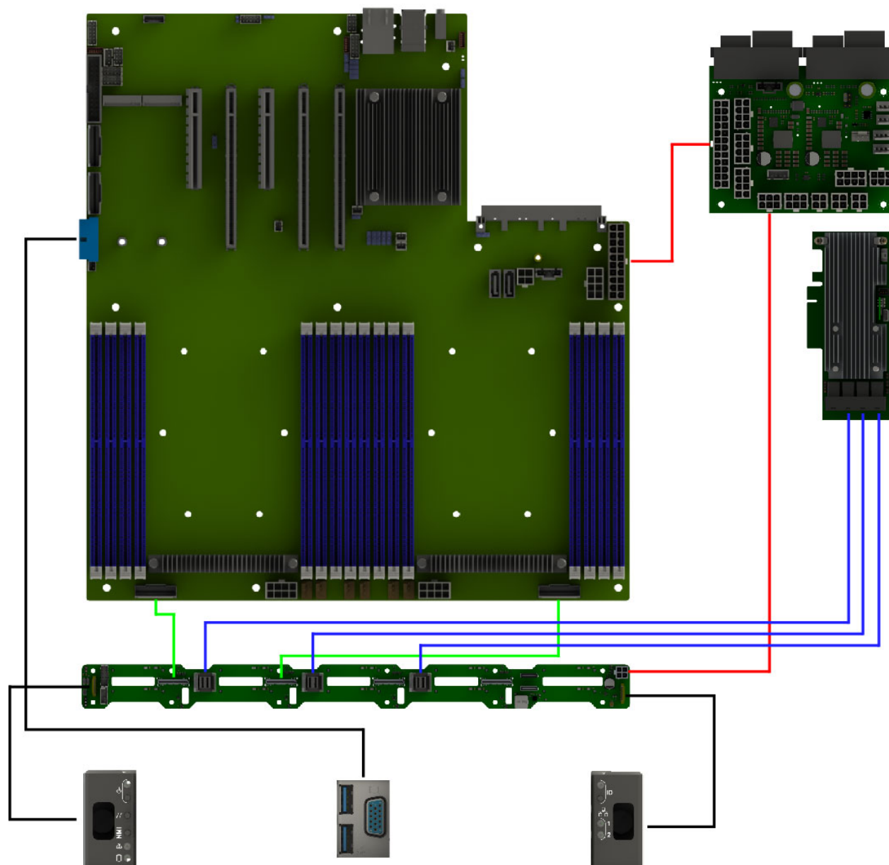
Рис. 30. Схема прокладки системных кабелей и кабелей Oculink-SLIMline X8-X8 с подключением PCIe RAID
