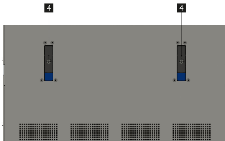
Рис. 23. Установка верхней крышки сервера
