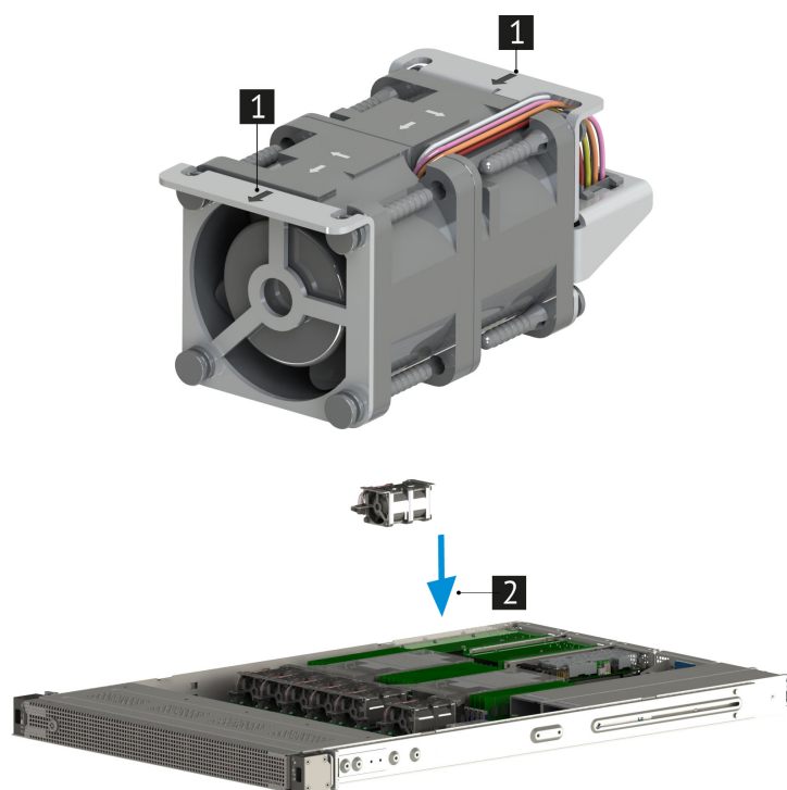
Рис. 32. Подключение вентилятора
