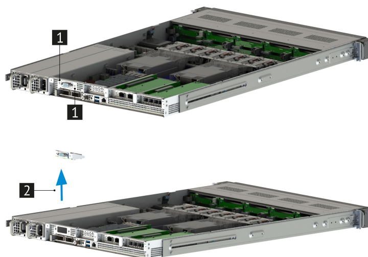
Рис. 58. Извлечение карты VGA
