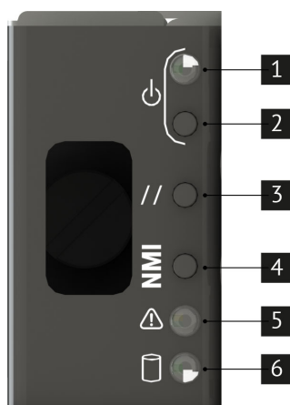
Рис. 4. Левая панель управления
