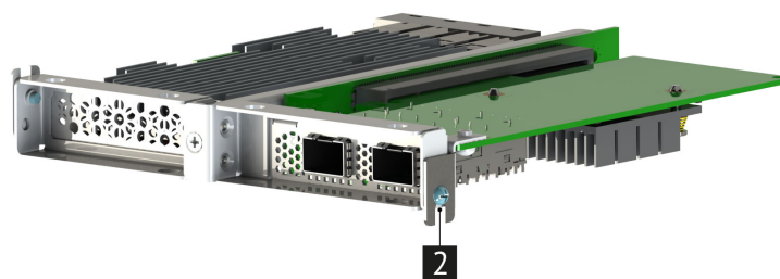
Рис. 57. Установка карты расширения
