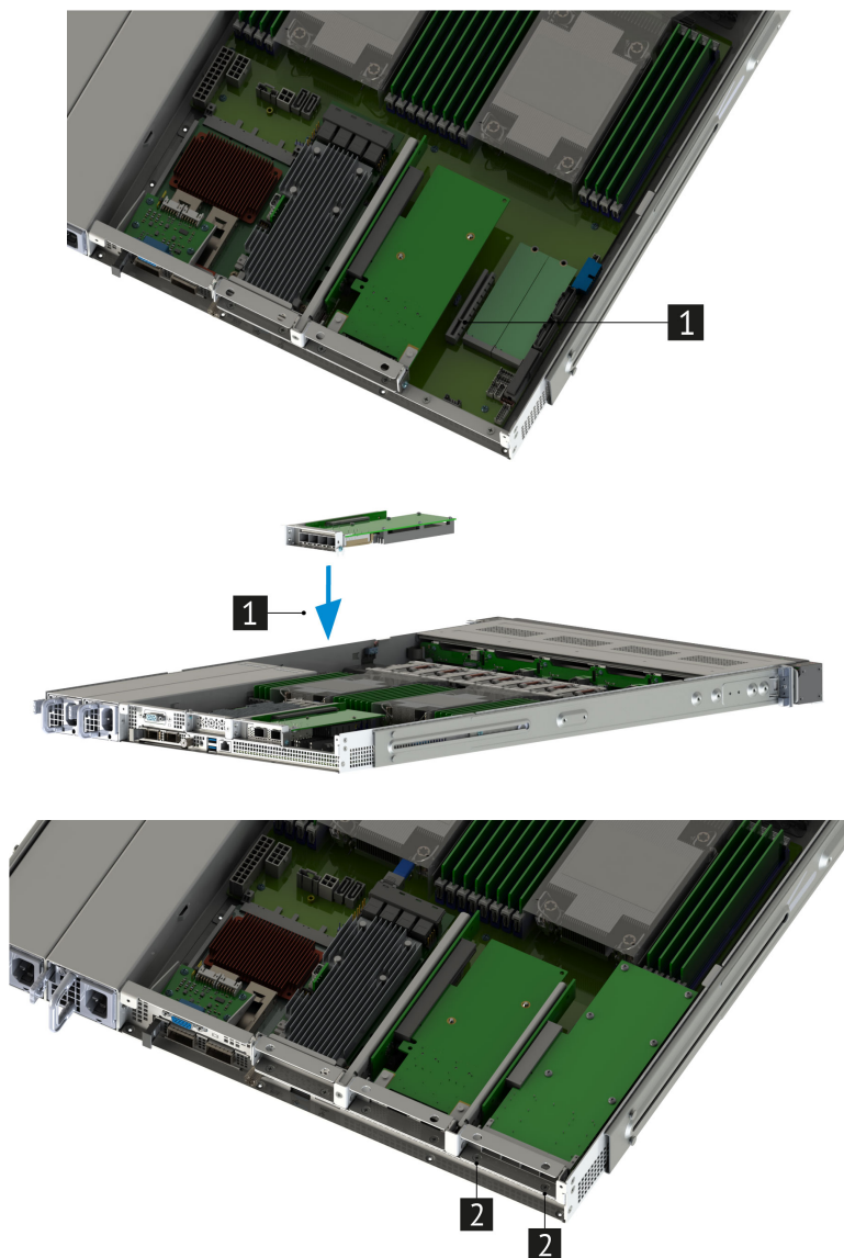
Рис. 49. Установка райзера PCIe 1U x8-x8
