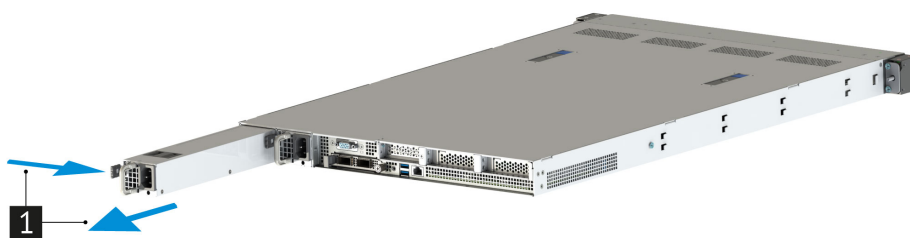
Рис. 63. Извлечение блока питания из сервера
