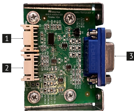
Рис. 15. Плата VGA (НИКА.468349.001)
