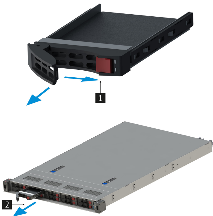
Рис. 43. Извлечение дисков
