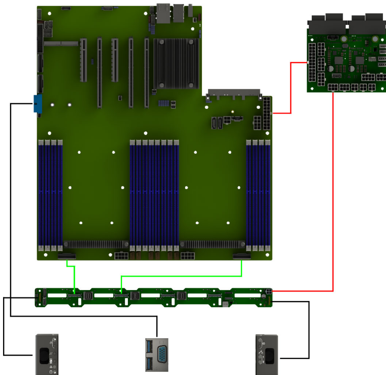
Рис. 29. Схема прокладки системных кабелей и кабелей Oculink-SLIMline X8-X8
