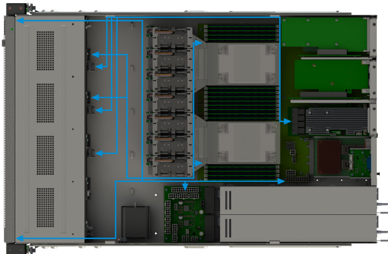
Рис. 26. Схема прокладки кабелей в сервере
