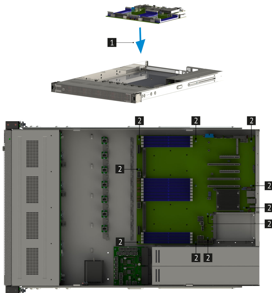
Рис. 42. Установка материнской платы в сервер
