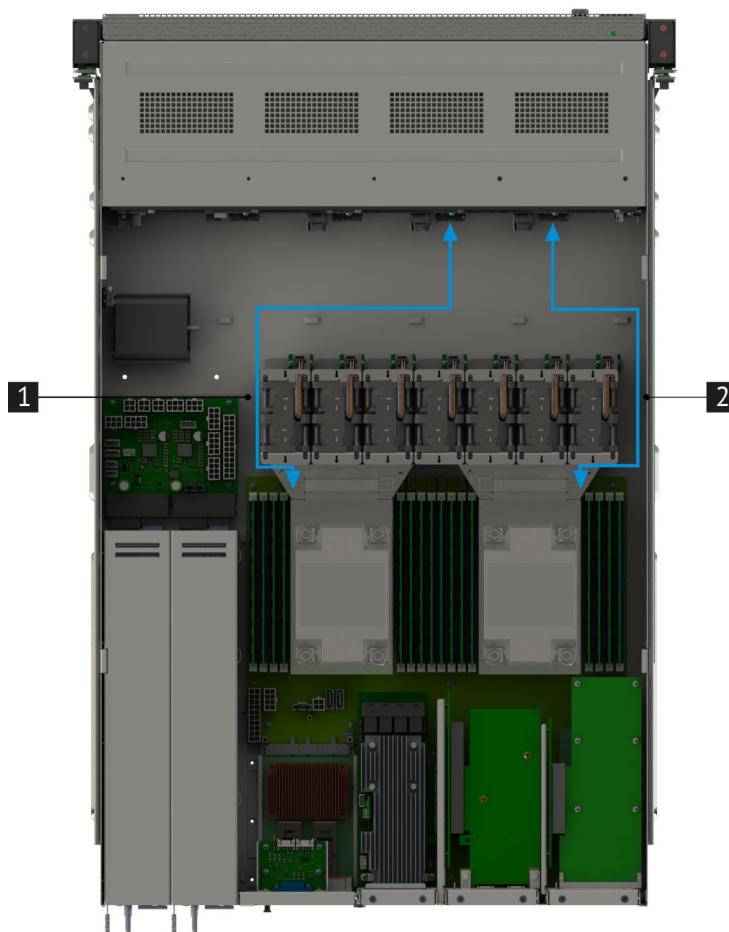
Рис. 46. Схема прокладки кабелей Oculink-SLIMline X8-X8
