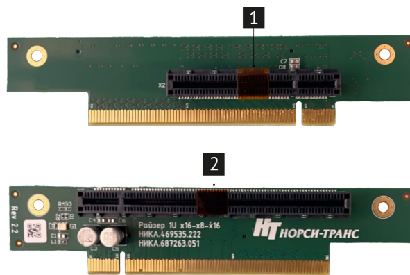
Рис. 14. Райзер 1U x16-x8-x16 (НИКА.469535.222)
