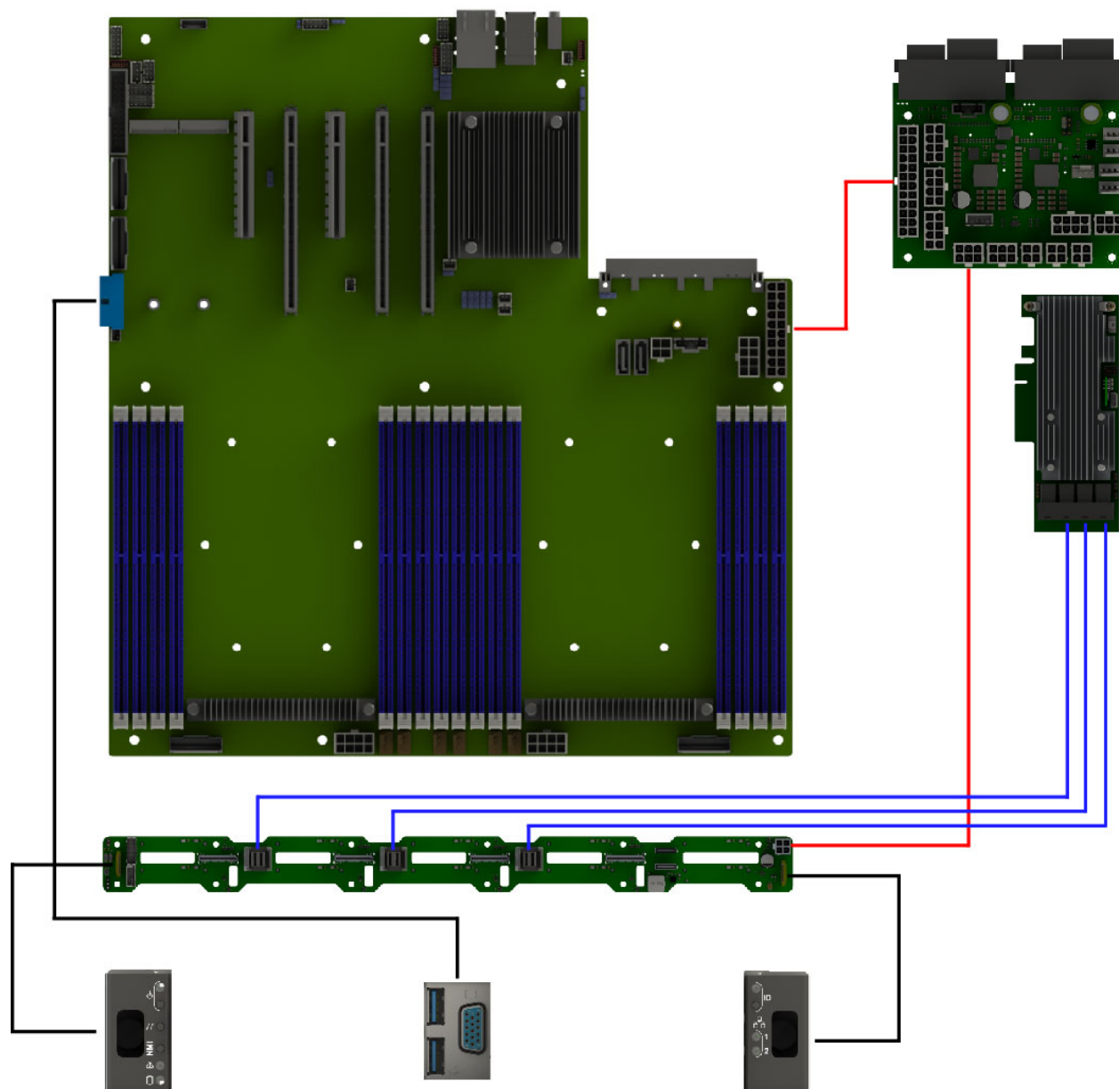
Рис. 28. Схема прокладки системных кабелей и кабелей питания с подключением PCIe RAID
