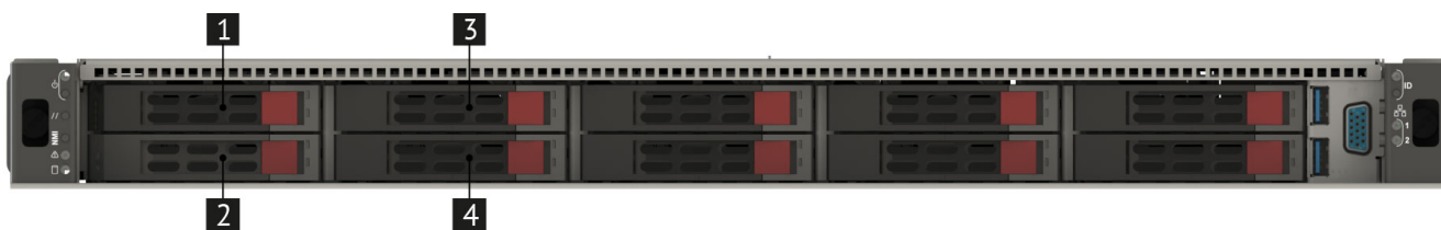
Рис. 47. Место установки NVMe-дисков в сервер
