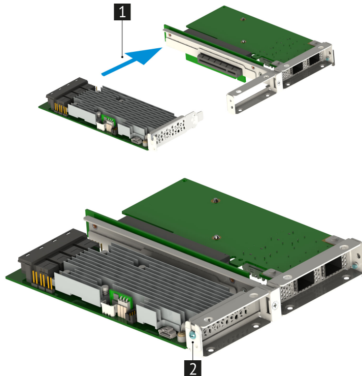
Рис. 53. Установка контроллера дискового MegaRAID 9361-16i
