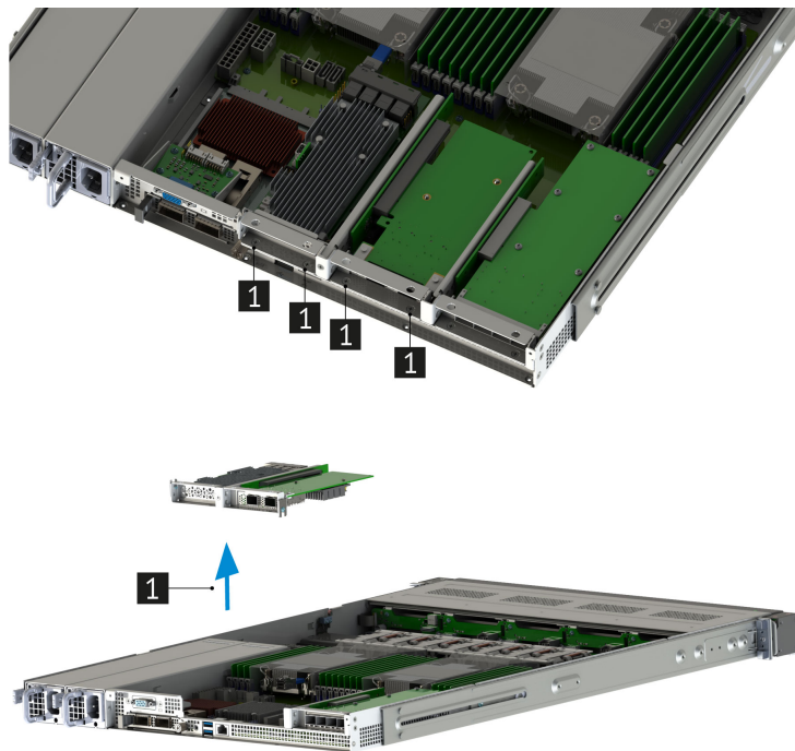
Рис. 50. Извлечение райзера PCIe 1U x16-x8-x16
