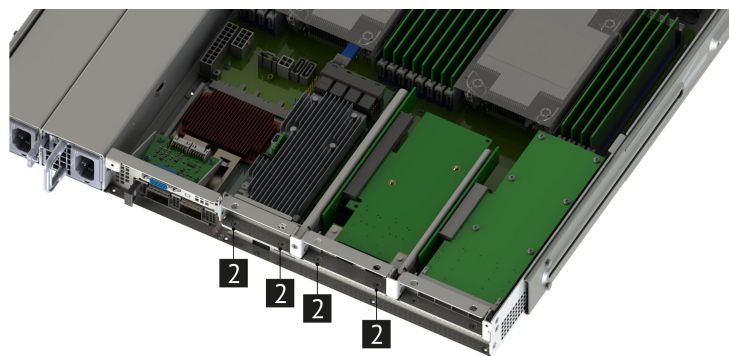
Рис. 51. Установка райзера PCIe 1U x16-x8-x16
