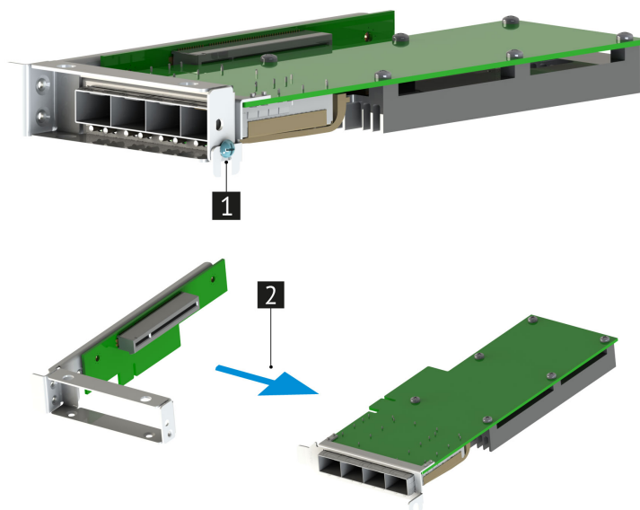
Рис. 54. Извлечение карты расширения
