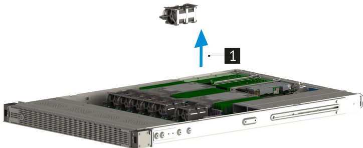
Рис. 31. Извлечение вентилятора из сервера
