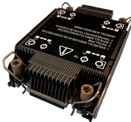
Рис. 36. Радиатор для сервера
