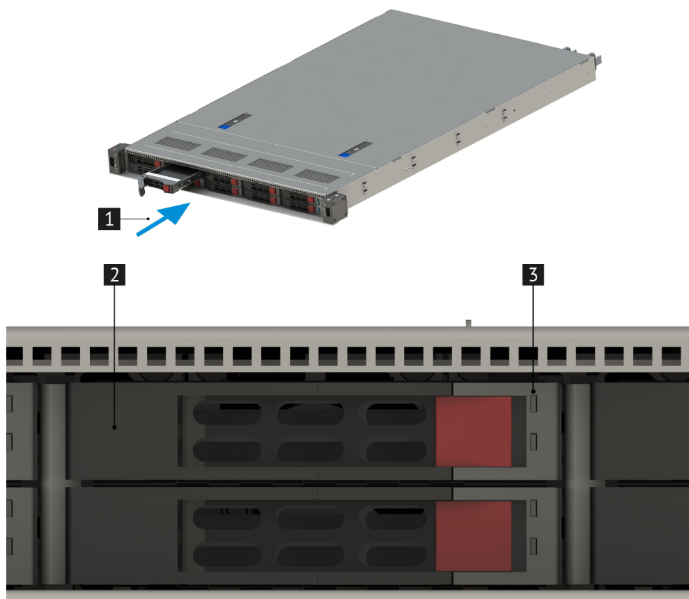
Рис. 44. Установка дисков
