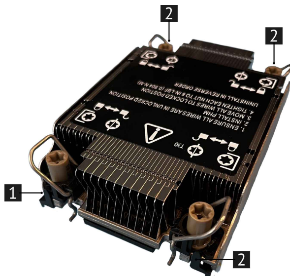
Рис. 38. Снятие процессора с радиатора
