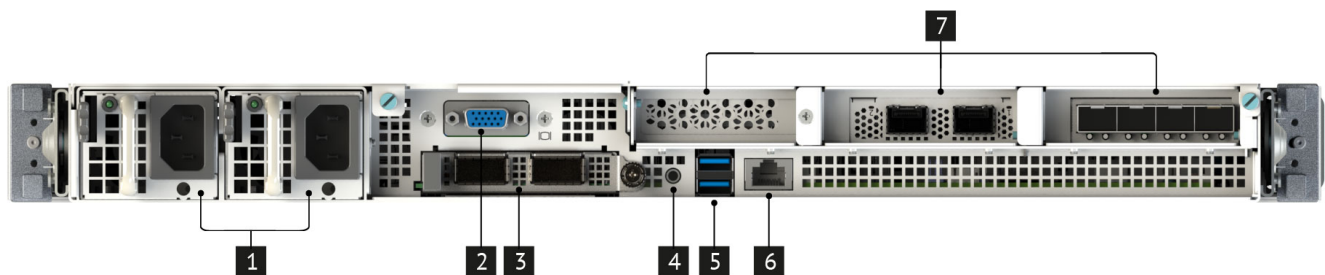
Рис. 6. Вид сервера сзади
