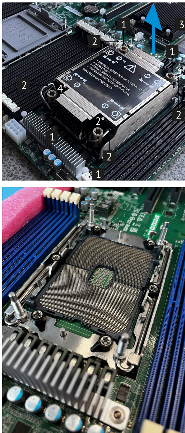
Рис. 37. Снятие модуля процессора с радиатором
