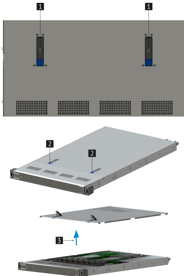
Рис. 22. Снятие верхней крышки сервера
