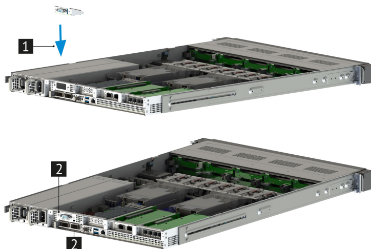
Рис. 59. Установка карты VGA
