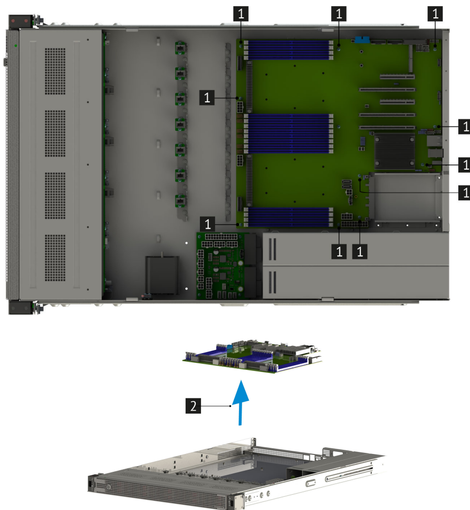
Рис. 41. Извлечение материнской платы из сервера
