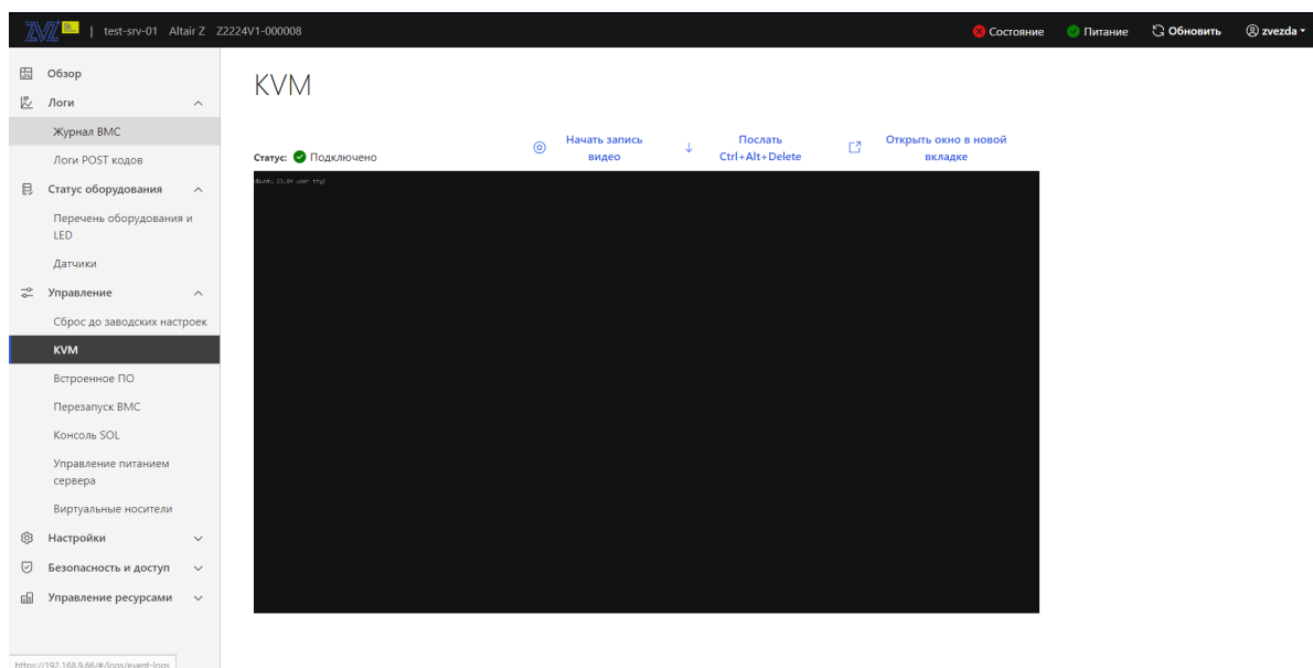
Рис. 83. Окно «KVM»
