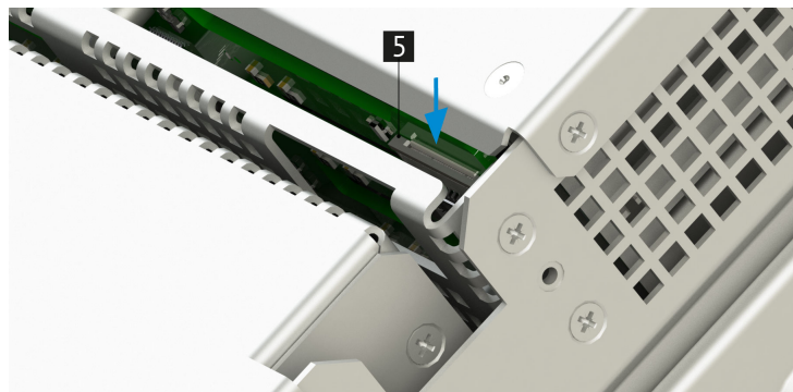
Рис. 47. Соединитель пленочного кабеля.
