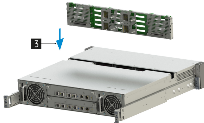
Рис. 45. Установка рамы с платой объединительной 25SFF
