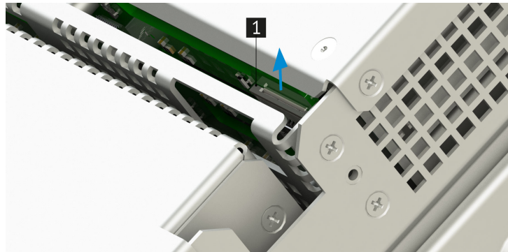
Рис. 38. Соединитель пленочного кабеля.
