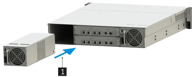
Рис. 52. Установка блока питания
