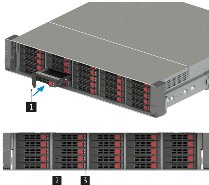
Рис. 37. Установка диска SATA
