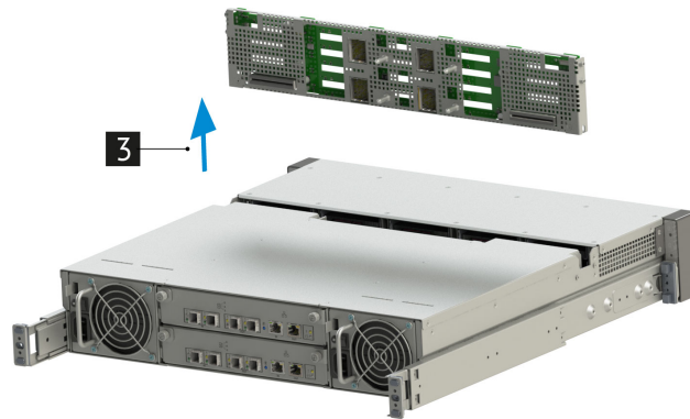
Рис. 40. Извлечение рамы с платой объединительной 25SFF
