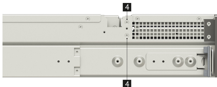
Рис. 46. Винты фиксирующие раму с платой объединительной 25SFF в дисковом массиве.
