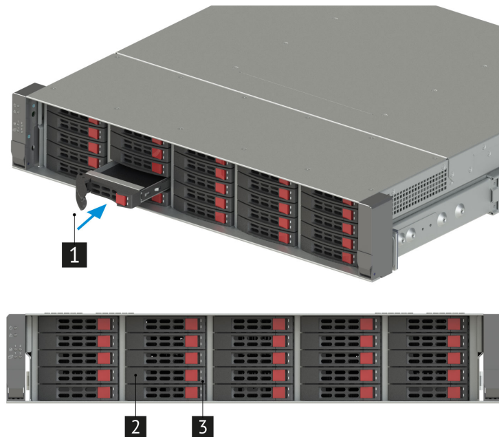
Рис. 35. Установка дисков
