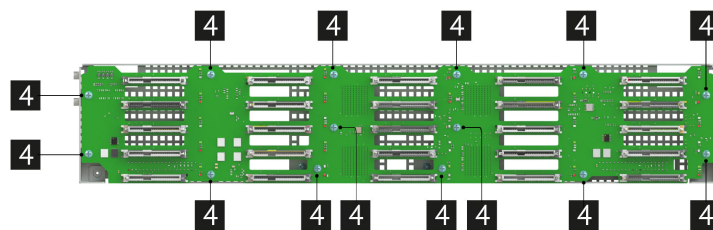
Рис. 41. Винты фиксирующие плату объединительную 25SFF
