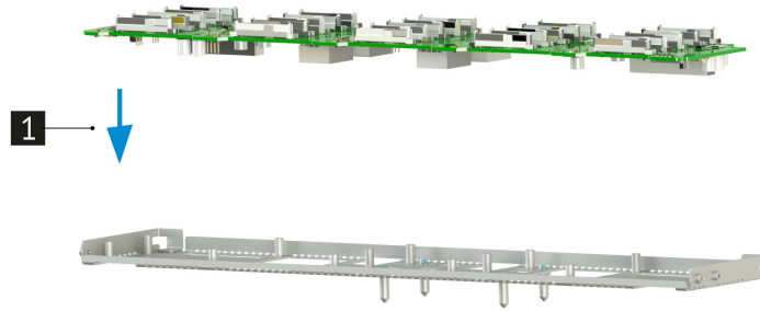
Рис. 43. Установка платы объединительной 25SFF
