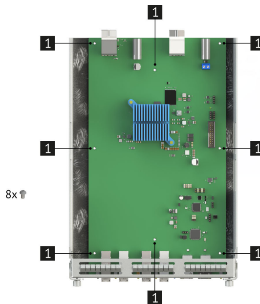
Рис. 30. Винты фиксирующие плату SAS-экспандера.
