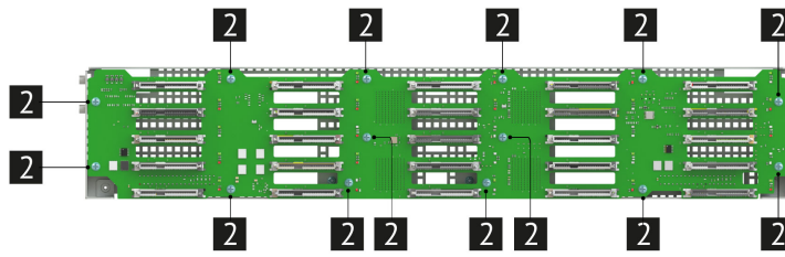
Рис. 44. Винты фиксирующие плату объединительную 25SFF.
