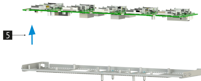
Рис. 42. Извлечение платы объединительной 25SFF
