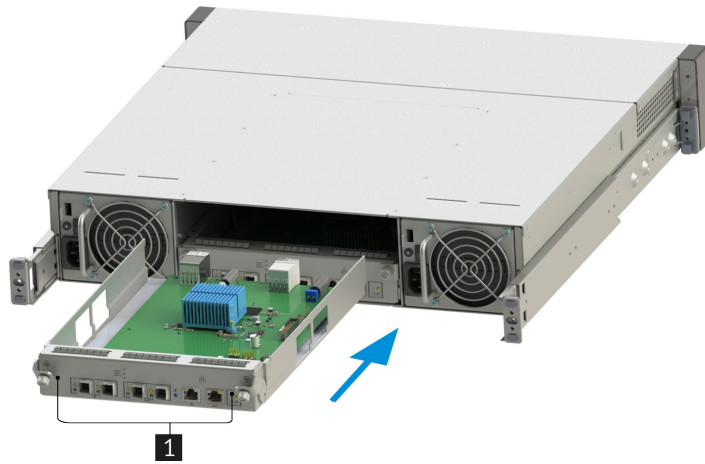
Рис. 27. Установка модуля SAS-экспандера №2 в дисковый массив
