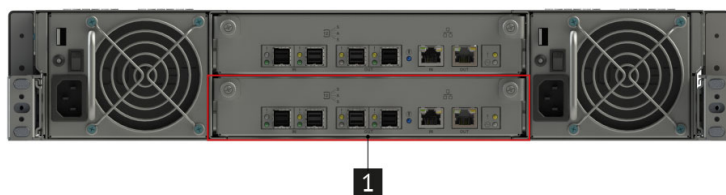
Рис. 36. Установленный модуль SAS-экспандера №1
