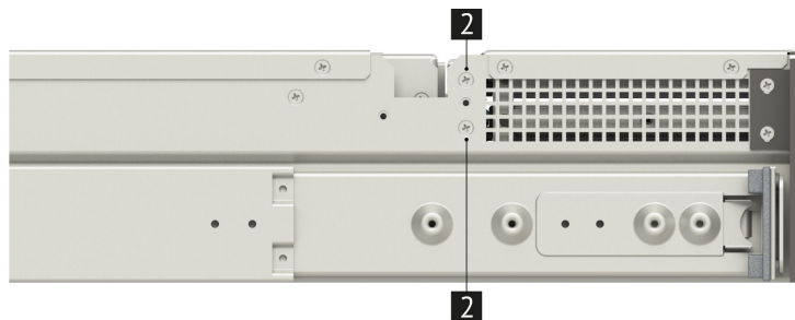
Рис. 39. Винты фиксирующие раму с платой объединительной 25SFF в дисковом массиве.
