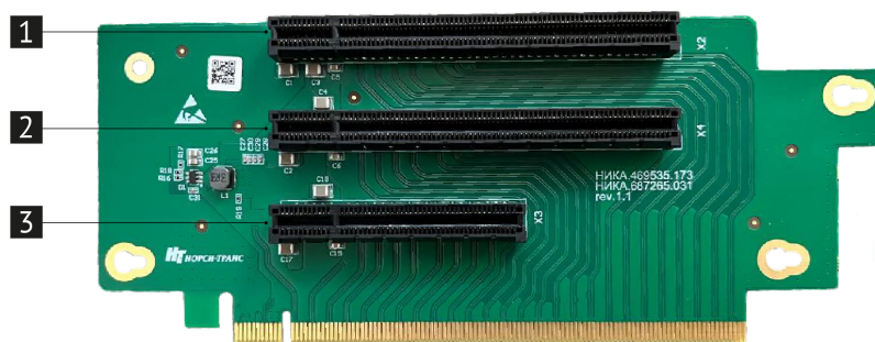
Рис. 19. Райзер 1x24-16-16-8 (НИКА.469535.173)
