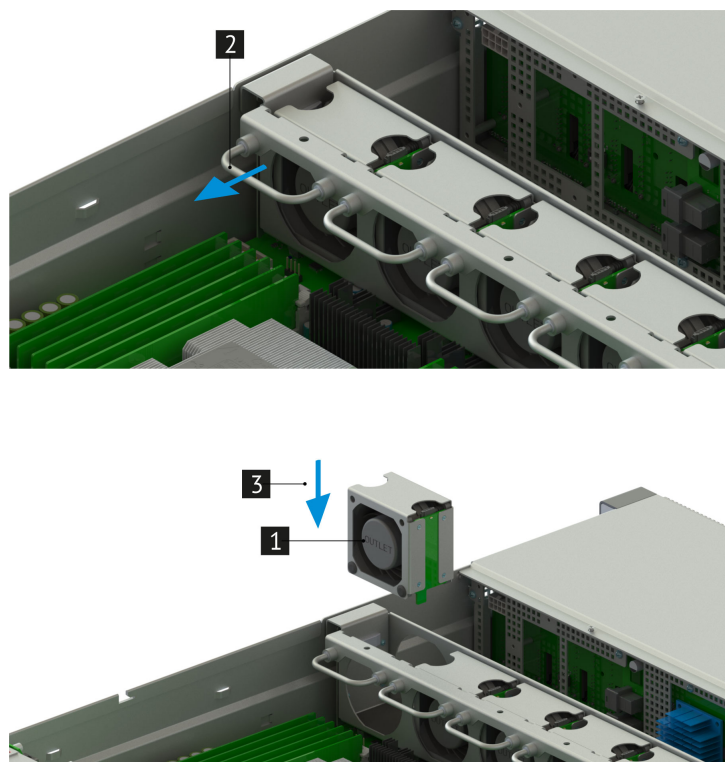
Рис. 37. Подключение вентилятора
