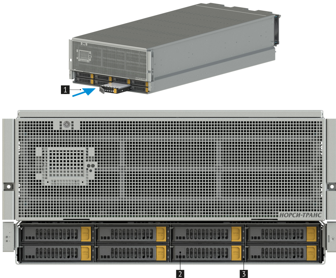
Рис. 44. Установка дисков
