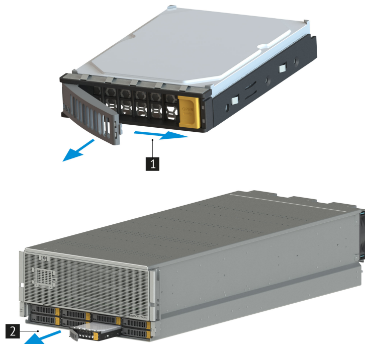
Рис. 43. Извлечение дисков
