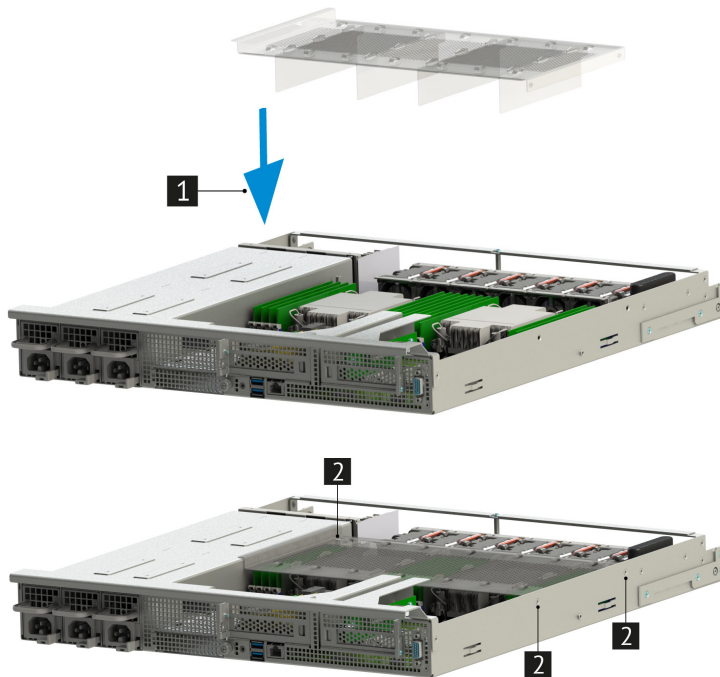
Рис. 25. Установка воздушного кожуха
