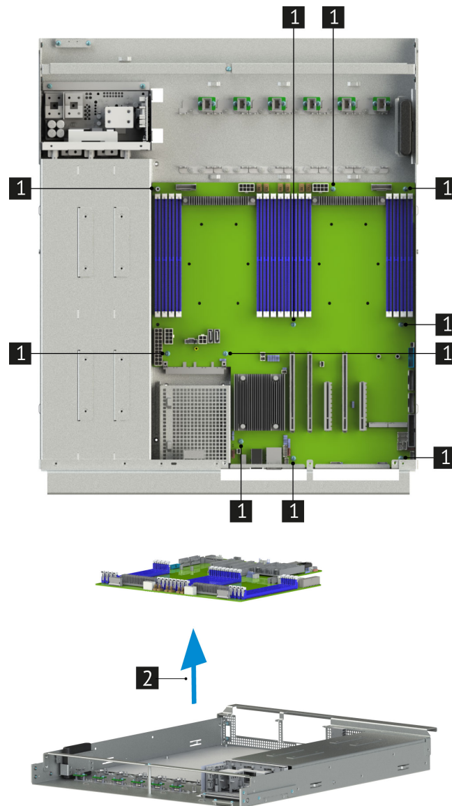
Рис. 41. Извлечение материнской платы из сервера
