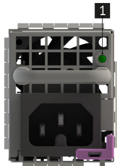
Рис. 57. Светодиодная индикация состояния блока питания
