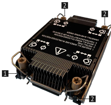
Рис. 38. Снятие процессора с радиатора
