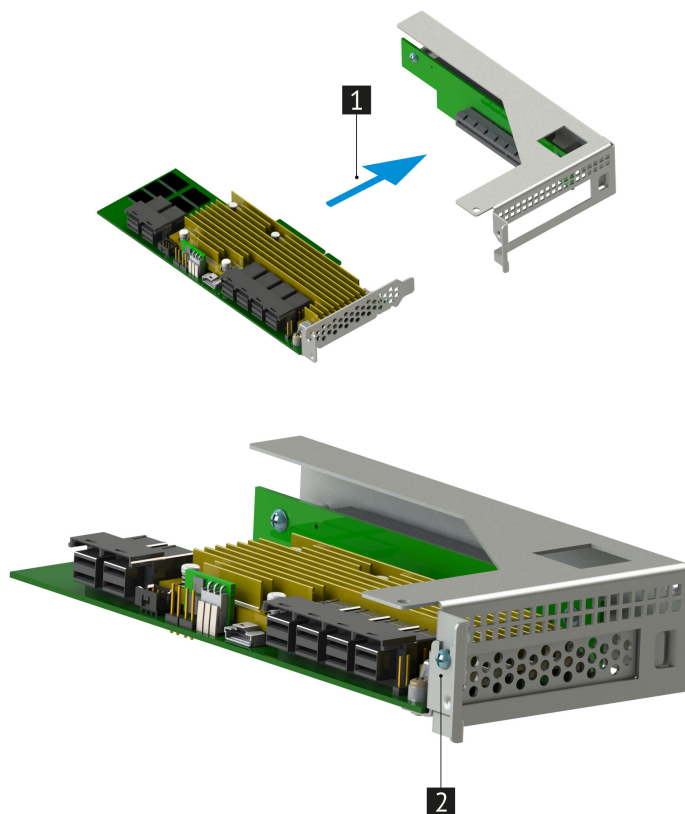
Рис. 52. Установка контроллера дискового MegaRAID 9361-24i
