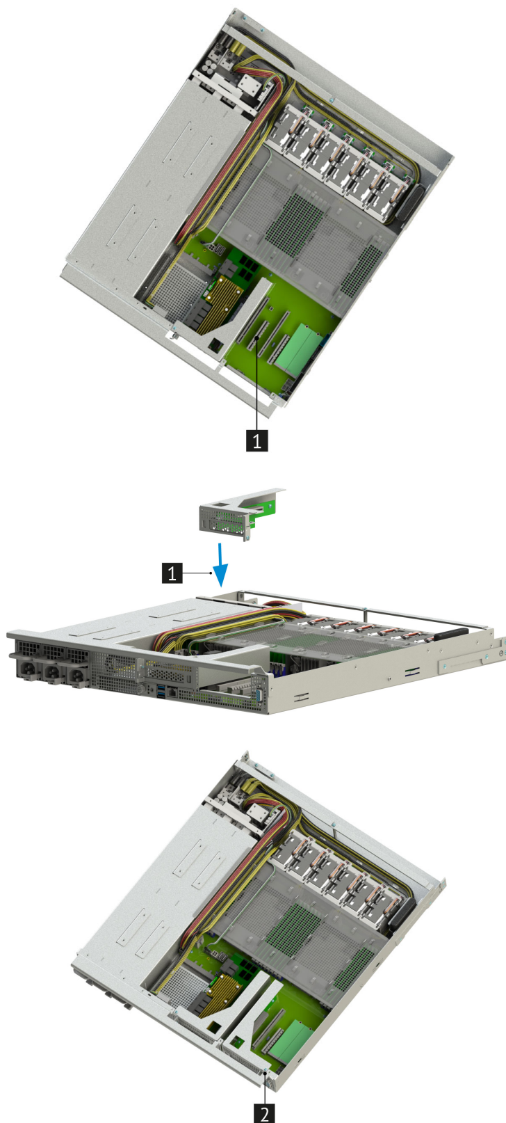
Рис. 48. Установка райзера PCIe 1U x8-x8
