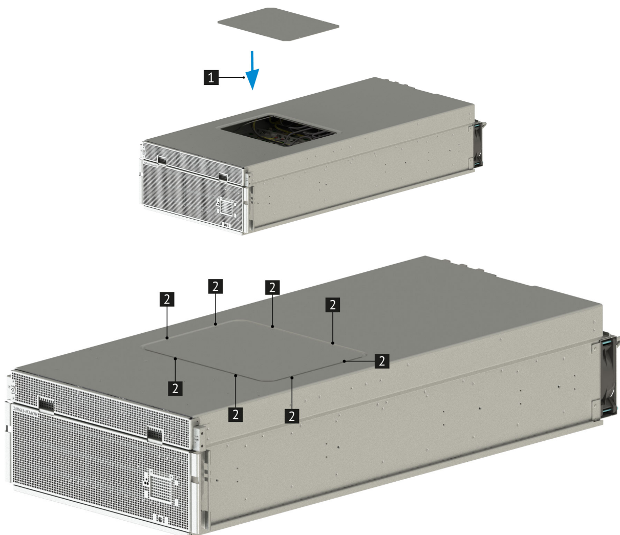
Рис. 56. Установка технологической панели
