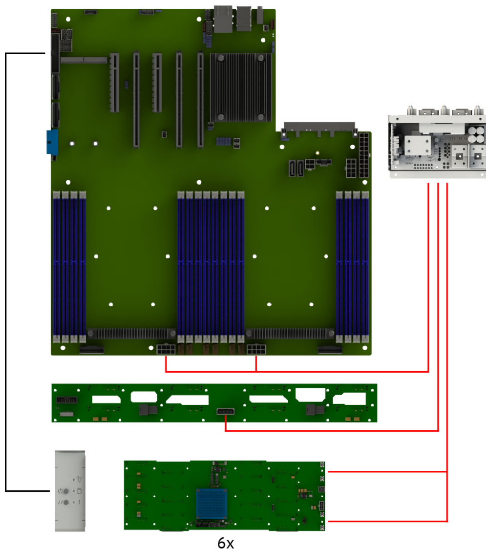
Рис. 27. Схема прокладки системных кабелей и кабелей питания
