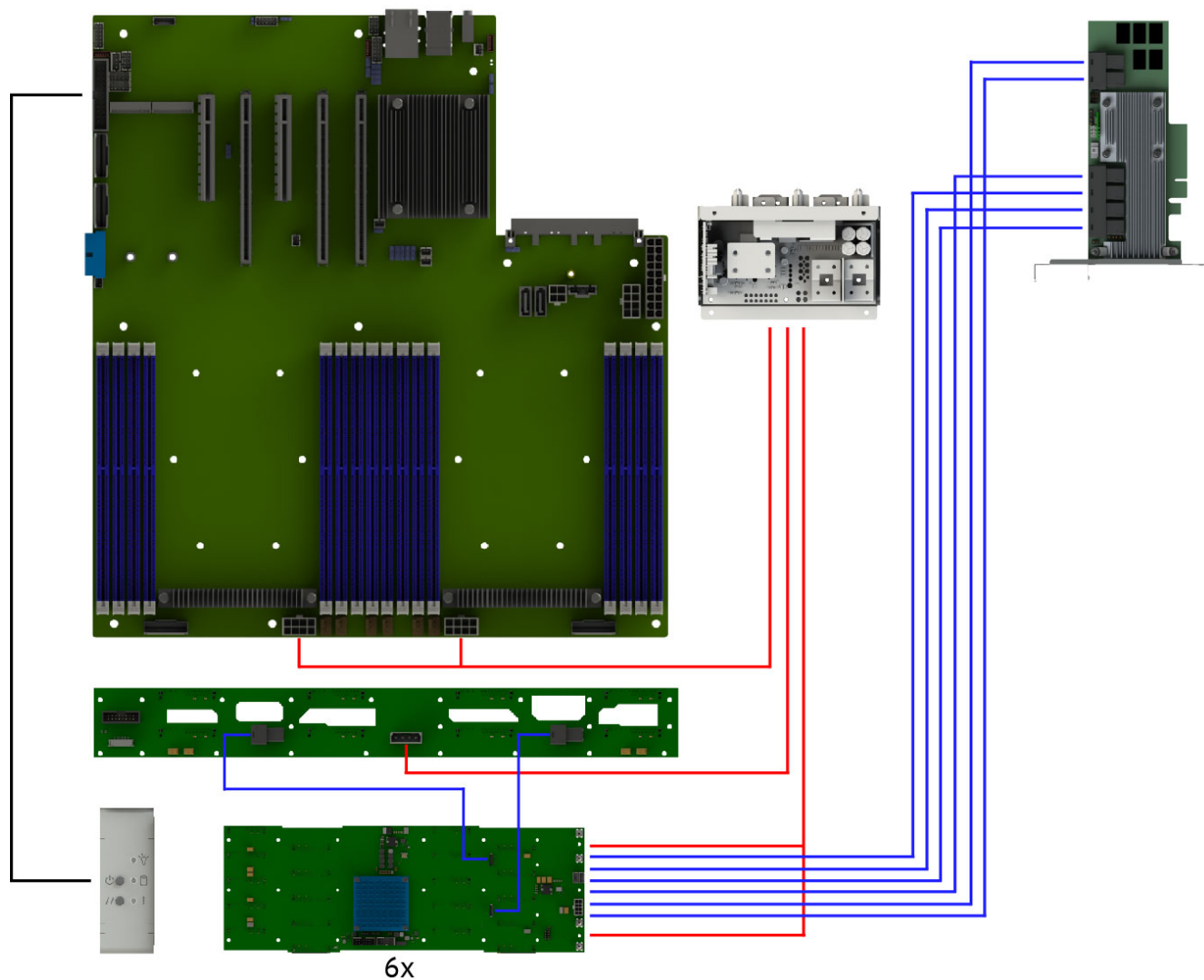
Рис. 28. Схема прокладки системных кабелей и кабелей питания с подключением PCIe RAID
