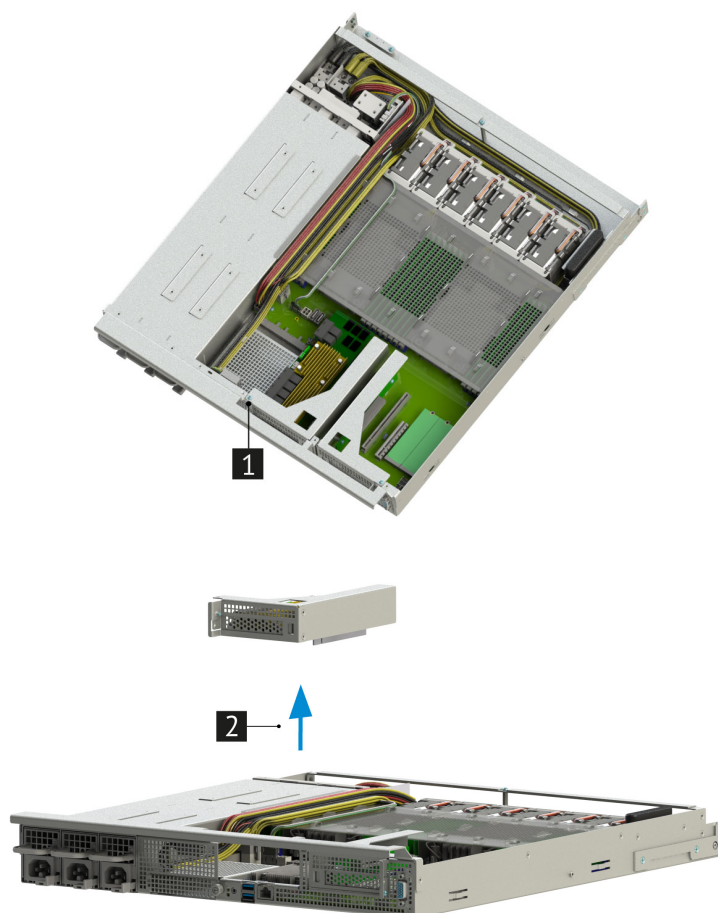
Рис. 49. Извлечение райзера PCIe 1U x16-x8-x16
