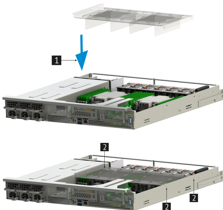
Рис. 25. Установка воздушного кожуха
