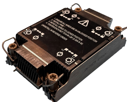
Рис. 36. Радиатор для сервера
