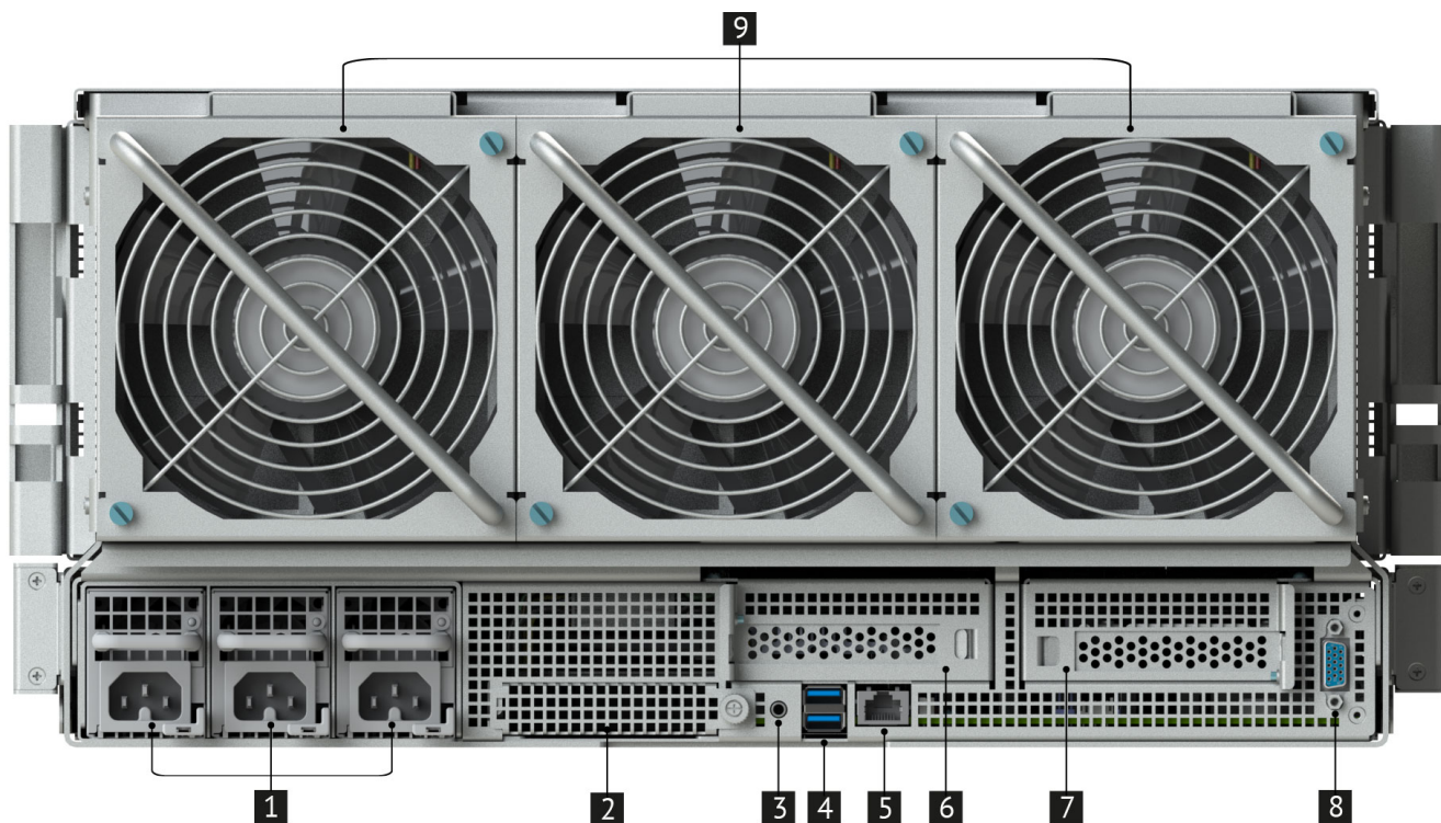
Рис. 4. Вид сервера сзади
