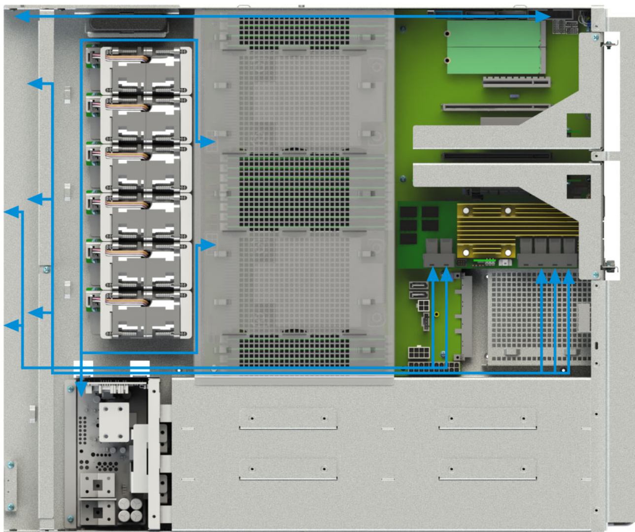
Рис. 26. Схема прокладки кабелей в модуле НИКА.467239.008 сервера
