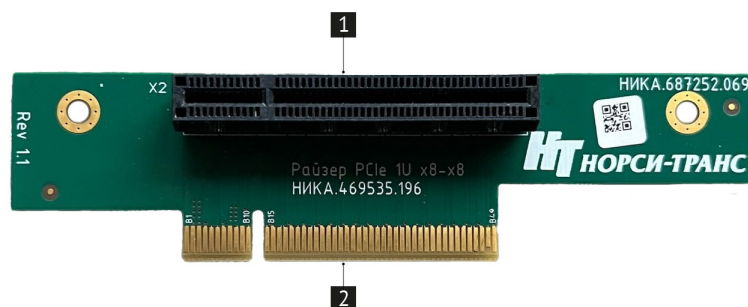
Рис. 12. Райзер PCIe 1U x8-x8 (НИКА.469535.196)
