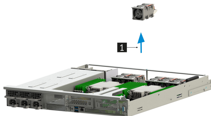
Рис. 29. Извлечение вентилятора из сервера
