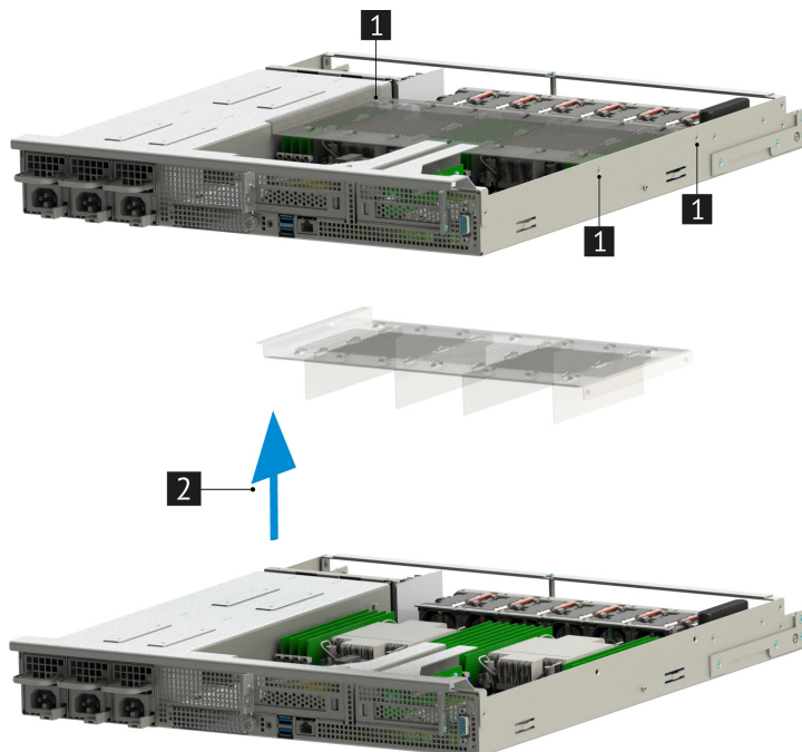
Рис. 24. Извлечение воздушного кожуха
