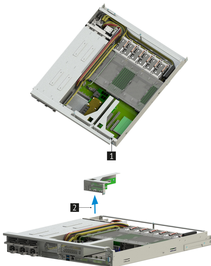
Рис. 47. Извлечение райзера PCIe 1U x8-x8
