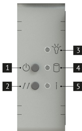
Рис. 3. Левая панель управления
