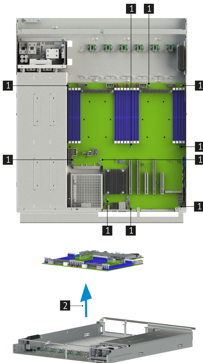
Рис. 41. Извлечение материнской платы из сервера
