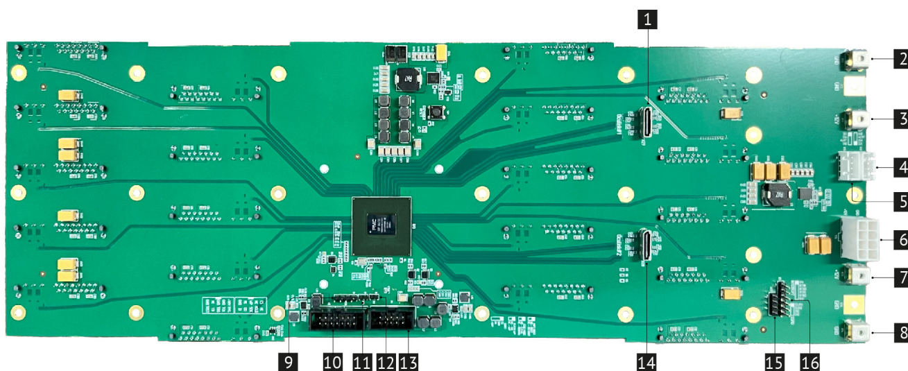
Рис. 10. Плата дискового массива (НИКА.469535.115)
