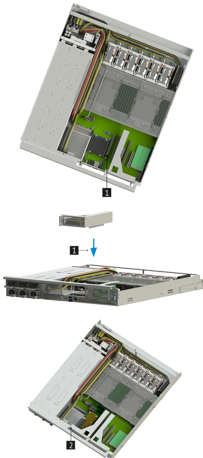
Рис. 50. Установка райзера PCIe 1U x16-x8-x16
