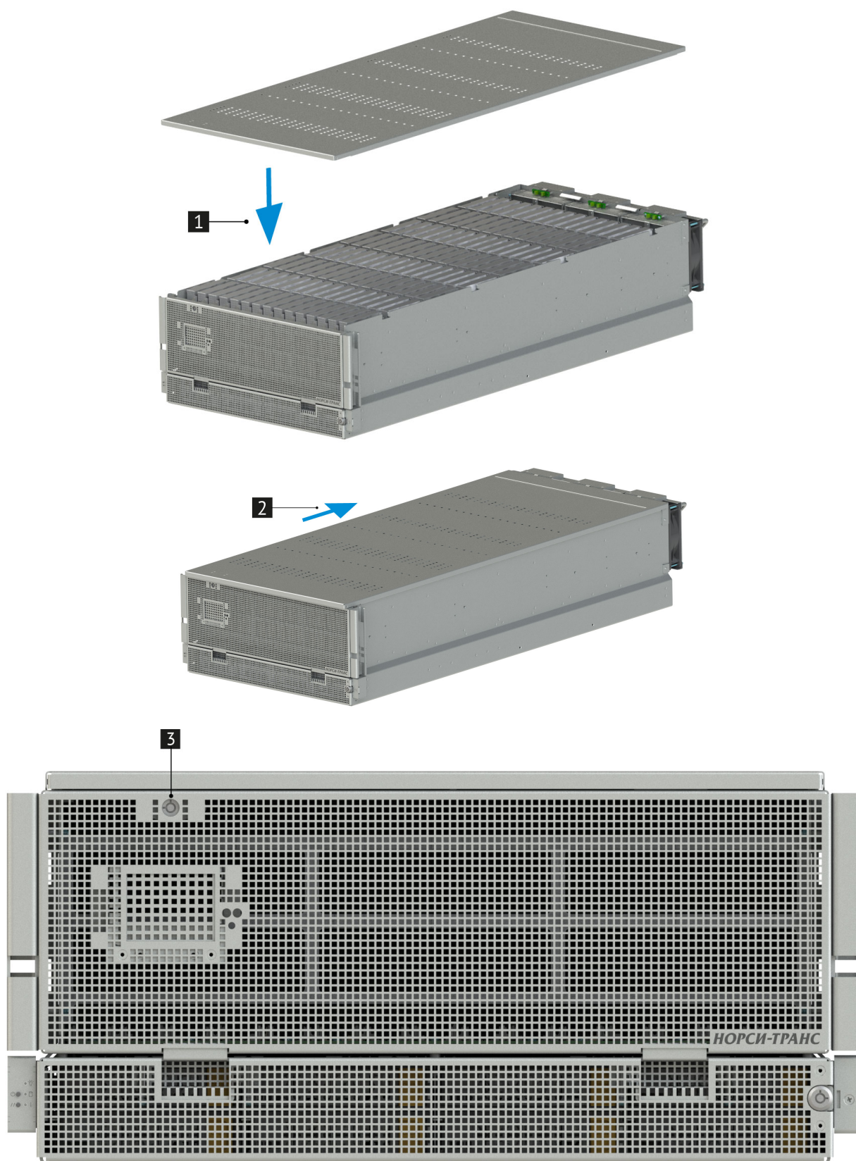
Рис. 21. Установка верхней крышки платформы
