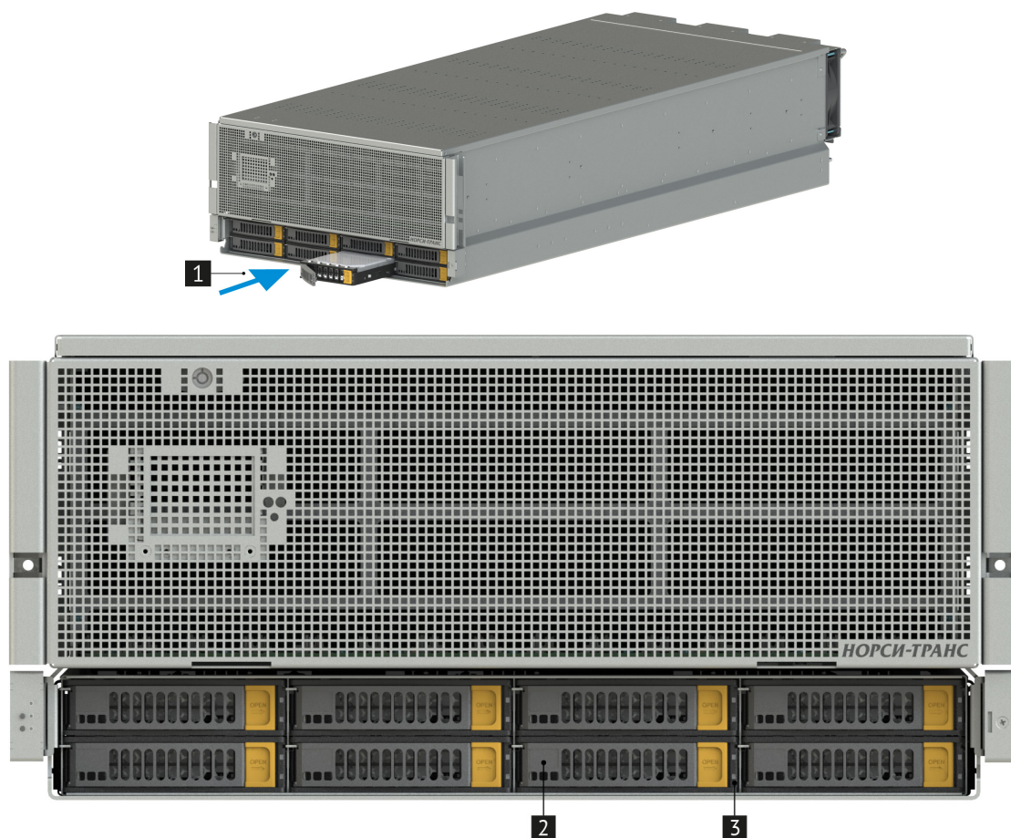
Рис. 44. Установка дисков
