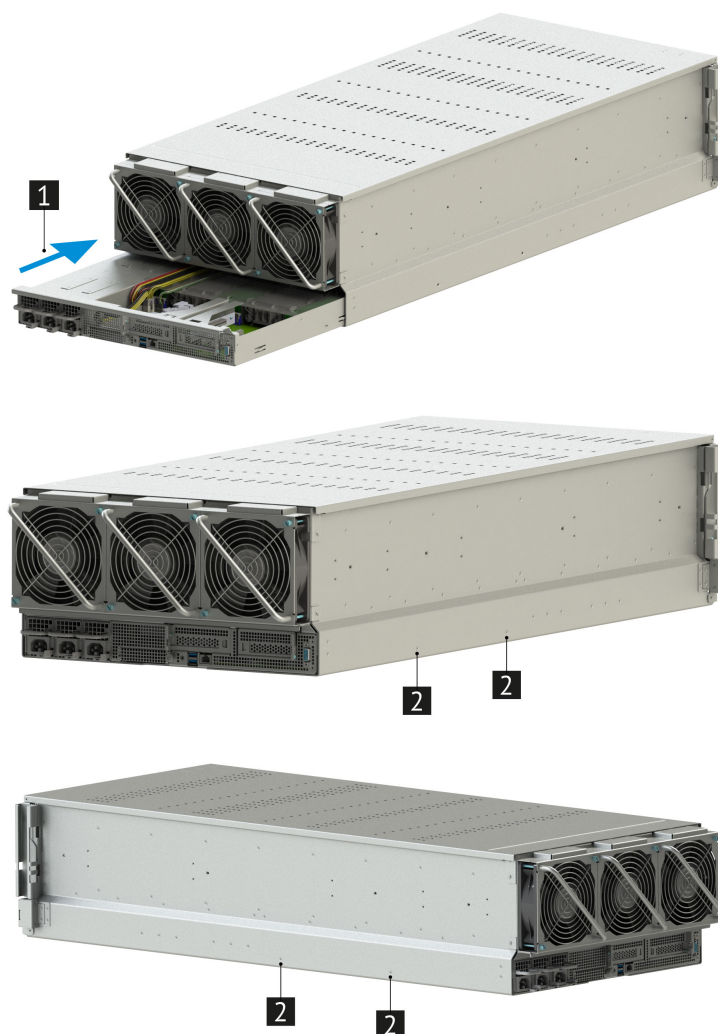
Рис. 23. Установка модуля НИКА.467239.008
