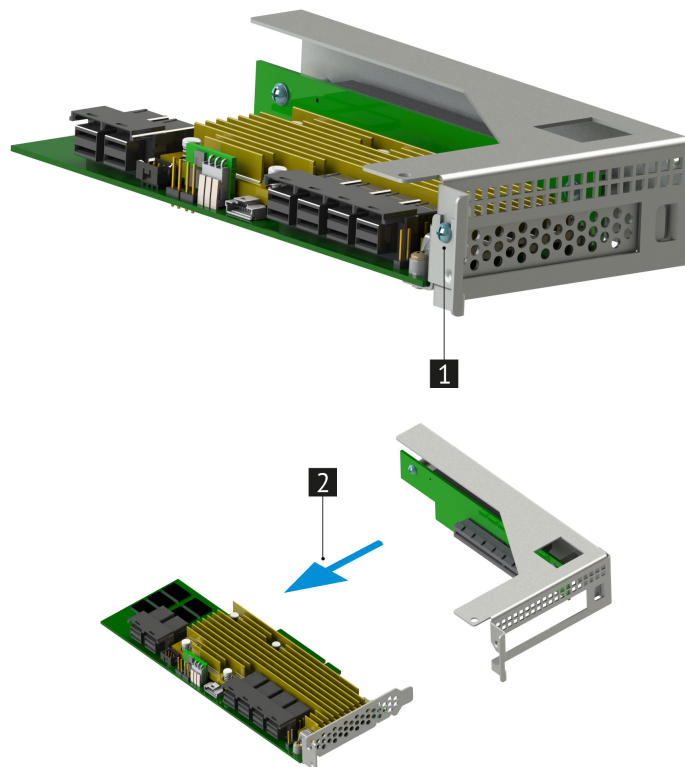
Рис. 51. Извлечение контроллера дискового MegaRAID 9361-24i
