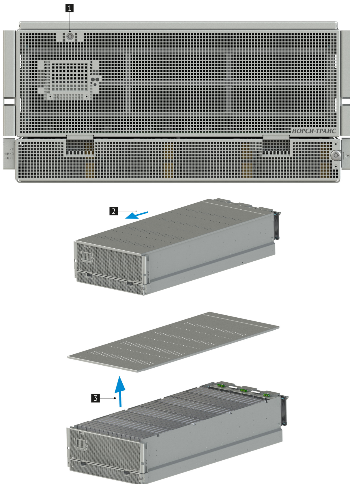
Рис. 20. Снятие верхней крышки платформы
