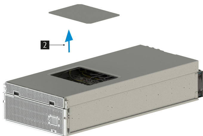
Рис. 55. Снятие технологической панели
