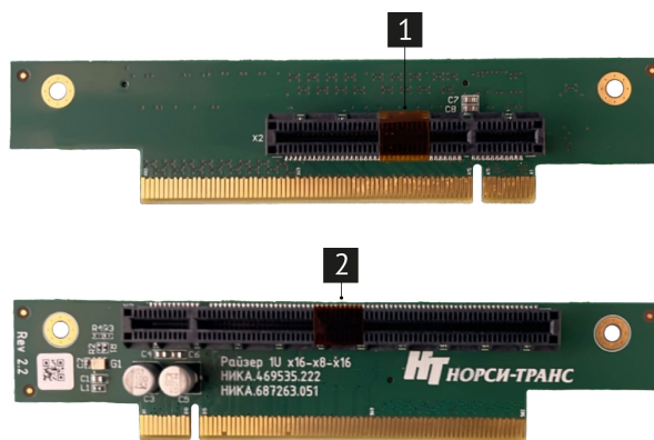
Рис. 13. Райзер PCIe 1U x16-x8-x16 (НИКА.469535.222)
