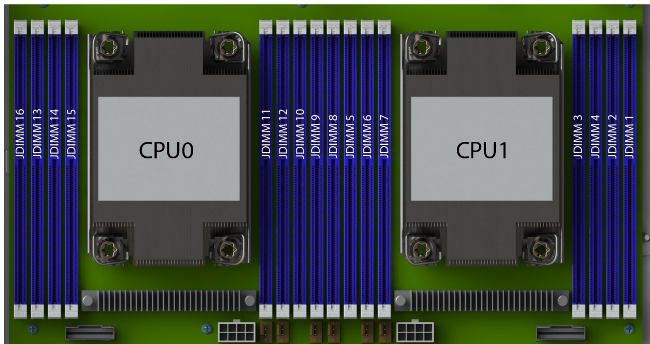
Рис. 33. Расположение разъемов
