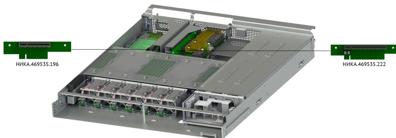
Рис. 11. Расположение PCIe-райзеров в модуле НИКА.467239.008 сервера
