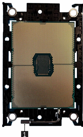
Рис. 39. Снятие процессора с радиатора
