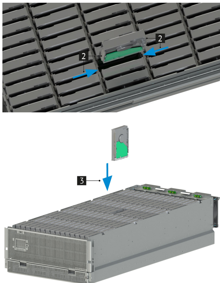
Рис. 46. Установка диска в массив дисков
