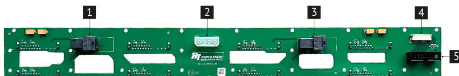
Рис. 9. Плата дискового массива A8 (НИКА.469535.013)
