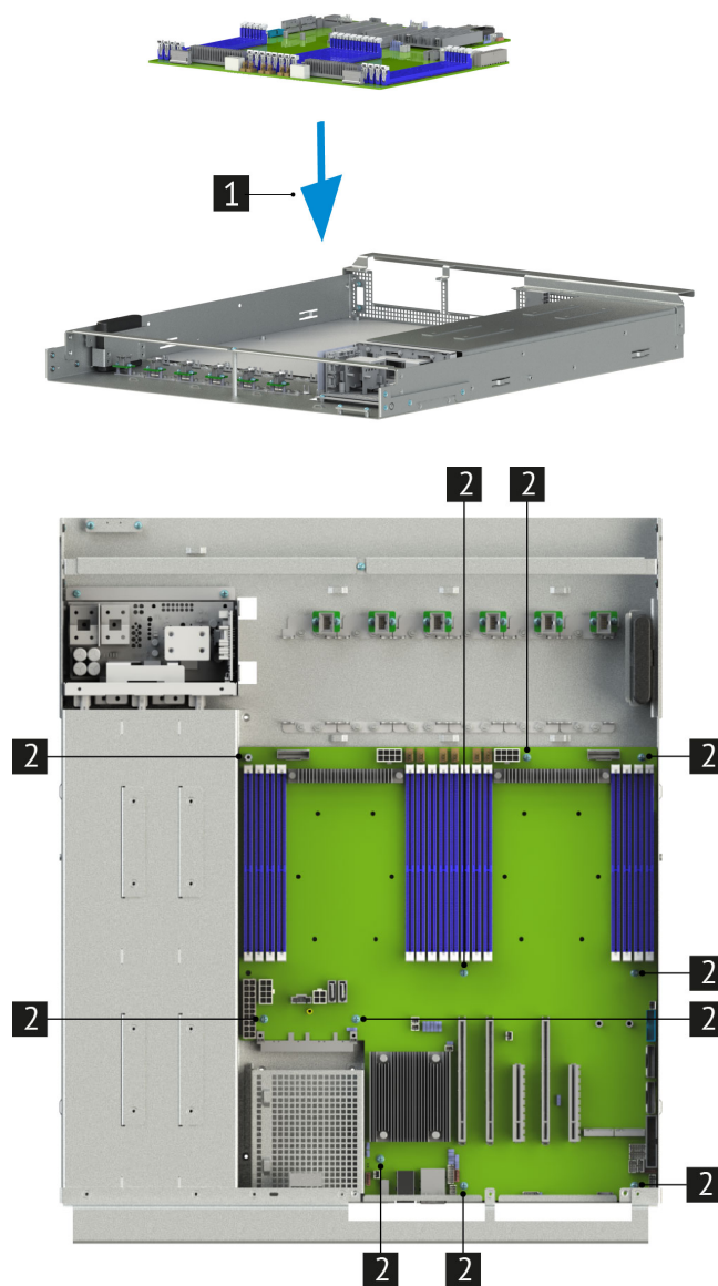
Рис. 42. Установка материнской платы в сервер
