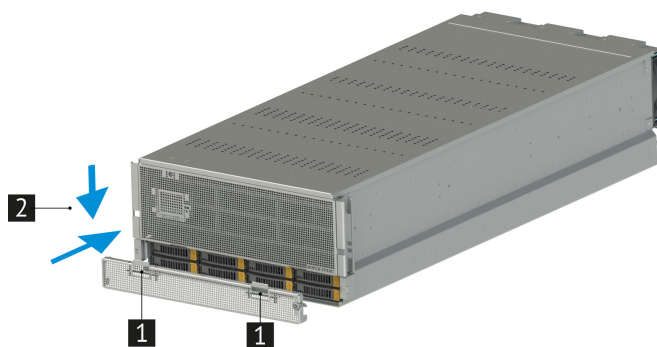
Рис. 18. Установка передней панели
