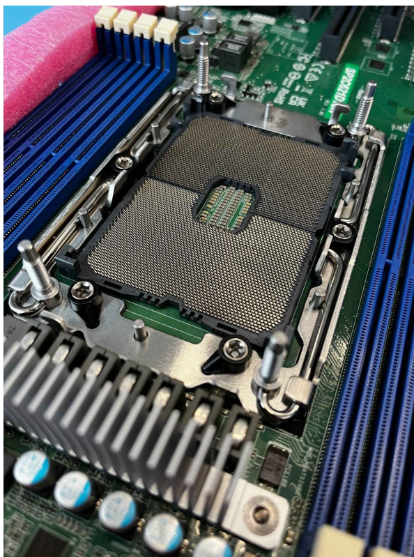
Рис. 37. Снятие модуля процессора с радиатором
