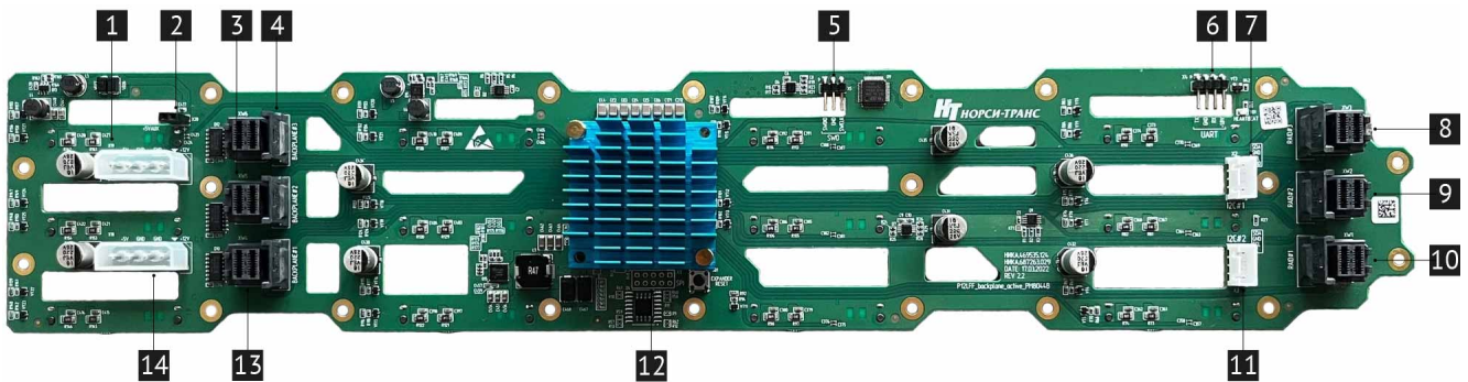
Рис. 14. Плата расширения 12LFF (НИКА.469535.124)
