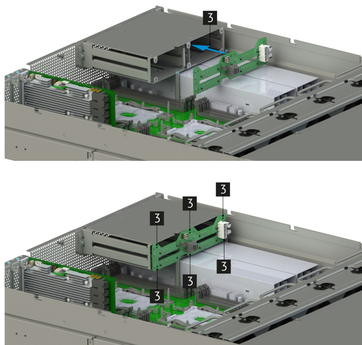
Рис. 23. Установка каркаса НИКА.301233.012
