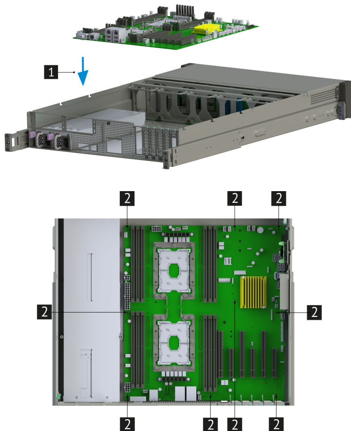
Рис. 40. Установка материнской платы
