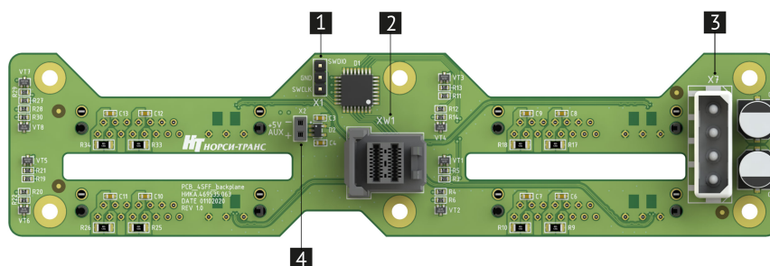
Рис. 13. Плата расширения 4SFF (НИКА.469535.063)
