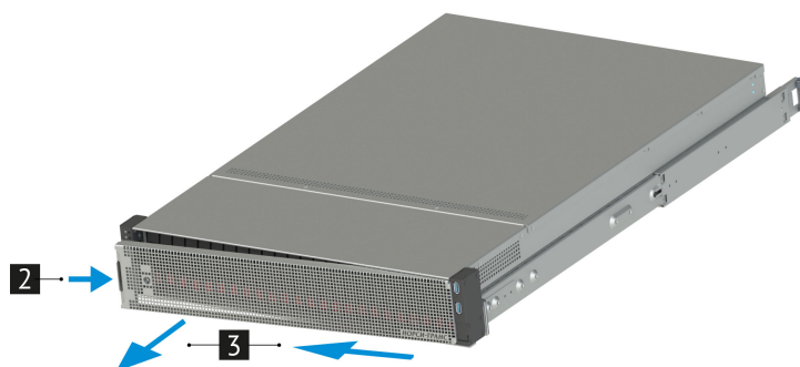
Рис. 17. Снятие передней панели
