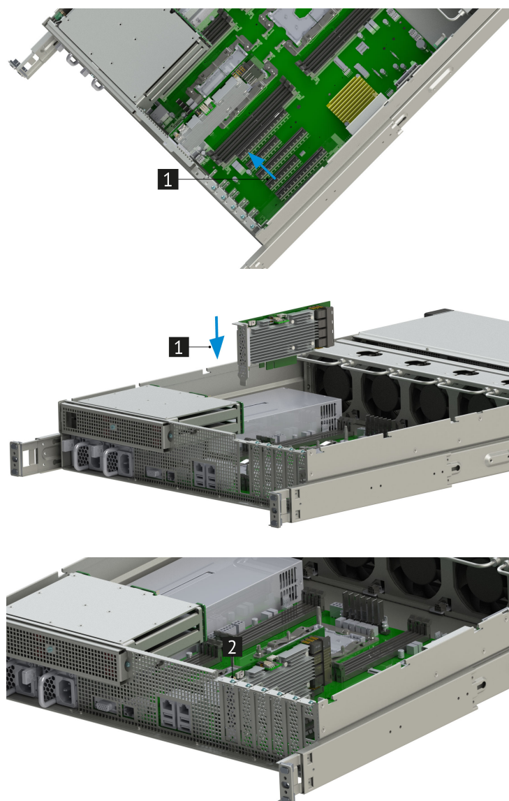
Рис. 46. Установка MegaRAID SAS 9361-16i
