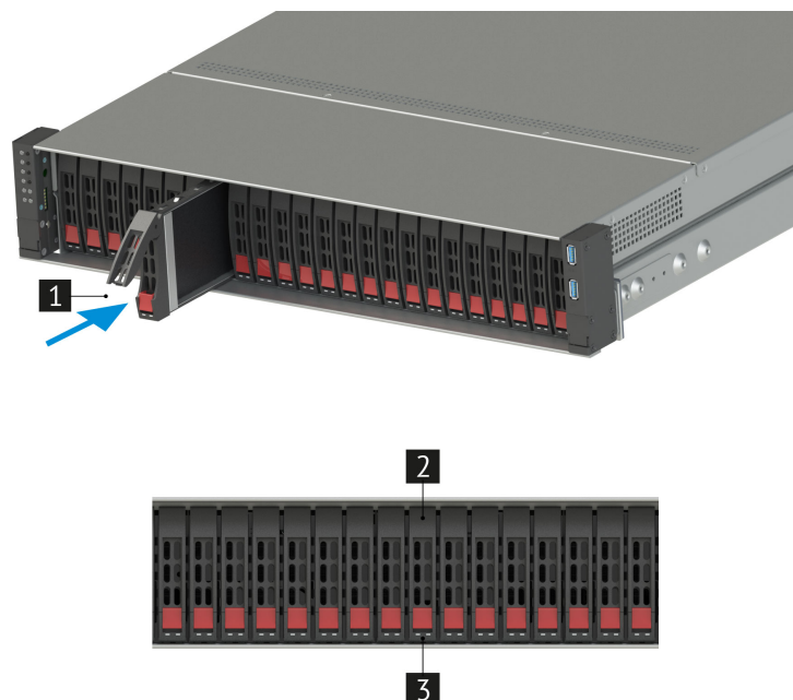
Рис. 42. Установка дисков
