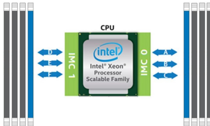
Рис. 29. Каналы памяти
