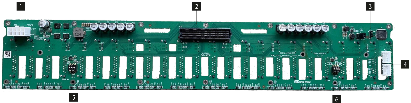
Рис. 11. Плата объединительная 24SFF (НИКА.469535.060)
