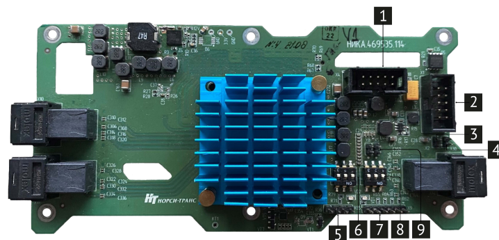
Рис. 12. Плата расширения A24SFF (НИКА.469535.114)
