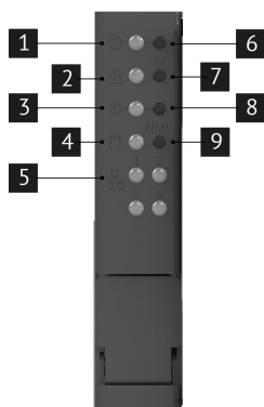
Рис. 3. Левая панель управления
