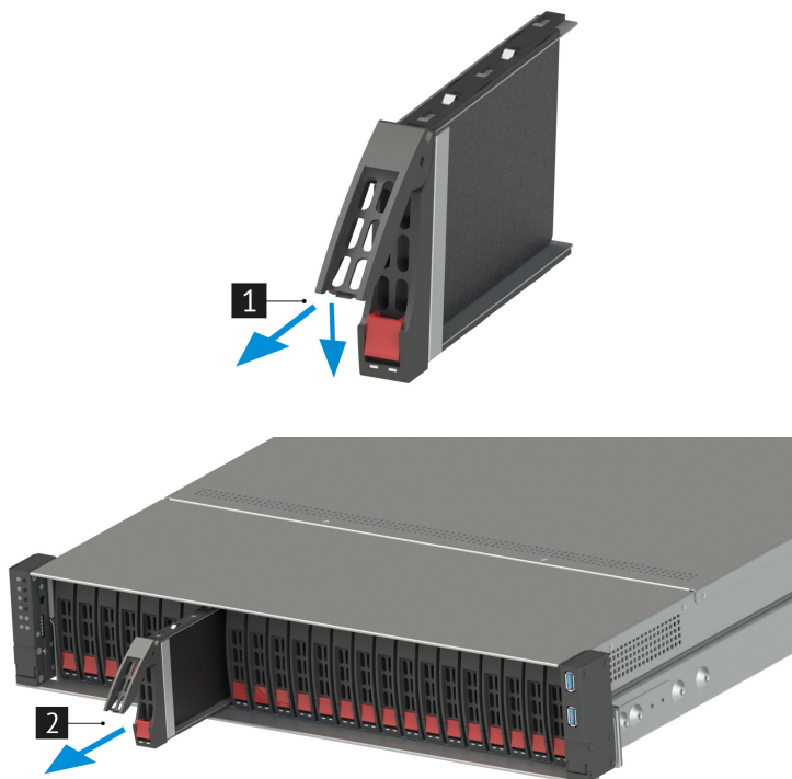
Рис. 41. Извлечение дисков
