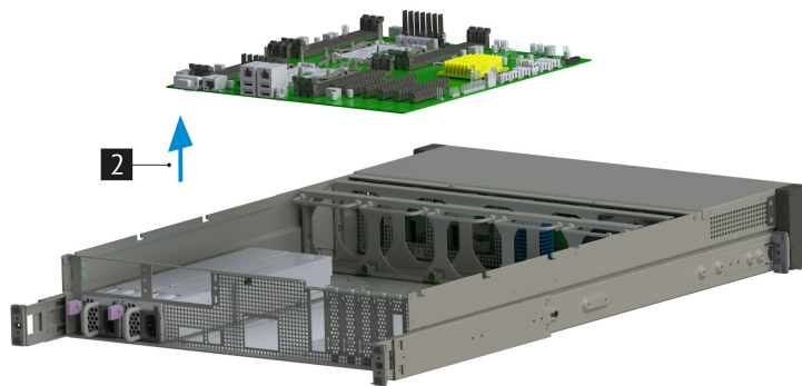
Рис. 39. Извлечение материнской платы
