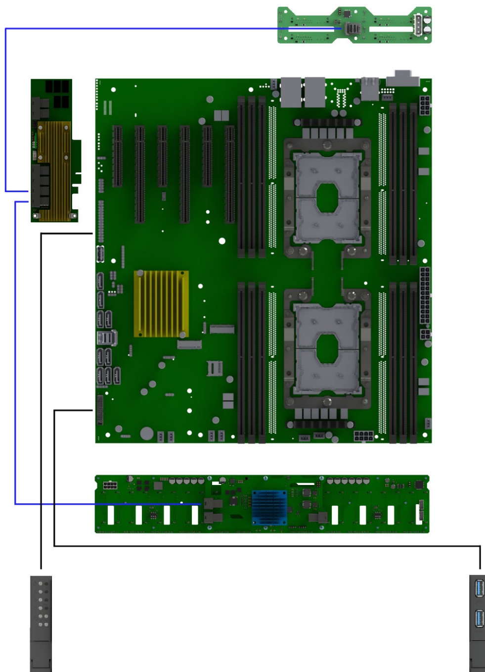
Рис. 25. Схема прокладки системных кабелей и кабелей питания
