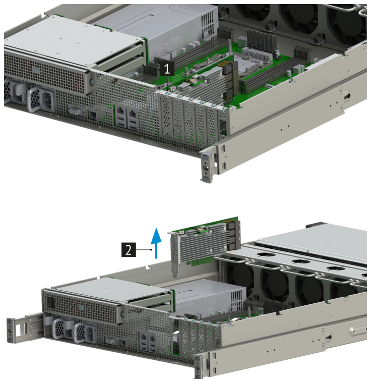
Рис. 45. Извлечение MegaRAID SAS 9361-16i
