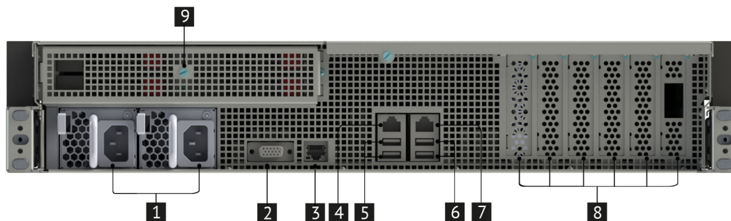
Рис. 5. Вид сервера сзади
