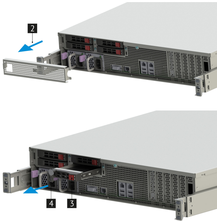
Рис. 43. Извлечение дисков
