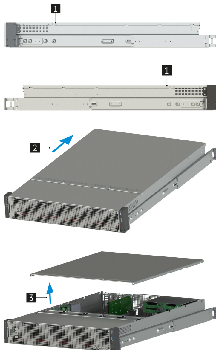
Рис. 20. Снятие задней крышки платформы
