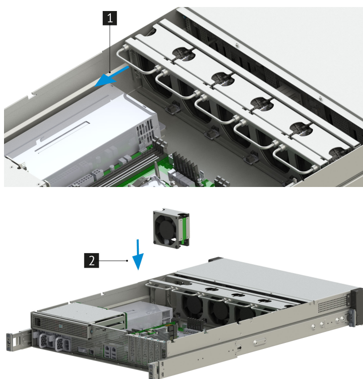
Рис. 27. Подключение вентилятора
