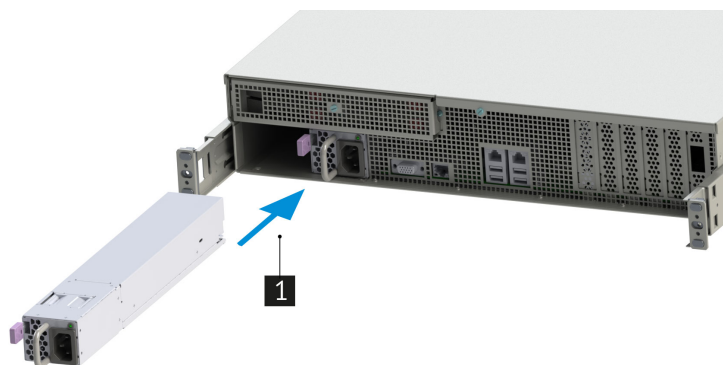
Рис. 51. Установка блока питания
