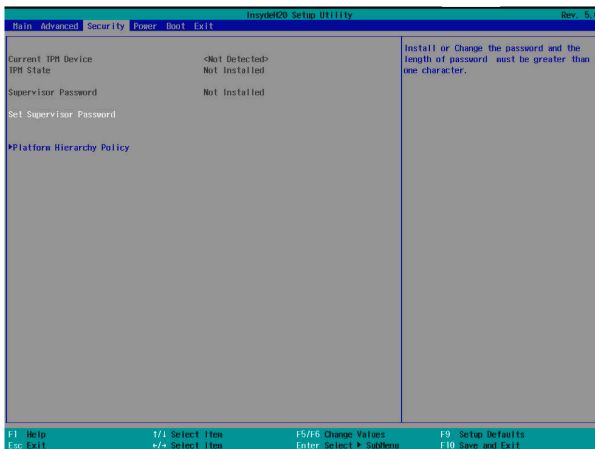
Рис. 57. Разделы меню «Security»
