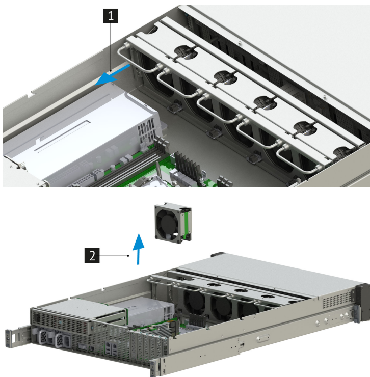
Рис. 26. Извлечение вентилятора
