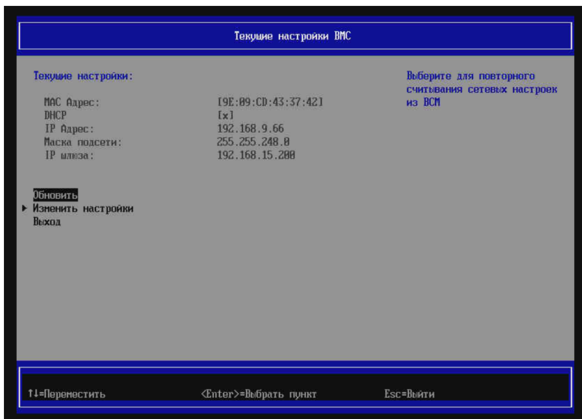
Рис. 73. Меню «Текущие настройки ВМС»
