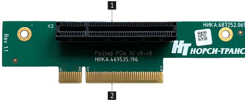
Рис. 13. Райзер PCIe 1U x8-x8 (НИКА.469535.196)
