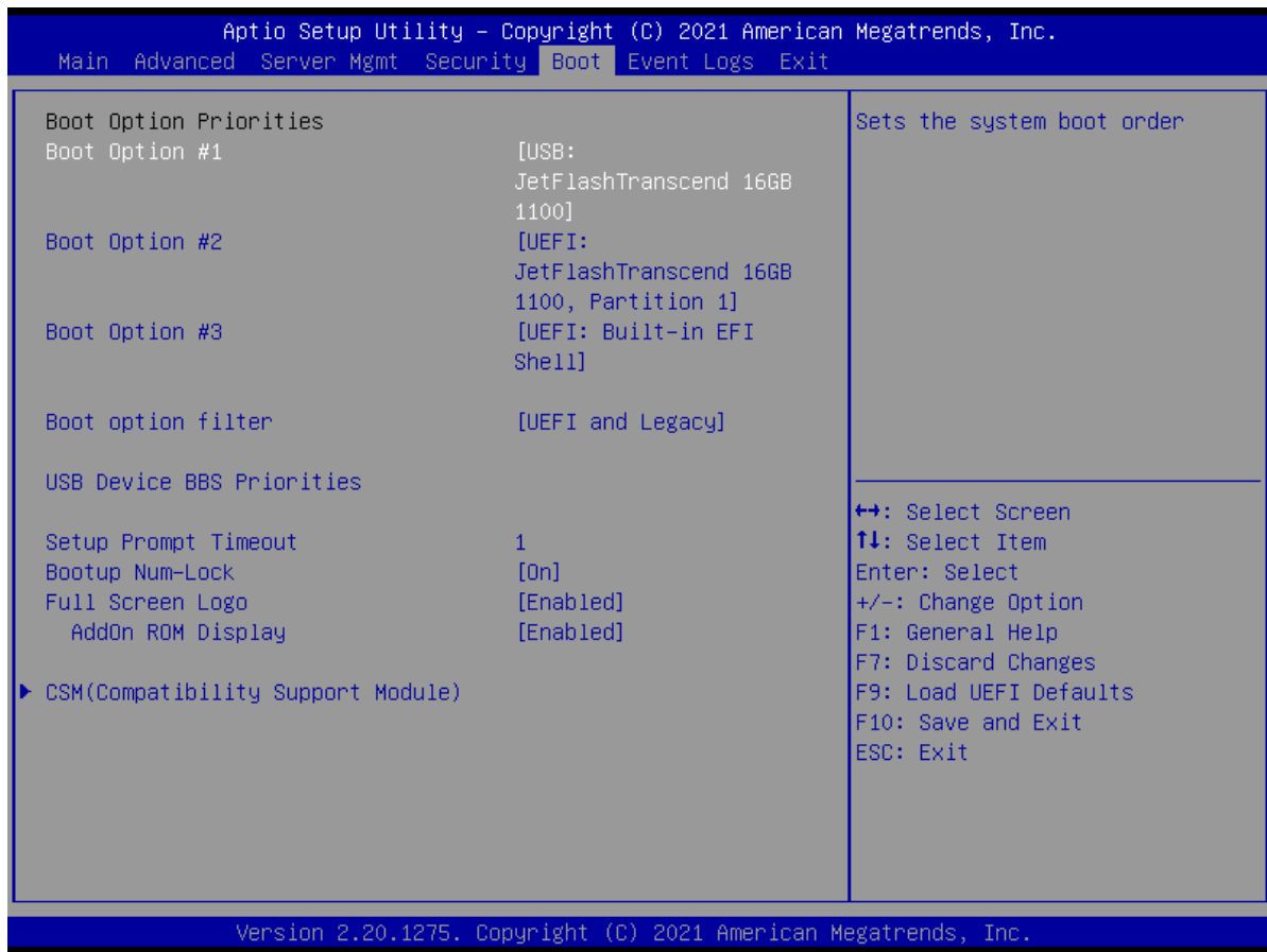
Рис. 103. Разделы меню «Boot»
