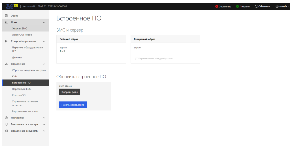
Рис. 97. Окно «Встроенное ПО»
