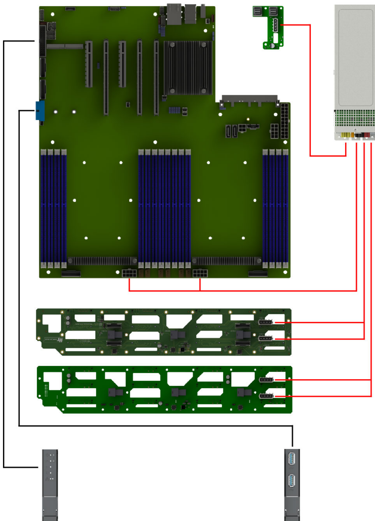
Рис. 35. Схема прокладки системных кабелей и кабелей питания при использовании платы расширения 2SFF NVMe (НИКА.469535.220)
