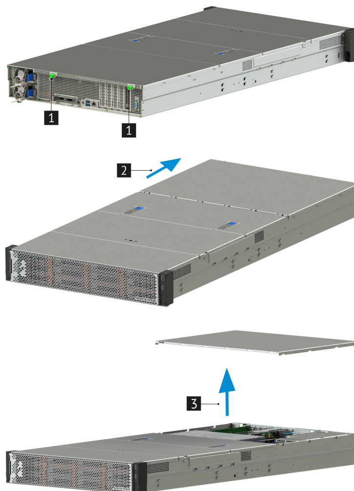
Рис. 27. Снятие задней крышки сервера
