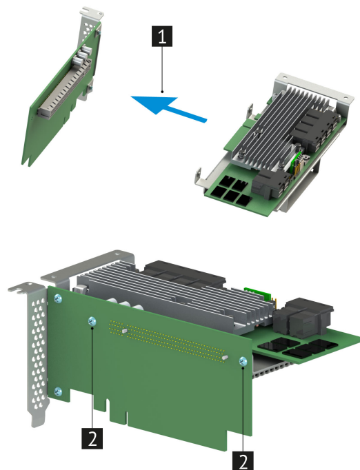
Рис. 66. Установка контроллера дискового MegaRAID 9361-24i
