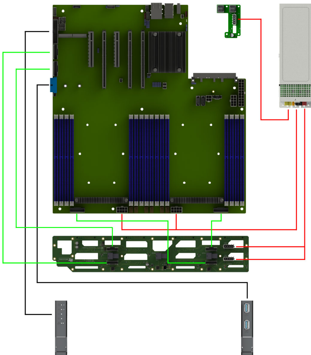
Рис. 38. Схема прокладки системных кабелей и кабелей SlimSAS-SlimSAS X8-X8 при использовании платы расширения 2SFF NVMe (НИКА.469535.220)
