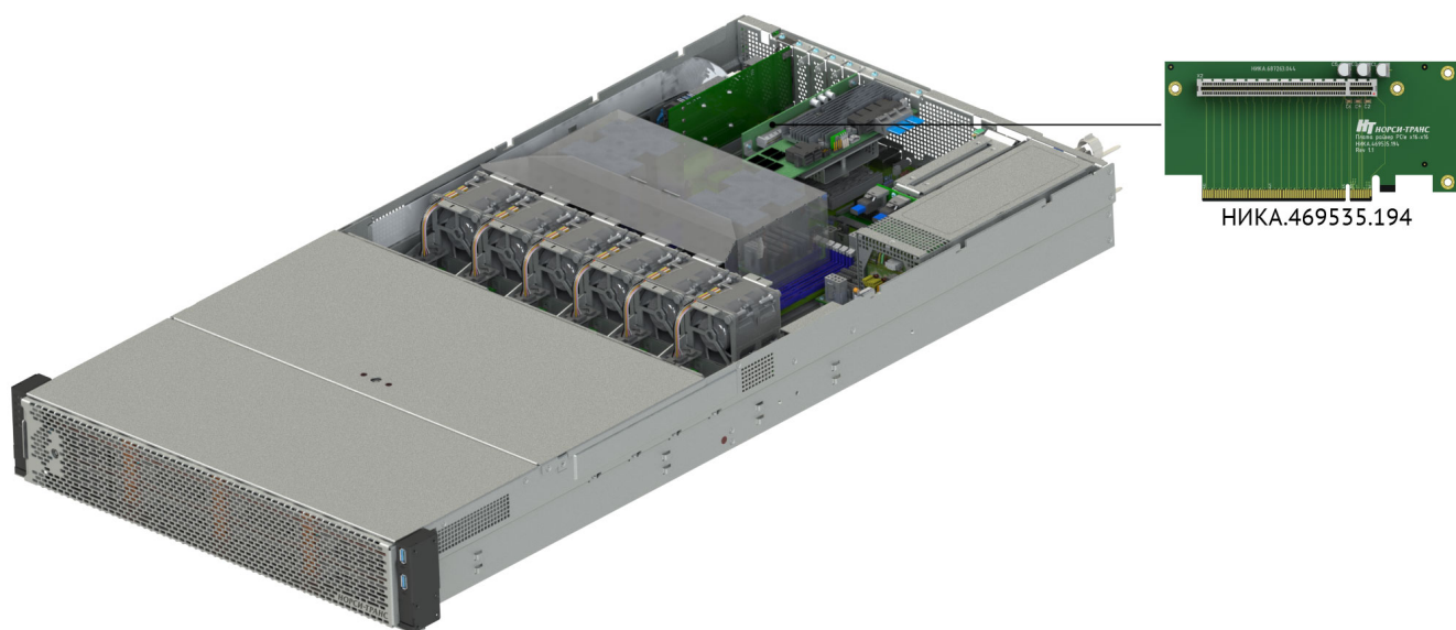
Рис. 14. Расположение PCIe-райзеров в сервере
