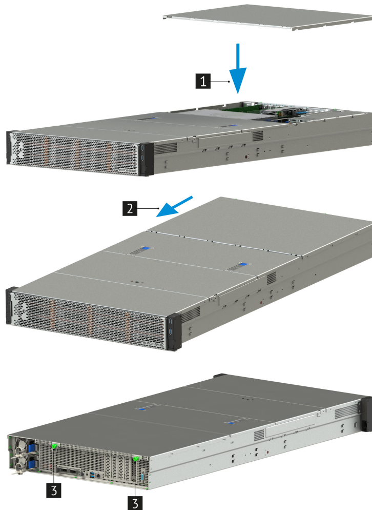
Рис. 28. Установка задней крышки сервера
