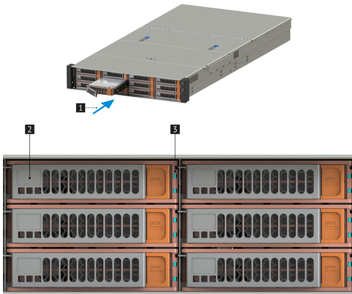
Рис. 55. Установка дисков
