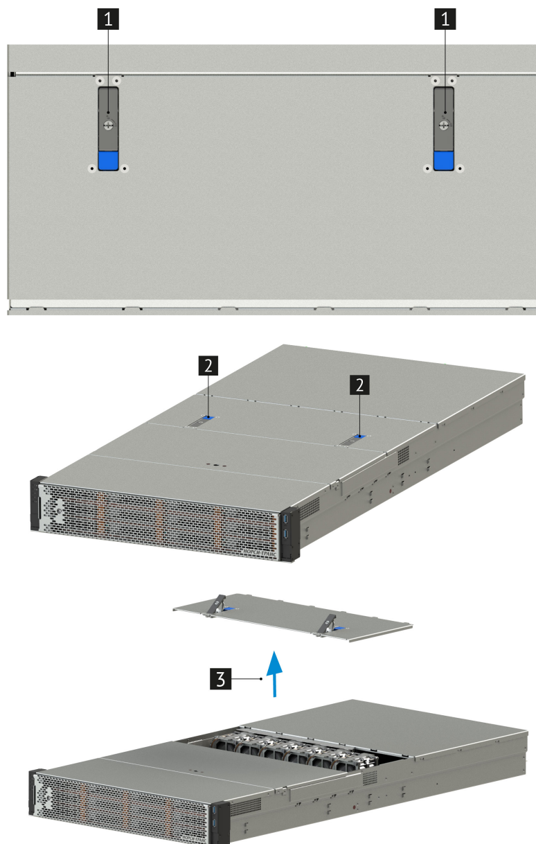
Рис. 25. Снятие крышки вентиляторов корпуса сервера
