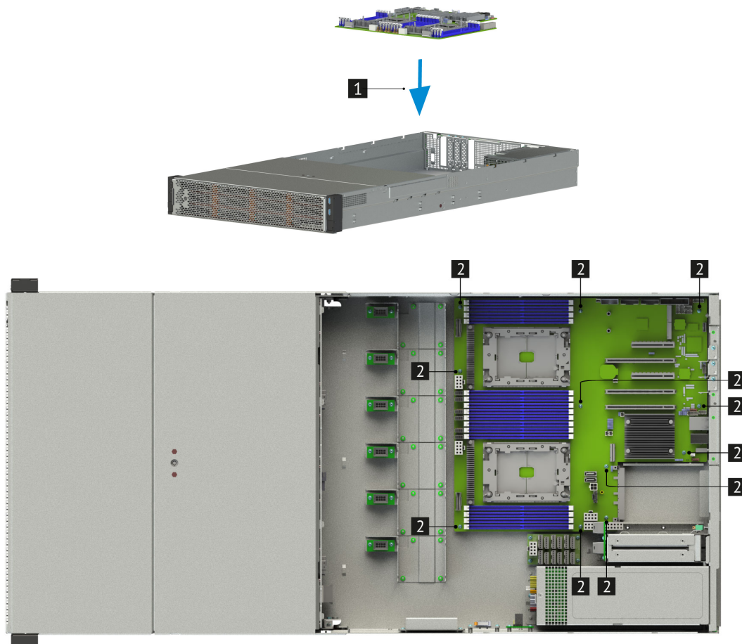
Рис. 53. Установка материнской платы в сервер
