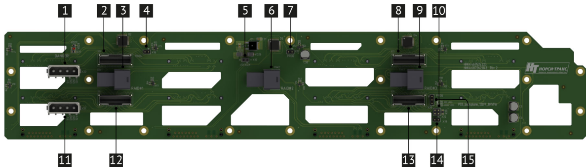
Рис. 10. Плата расширения 12LFF 8NVMe (НИКА.469535.223)
