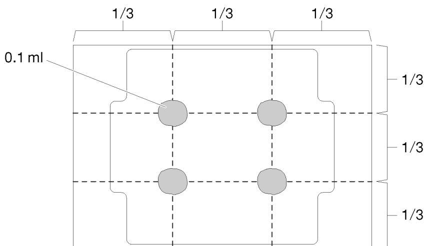
Рис. 51. Нанесение термопасты
