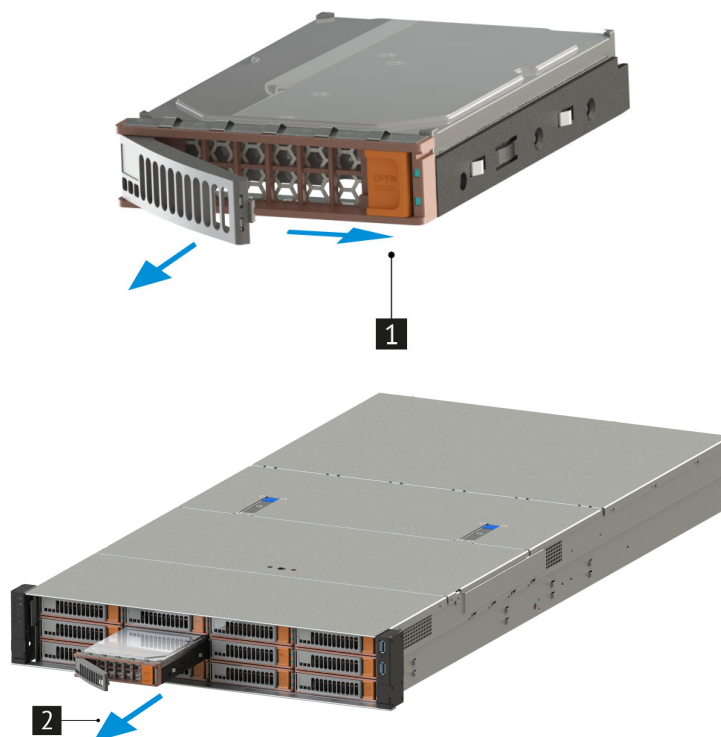
Рис. 54. Извлечение дисков
