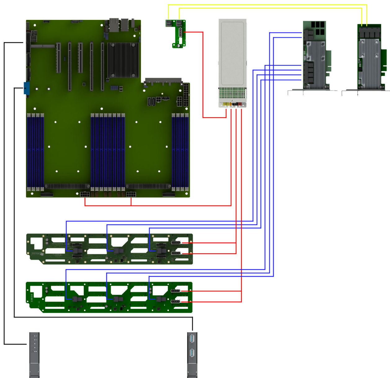
Рис. 36. Схема прокладки системных кабелей и кабелей питания с подключением PCIe RAID при использовании платы расширения 2SFF NVMe (НИКА.469535.220)
