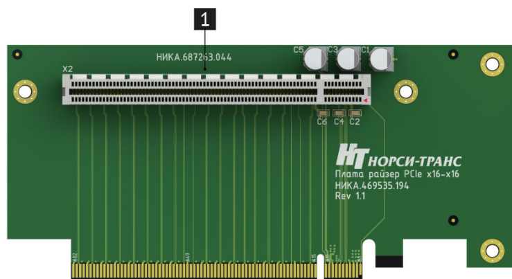
Рис. 15. Райзер PCIe x16-x16 (НИКА.469535.194)
