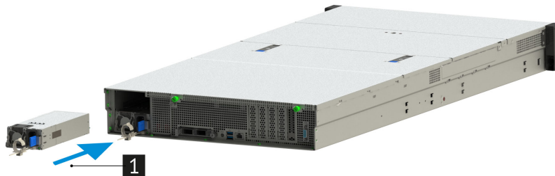
Рис. 75. Установка блока питания сервера
