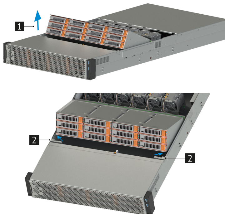
Рис. 29. Извлечение внутренней дисковой кассеты/поворотной кассеты
