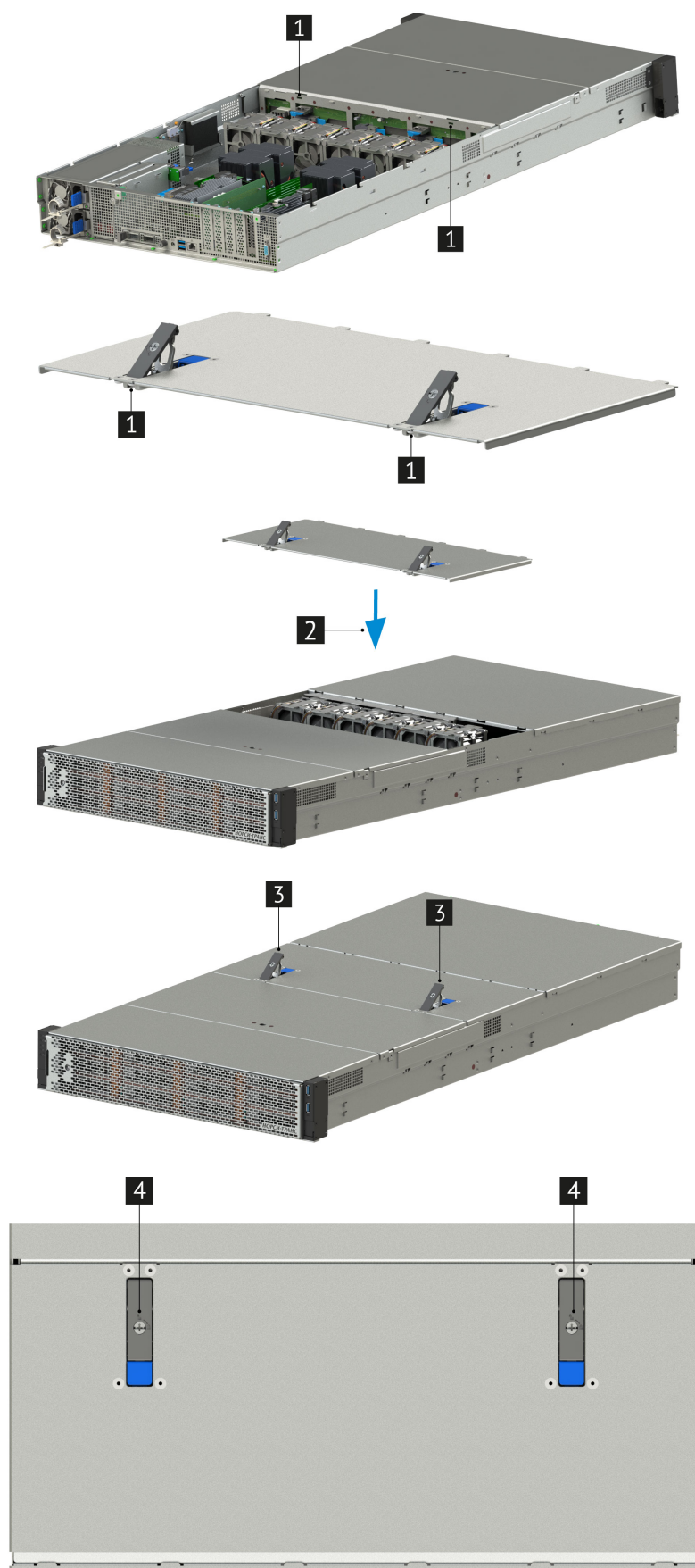
Рис. 26. Установка крышки вентиляторов корпуса сервера
