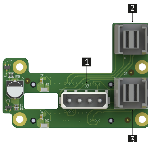
Рис. 13. Плата расширения 2SFF NVMe (НИКА.469535.220)
