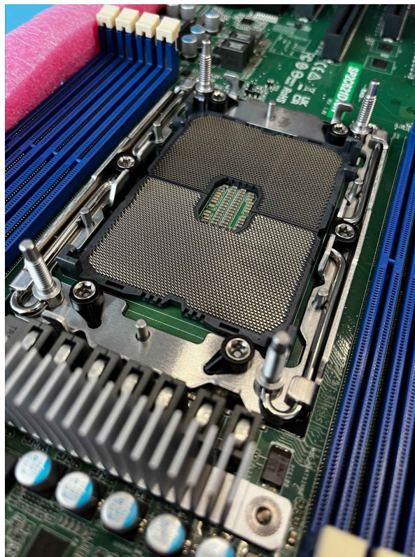
Рис. 48. Снятие модуля процессора с радиатором
