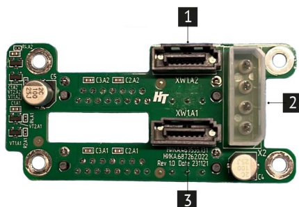
Рис. 12. Плата расширения 2SFF SATA (НИКА.469535.131)
