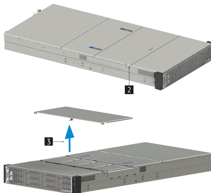
Рис. 23. Снятие крышки дисков корпуса сервера
