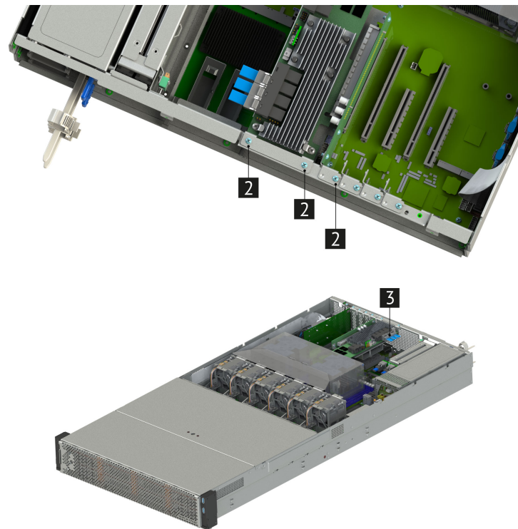
Рис. 64. Установка райзера PCIe x16-x16
