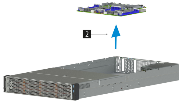
Рис. 52. Извлечение материнской платы из сервера
