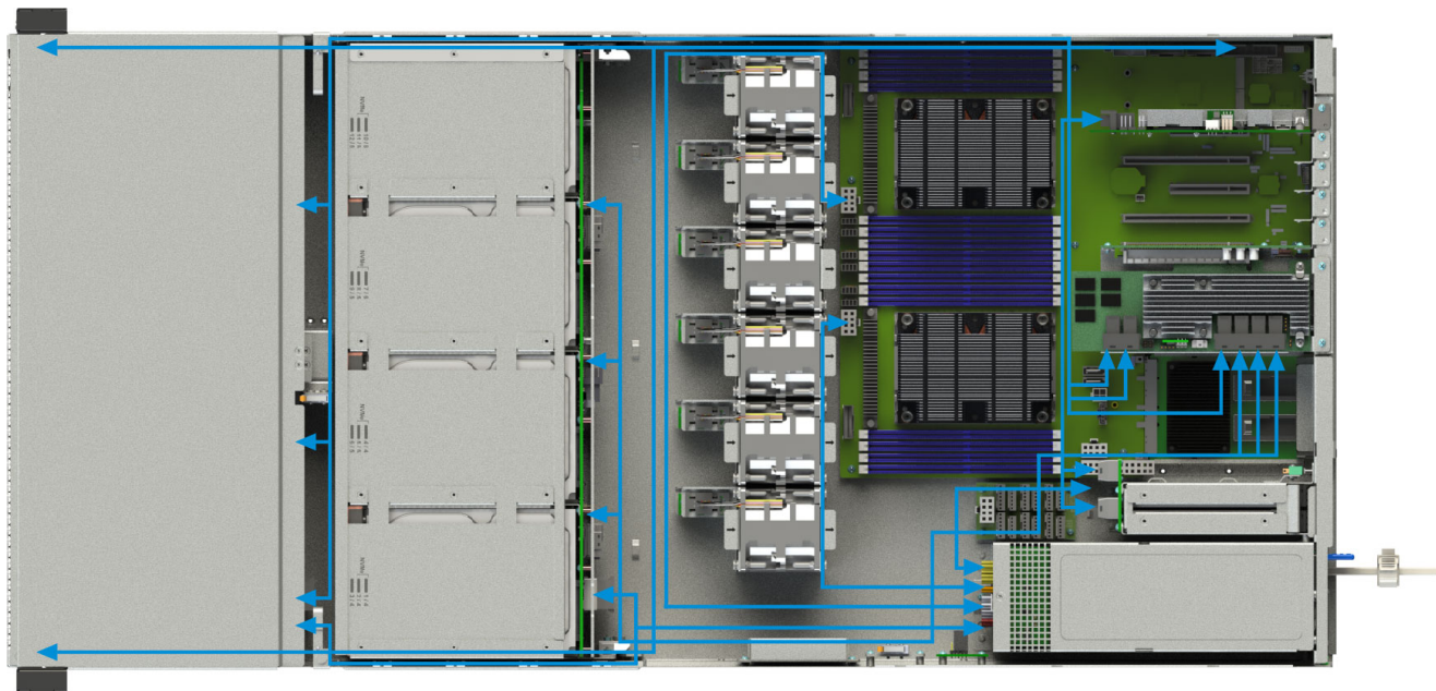
Рис. 33. Схема прокладки кабелей в сервере
