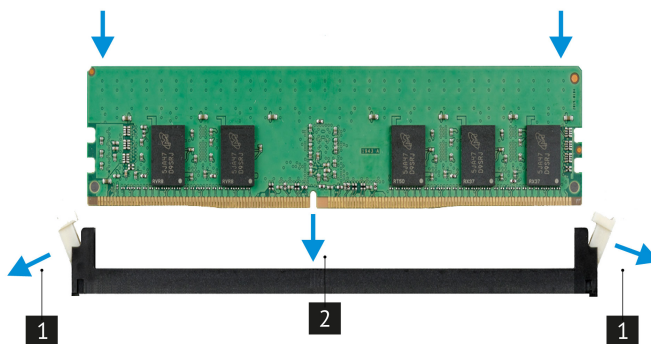
Рис. 46. Установка модуля ОЗУ
