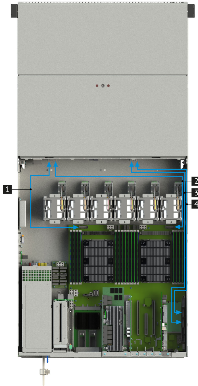
Рис. 59. Схема прокладки кабелей SlimSAS-SLIMline X8-X8
