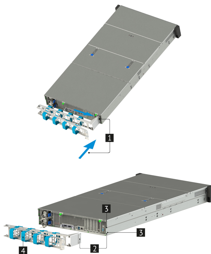
Рис. 18. Установка дополнительного кабельного органайзера.
