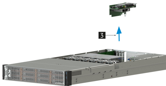
Рис. 63. Извлечение райзера PCIe x16-x16
