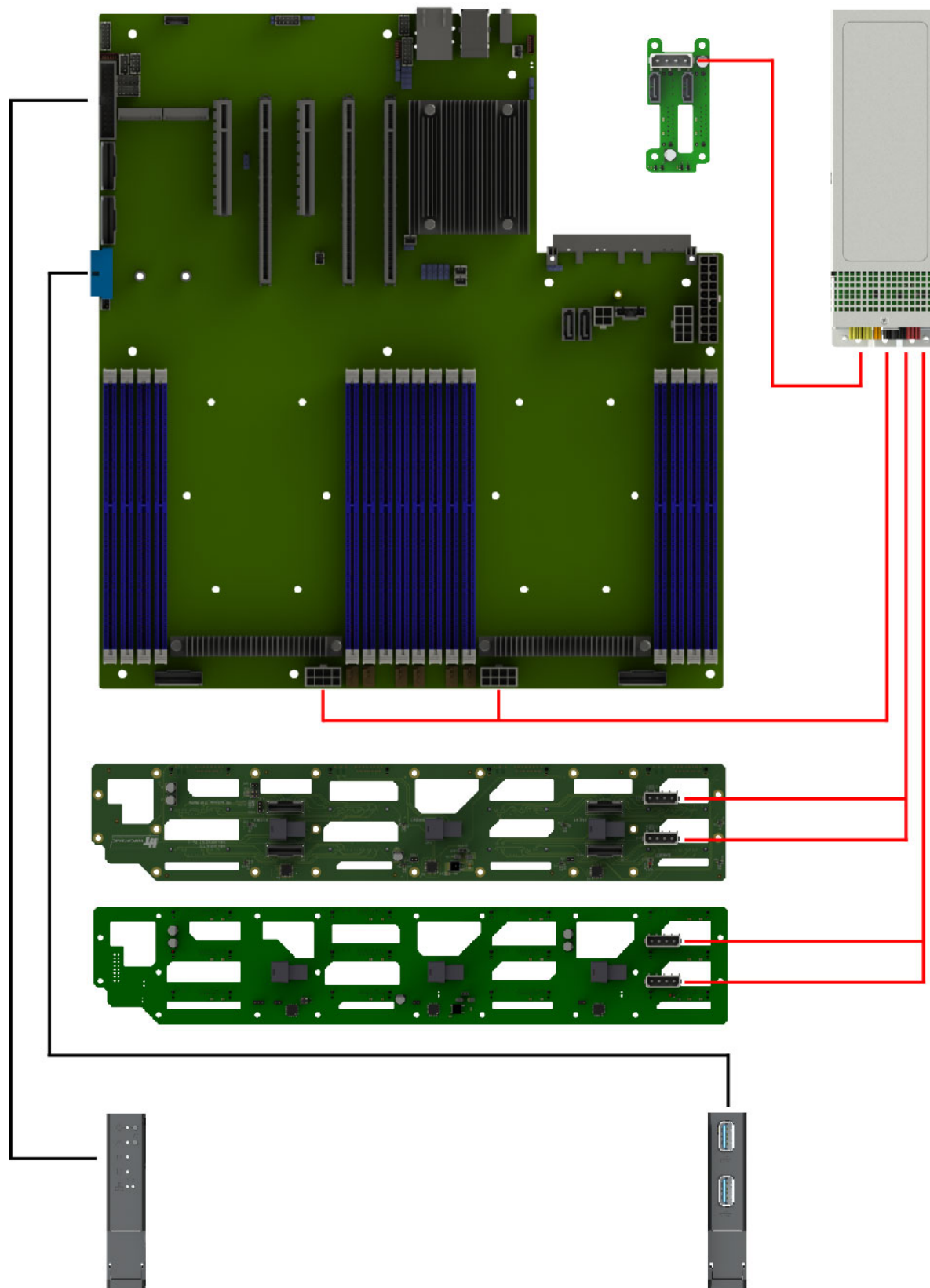
Рис. 34. Схема прокладки системных кабелей и кабелей питания при использовании платы расширения 2SFF SATA (НИКА.469535.131)
