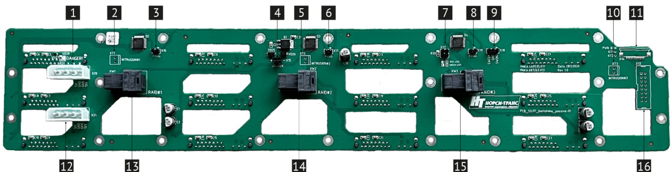
Рис. 11. Плата расширения 12LFF (НИКА.469535.071)
