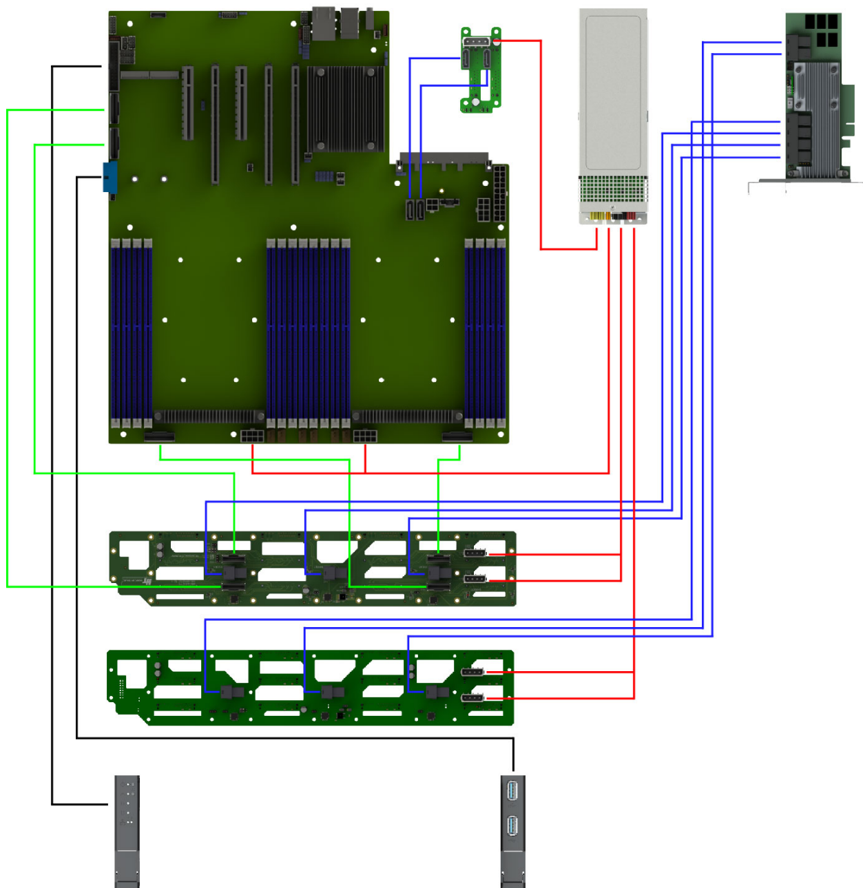
Рис. 41. Схема прокладки системных кабелей и кабелей Oculink-SLIMline X8-X8 с подключением PCIe RAID при использовании платы расширения 2SFF SATA (НИКА.469535.131)
