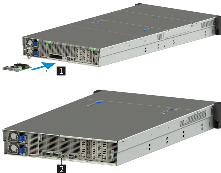
Рис. 70. Установка карты OCP 3.0 PCIe x16
