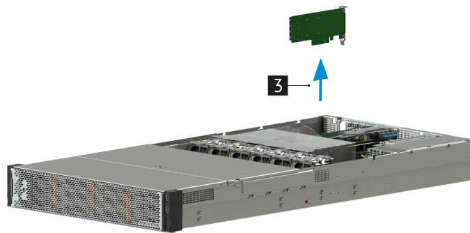
Рис. 67. Извлечение контроллера дискового MegaRAID 9361-16i
