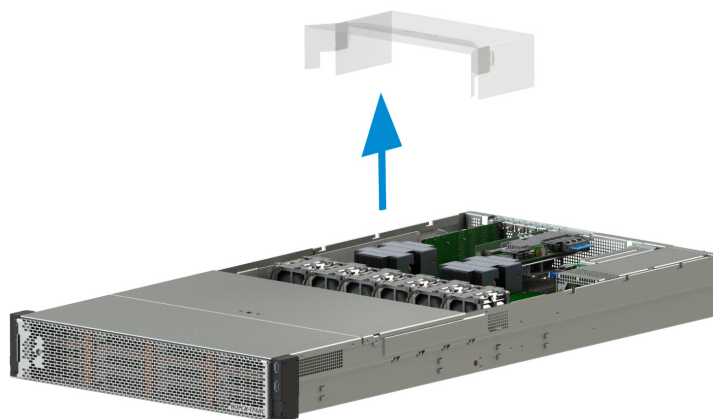
Рис. 31. Извлечение воздушного кожуха
