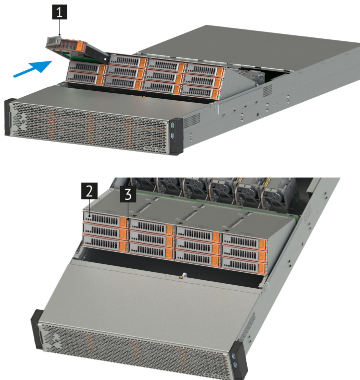
Рис. 57. Извлечение дисков
