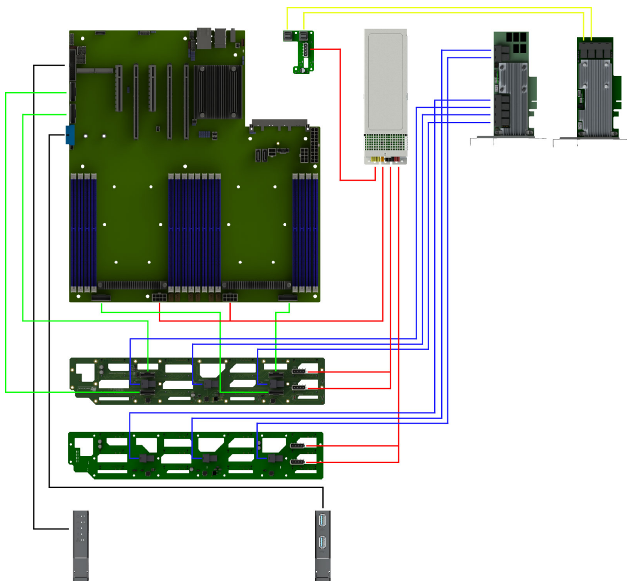
Рис. 40. Схема прокладки системных кабелей и кабелей Oculink-SLIMline X8-X8 с подключением PCIe RAID при использовании платы расширения 2SFF NVMe (НИКА.469535.220)
