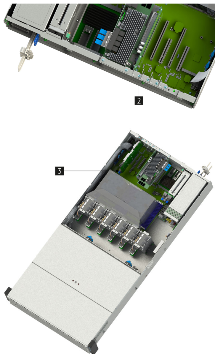
Рис. 68. Установка контроллера дискового MegaRAID 9361-16i
