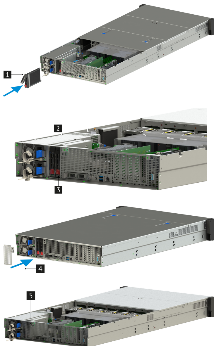
Рис. 62. Установка тыльных дисков
