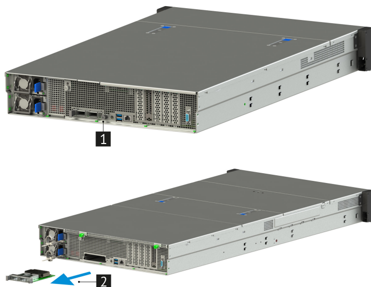
Рис. 69. Извлечение карты OCP 3.0 PCIe x16
