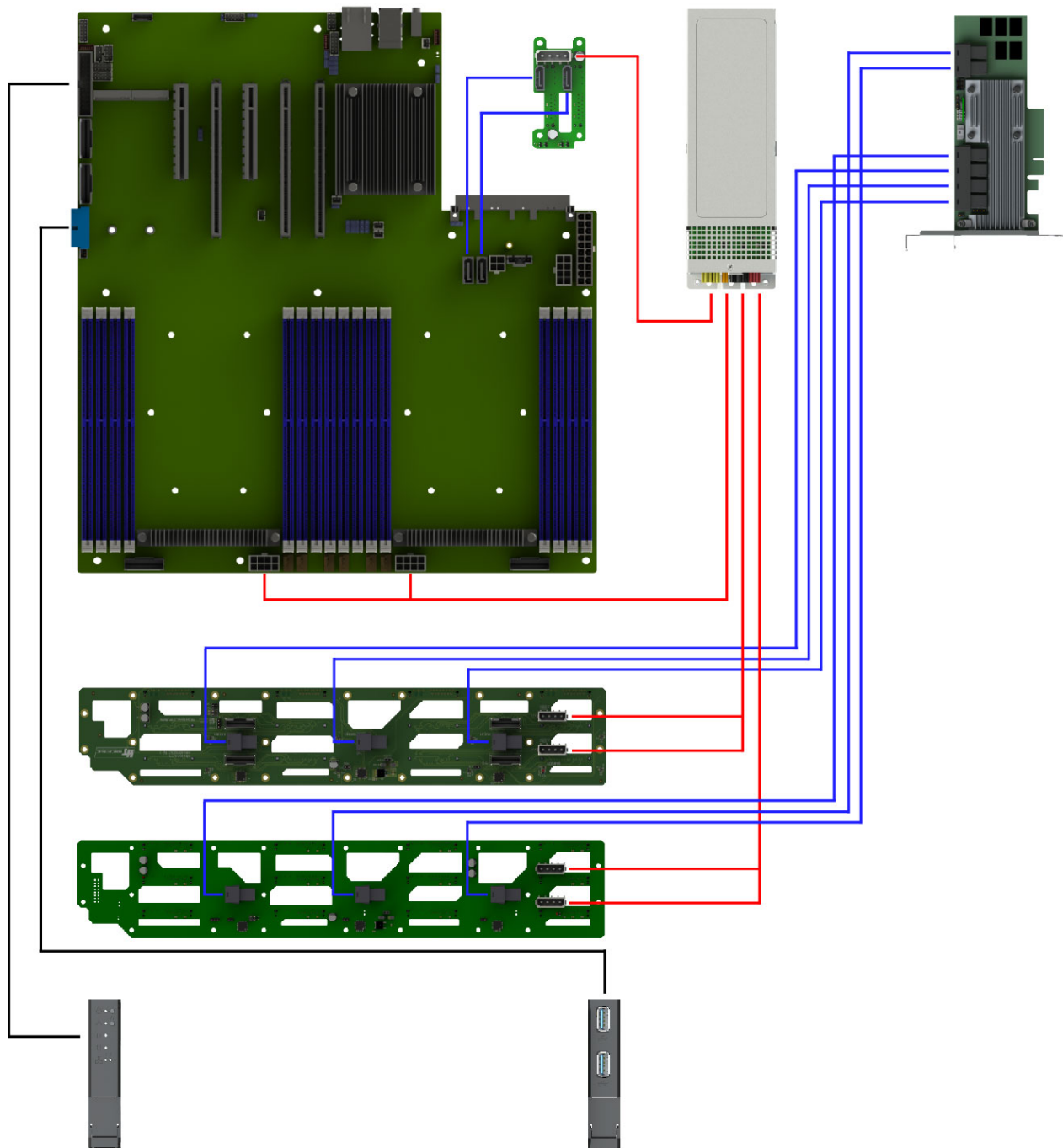
Рис. 37. Схема прокладки системных кабелей и кабелей питания с подключением PCIe RAID при использовании платы расширения 2SFF SATA (НИКА.469535.131)
