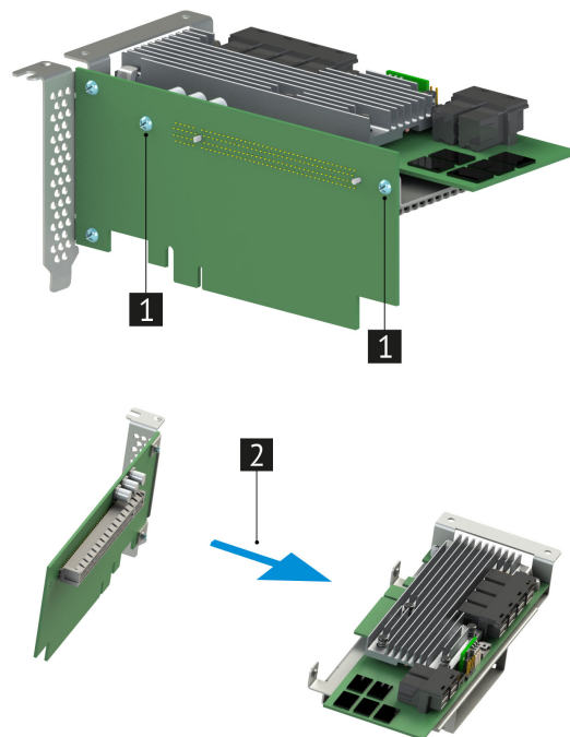
Рис. 65. Извлечение контроллера дискового MegaRAID 9361-24i
