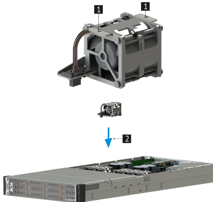
Рис. 43. Подключение вентилятора
