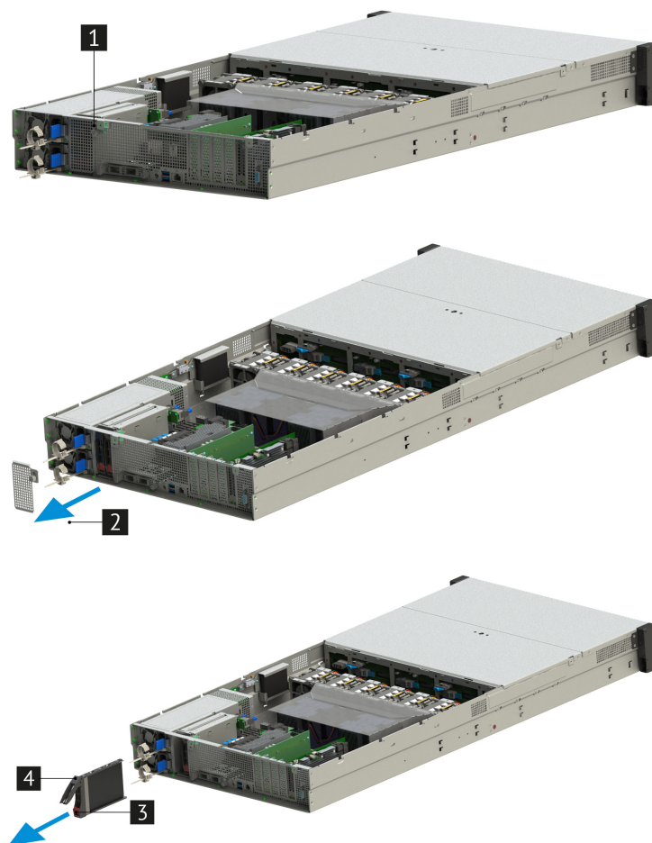
Рис. 61. Извлечение тыльных дисков
