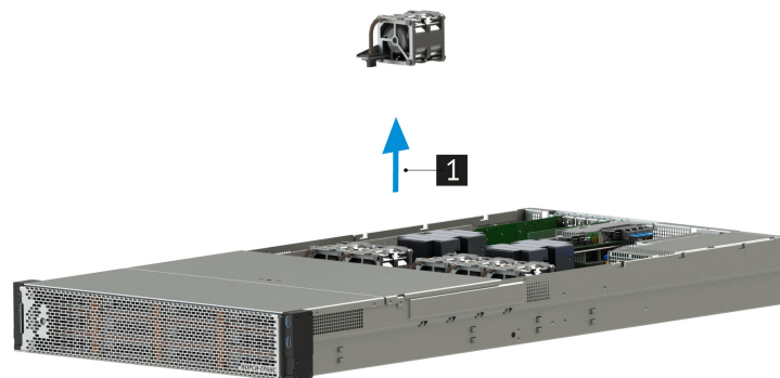
Рис. 42. Извлечение вентилятора из сервера
