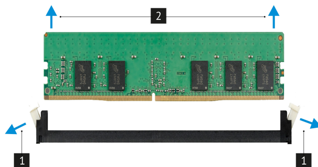
Рис. 45. Извлечение модуля ОЗУ
