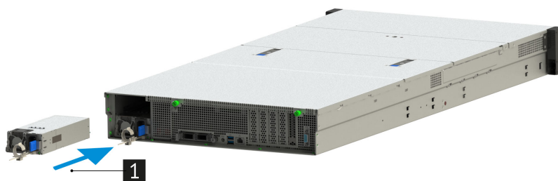
Рис. 73. Установка блока питания в сервер
