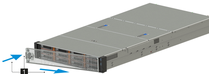
Рис. 21. Установка передней панели
