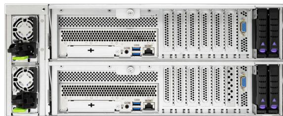
Сервер Тиара-А4 / Вид сзади
