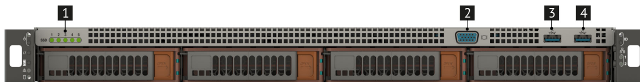
Рис. 3. Вид сервера спереди без защитной передней панели
