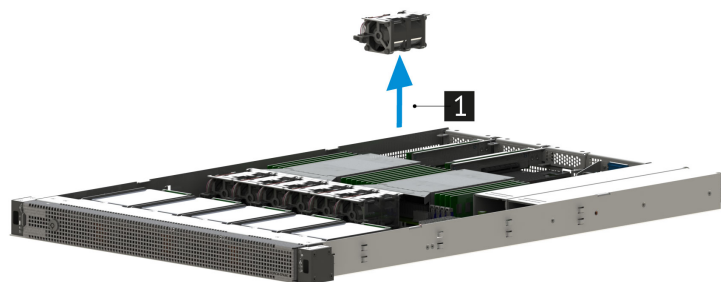
Рис. 30. Извлечение вентилятора из сервера
