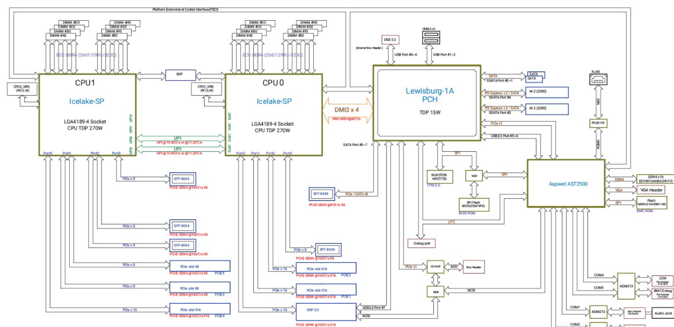
Рис. 1. Структурная схема материнской платы МП2х1ХS3G «Арктур»
