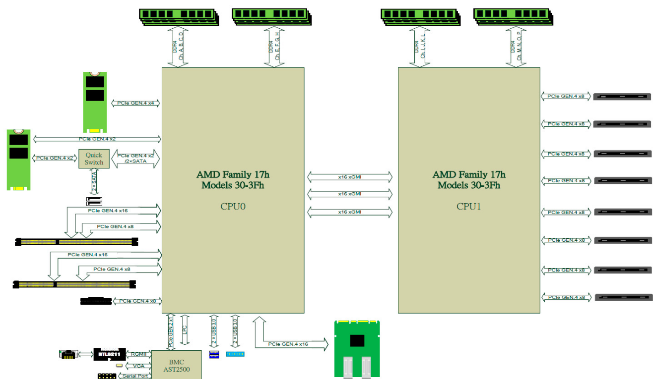
Рис. 1. Структурная схема материнской платы ASRock ROME2D16HM3
