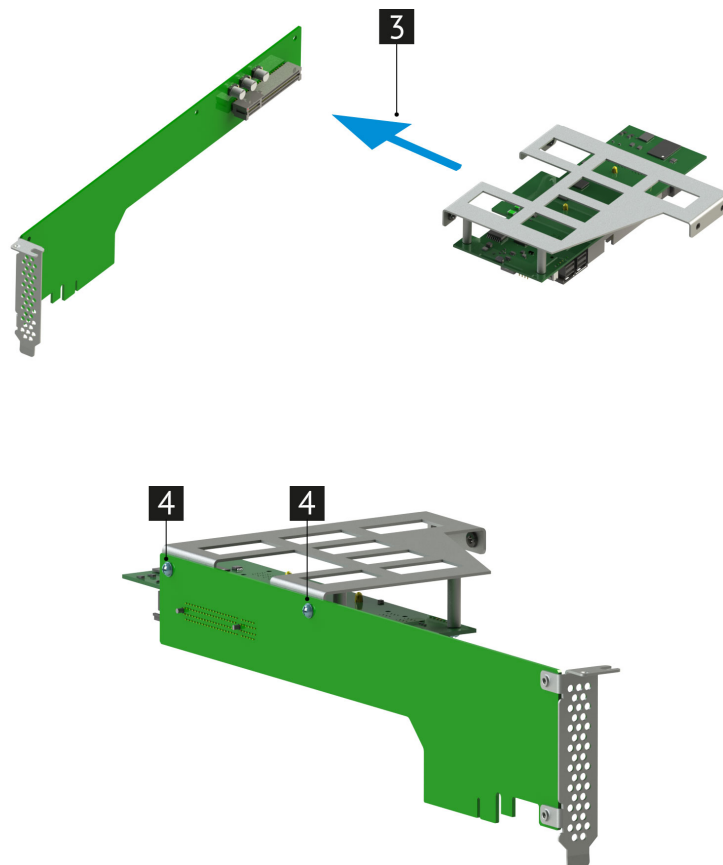
Рис. 49. Установка контроллера дискового SAS-3 RAID-24i
