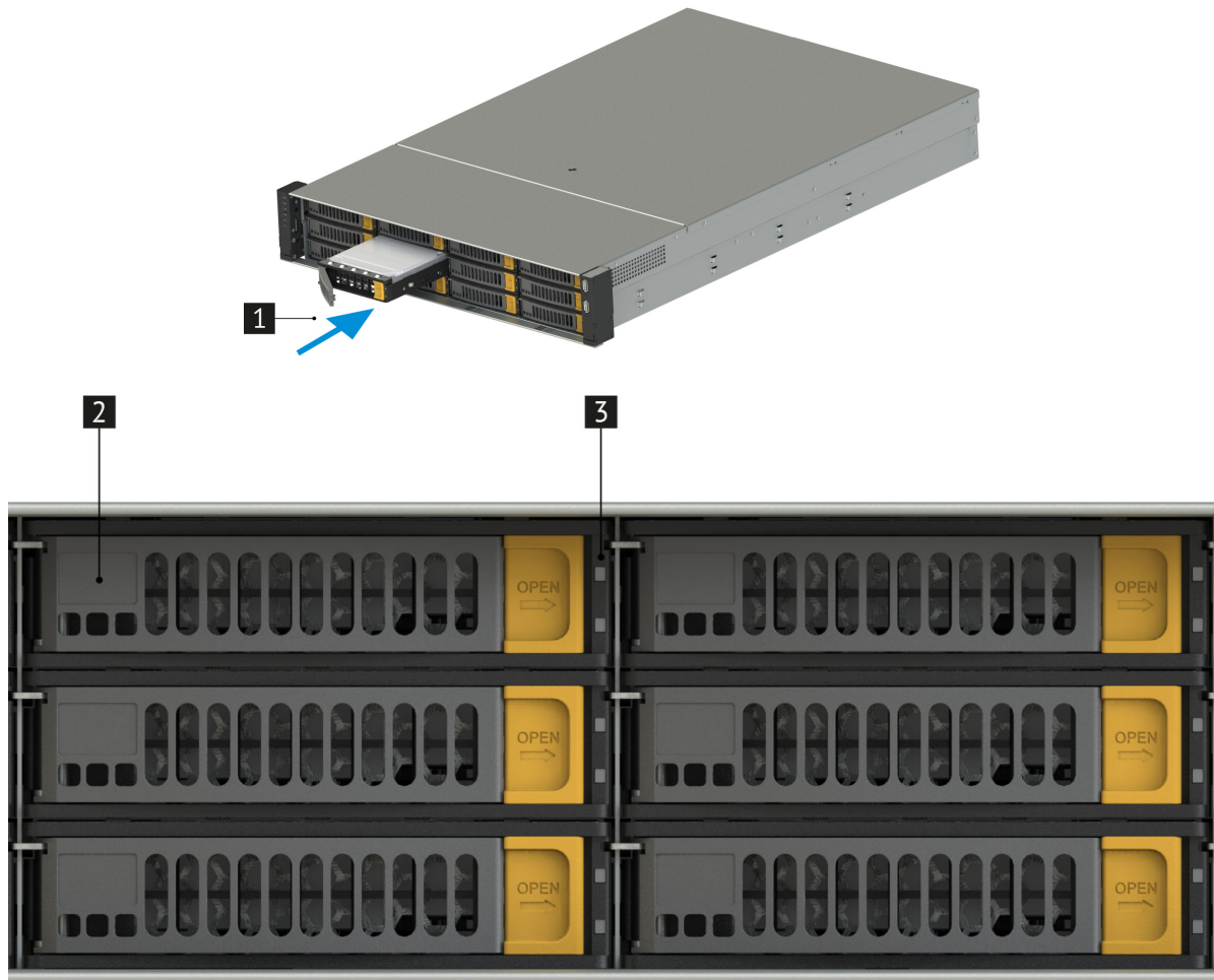
Рис. 43. Установка дисков
