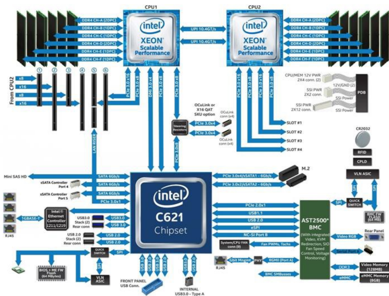
Рис. 1. Структурная схема материнской платы Rikor® R-BD-SXRM-XS16.EA.V6.0
