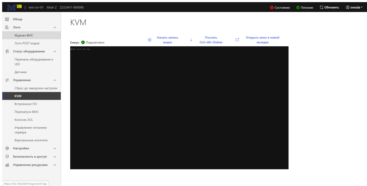
Рис. 83. Окно «KVM»
