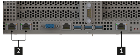
Рис. 10. Сетевые интерфейсы
