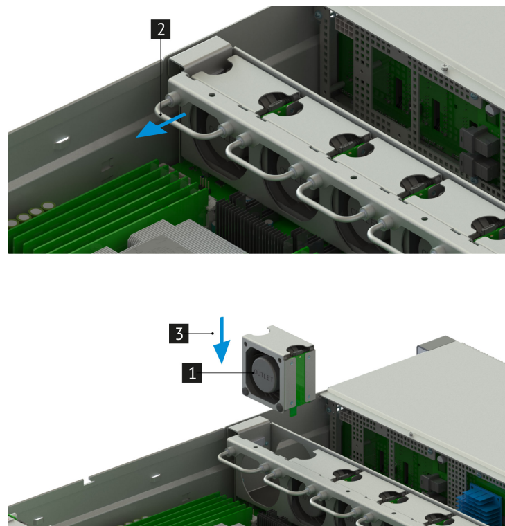
Рис. 37. Подключение вентилятора
