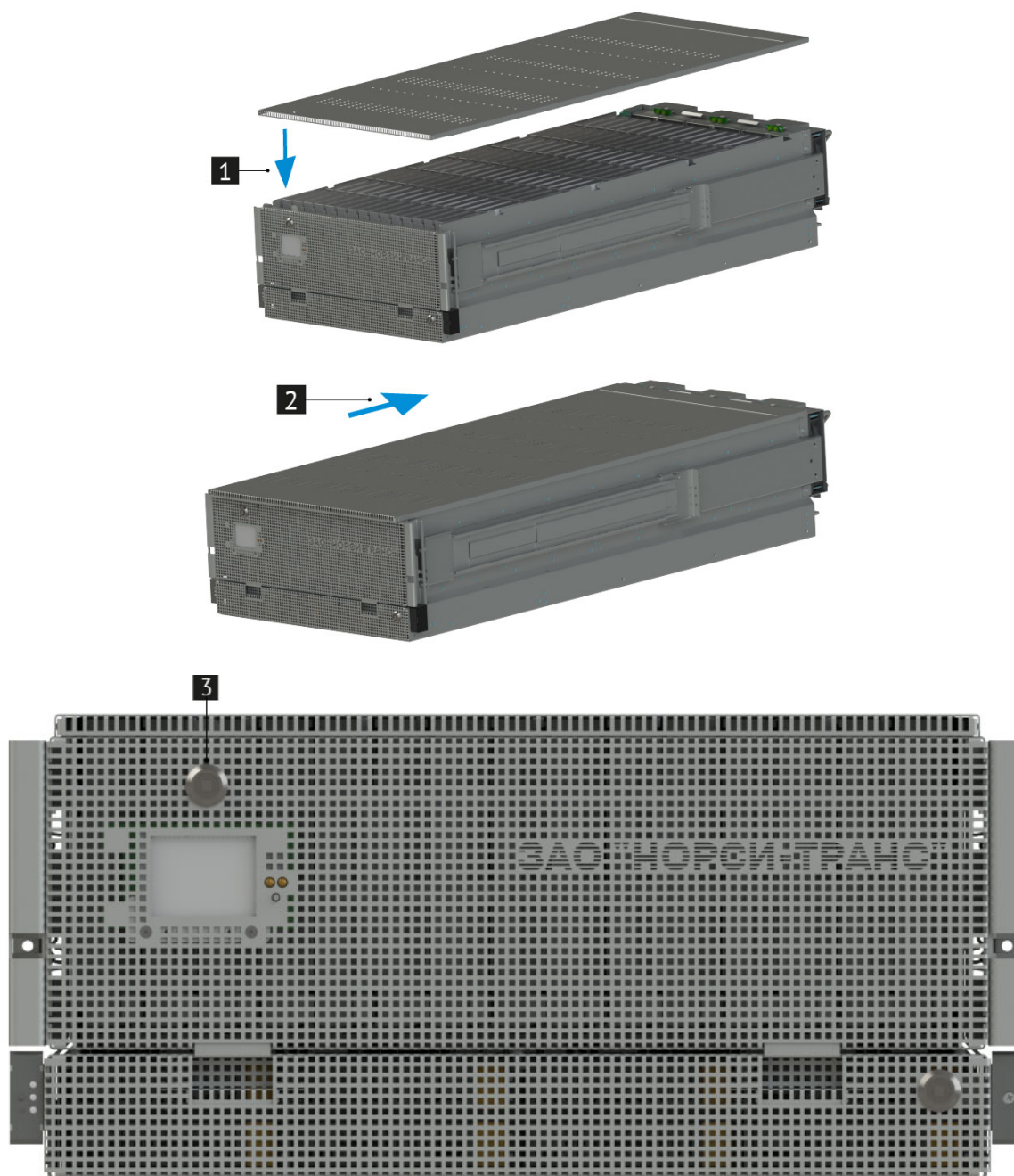
Рис. 19. Установка верхней крышки платформы
