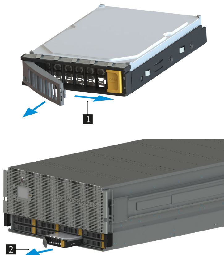
Рис. 42. Извлечение дисков
