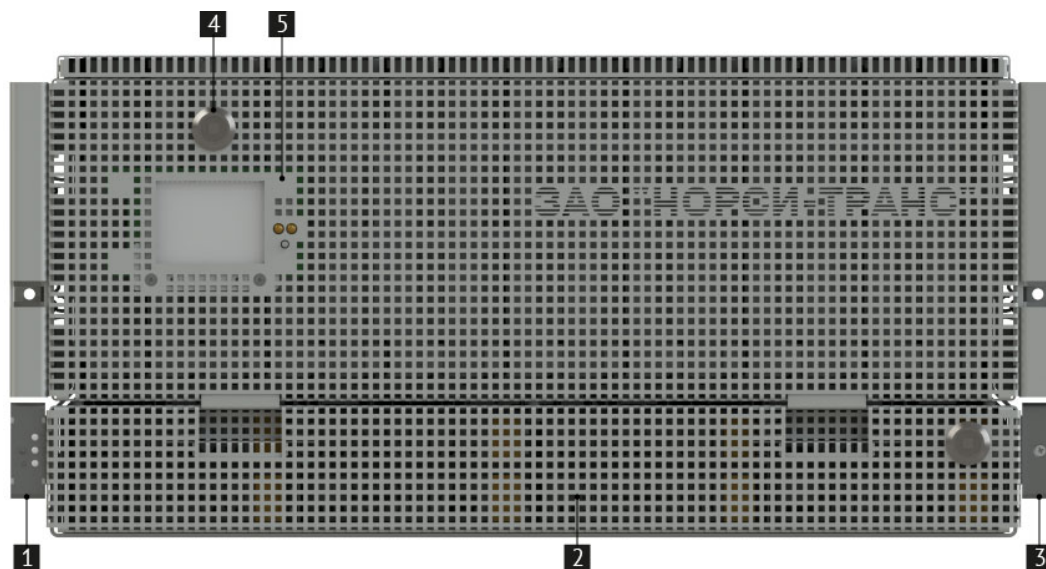
Рис. 2. Вид сервера спереди
