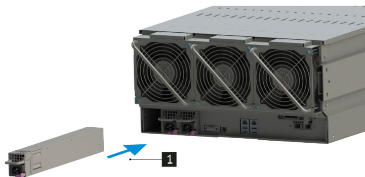
Рис. 58. Установка блока питания
