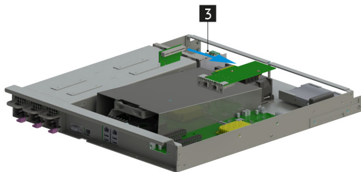
Рис. 50. Снятие карты расширения
