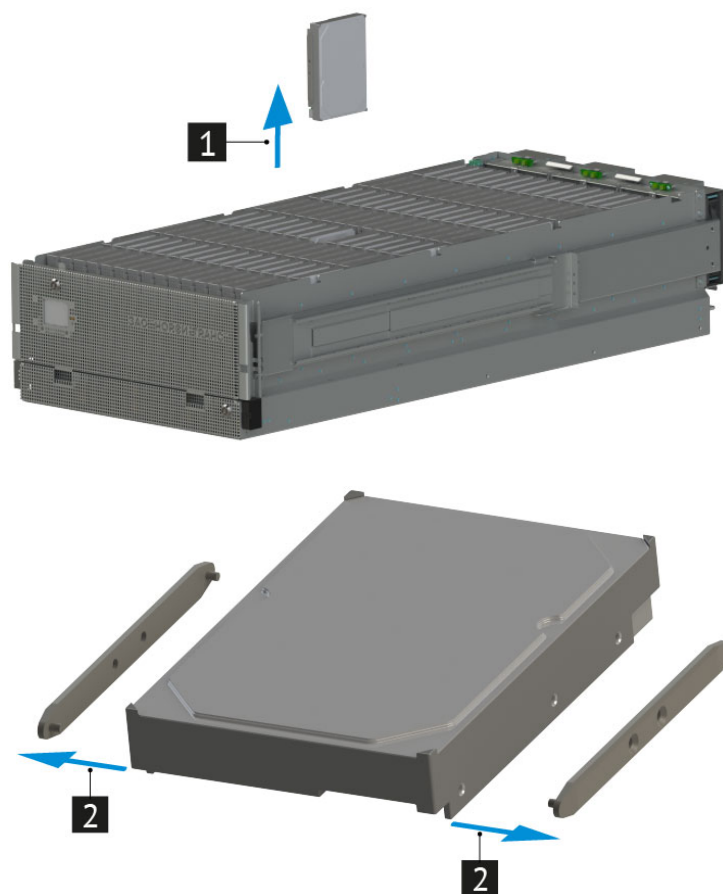
Рис. 44. Извлечение диска из массива дисков
