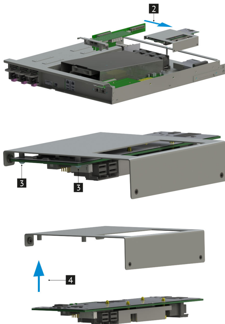
Рис. 52. Извлечение контроллера дискового SAS-3 RAID-24i
