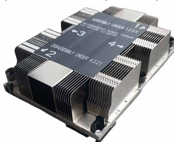
Рис. 34. 1U радиатор
