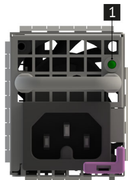
Рис. 54. Светодиодная индикация состояния блока питания
