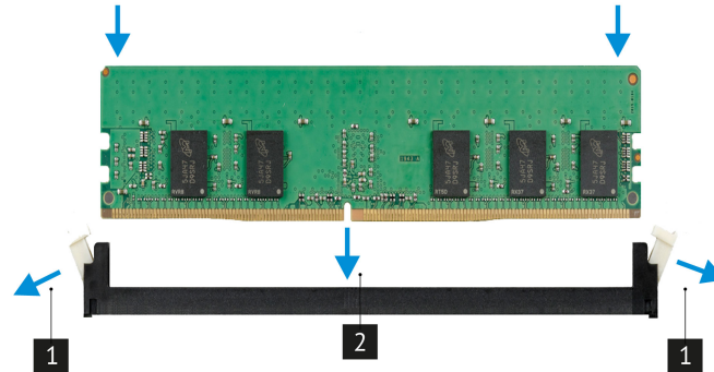
Рис. 33. Установка модуля ОЗУ.
