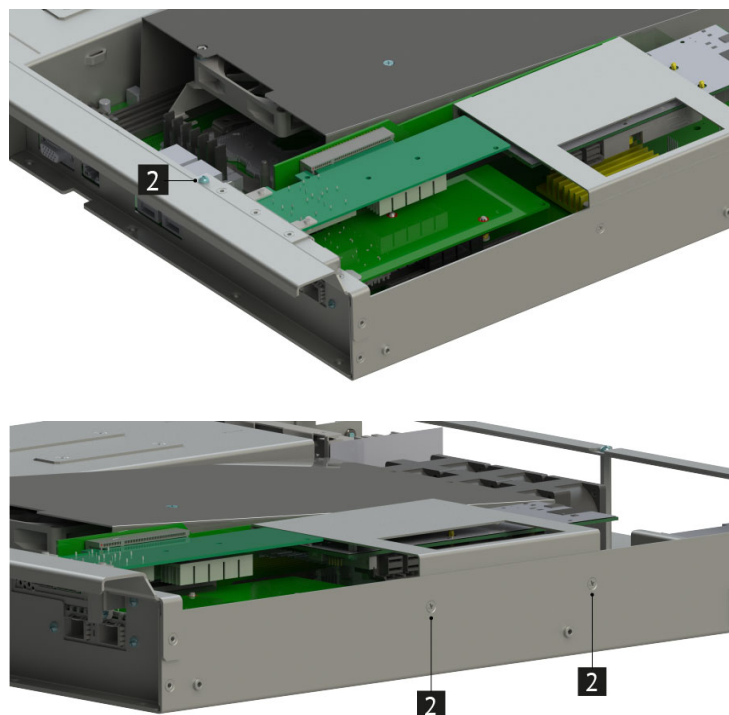
Рис. 47. Установка адаптера поворотного НИКА.469535.122 с картами расширения
