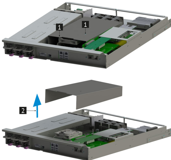
Рис. 22. Извлечение воздушного кожуха
