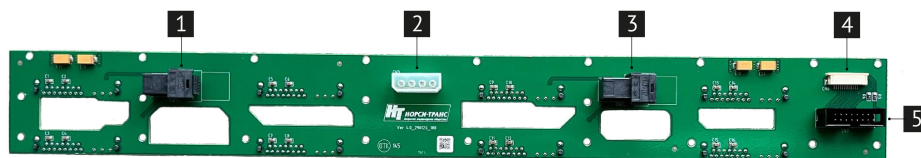
Рис. 10. Плата дискового массива A8 (НИКА.469535.013)
