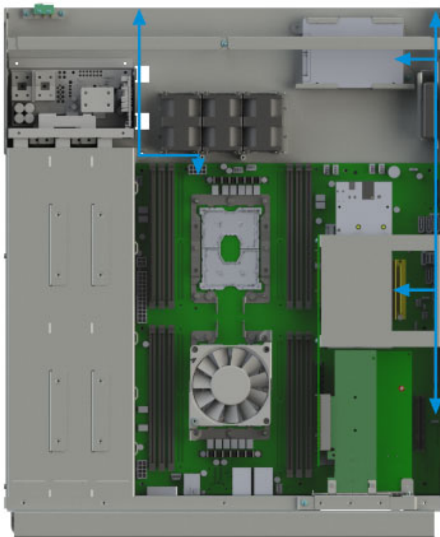
Рис. 24. Схема прокладки кабелей
