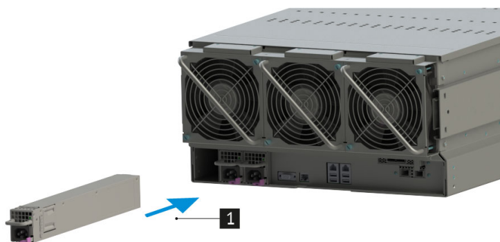
Рис. 56. Установка блока питания
