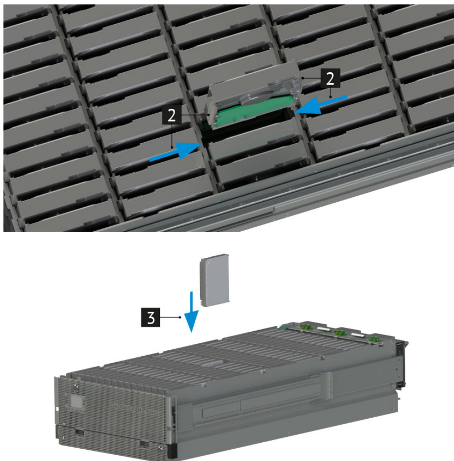
Рис. 45. Установка диска в массив дисков
