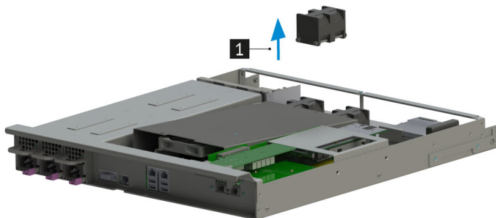
Рис. 26. Извлечение вентилятора из поддона заднего НИКА.301414.011
