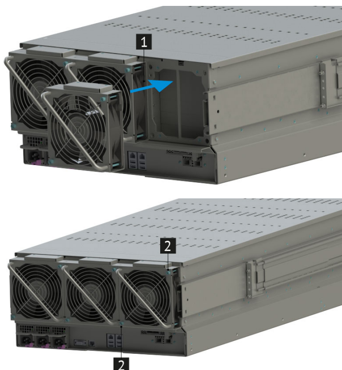
Рис. 29. Подключение наружного вентилятора к корпусу сервера
