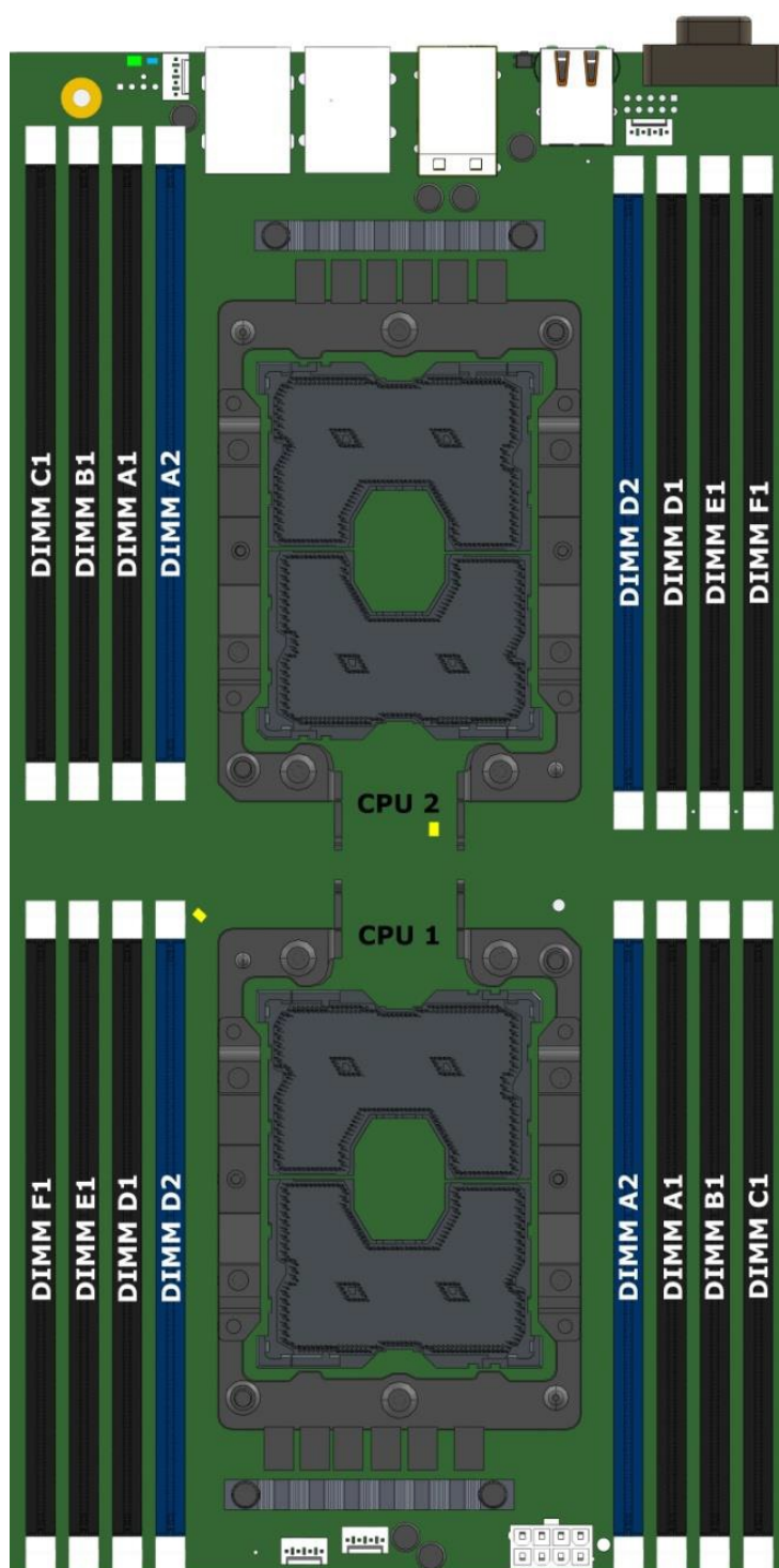
Рис. 30. Расположение разъемов.
