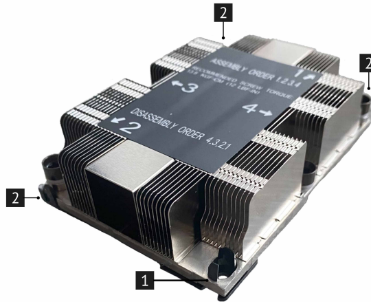
Рис. 37. Снятие процессора с 1U радиатора
