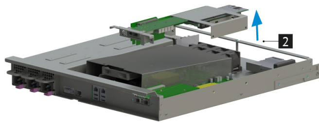
Рис. 46. Извлечение адаптера поворотного НИКА.469535.122 с картами расширения
