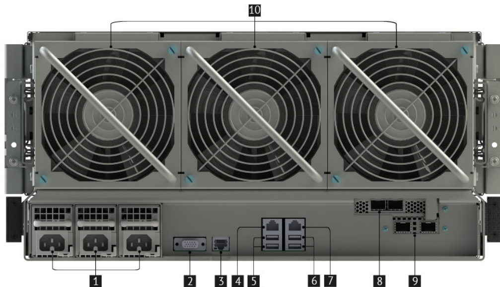
Рис. 4. Вид сервера сзади
