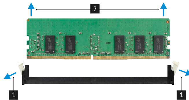
Рис. 32. Извлечение модуля ОЗУ.
