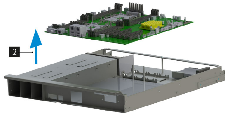
Рис. 40. Извлечение материнской платы
