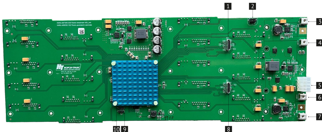
Рис. 11. Плата дискового массива (НИКА.469535.102)
