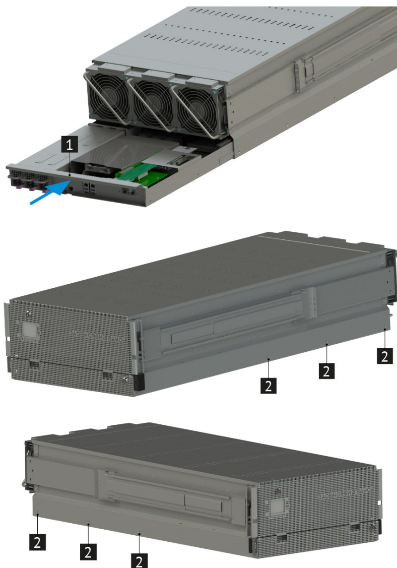
Рис. 21. Установка поддона заднего НИКА.301414.011
