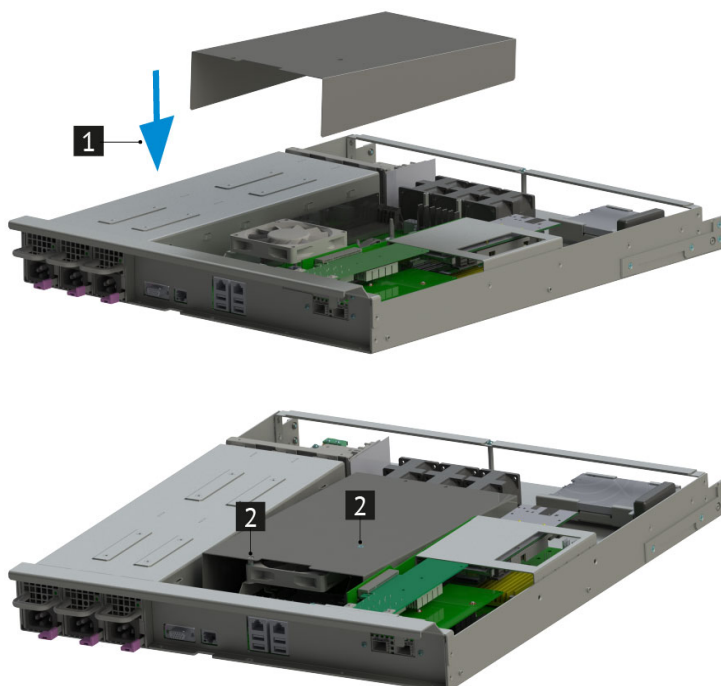
Рис. 23. Установка воздушного кожуха
