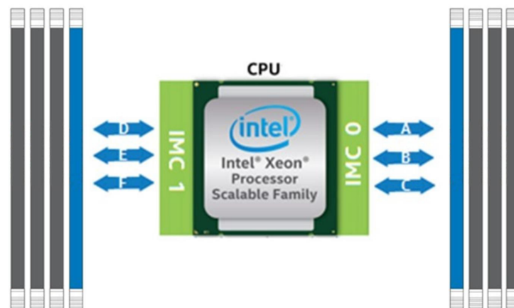
Рис. 31. Каналы памяти.
