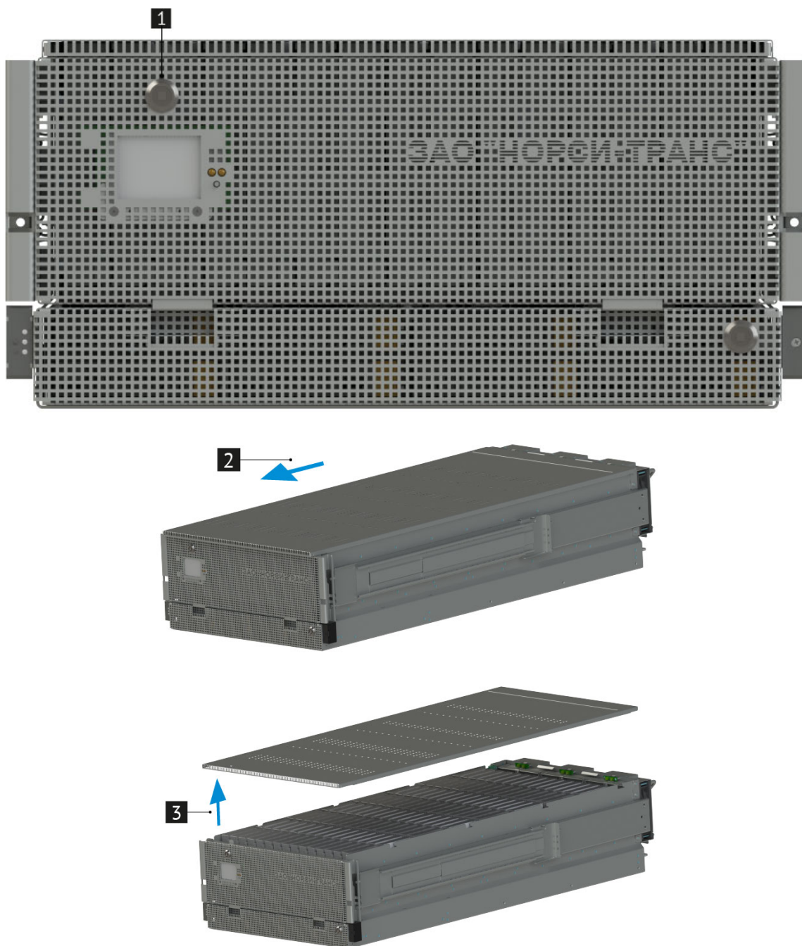
Рис. 18. Снятие верхней крышки платформы
