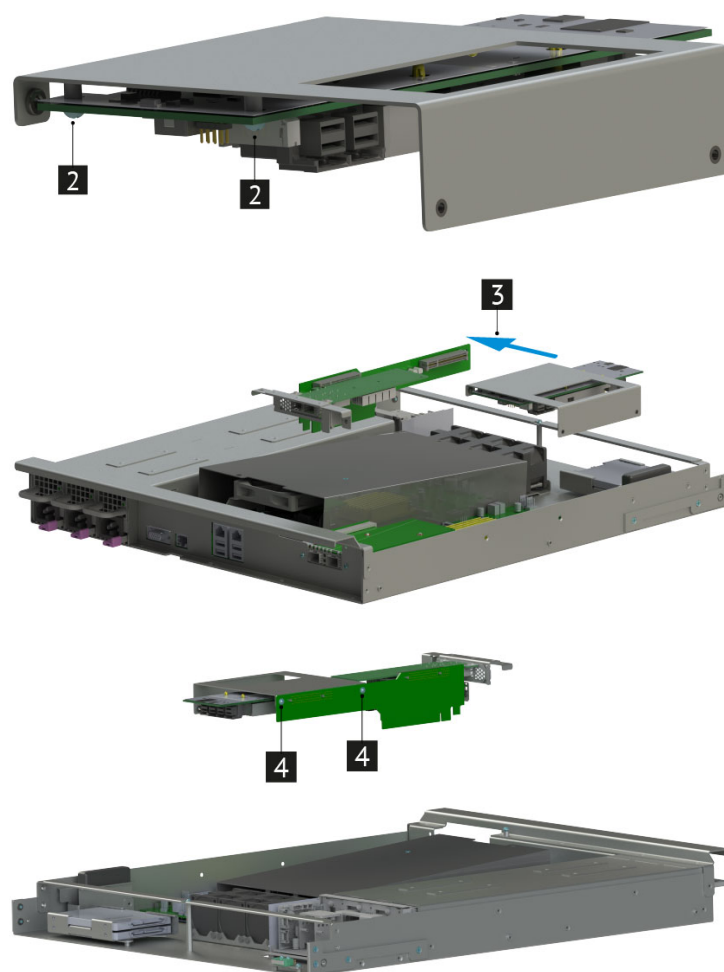
Рис. 53. Установка контроллера дискового SAS-3 RAID-24i
