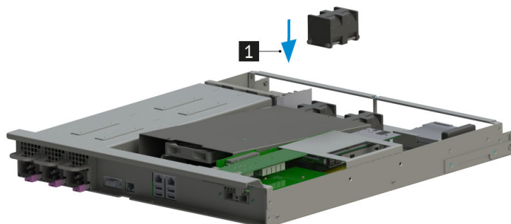
Рис. 27. Подключение вентилятора
