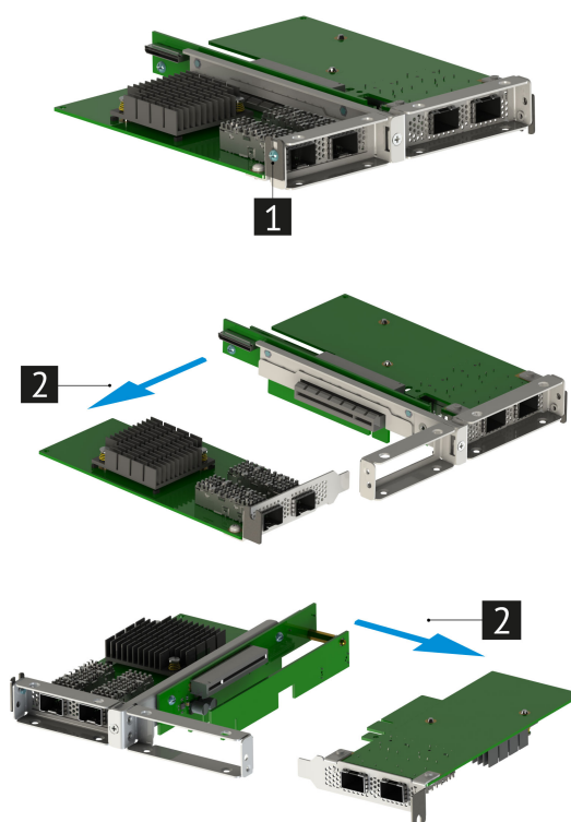
Рис. 51. Извлечение карт расширения
