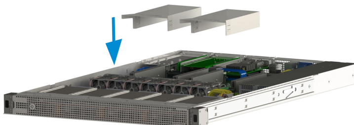
Рис. 23. Установка воздушного кожуха
