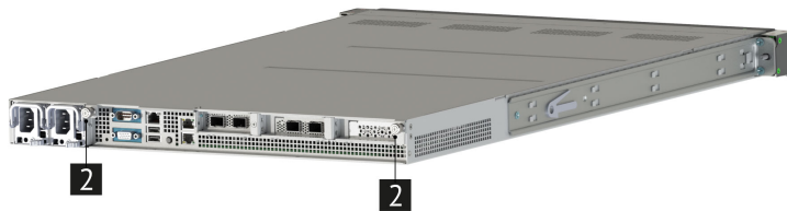
Рис. 21. Установка верхней крышки сервера
