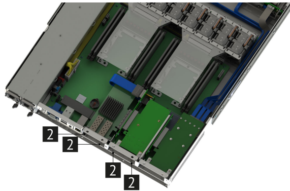
Рис. 48. Установка райзера PCIe 1U x16-x8-x8-Oc
