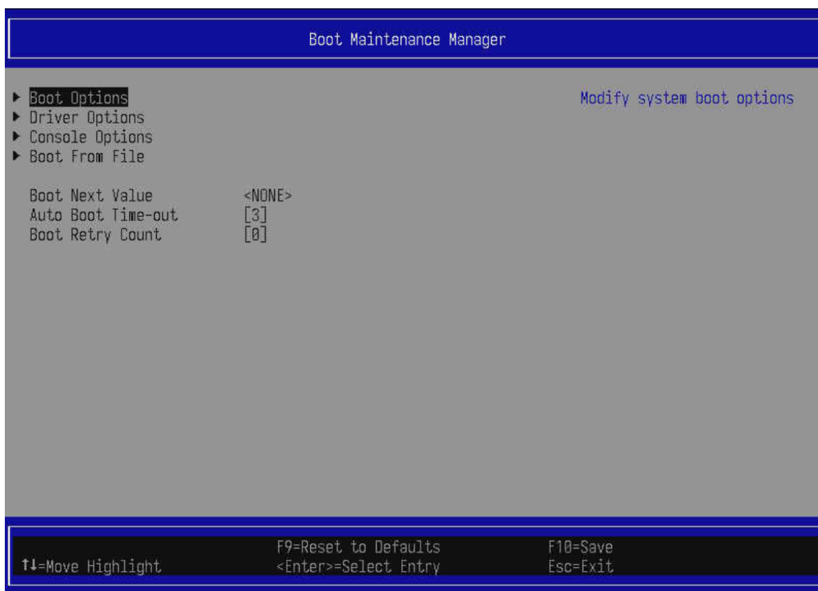
Рис. 67. Раздел меню «Boot Maintenance Manager»
