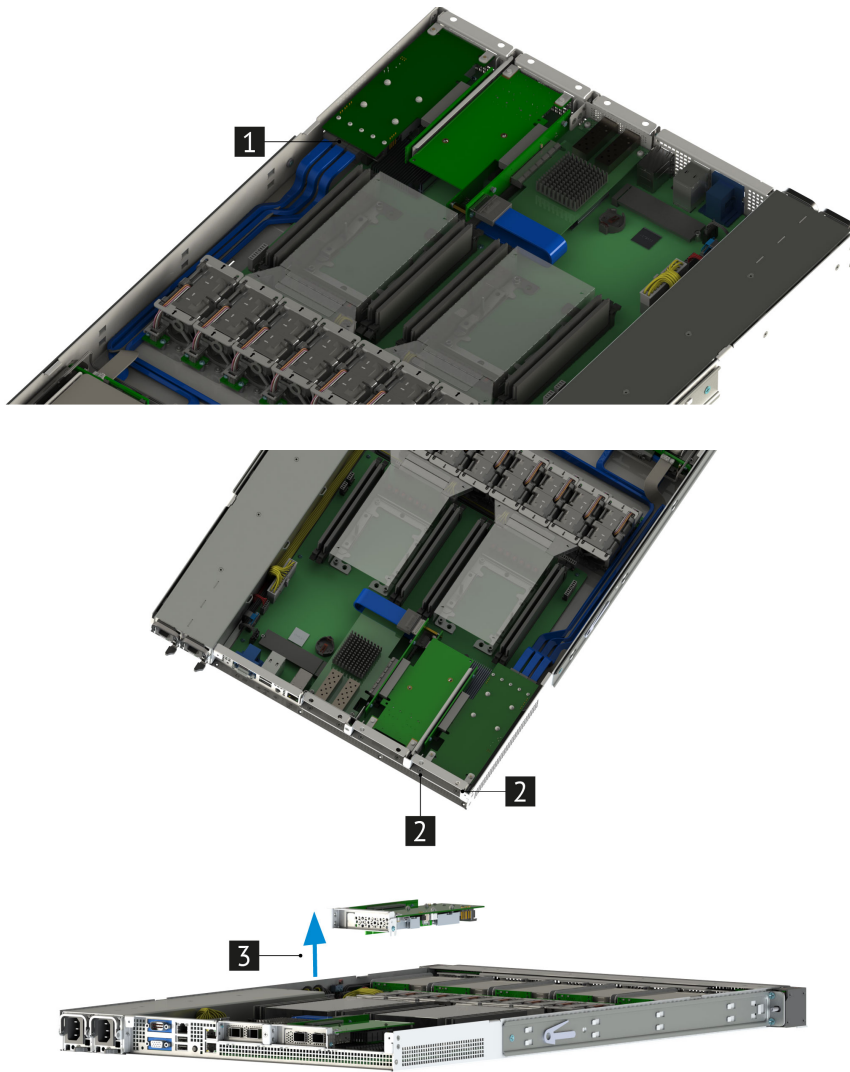
Рис. 45. Извлечение райзера PCIe 1U x8-x8
