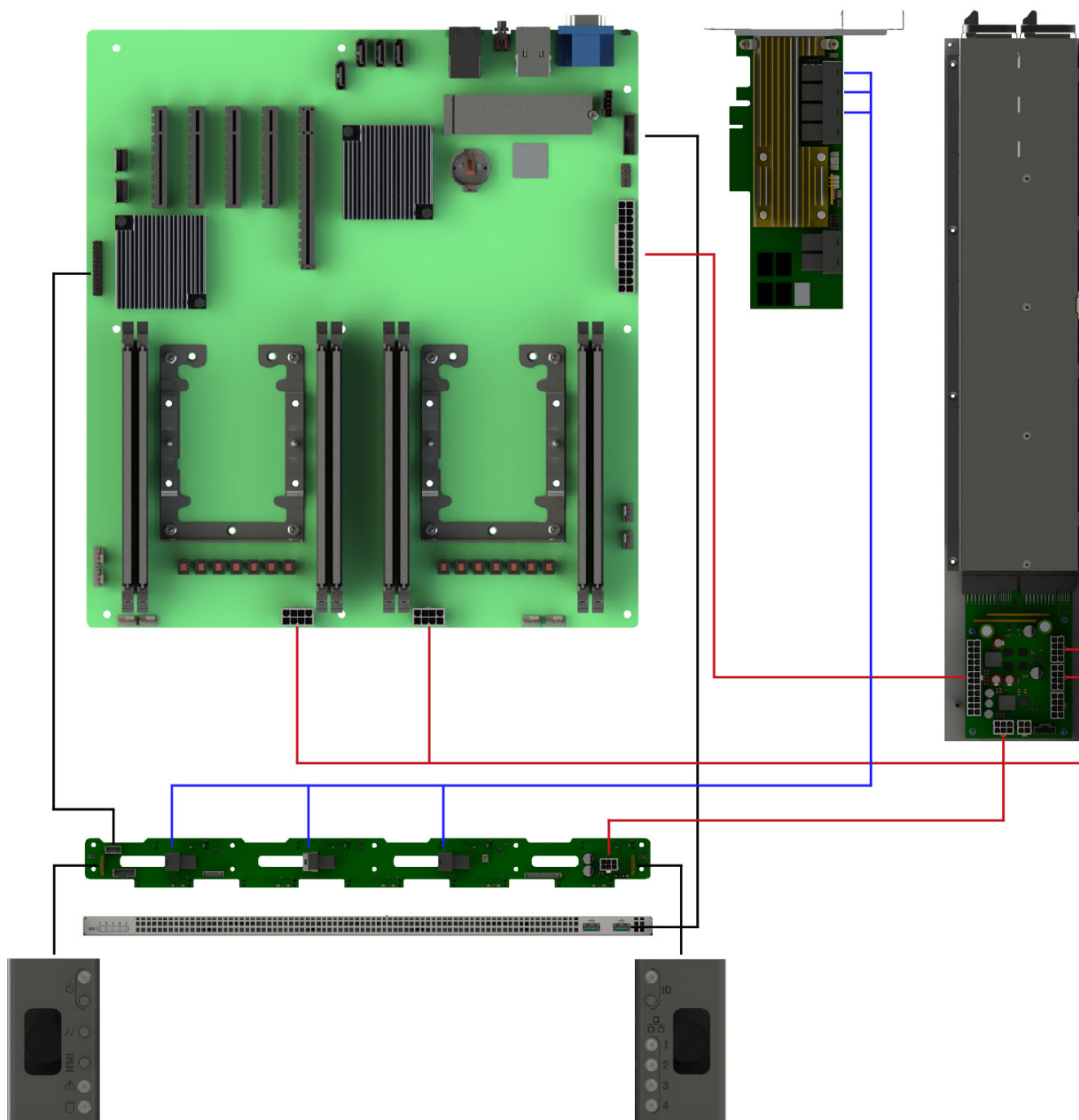
Рис. 25. Схема прокладки системных кабелей и кабелей питания в сервере
