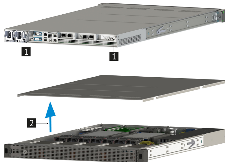
Рис. 20. Снятие верхней крышки сервера
