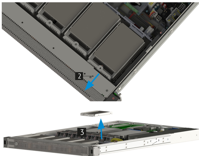
Рис. 40. Извлечение кассеты с SDD диском
