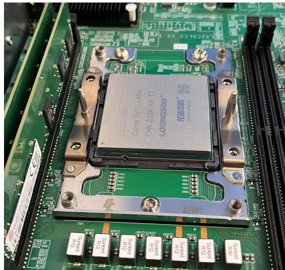
Рис. 35. Установка процессора
