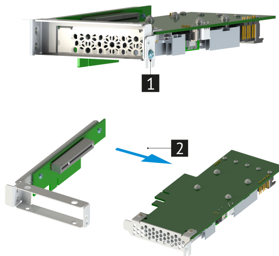
Рис. 49. Извлечение контроллера дискового MegaRAID 9361-16i
