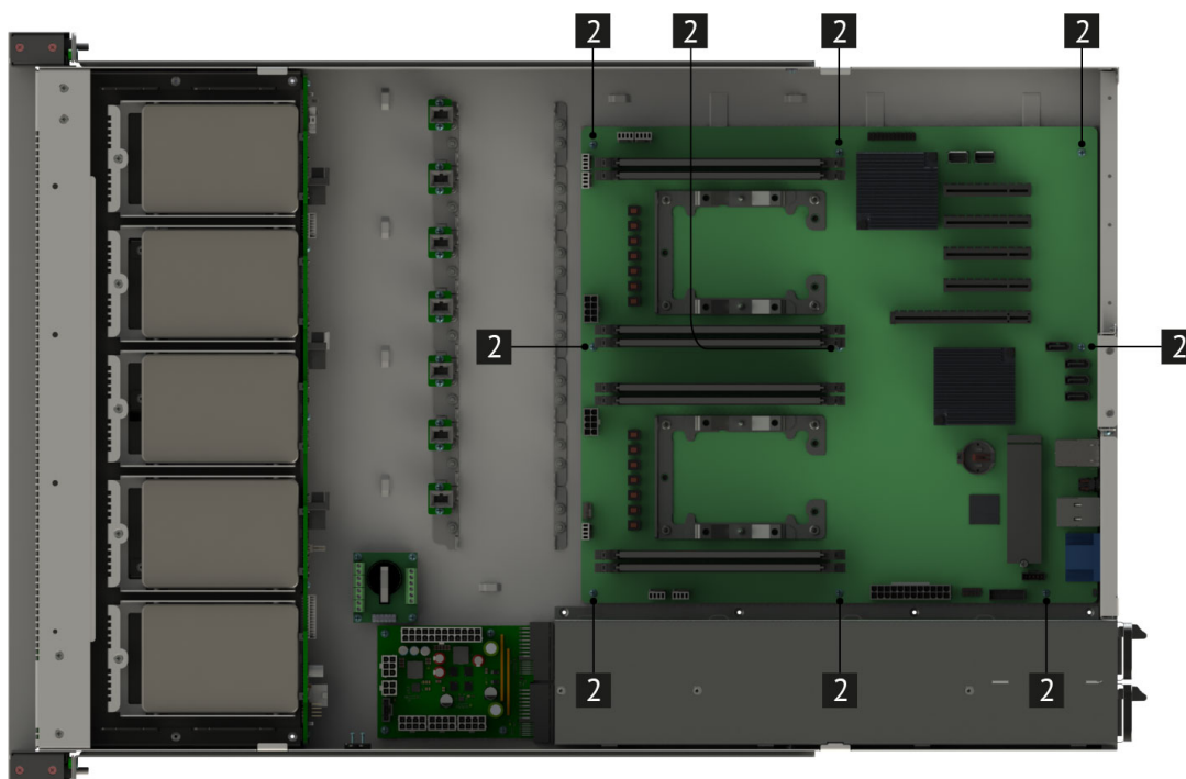
Рис. 37. Установка материнской платы в сервер
