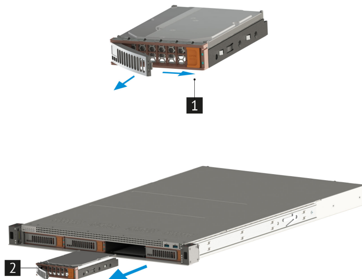
Рис. 38. Извлечение дисков
