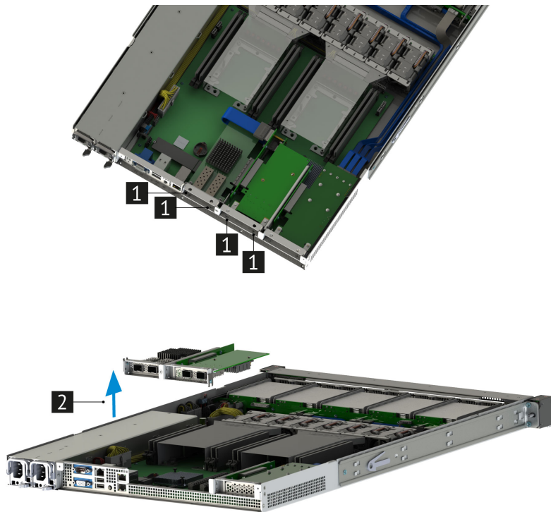
Рис. 47. Извлечение райзера PCIe 1U x16-x8-x8-Ос
