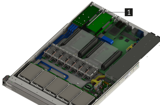
Рис. 44. Расположение райзера PCIe 1U x8-x8 в сервере
