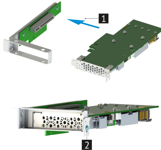
Рис. 50. Установка контроллера дискового MegaRAID 9361-16i
