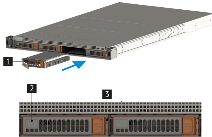
Рис. 39. Установка дисков
