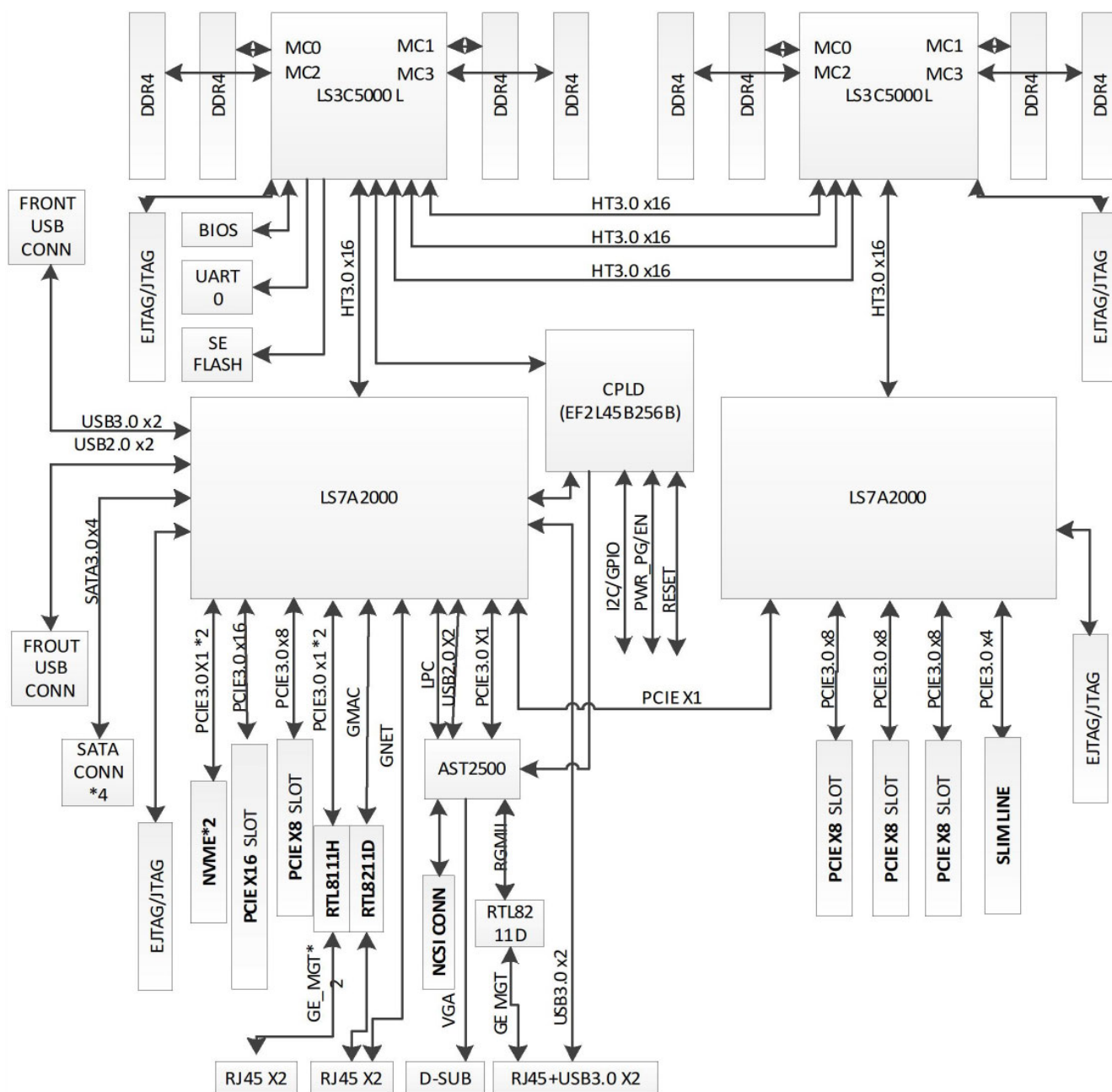
Рис. 1. Структурная схема материнской платы НТ «Дракон 2С-3С5» НИКА.469555.003
