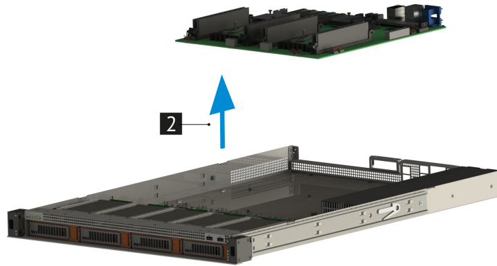
Рис. 36. Извлечение материнской платы из сервера
