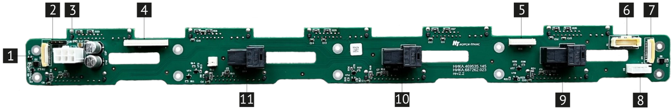
Рис. 11. Плата расширения 4LFF, 5SFF (НИКА.469535.145)
