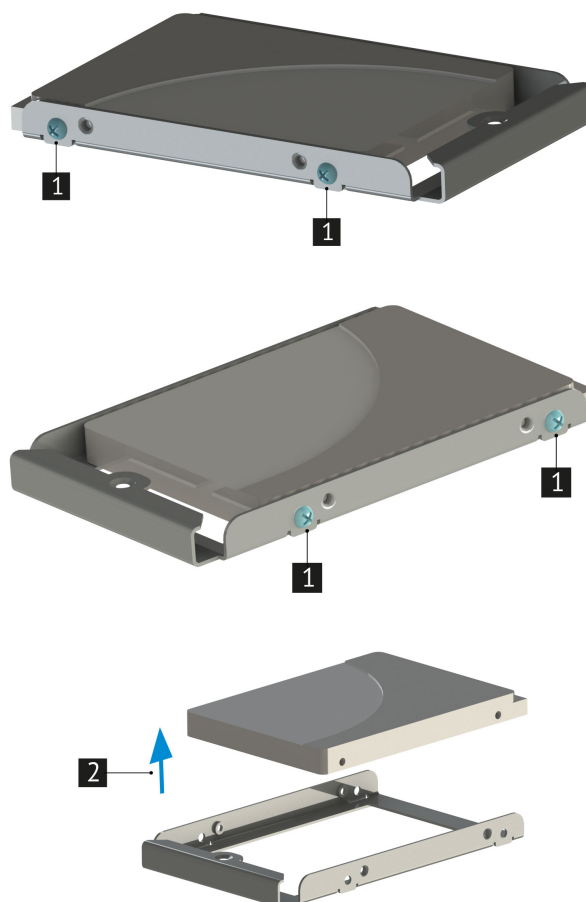
Рис. 42. Извлечение SDD диска из кассеты
