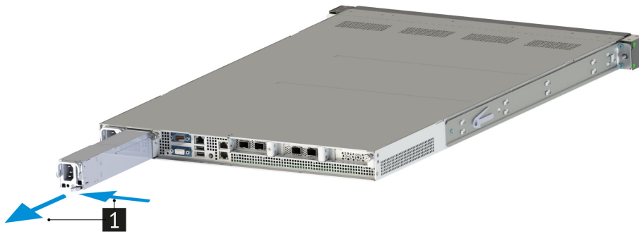
Рис. 54. Извлечение блока питания из сервера
