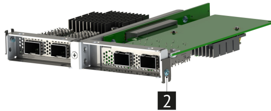
Рис. 52. Установка карт расширения
