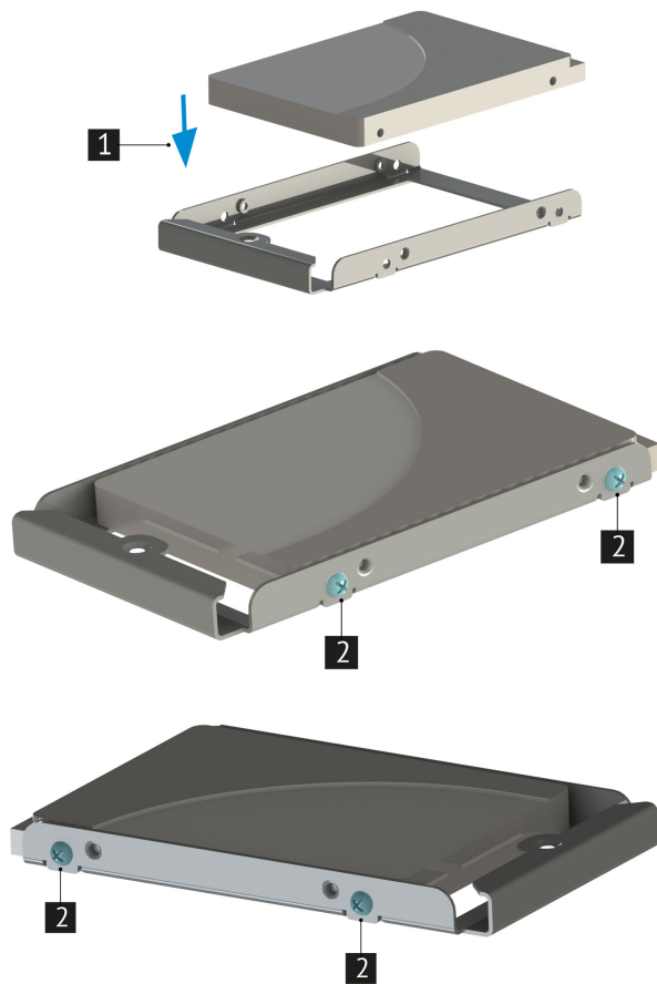
Рис. 43. Установка SSD диска в кассету
