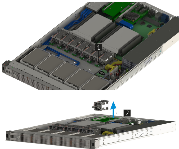
Рис. 26. Извлечение вентилятора из сервера
