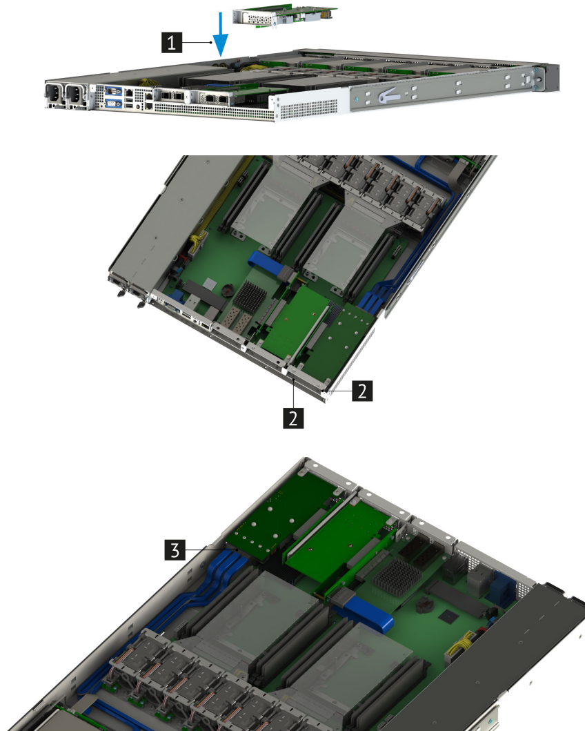
Рис. 46. Установка райзера PCIe 1U x8-x8
