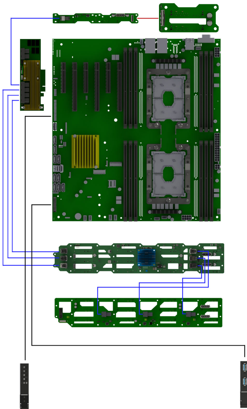
Рис. 34. Схема прокладки системных кабелей и кабелей питания
