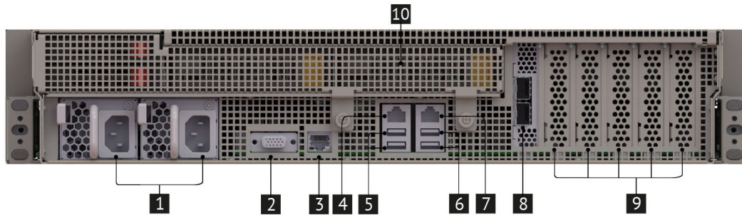
Рис. 5. Вид сервера сзади
