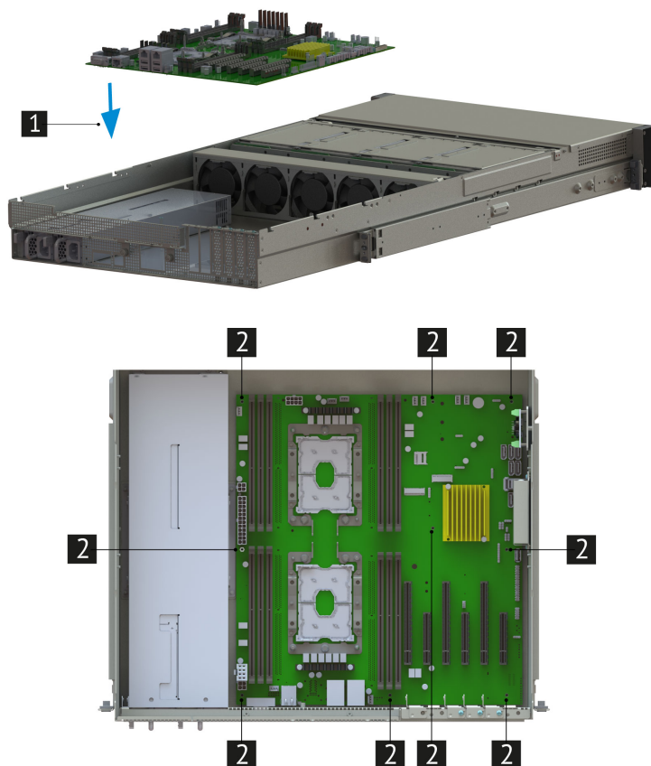
Рис. 49. Установка материнской платы
