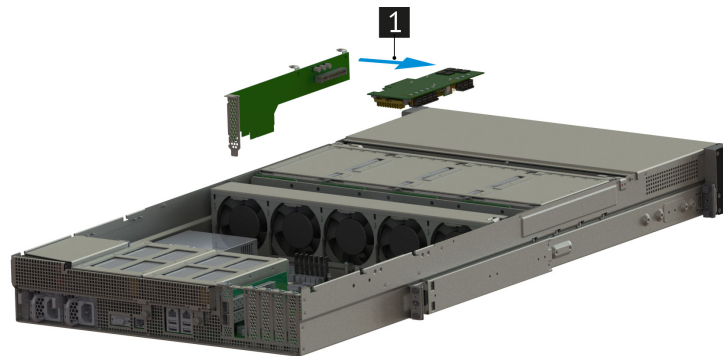
Рис. 59. Извлечение MegaRAID SAS 9361-24i из адаптера поворотного НИКА.469535.023
