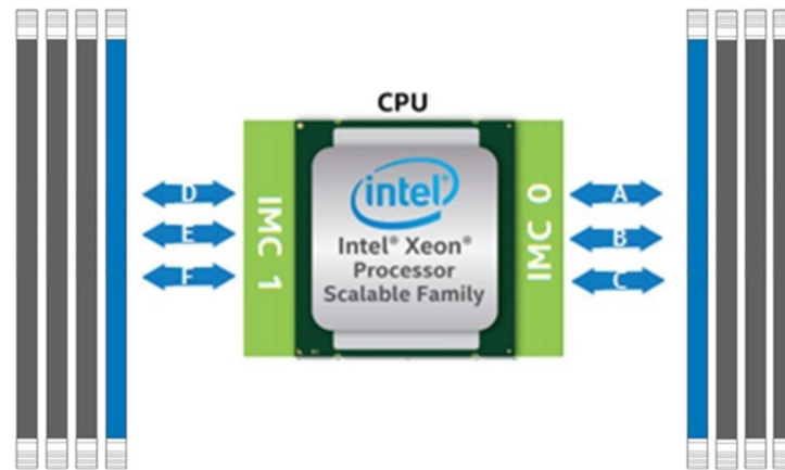
Рис. 38. Каналы памяти
