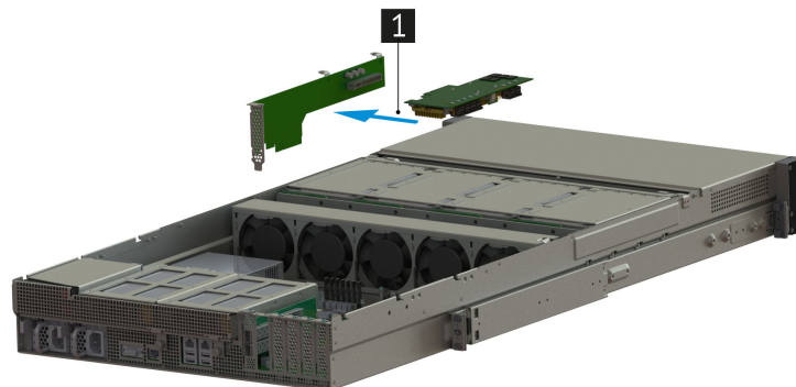
Рис. 60. Установка MegaRAID SAS 9361-24i в адаптер поворотный НИКА.469535.023
