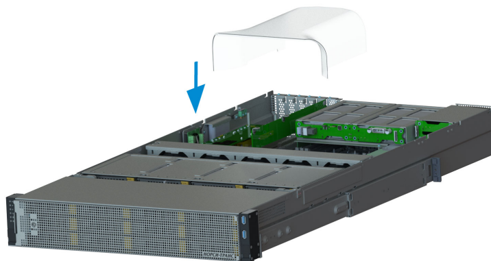
Рис. 30. Установка воздушного кожуха
