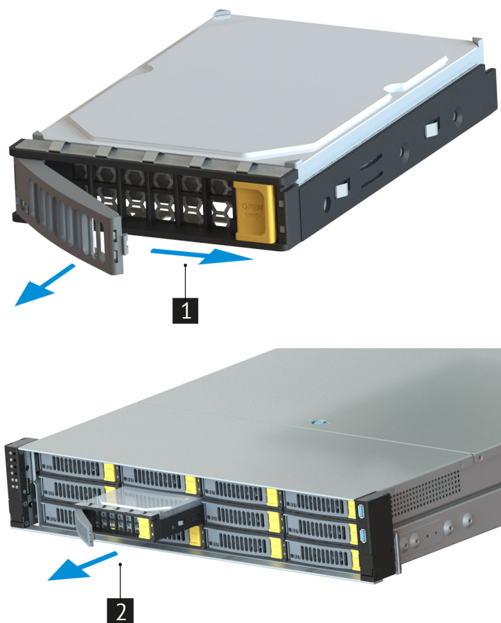
Рис. 50. Извлечение дисков
