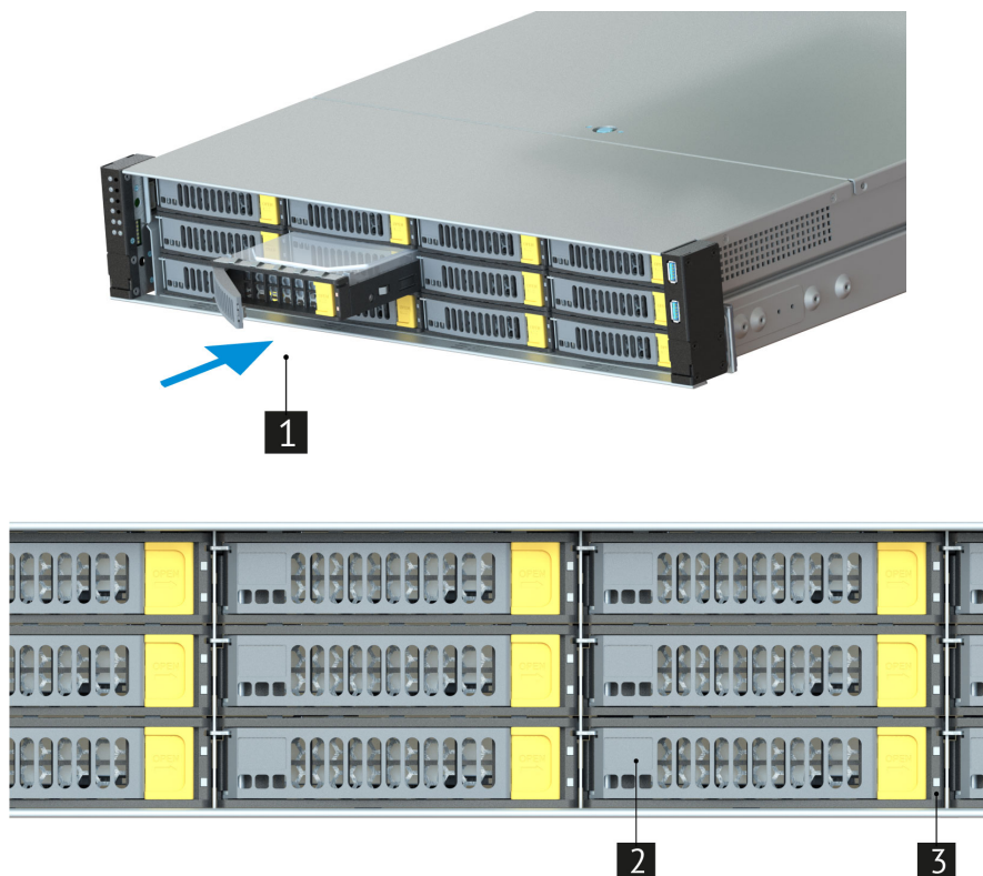
Рис. 51. Извлечение дисков
