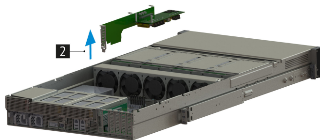
Рис. 57. Извлечение адаптера поворотного НИКА.469535.023
