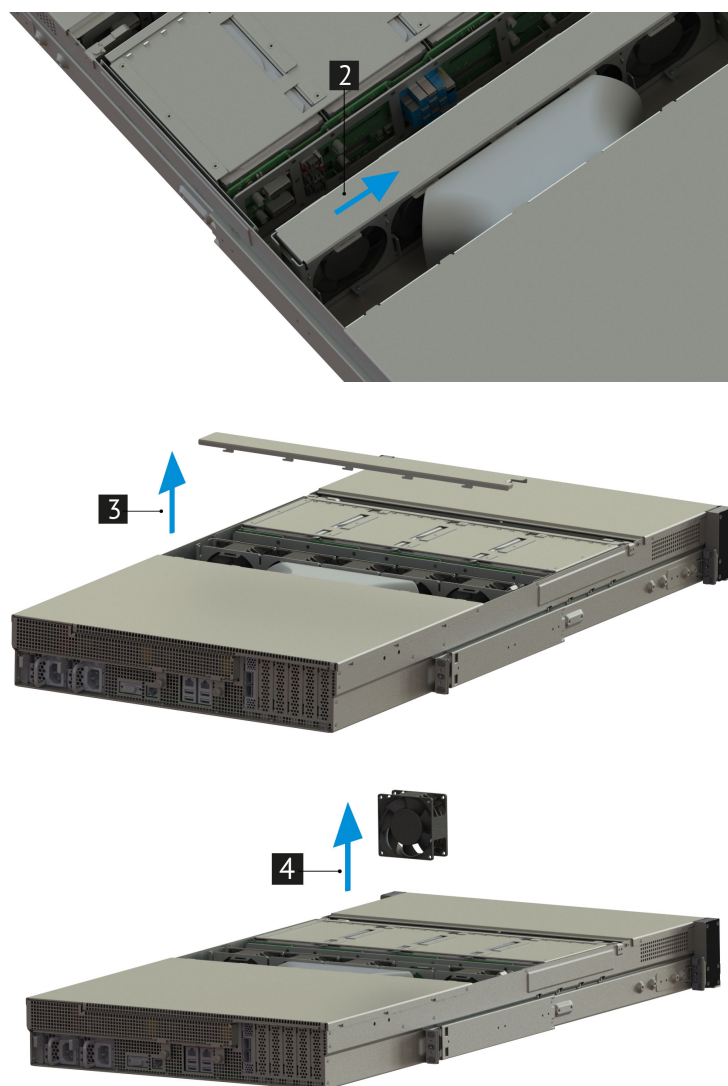
Рис. 35. Извлечение вентилятора
