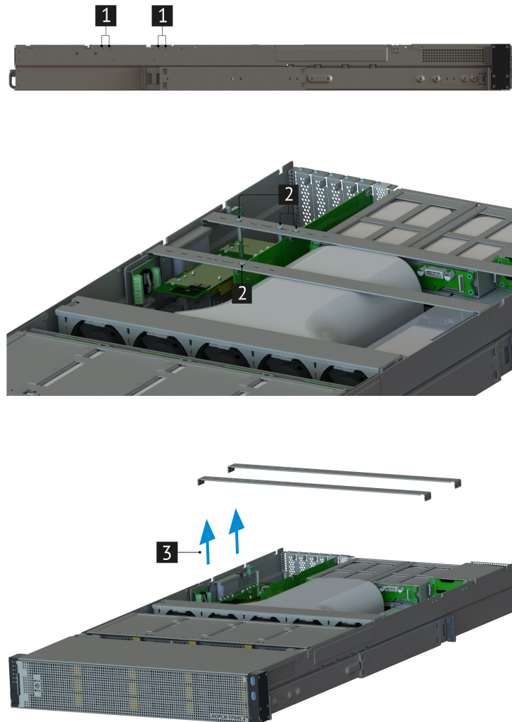
Рис. 27. Снятие скоб
