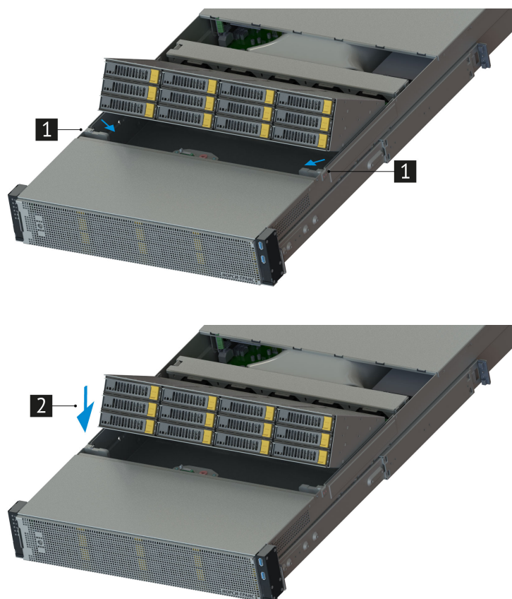
Рис. 24. Установка внутренней дисковой кассеты/поворотной кассеты
