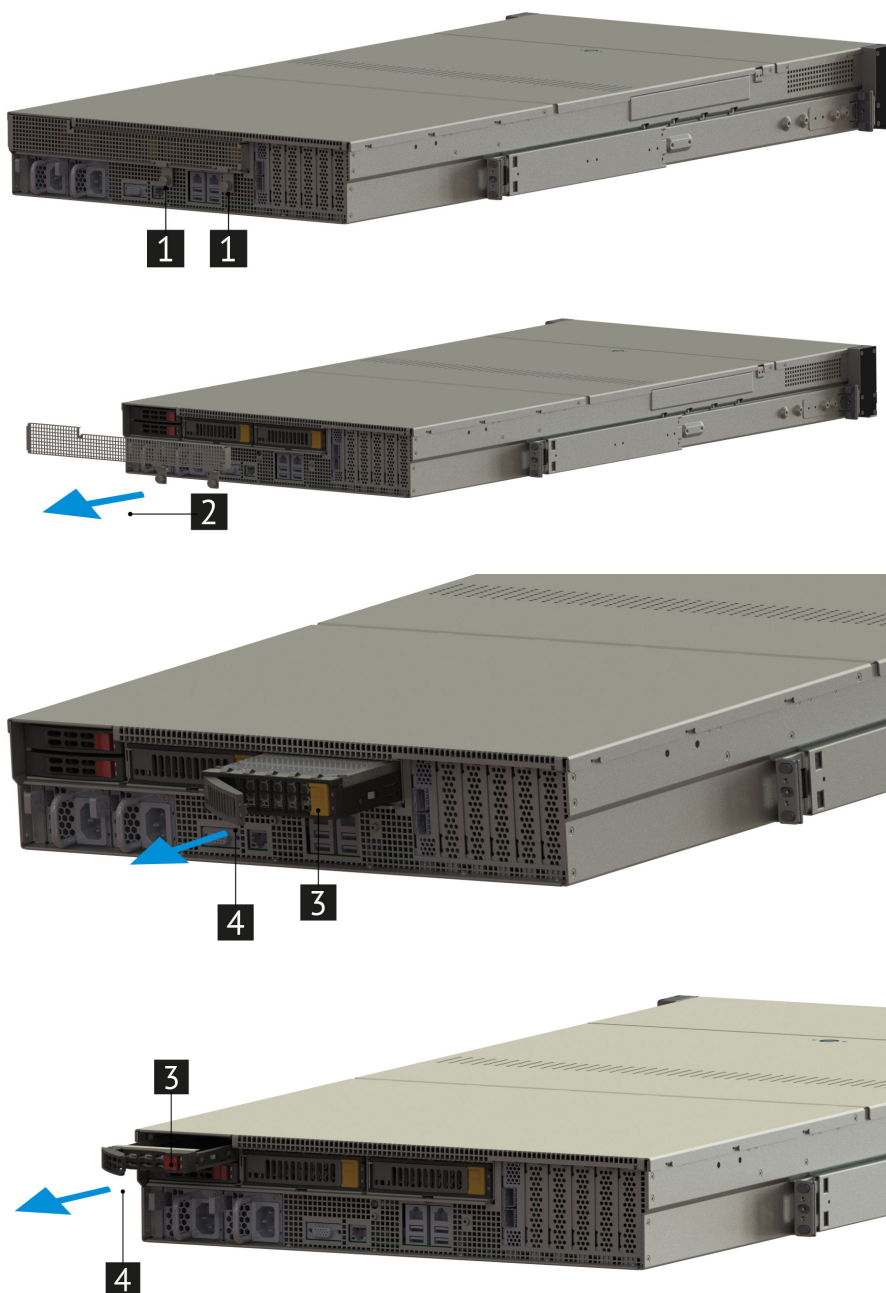
Рис. 54. Извлечение дисков
