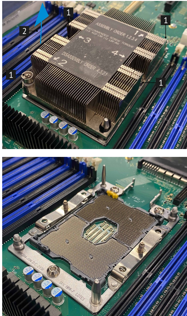
Рис. 43. Снятие модуля процессора с радиатором
