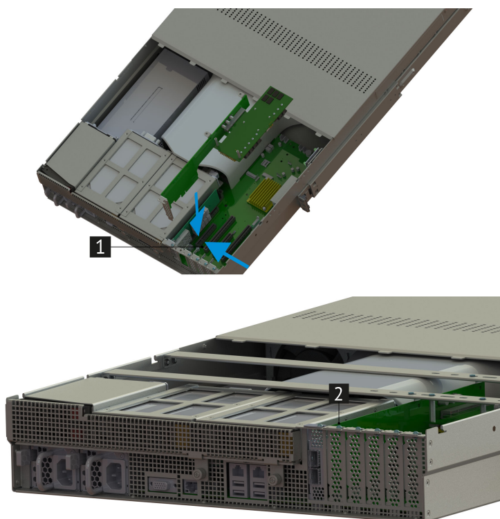
Рис. 58. Установка адаптера поворотного НИКА.469535.023
