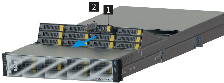
Рис. 52. Извлечение дисков
