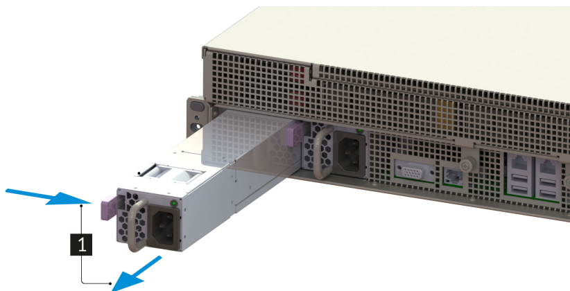
Рис. 62. Извлечение блока питания
