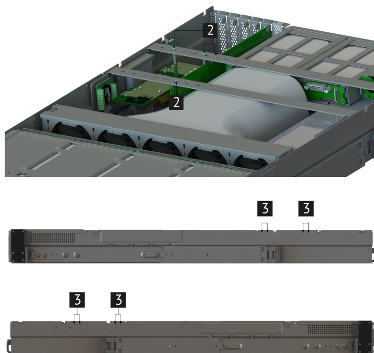
Рис. 28. Установка скоб
