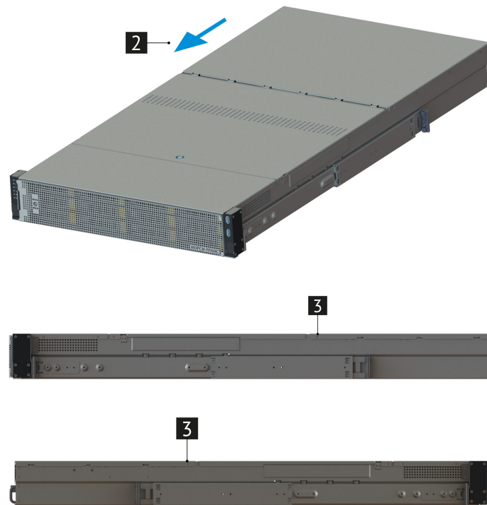
Рис. 26. Установка задней крышки платформы
