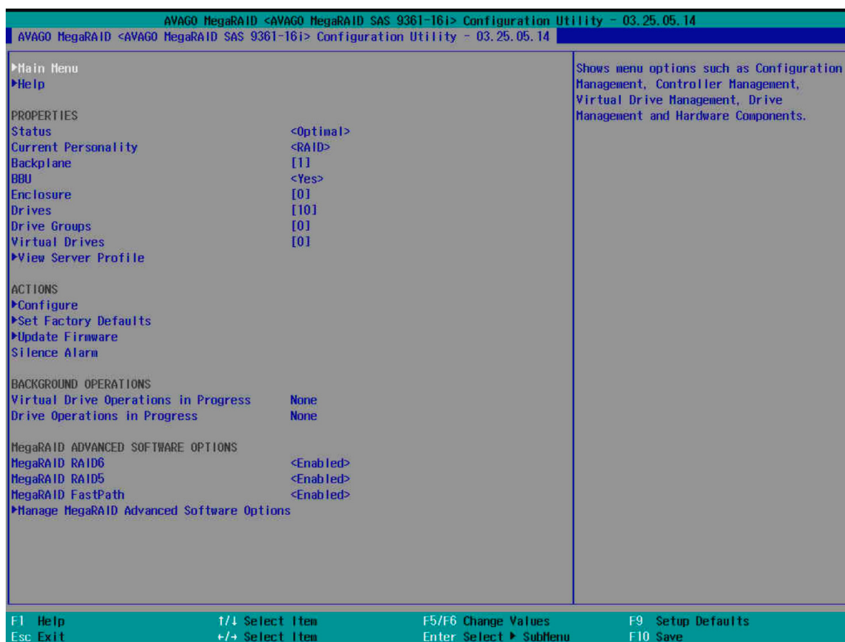
Рис. 77. Меню «AVAGO MegaRAID»
