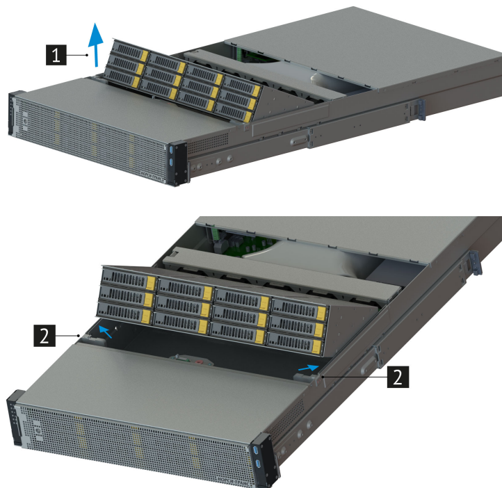
Рис. 23. Извлечение внутренней дисковой кассеты/поворотной кассеты
