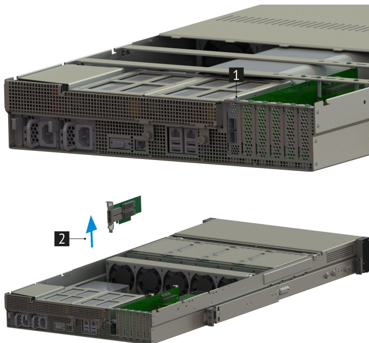
Рис. 55. Снятие карты расширения
