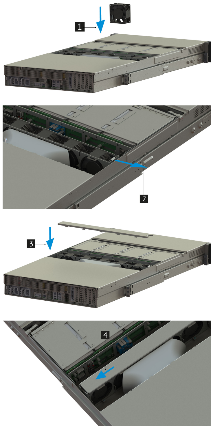
Рис. 36. Подключение вентилятора
