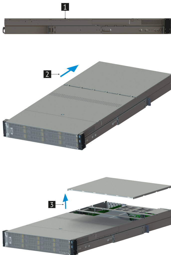
Рис. 25. Снятие задней крышки платформы
