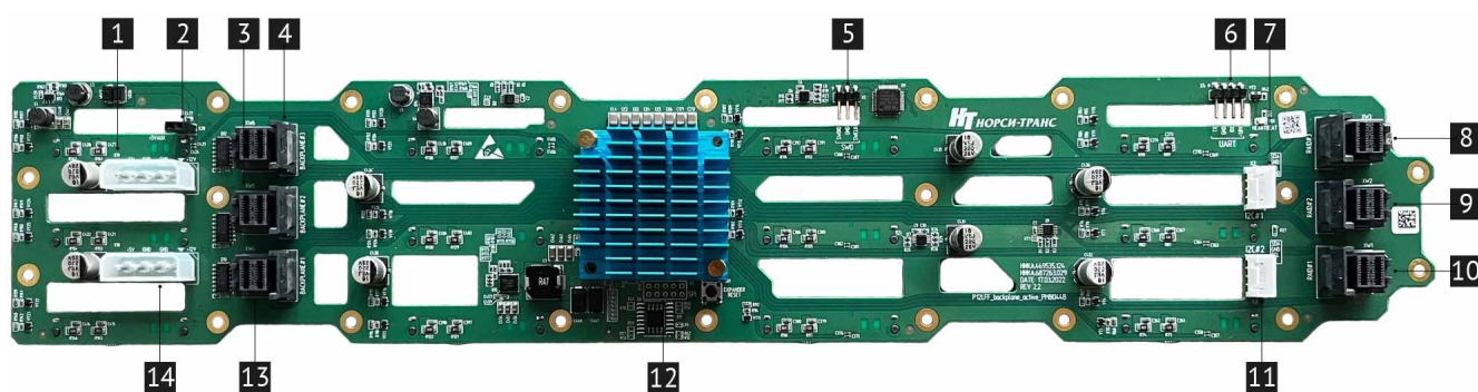
Рис. 14. Плата расширения 12LFF (НИКА.469535.124)
