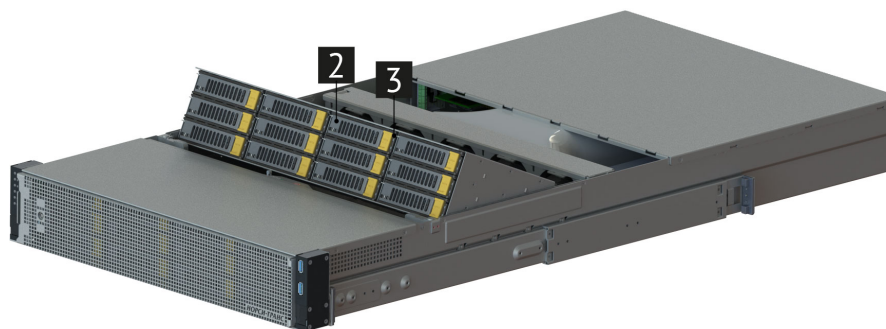
Рис. 53. Извлечение дисков
