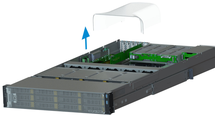
Рис. 29. Снятие воздушного кожуха
