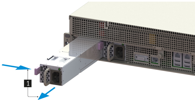
Рис. 64. Извлечение блока питания
