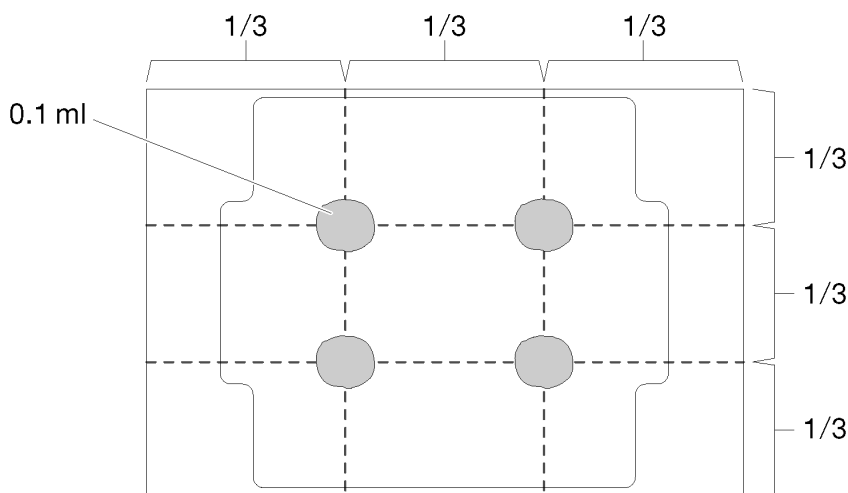
Рис. 47. Нанесение термопасты
