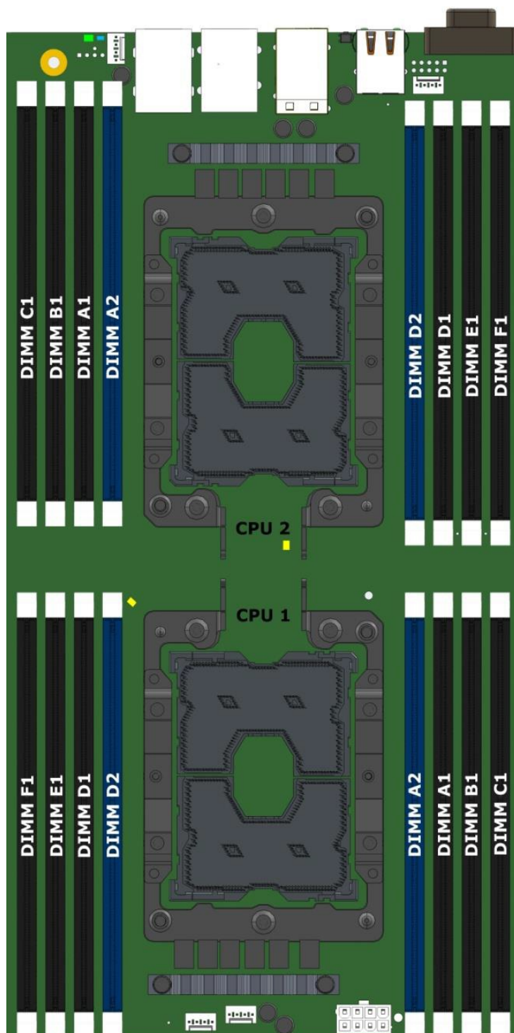
Рис. 37. Расположение разъемов
