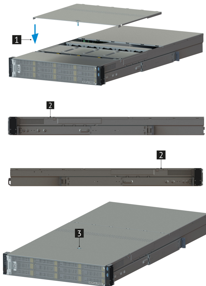
Рис. 22. Установка средней крышки платформы
