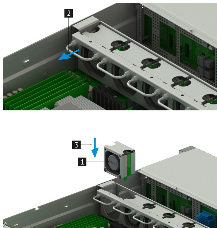
Рис. 37. Подключение вентилятора
