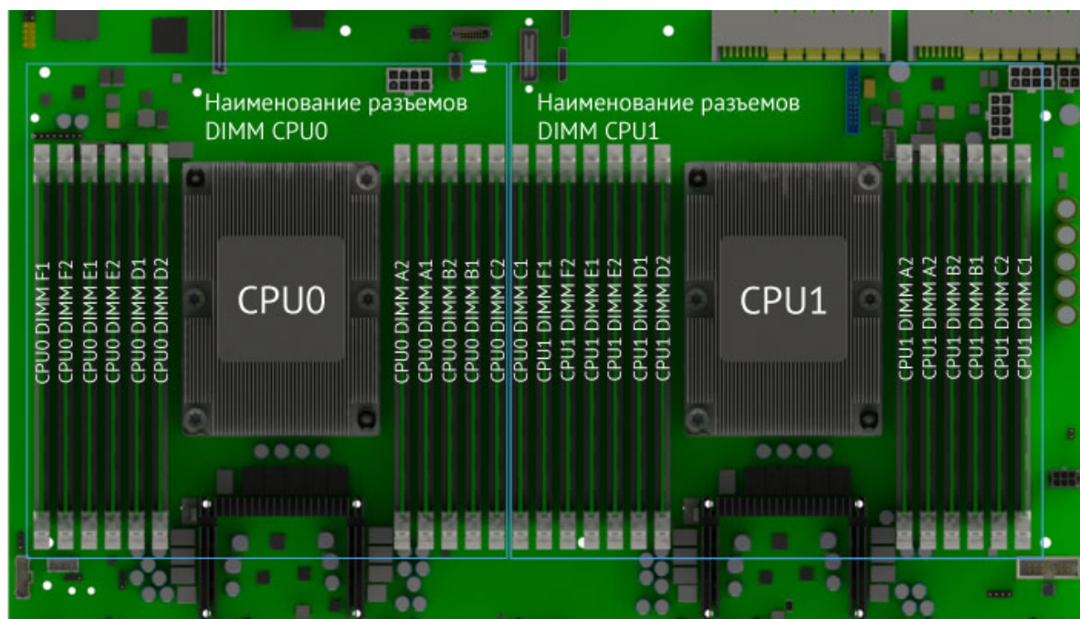
Рис. 38. Расположение разъемов
