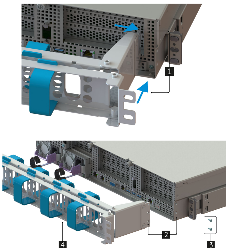
Рис. 24. Установка дополнительного кабельного органайзера
