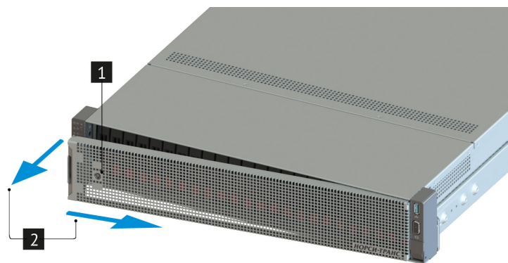
Рис. 25. Снятие передней панели
