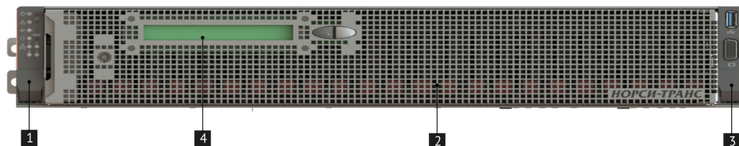
Рис. 2. Вид сервера спереди с информационной панелью
