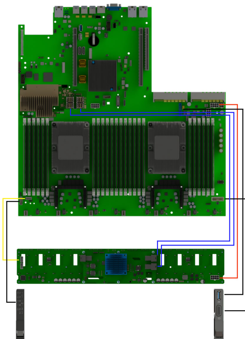
Рис. 33. Схема прокладки системных кабелей и кабелей питания с подключением наплатного RAID
