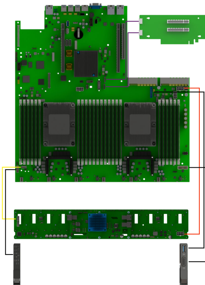
Рис. 35. Схема прокладки системных кабелей и кабелей OcuLink только в случае подключения Райзера 3x16-8-8 (НИКА.469535.047)
