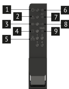
Рис. 4. Левая панель управления
