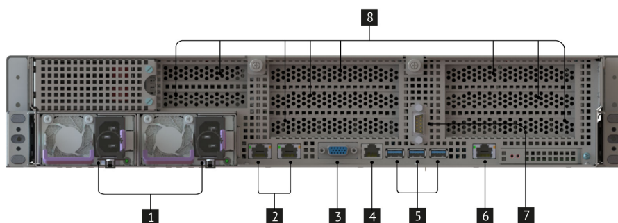
Рис. 6. Вид сервера сзади
