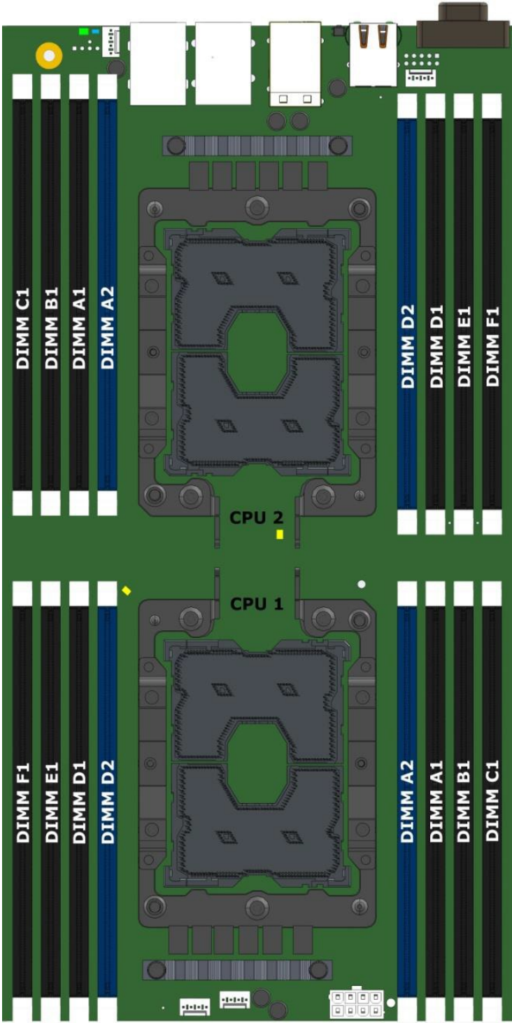
Рис. 37. Расположение разъемов
