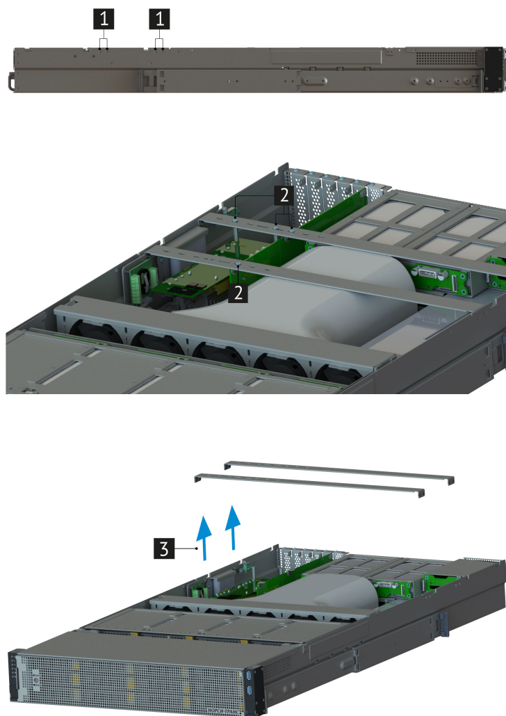
Рис. 27. Снятие скоб
