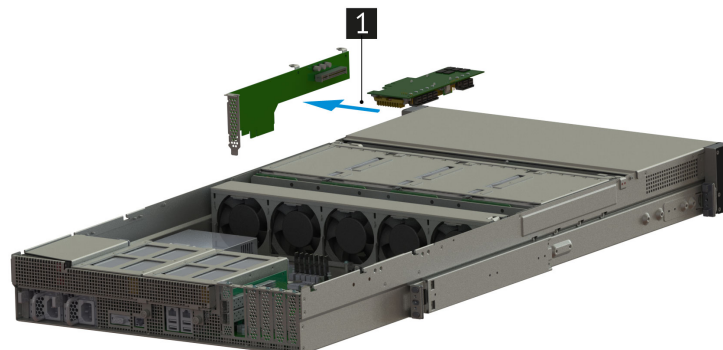
Рис. 60. Установка MegaRAID SAS 9361-24i в адаптер поворотный НИКА.469535.023
