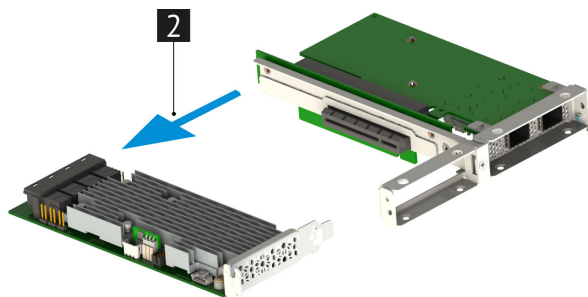
Рис. 54. Извлечение контроллера дискового MegaRAID 9361-16i
