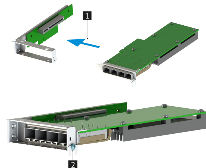
Рис. 57. Установка карты расширения
