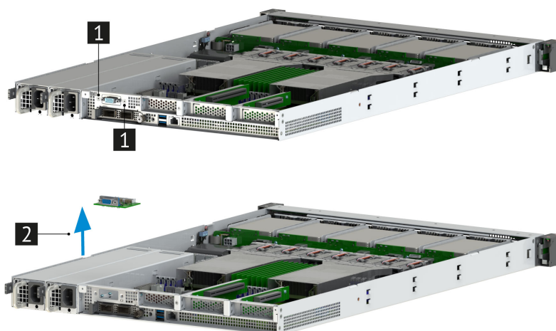
Рис. 60. Извлечение карты VGA
