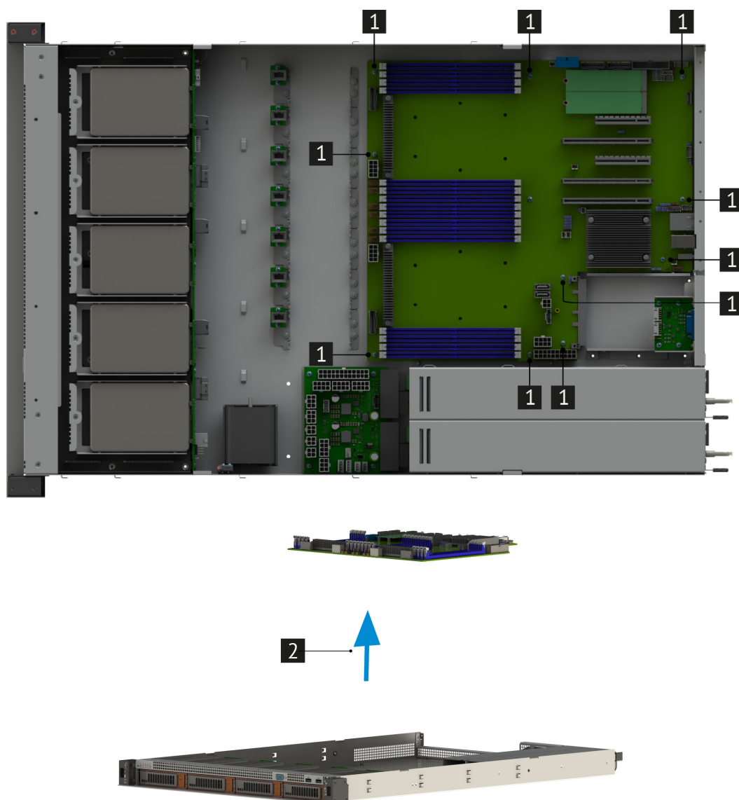
Рис. 40. Извлечение материнской платы из сервера
