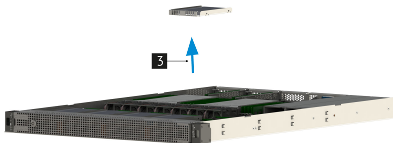
Рис. 46. Извлечение кассеты с SSD диском
