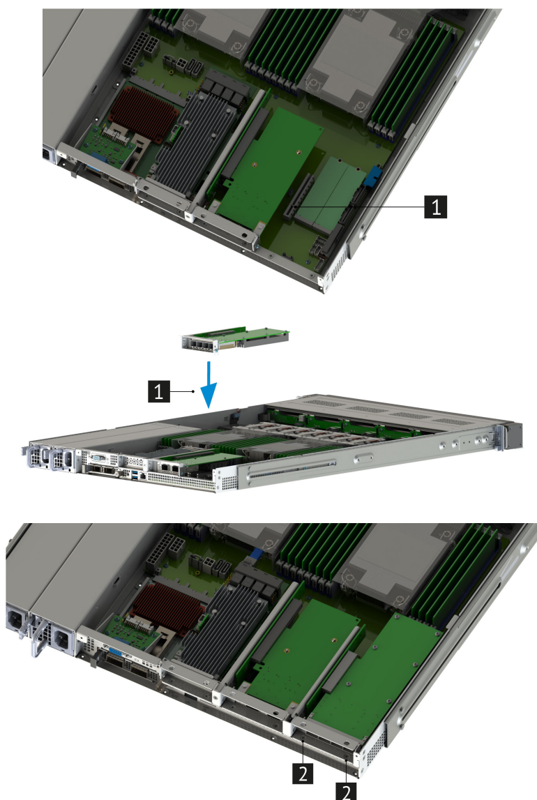
Рис. 51. Установка райзера PCIe 1U x8-x8
