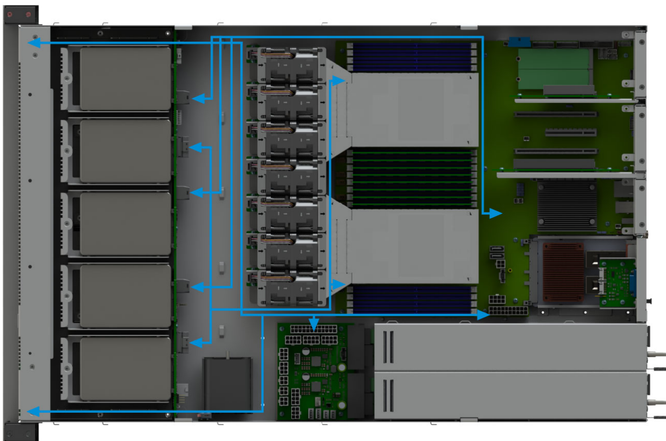
Рис. 26. Схема прокладки кабелей в сервере
