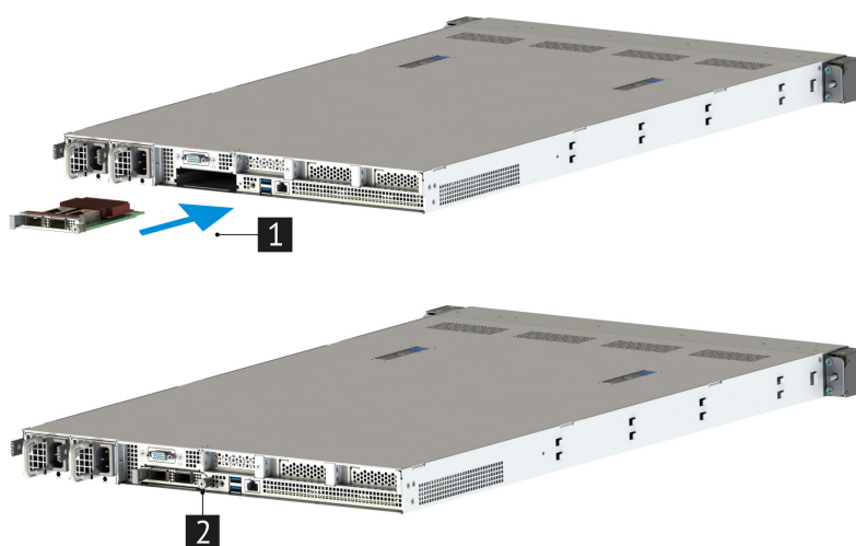
Рис. 63. Установка карты OCP 3.0 PCIe x16
