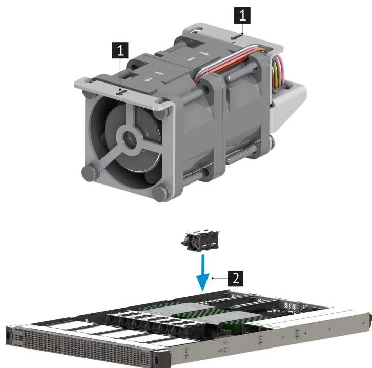
Рис. 31. Подключение вентилятора
