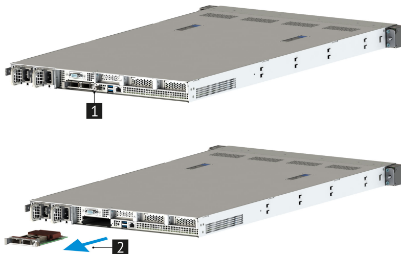
Рис. 62. Извлечение карты OCP 3.0 PCIe x16
