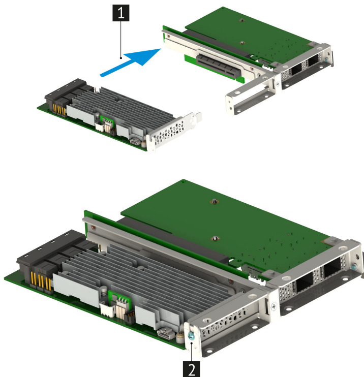
Рис. 55. Установка контроллера дискового MegaRAID 9361-16i
