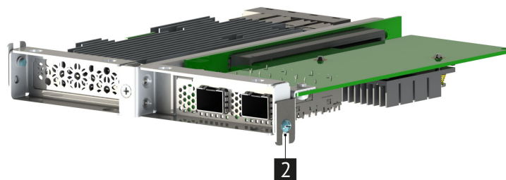
Рис. 59. Установка карты расширения
