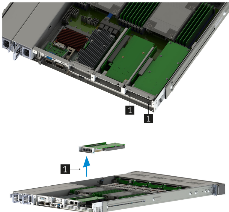
Рис. 50. Извлечение райзера PCIe 1U x8-x8
