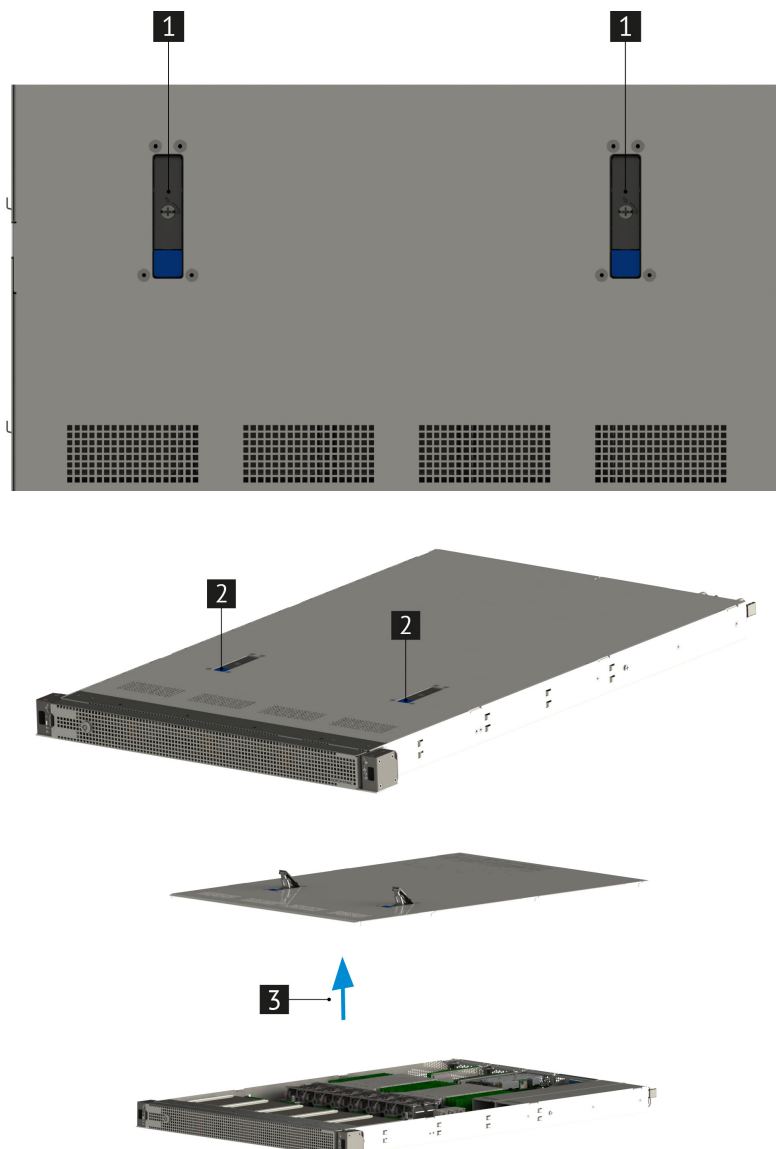
Рис. 22. Снятие верхней крышки сервера
