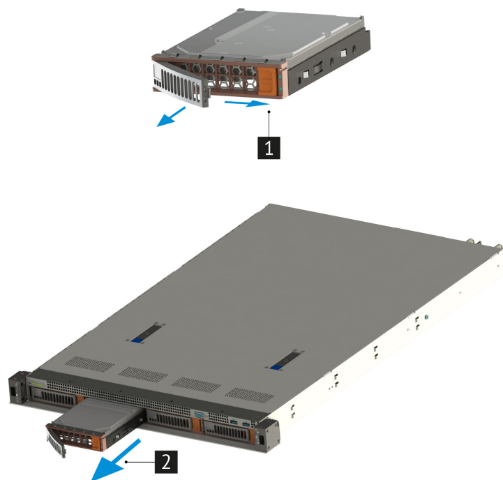
Рис. 42. Извлечение дисков
