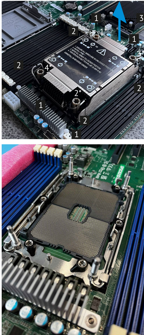
Рис. 36. Снятие модуля процессора с радиатором
