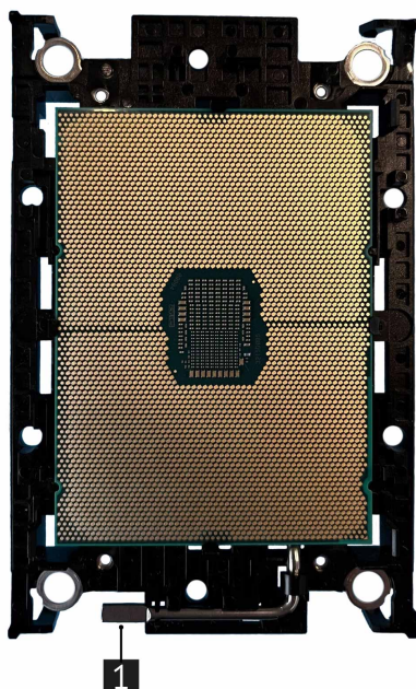
Рис. 38. Снятие процессора с радиатора
