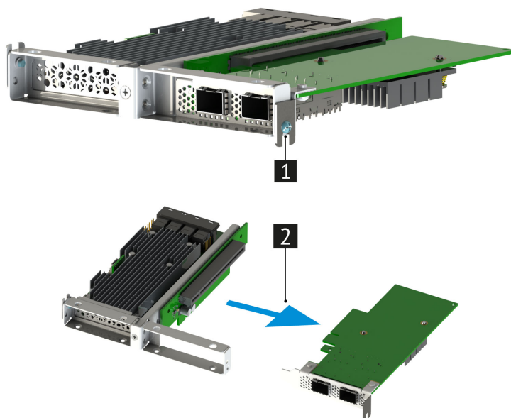
Рис. 58. Извлечение карты расширения
