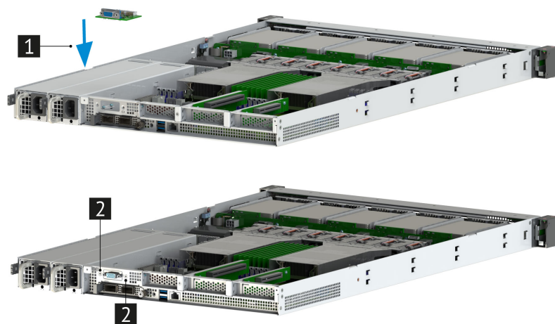
Рис. 61. Установка карты VGA
