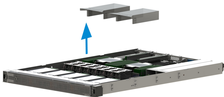
Рис. 24. Извлечение воздушного кожуха
