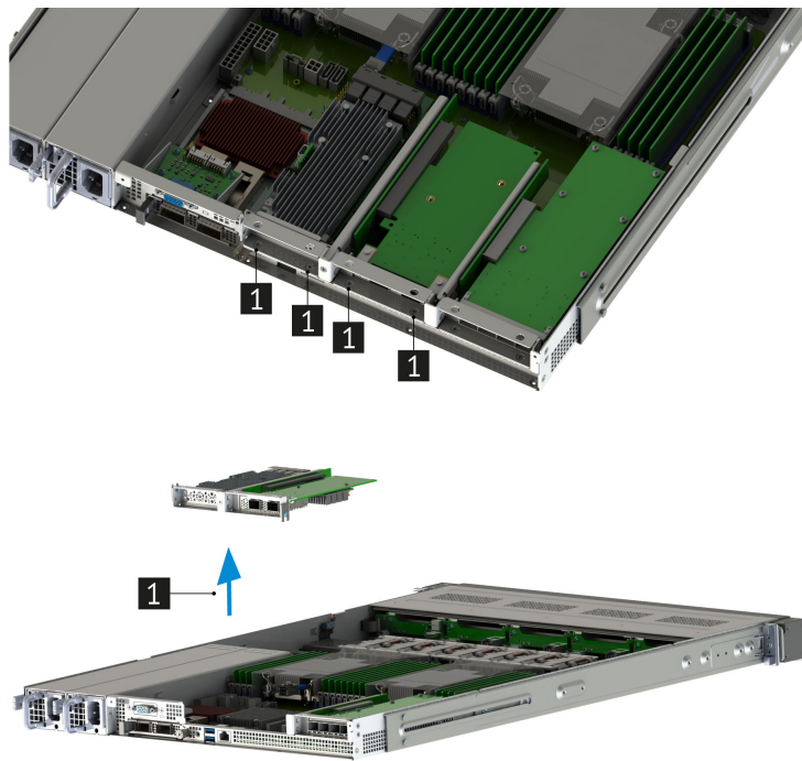
Рис. 52. Извлечение райзера PCIe 1U x16-x8-x16
