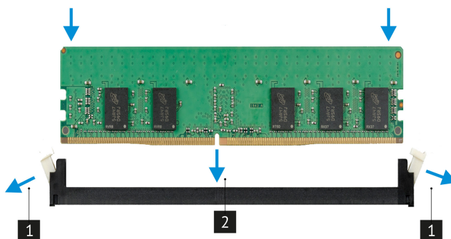
Рис. 34. Установка модуля ОЗУ.
