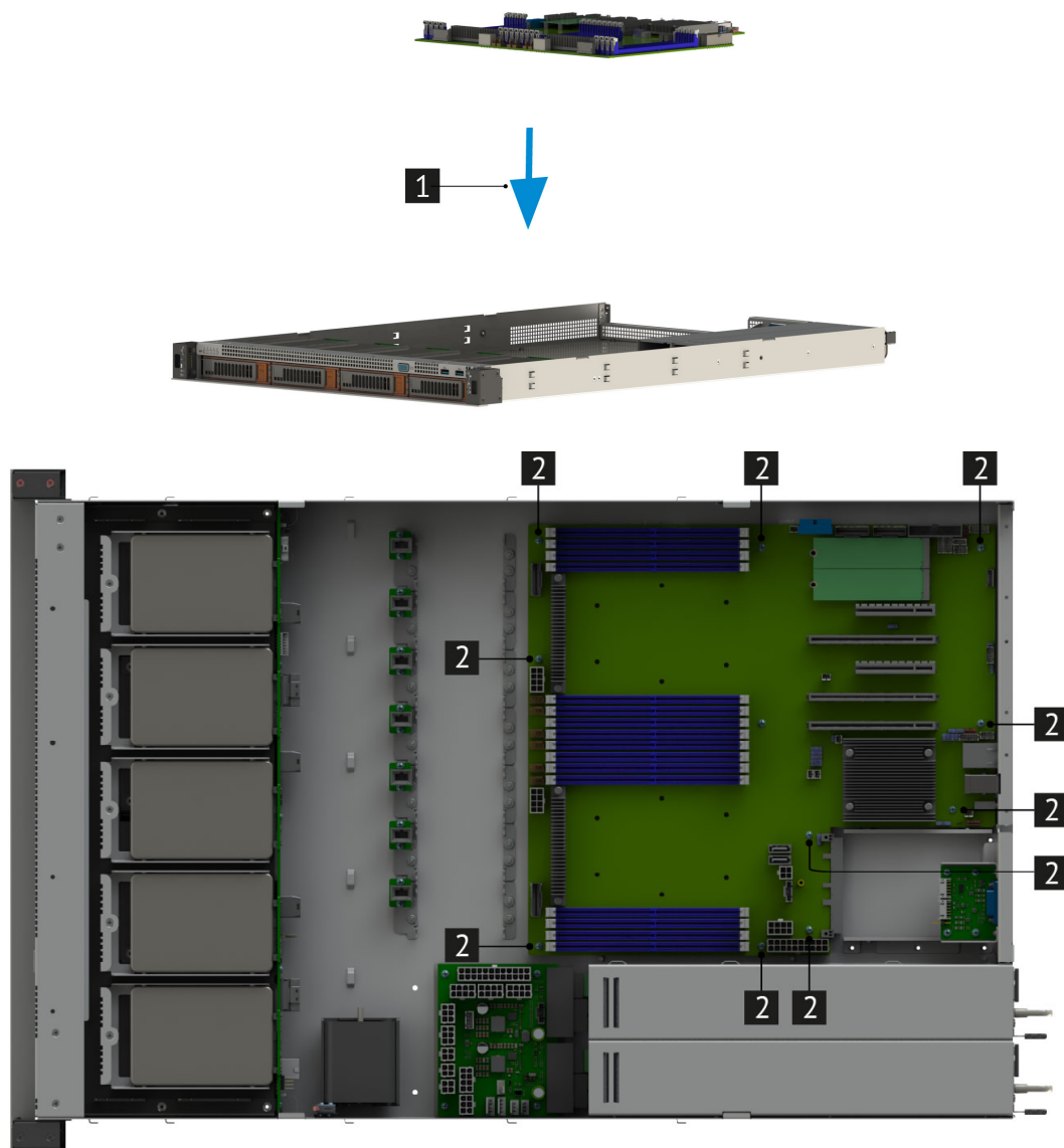
Рис. 41. Установка материнской платы в сервер
