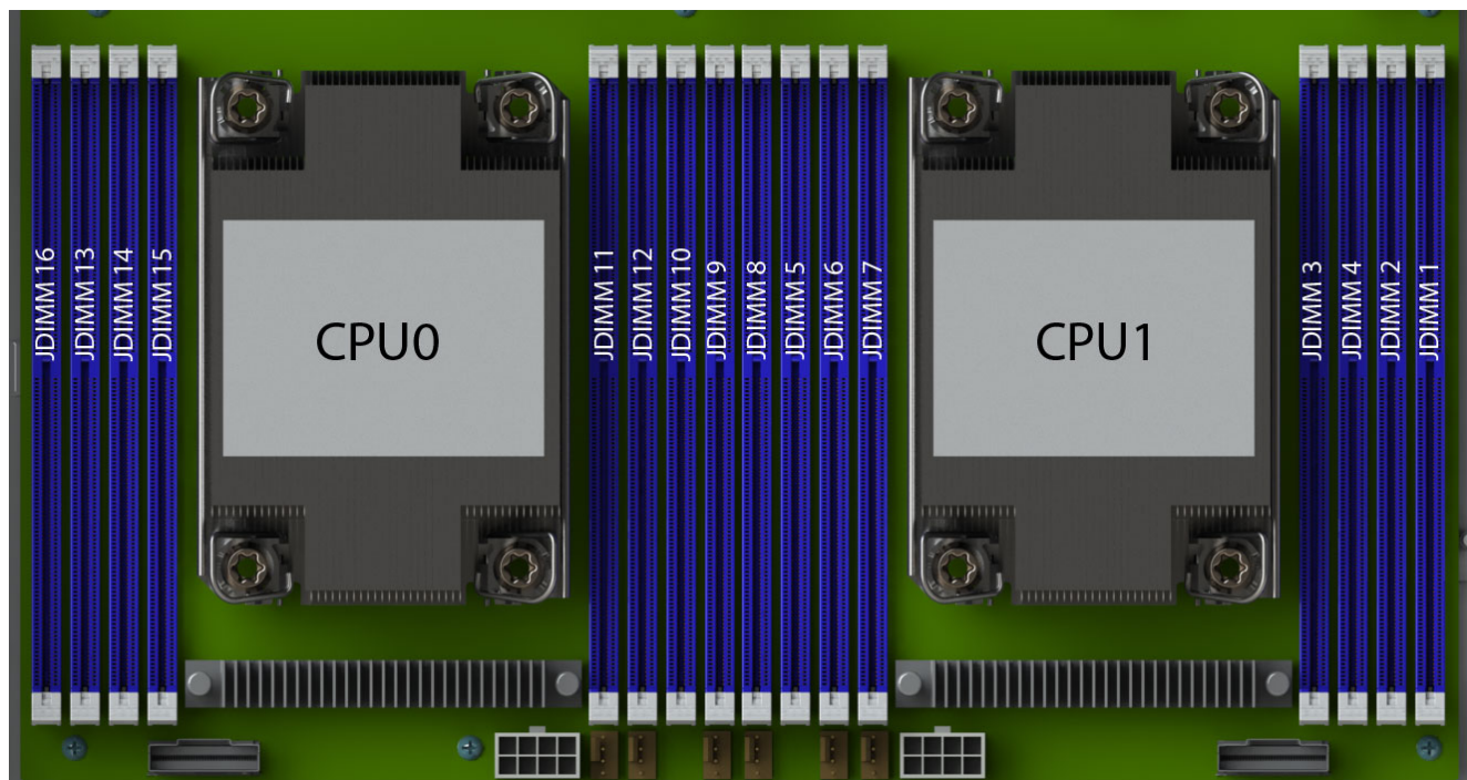
Рис. 32. Расположение разъемов
