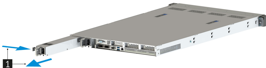
Рис. 67. Извлечение блока питания сервера
