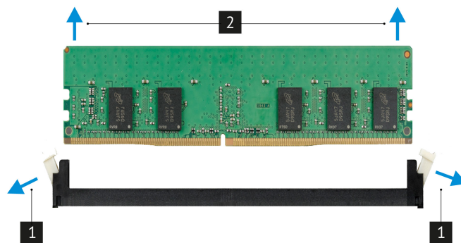
Рис. 33. Извлечение модуля ОЗУ.
