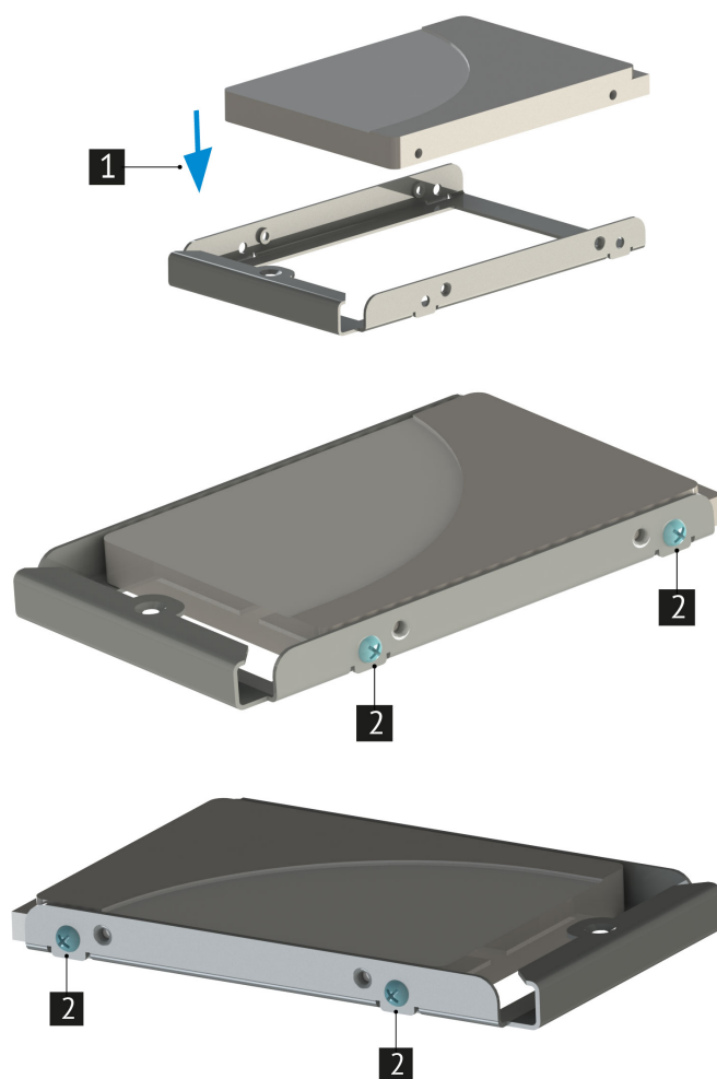
Рис. 49. Установка SSD диска в кассету
