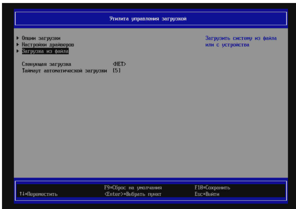
Рис. 78. Меню «Утилита управления загрузкой»
