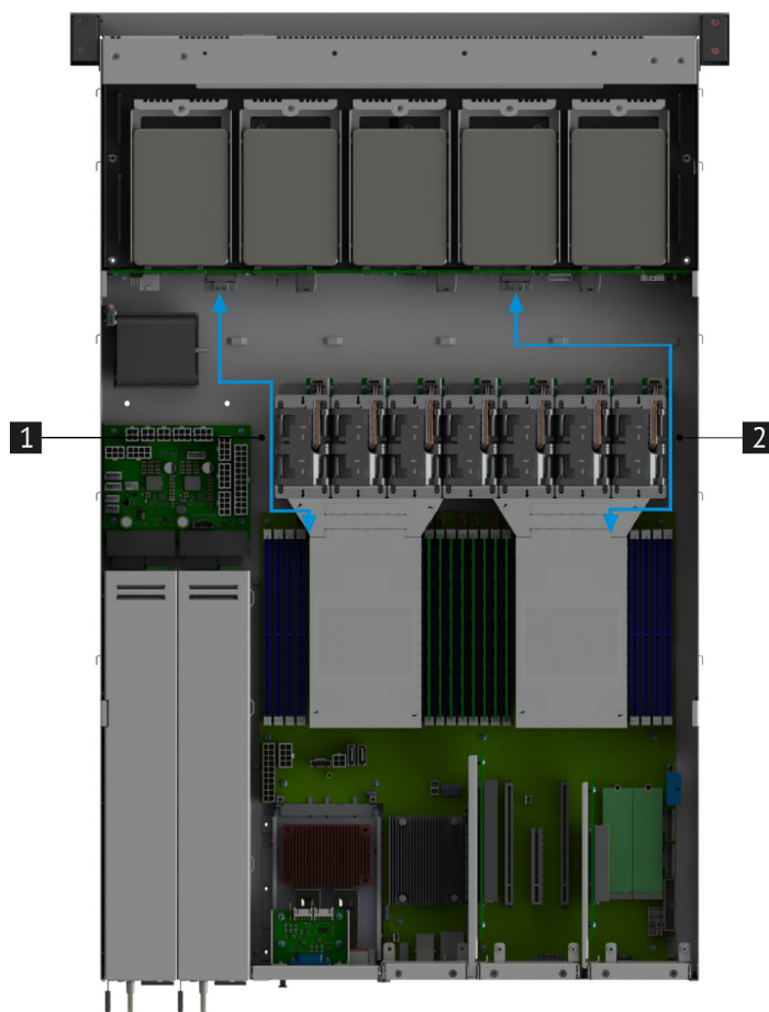
Рис. 45. Схема прокладки кабелей Oculink-SLIMline X8-X8
