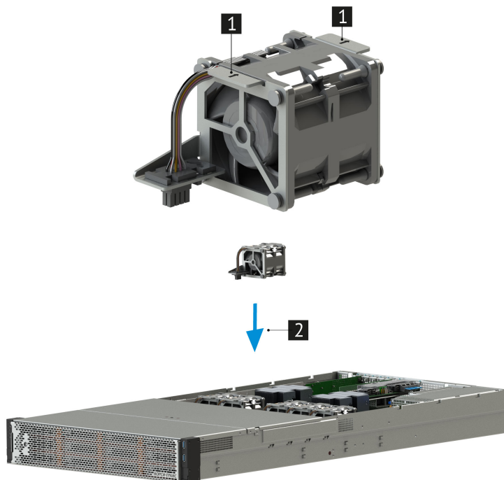
Рис. 43. Подключение вентилятора
