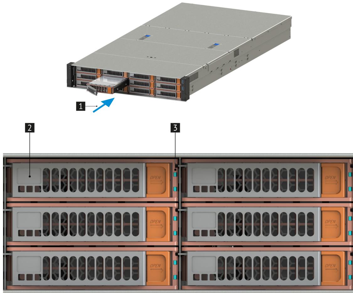
Рис. 55. Установка дисков
