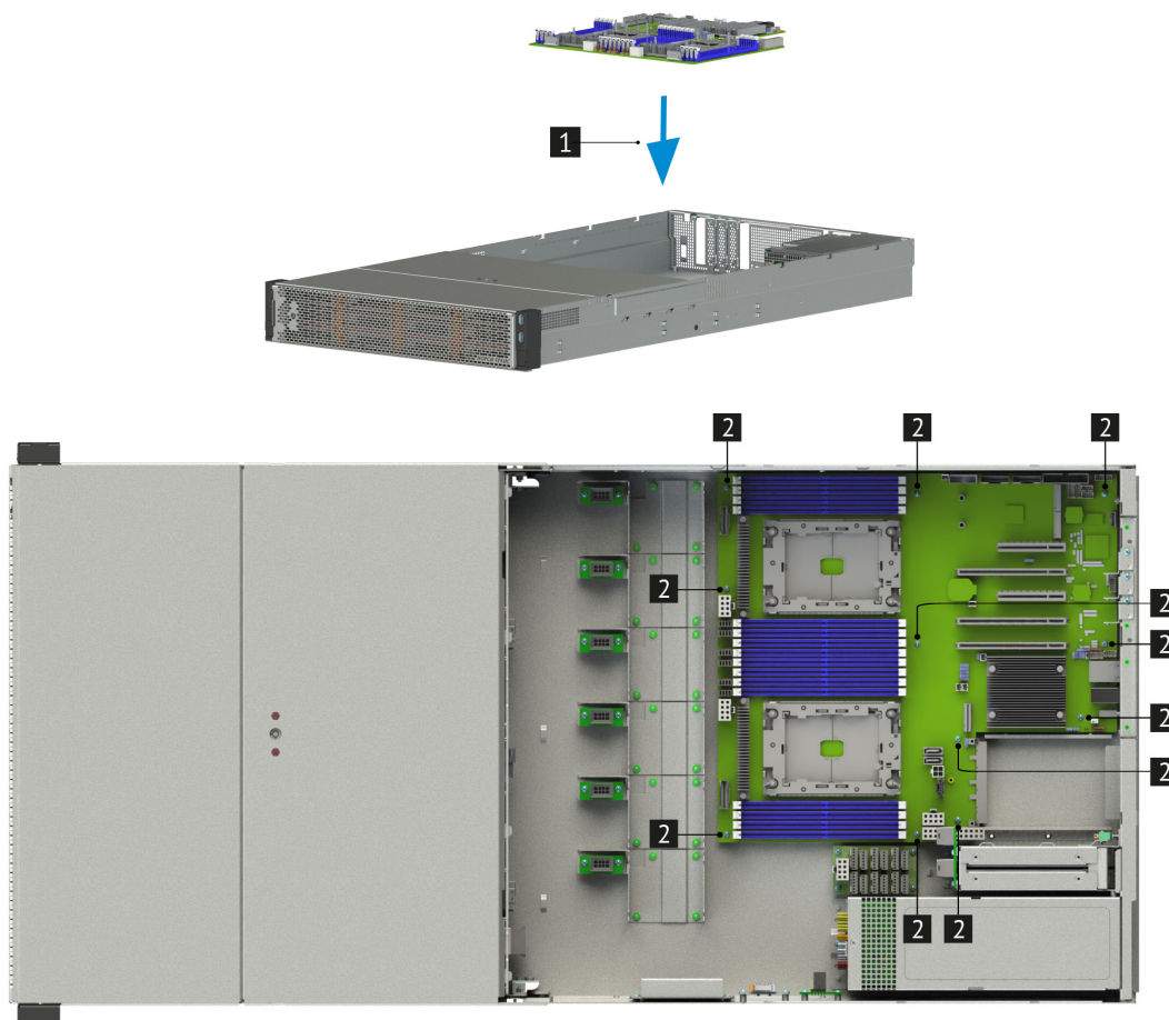
Рис. 53. Установка материнской платы в сервер
