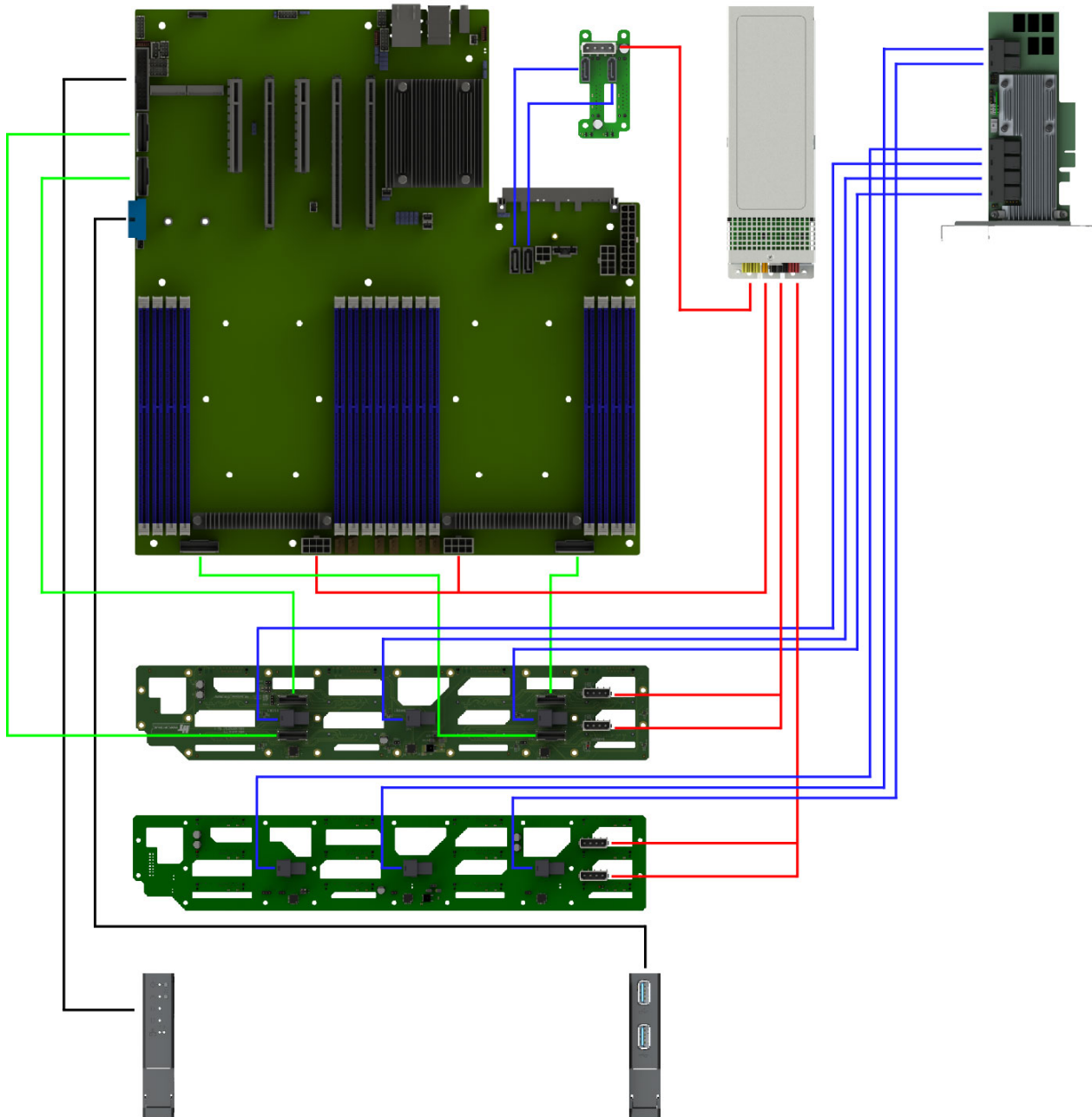
Рис. 41. Схема прокладки системных кабелей и кабелей Oculink-SLIMline X8-X8 с подключением PCIe RAID при использовании платы расширения 2SFF SATA (НИКА.469535.131)
