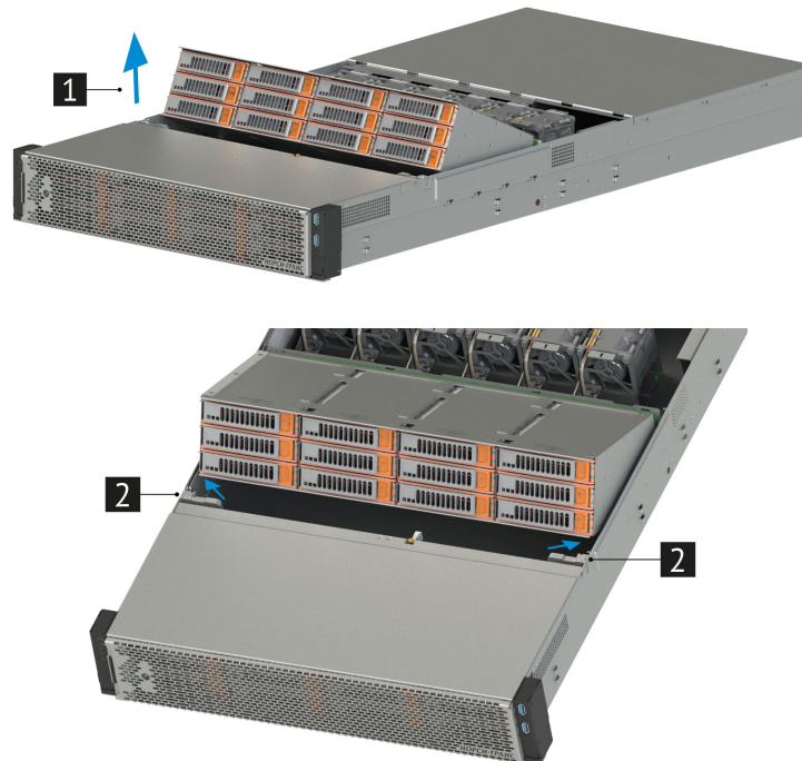
Рис. 29. Извлечение внутренней дисковой ленты/поворотной ленты
