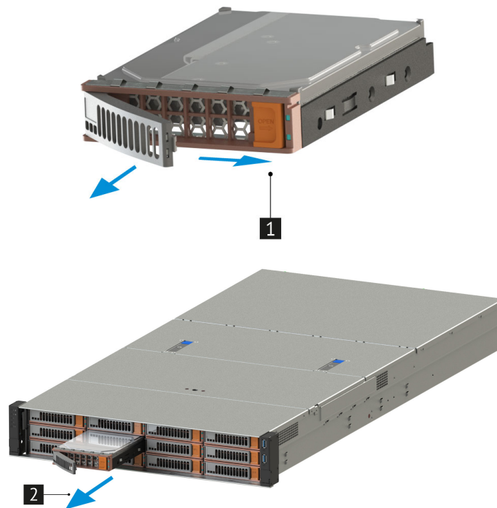
Рис. 54. Извлечение дисков
