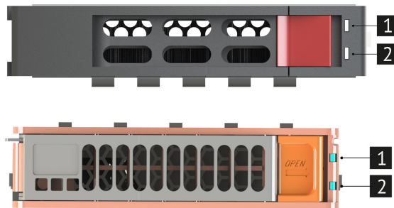
Рис. 8. Индикация дисков
