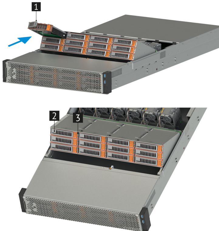
Рис. 57. Извлечение дисков
