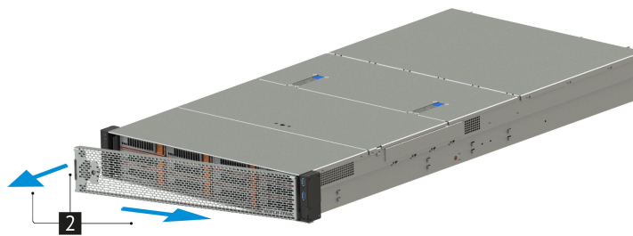
Рис. 20. Снятие передней панели
