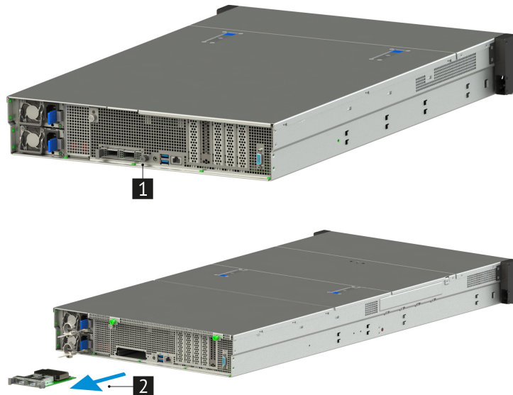
Рис. 69. Извлечение карты OCP 3.0 PCIe x16
