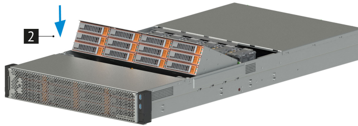
Рис. 30. Установка внутренней дисковой кассеты/поворотной кассеты
