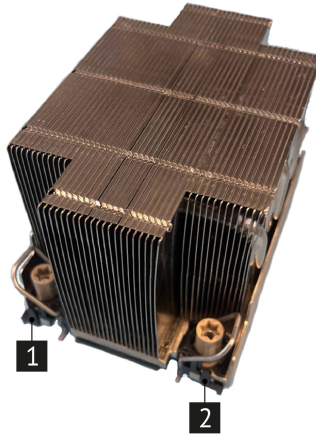
Рис. 49. Снятие процессора с радиатора
