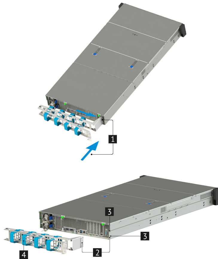
Рис. 18. Установка дополнительного кабельного органайзера.
