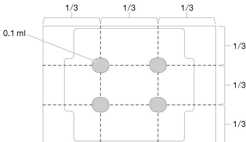
Рис. 51. Нанесение термопасты
