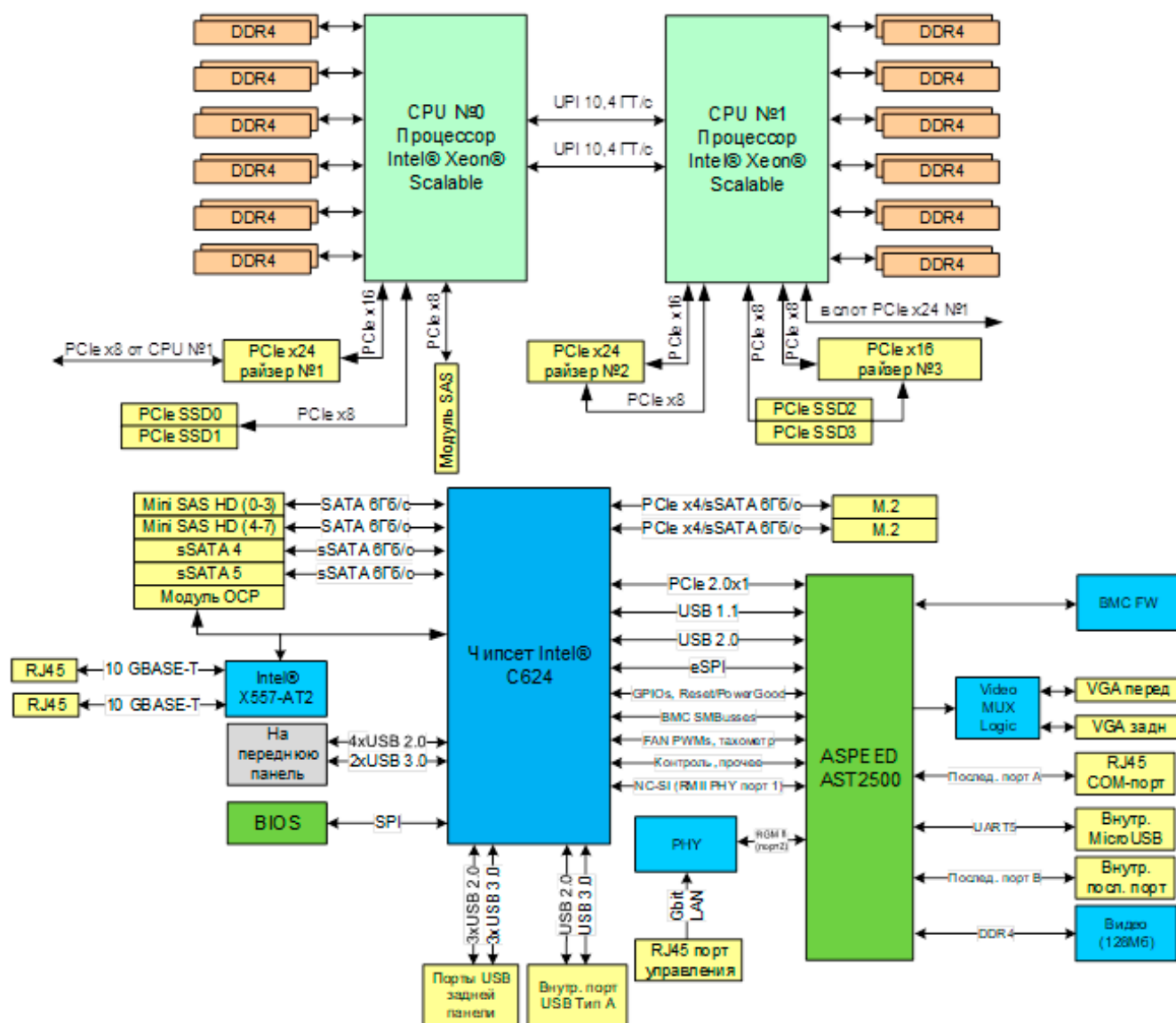
Рис. 1. Структурная схема материнской платы «НТ» НИКА.469555.001
