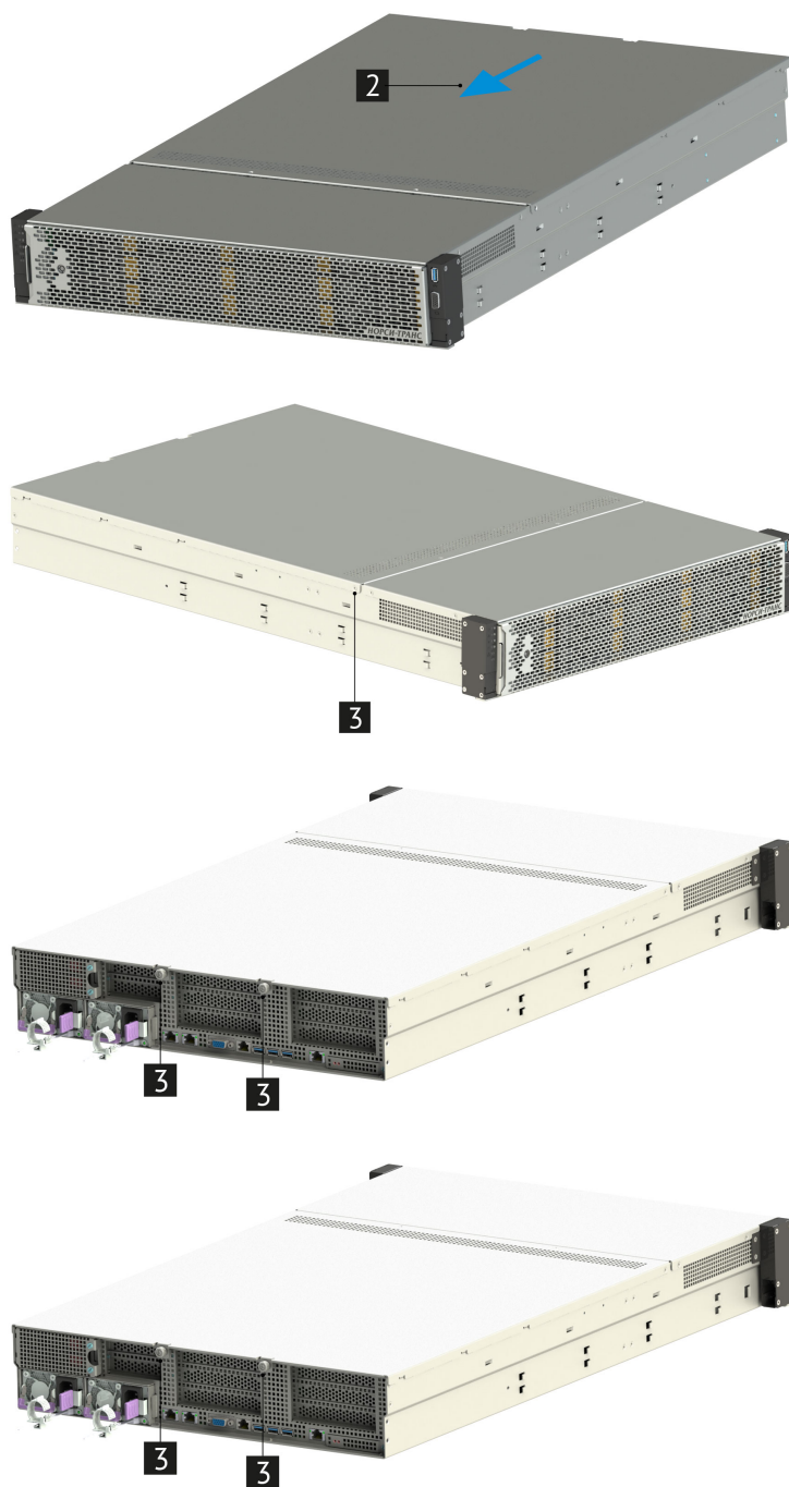
Рис. 25. Установка верхней крышки сервера
