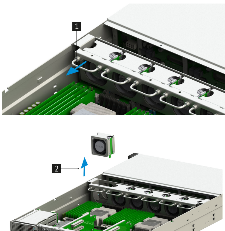
Рис. 31. Извлечение вентилятора из сервера
