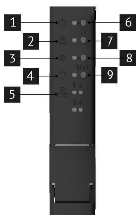
Рис. 3. Левая панель управления
