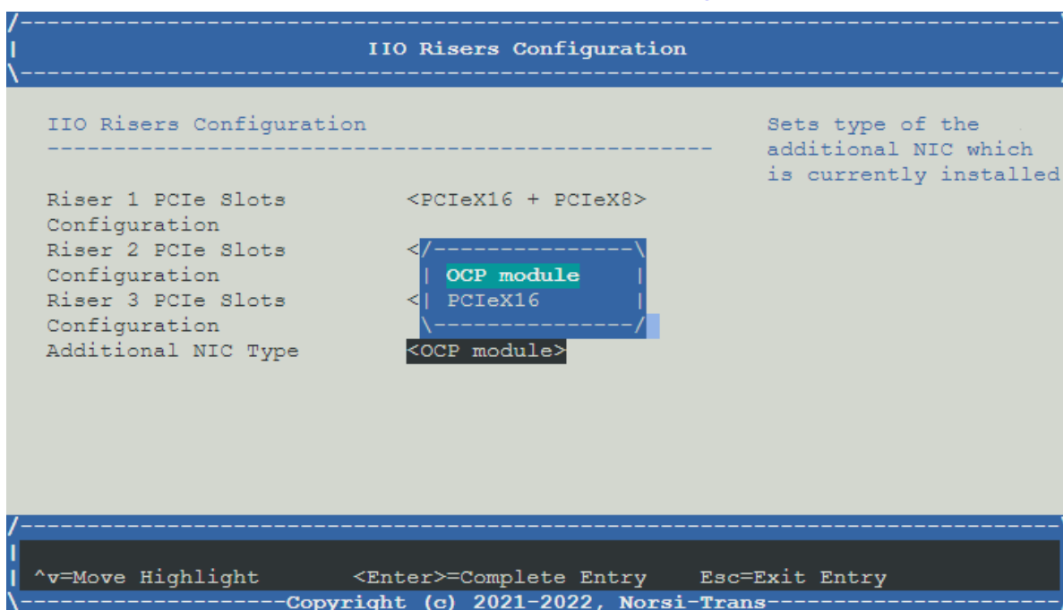
Рис. 85. Меню I/O Risers Configuration
