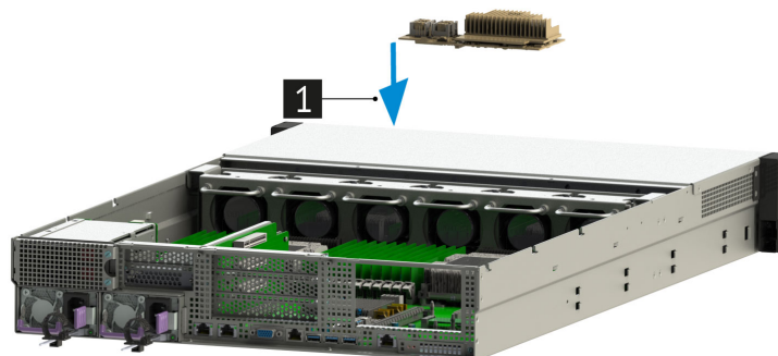
Рис. 56. Установка наплатного RAID-контроллера
