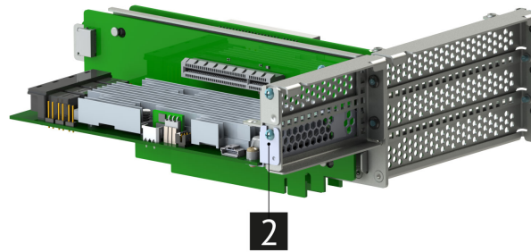
Рис. 54. Установка контроллера дискового MegaRAID 9361-16i
