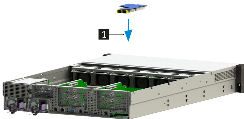
Рис. 58. Установка карты OCP 2.0
