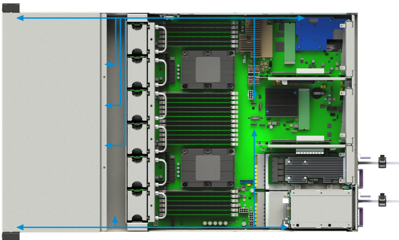
Рис. 26. Схема прокладки кабелей в сервере
