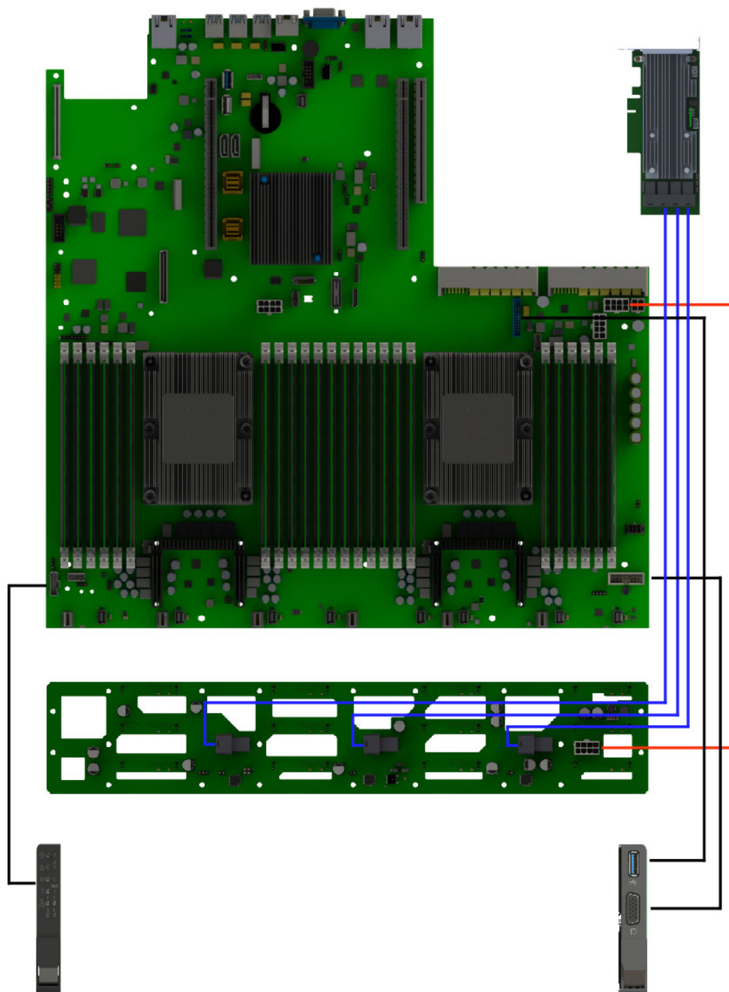
Рис. 29. Схема прокладки системных кабелей с подключением PCIe RAID
