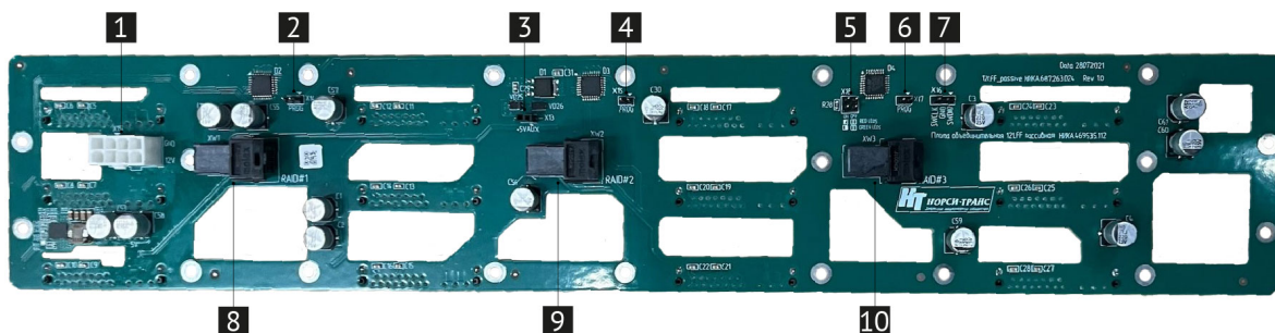
Рис. 11. Плата расширения 12LFF пассивная (НИКА.469535.112)
