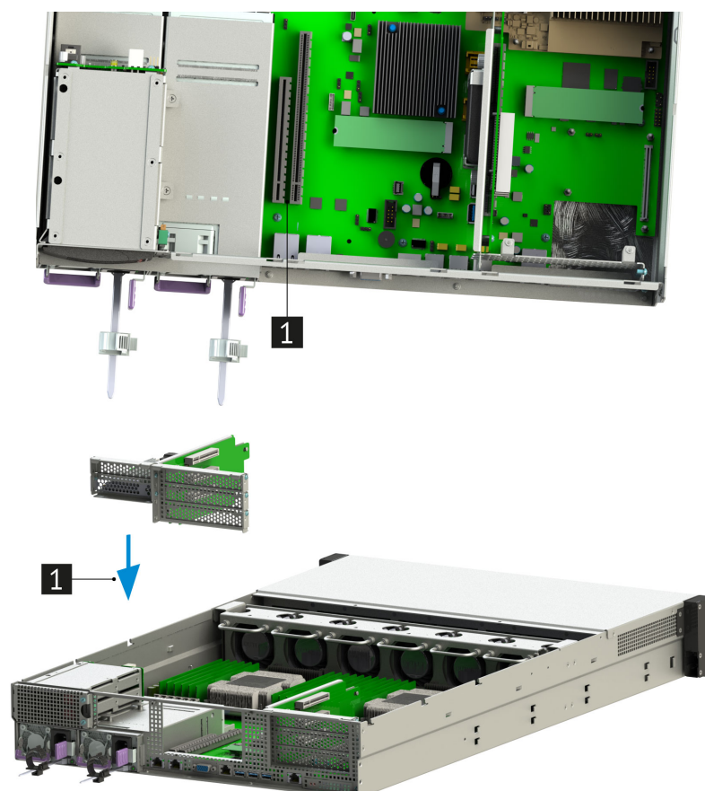
Рис. 52. Установка райзеров PCIe 1x24-8-8-8, PCIe 3x16-8-8
