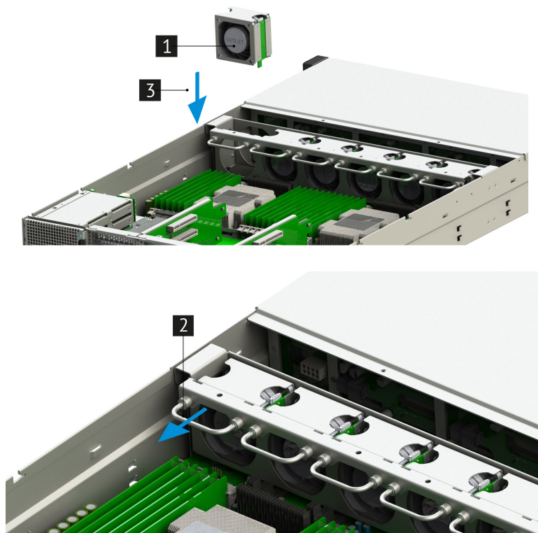
Рис. 32. Подключение вентилятора
