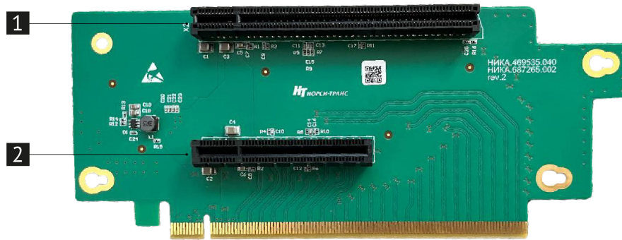
Рис. 13. Райзер 1x24-16-8 (НИКА.469535.040)
