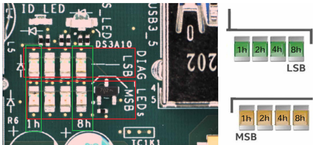
Рис. 6. Расположение и определение POST CODE LED
