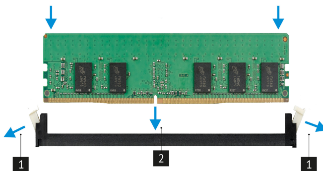
Рис. 37. Установка модуля ОЗУ.
