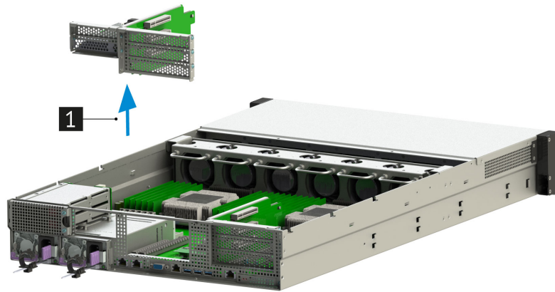
Рис. 51. Извлечение райзеров PCIe 1x24-8-8-8, PCIe 3x16-8-8
