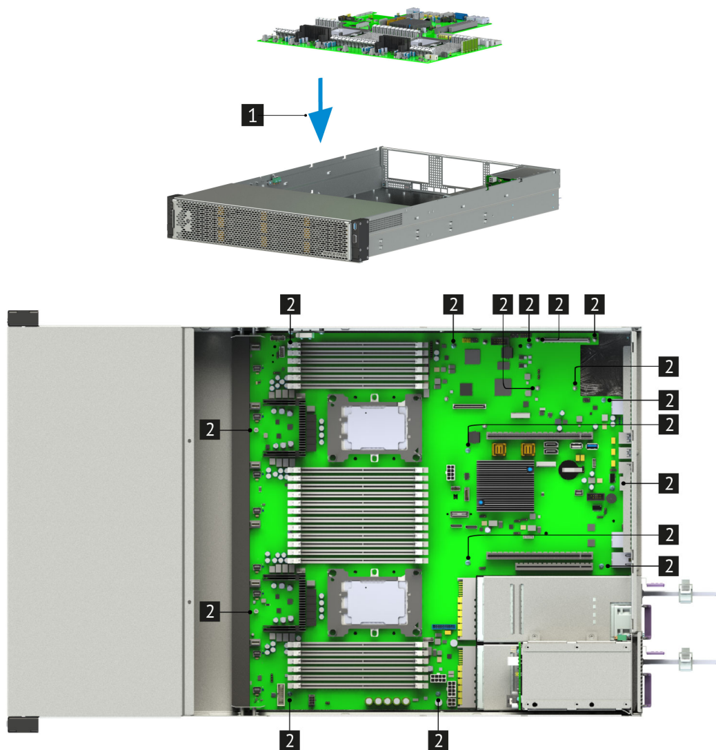
Рис. 44. Установка материнской платы в сервер
