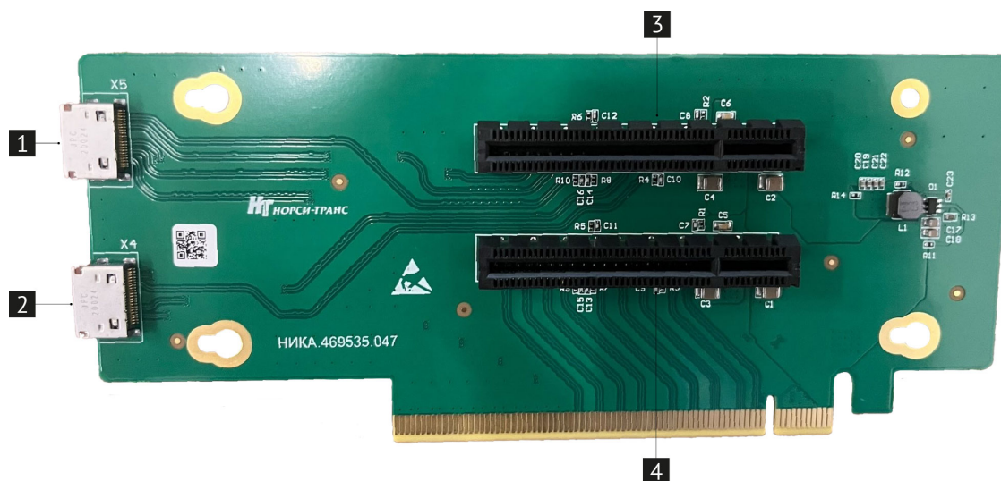
Рис. 17. Райзер 3x16-8-8 (НИКА.469535.047)
