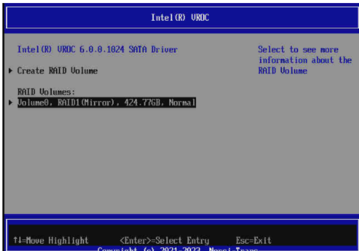
Рис. 76. Меню Intel (R) VROC с готовым массивом
