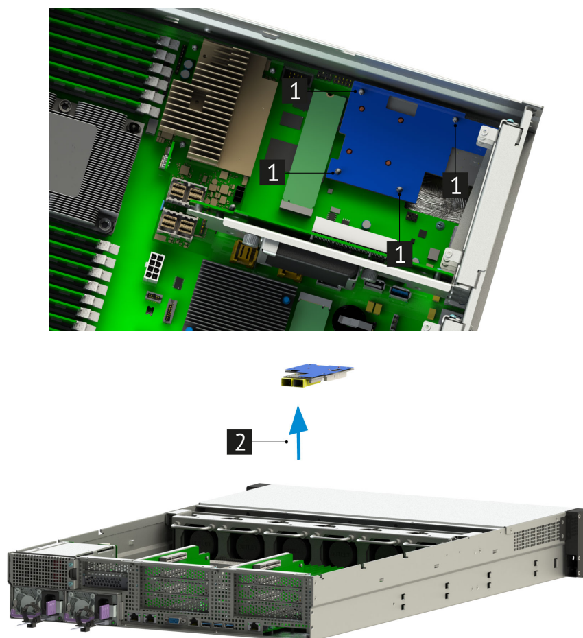
Рис. 57. Извлечение карты ОСР 2.0
