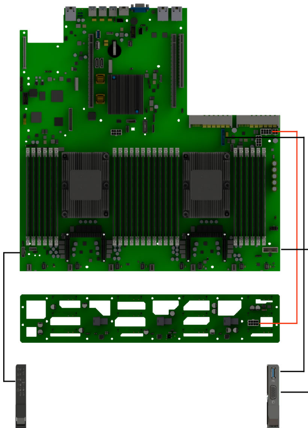
Рис. 27. Схема прокладки системных кабелей и кабелей питания
