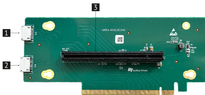
Рис. 16. Райзер 3x16-16 (НИКА.469535.046)
