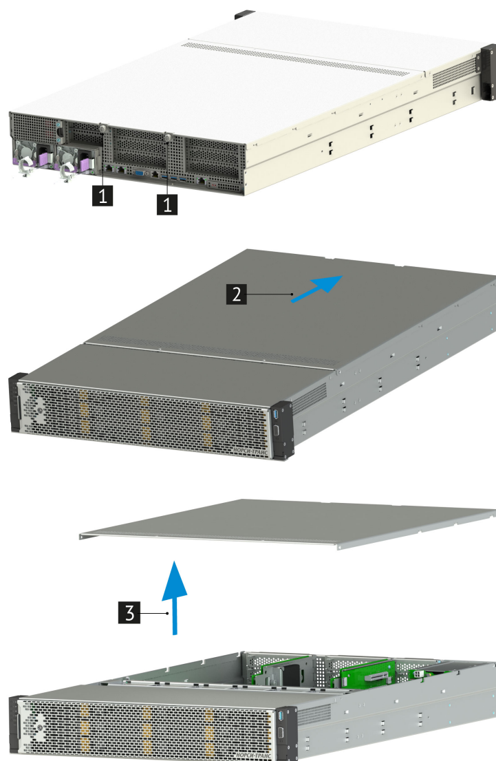
Рис. 24. Снятие верхней крышки сервера
