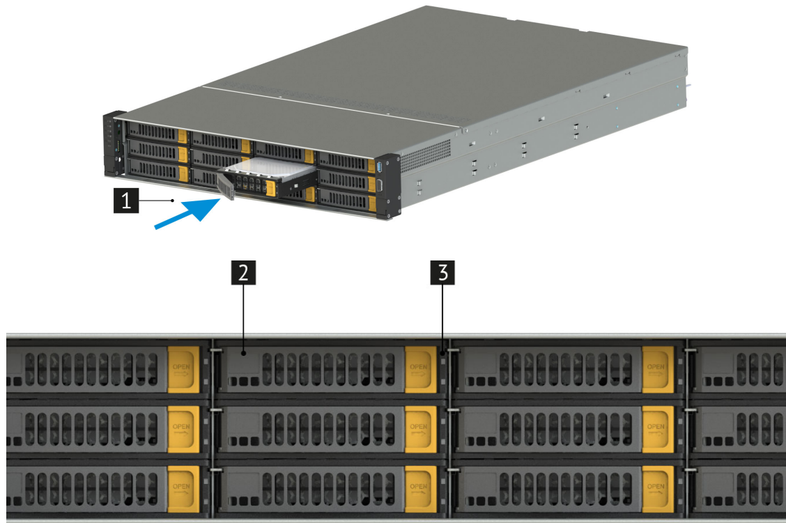
Рис. 46. Установка дисков
