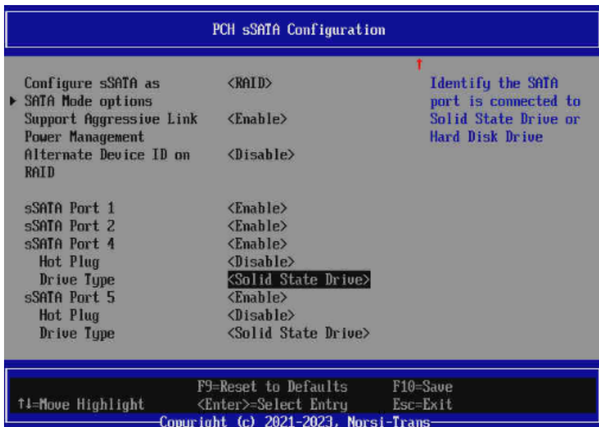
Рис. 79. Меню PCH SATA Configuration
