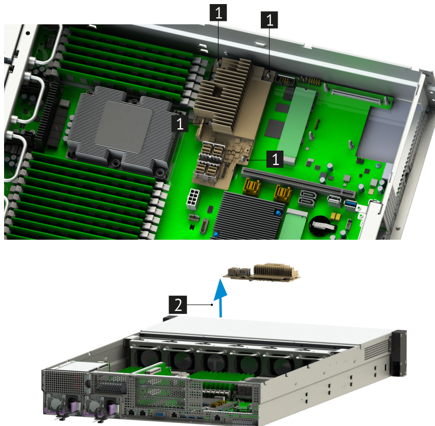
Рис. 55. Извлечение наплатного RAID-контроллера
