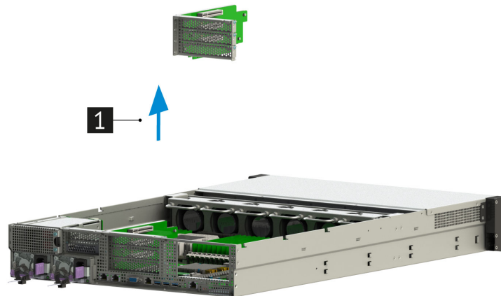
Рис. 49. Извлечение райзера PCIe 1x24-8-8-8
