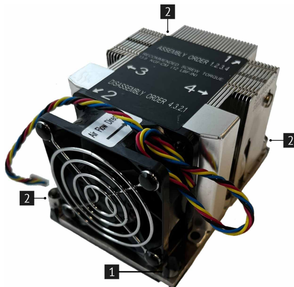
Рис. 40. Снятие процессора с радиатора
