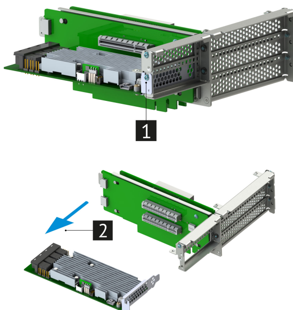
Рис. 53. Извлечение контроллера дискового MegaRAID 9361-16i
