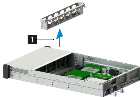
Рис. 33. Извлечение каркаса блока вентиляторов из сервера
