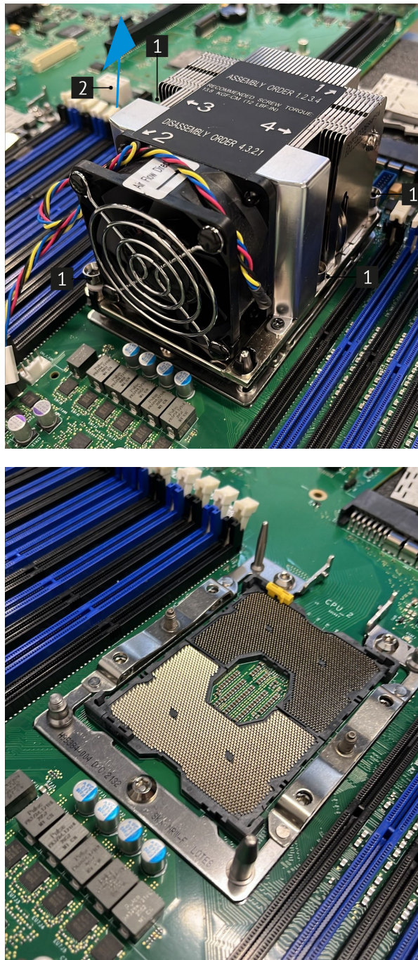
Рис. 39. Снятие модуля процессора с радиатором
