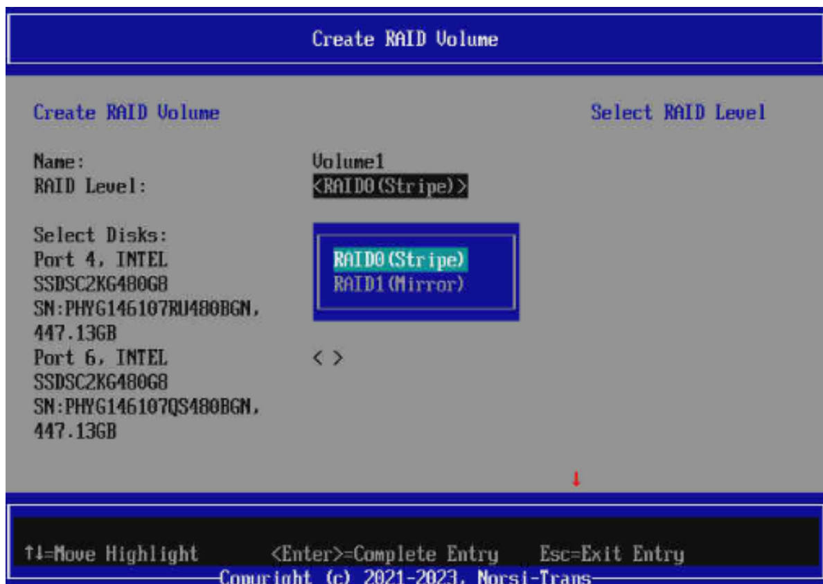
Рис. 74. Меню Intel (R) VROC
