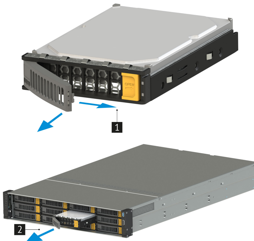
Рис. 45. Извлечение дисков
