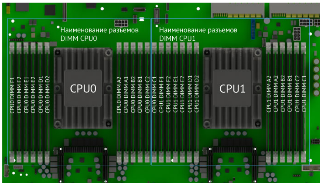
Рис. 35. Расположение разъемов
