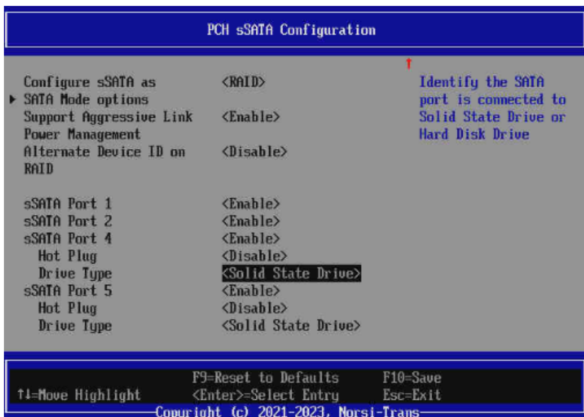
Рис. 78. Меню PCH SATA Configuration
