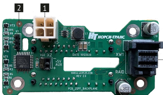
Рис. 12. Плата расширения 2SFF (НИКА.469535.038)
