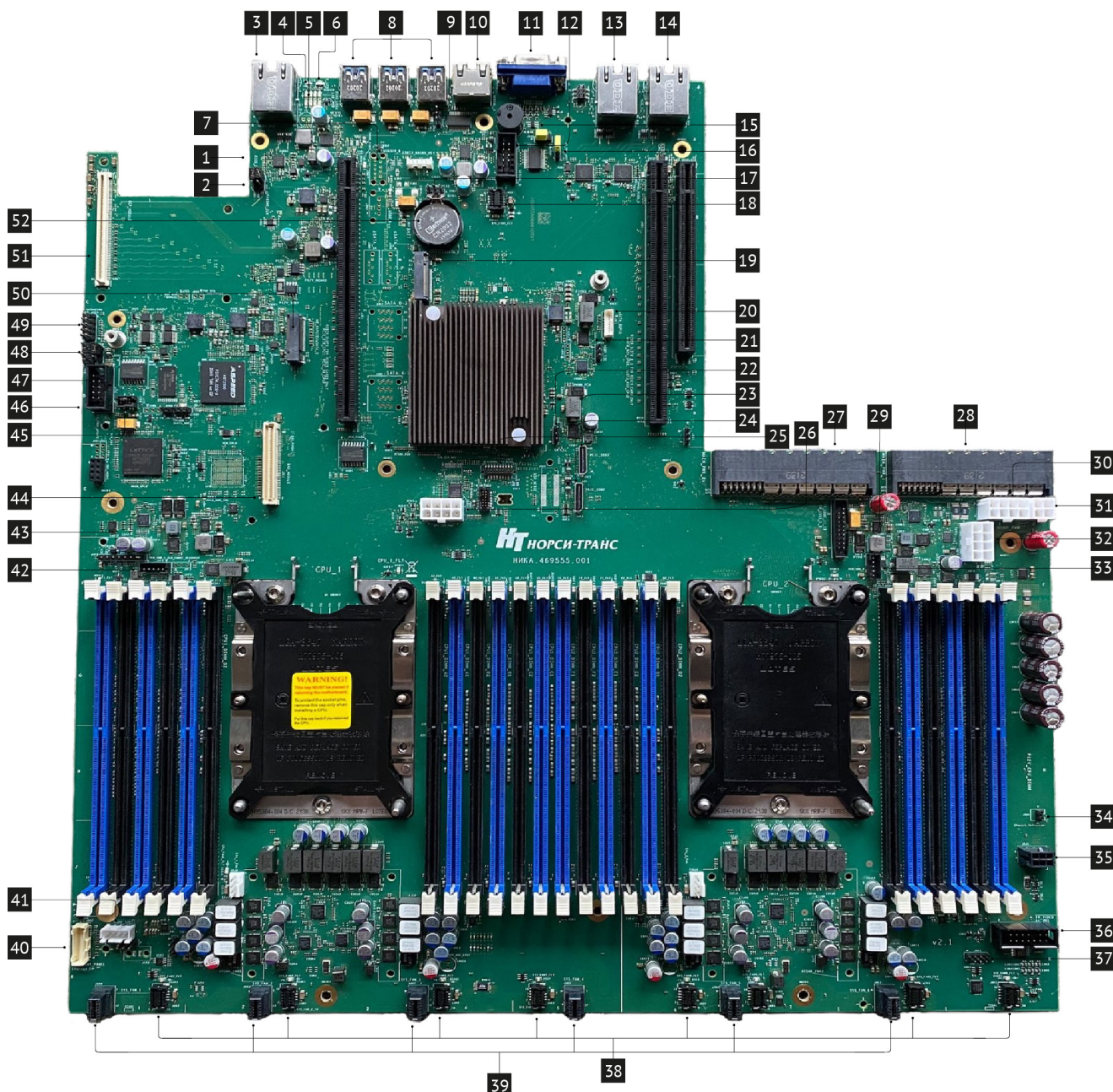
Рис. 10. Соединители и переключатели материнской платы
