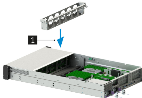
Рис. 34. Установка каркаса блока вентиляторов в сервер
