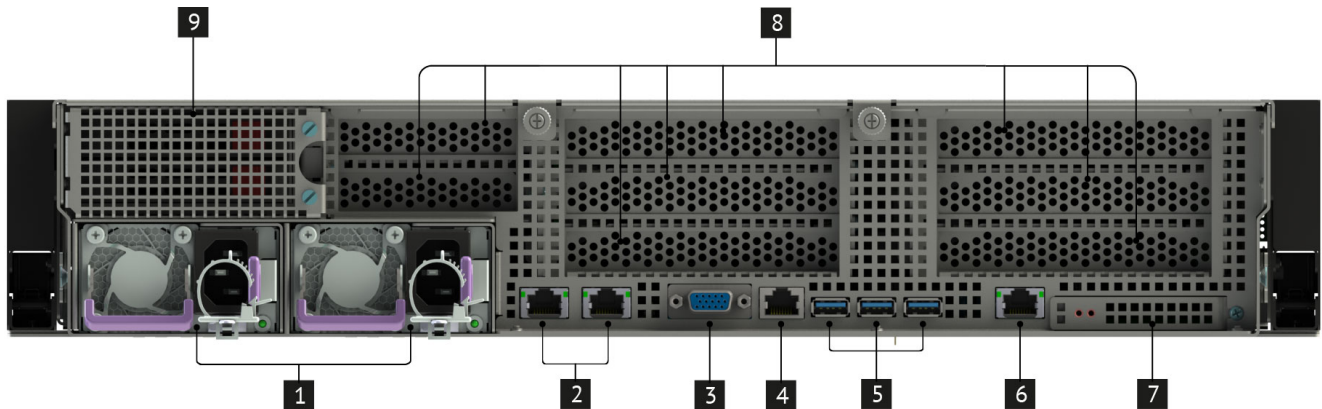
Рис. 5. Вид сервера сзади
