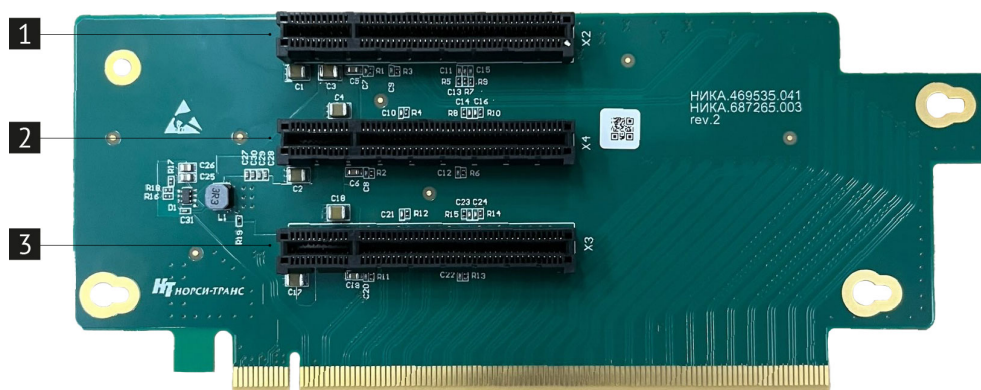
Рис. 14. Райзер 1x24-8-8-8 (НИКА.469535.041)
