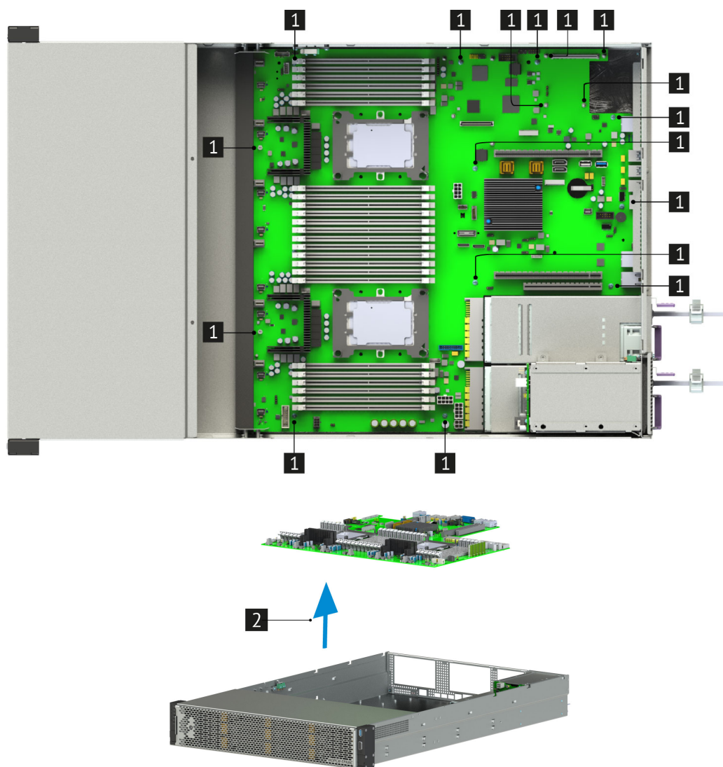
Рис. 43. Извлечение материнской платы из сервера
