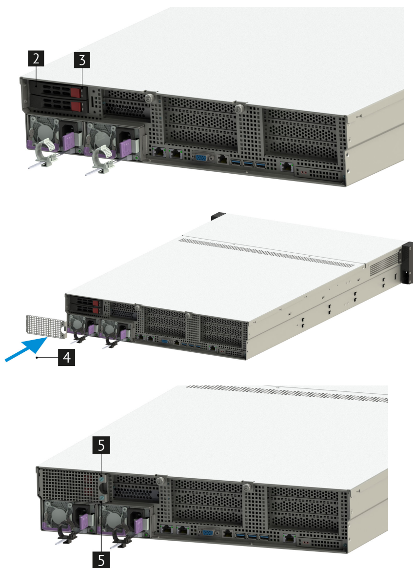
Рис. 48. Установка тыльных дисков
