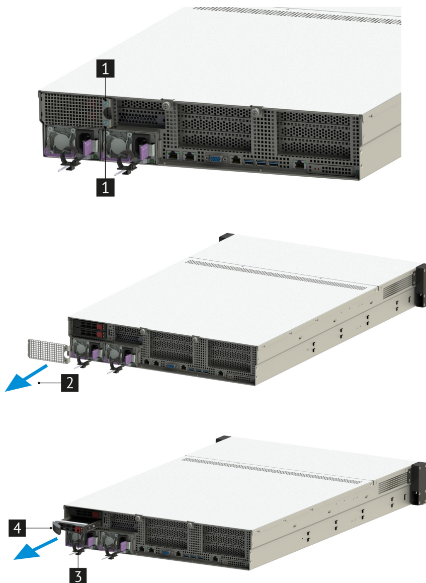
Рис. 47. Извлечение тыльных дисков
