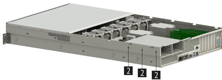
Рис. 25. Установка кожуха БП
