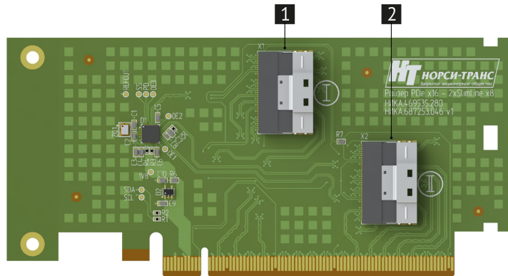
Рис. 13. Райзер PCIe x16-2xSlimLine x8 (НИКА.469535.280)
