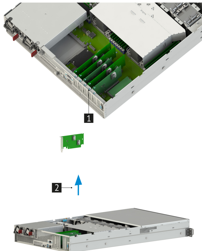
Рис. 50. Извлечение райзера PCIe x16-2xSlimLine x8
