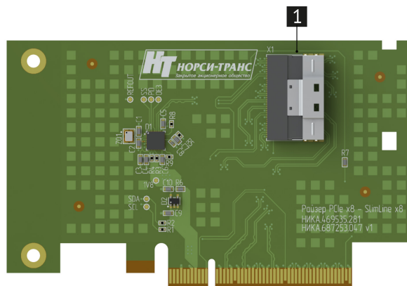
Рис. 14. Райзер PCIe x8-SlimLine x8 (НИКА.469535.281)
