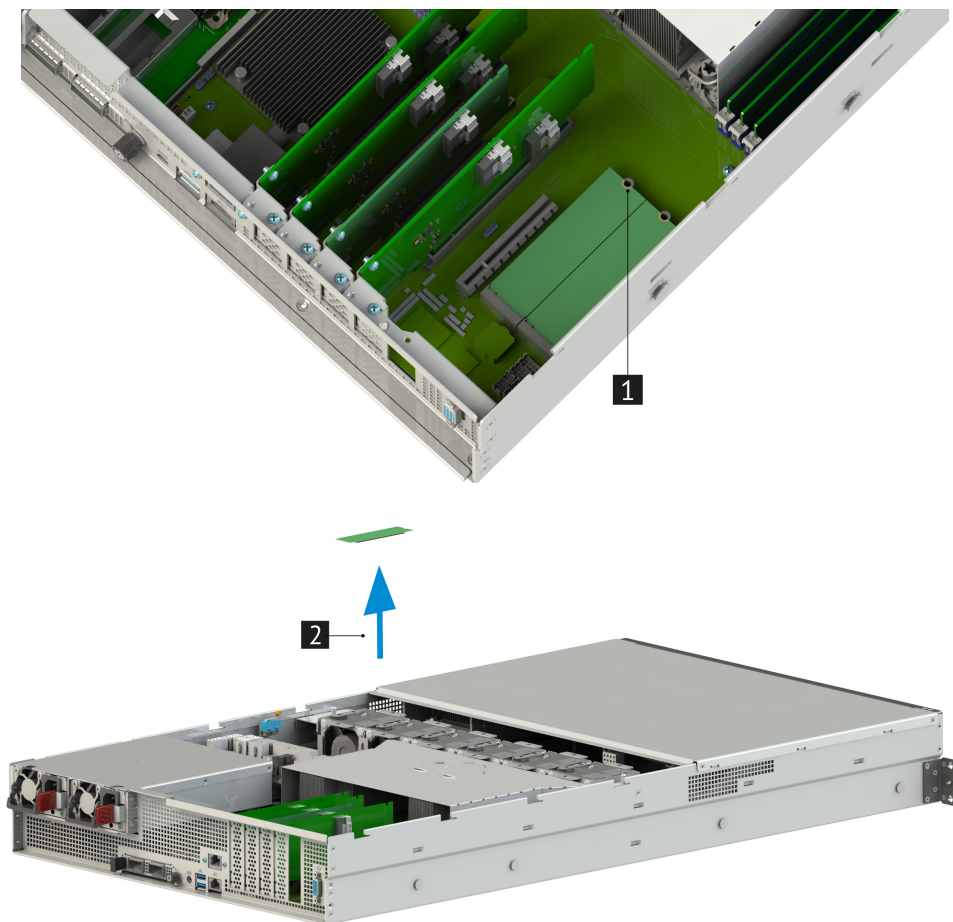
Рис. 43. Извлечение M.2 диска
