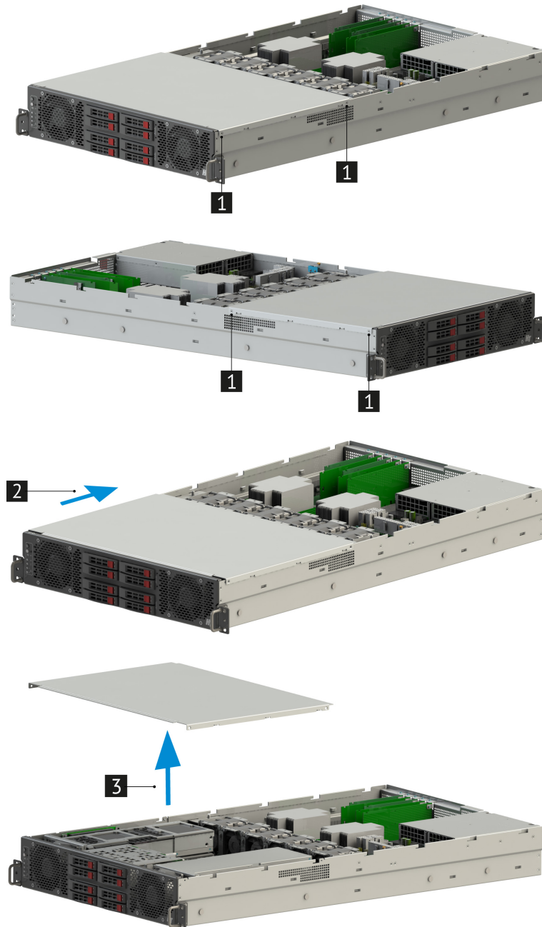
Рис. 20. Снятие передней крышки платформы
