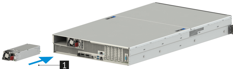
Рис. 62. Установка блока питания в сервер
