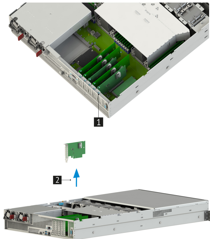
Рис. 52. Извлечение райзера PCIe x8-SlimLine x8
