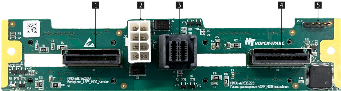
Рис. 11. Плата расширения 4SFF MCIО пассивная (НИКА.469535.228)
