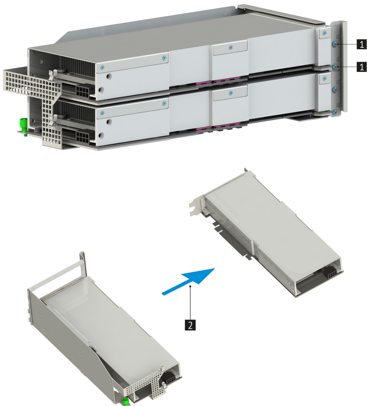
Рис. 58. Извлечение карты GPU из кассеты
