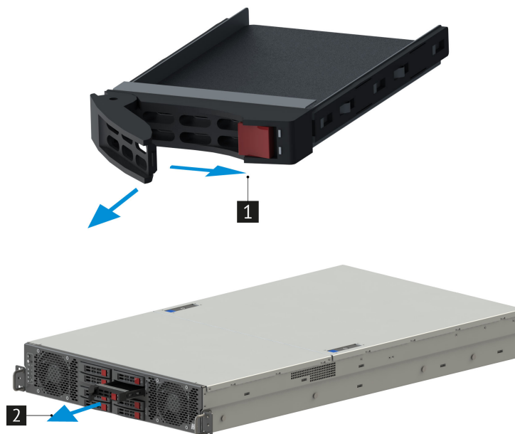
Рис. 47. Извлечение дисков
