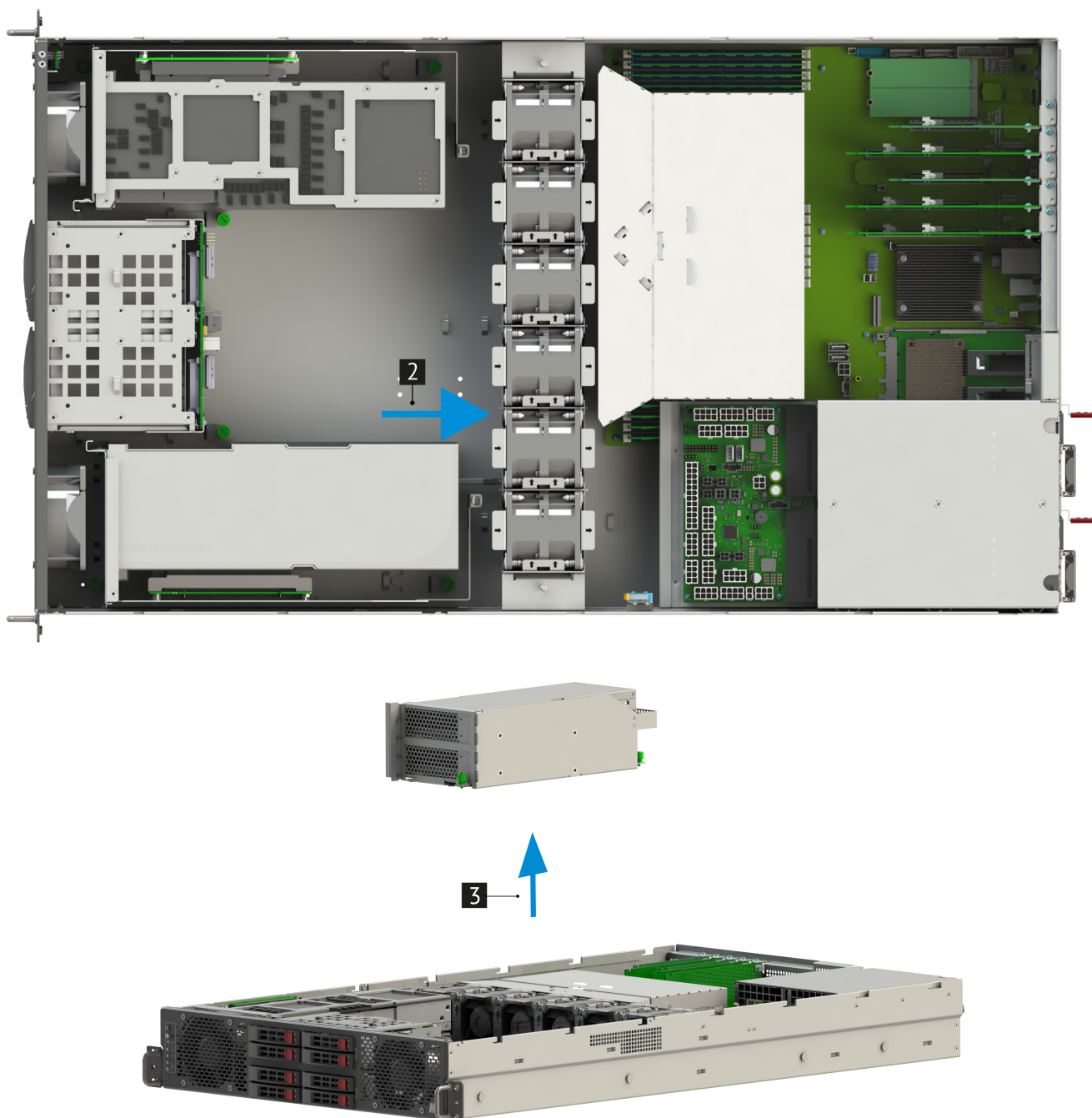
Рис. 56. Извлечение карт GPU
