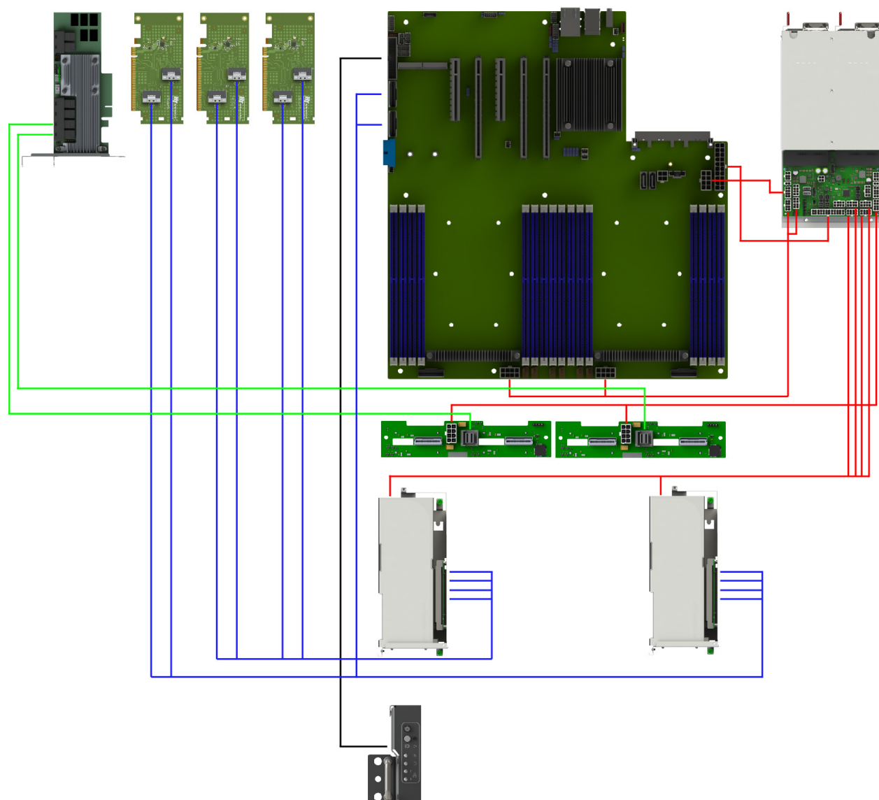
Рис. 32. Схема прокладки системных кабелей, кабелей питания, кабелей для подключения дисков SAS/SATA с подключением PCIe RAID
