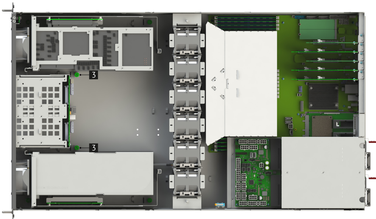
Рис. 27. Установка каркасов под диски SFF
