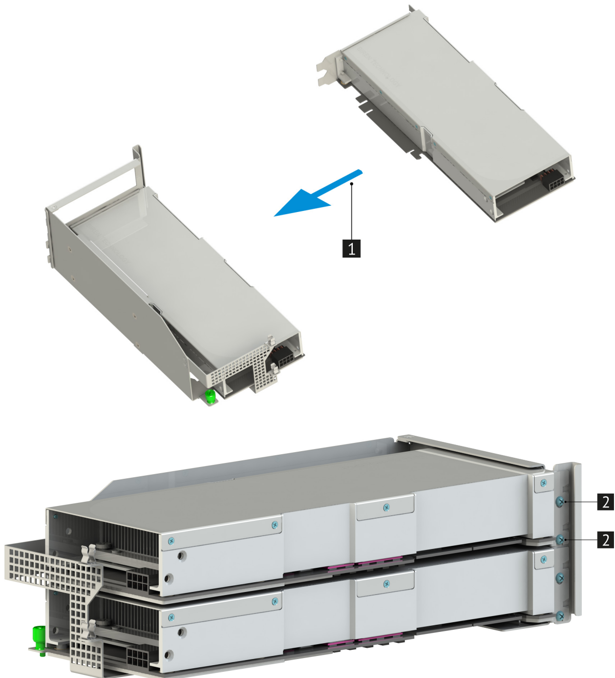
Рис. 59. Установка карты GPU в кассету
