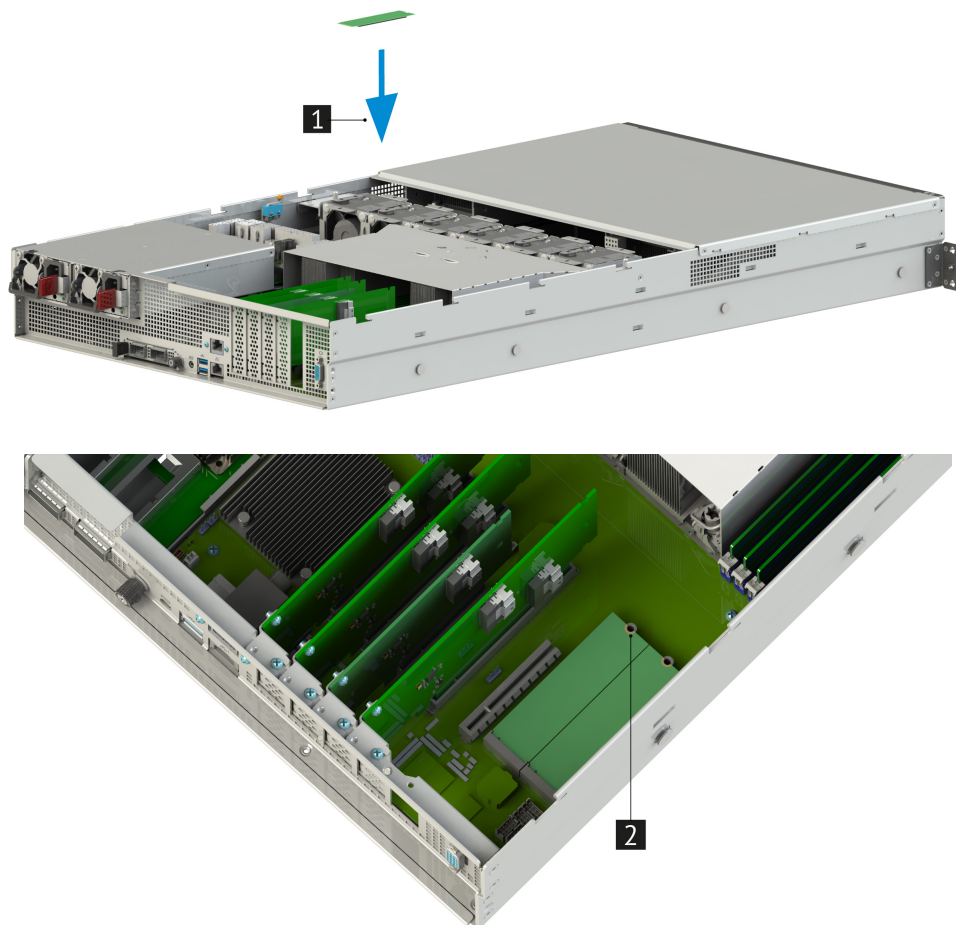
Рис. 44. Установка M.2 диска
