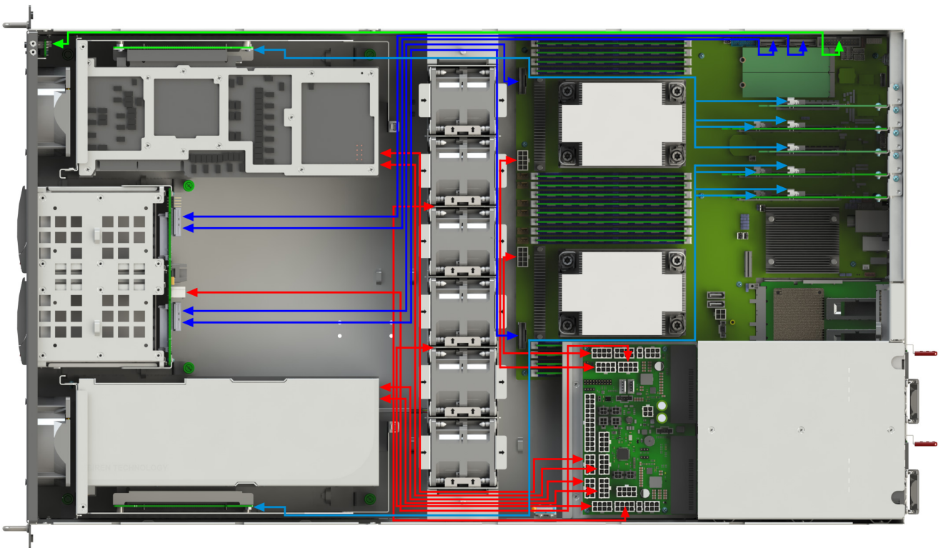
Рис. 28. Схема прокладки кабелей в сервере
