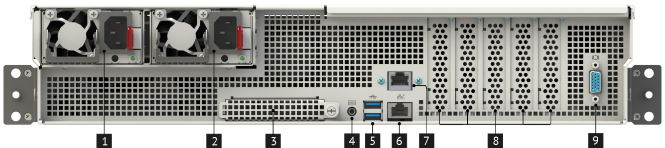
Рис. 6. Вид сервера сзади
