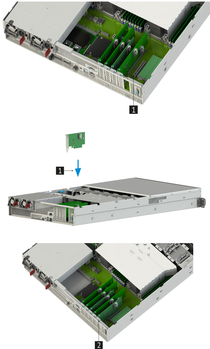
Рис. 53. Установка райзера PCIe x8-SlimLine x8
