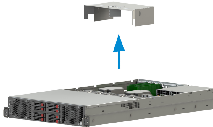
Рис. 22. Извлечение воздушного кожуха
