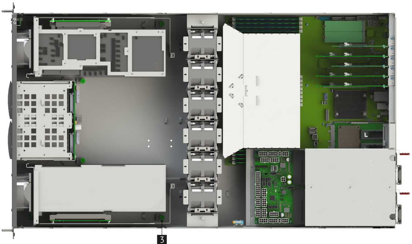
Рис. 57. Установка карт GPU
