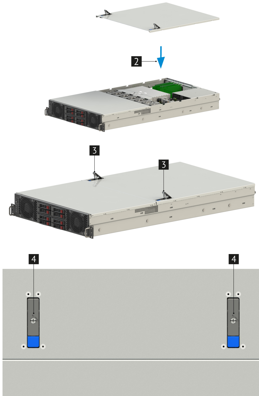
Рис. 19. Установка задней верхней крышки сервера
