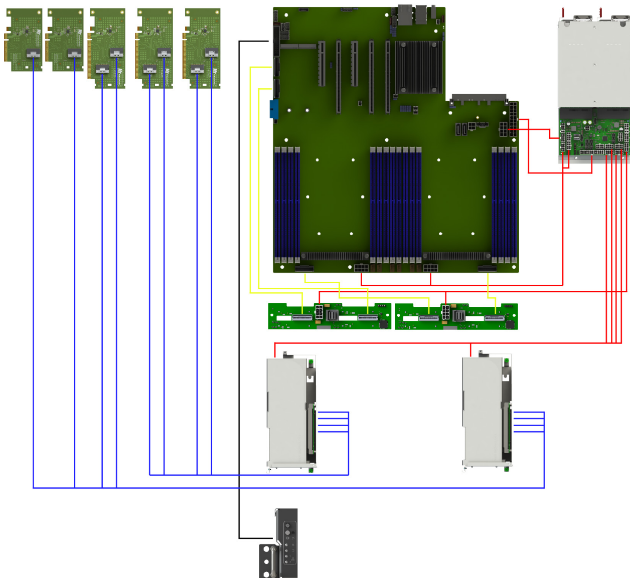
Рис. 30. Схема прокладки системных кабелей, кабелей для подключения дисков NVMe
