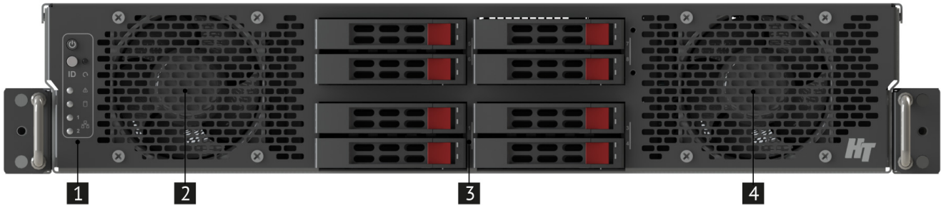
Рис. 3. Вид сервера спереди с 8-ю установленными жесткими дисками
