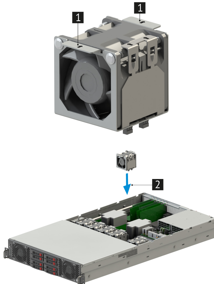
Рис. 34. Подключение вентилятора
