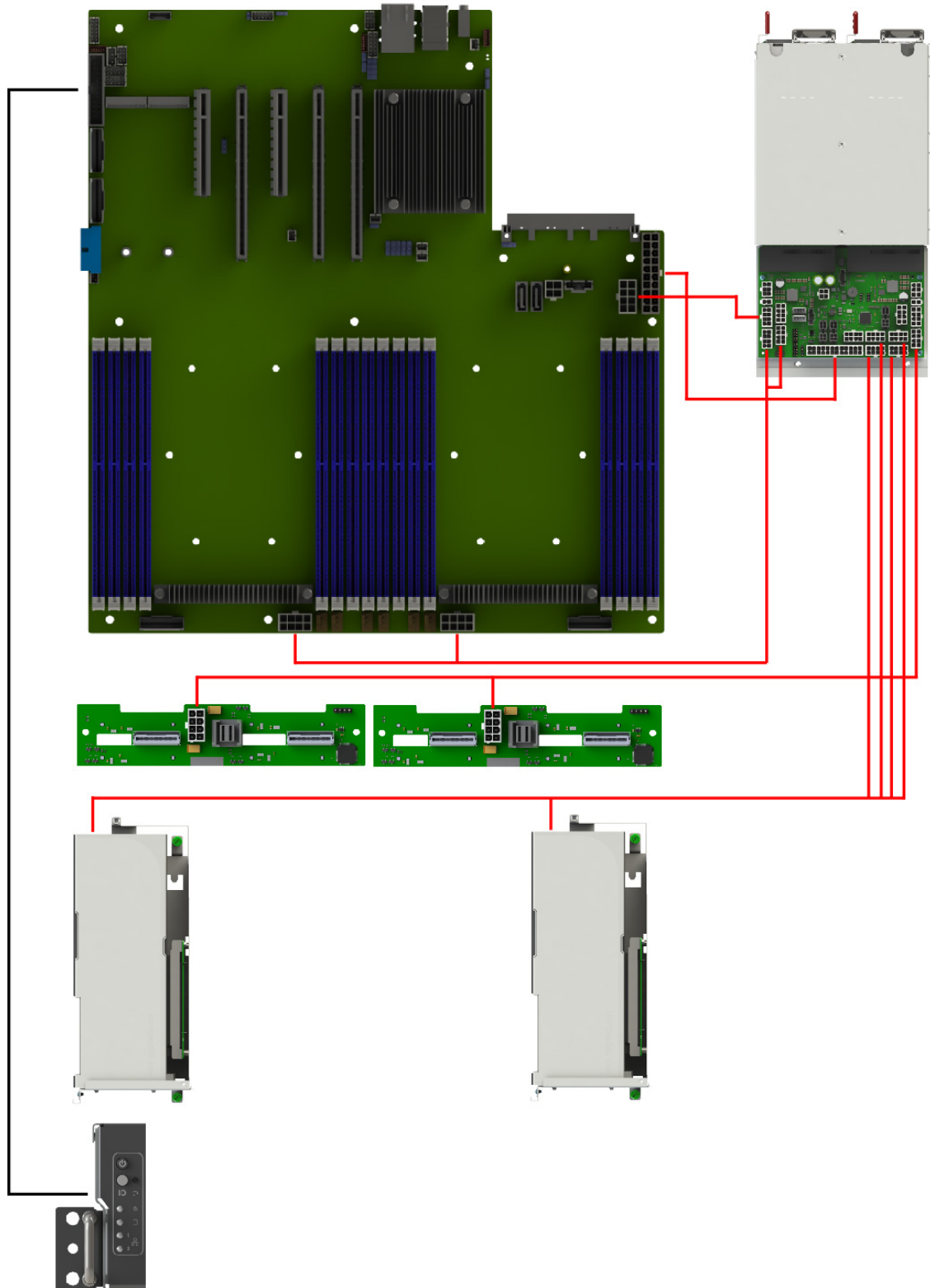
Рис. 29. Схема прокладки системных кабелей и кабелей питания
