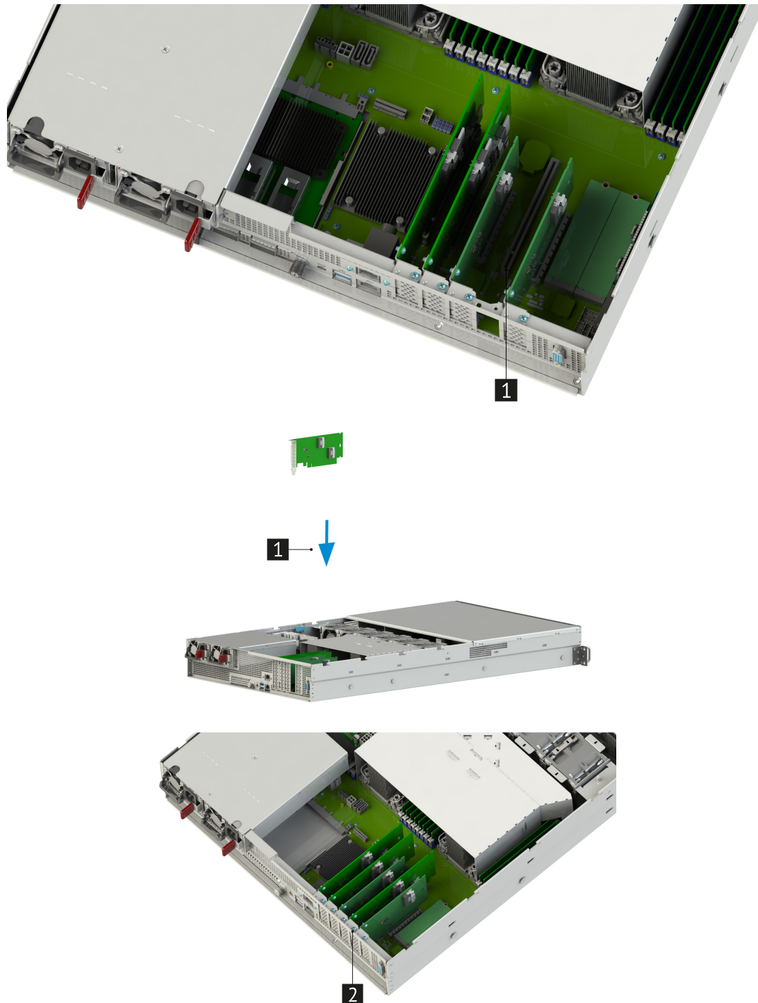
Рис. 51. Установка райзера PCIe x16-2xSlimLine x8
