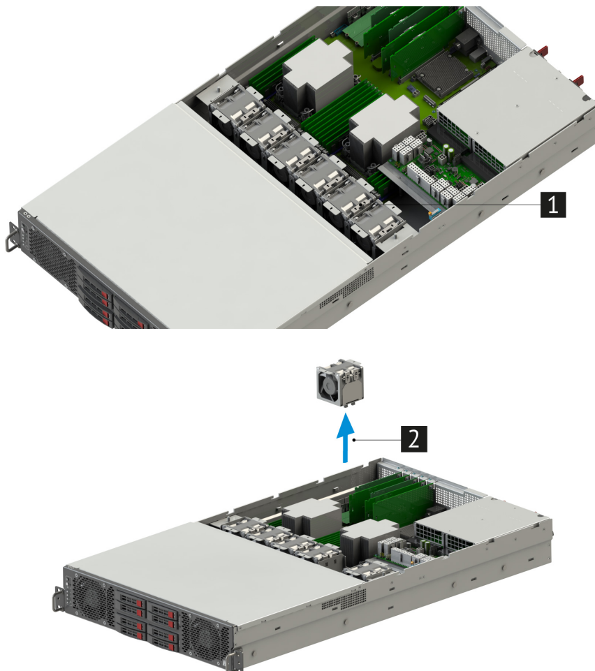
Рис. 33. Извлечение вентилятора из сервера
