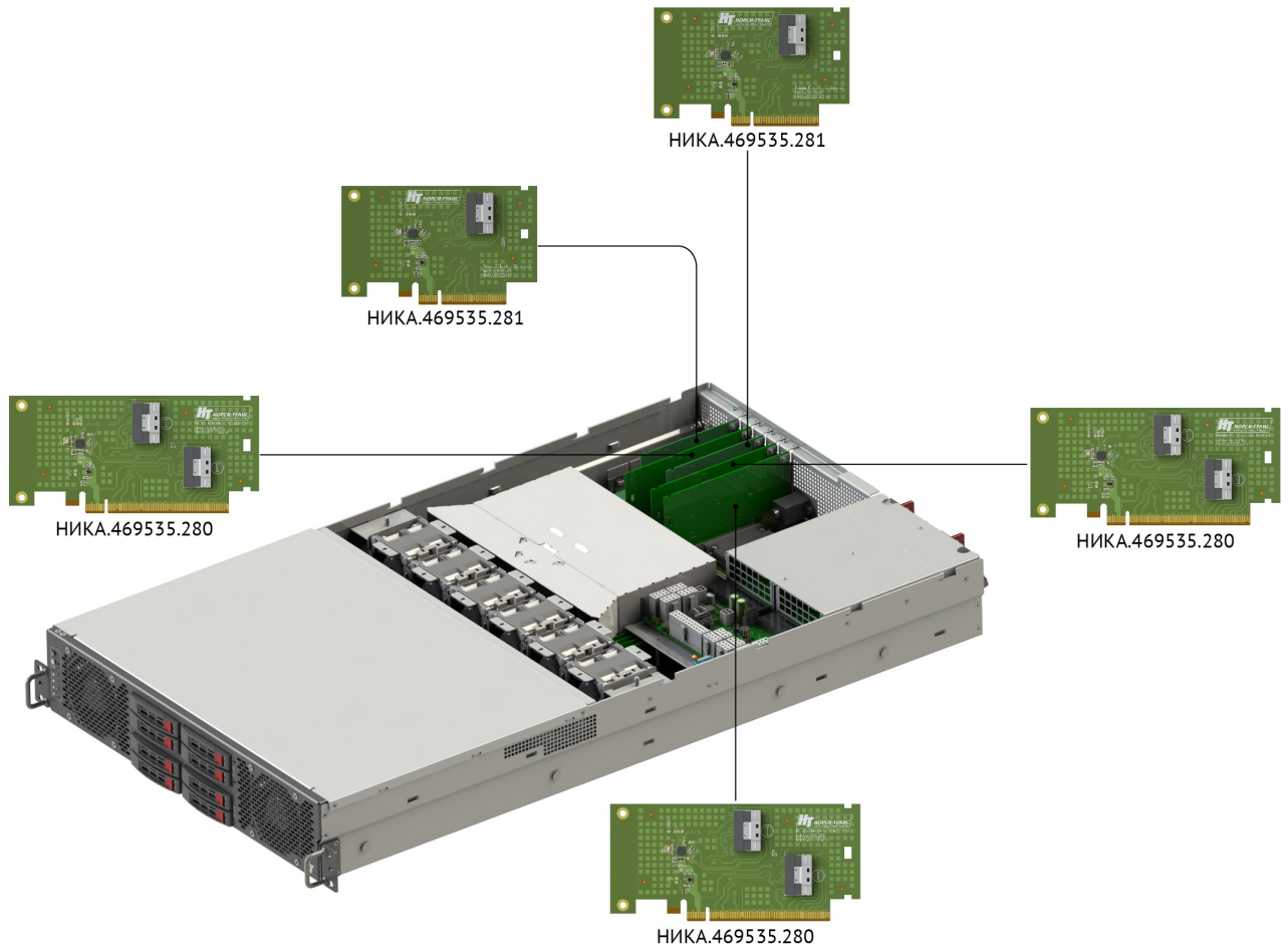
Рис. 12. Расположение PCIe-райзеров в сервере
