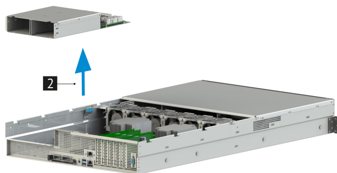
Рис. 24. Извлечение кожуха БП
