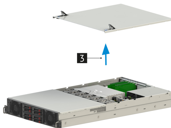
Рис. 18. Снятие задней верхней крышки сервера
