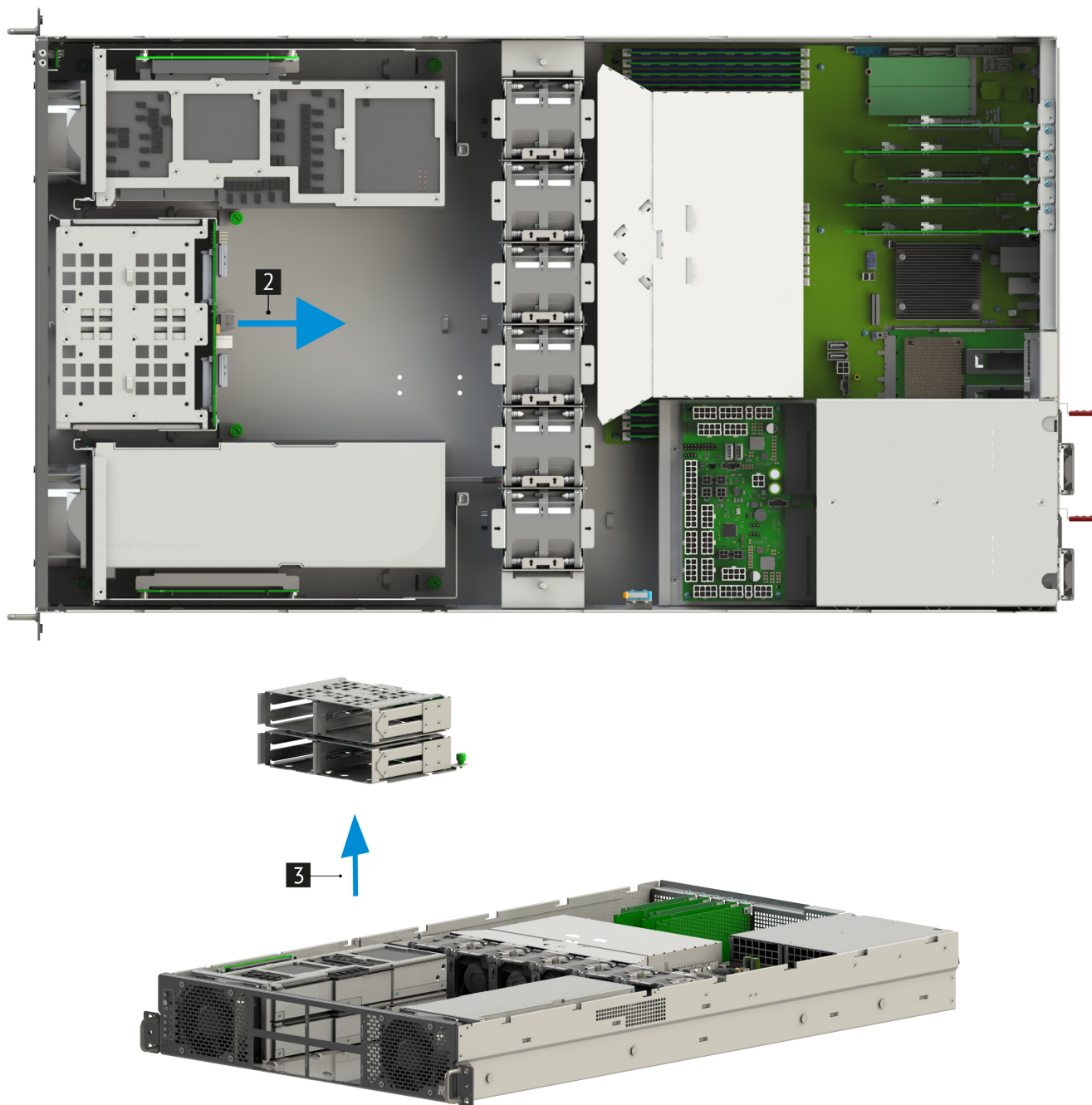
Рис. 26. Извлечение карасов под диски SFF
