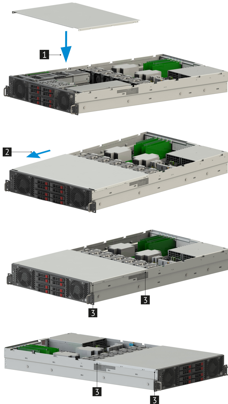
Рис. 21. Установка передней крышки платформы
