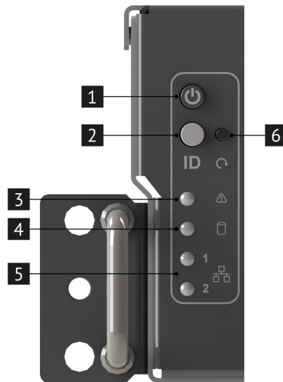
Рис. 5. Левая панель управления
