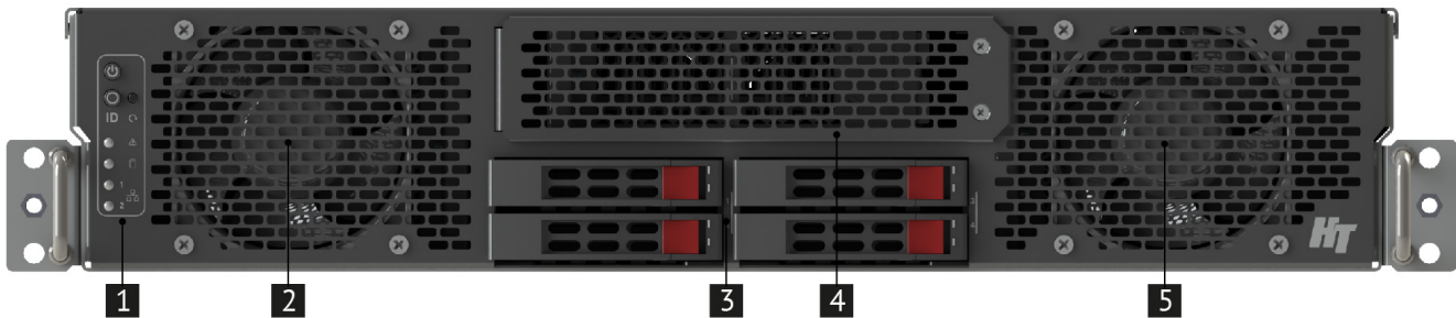
Рис. 4. Вид сервера спереди с 4-мя установленными жесткими дисками
