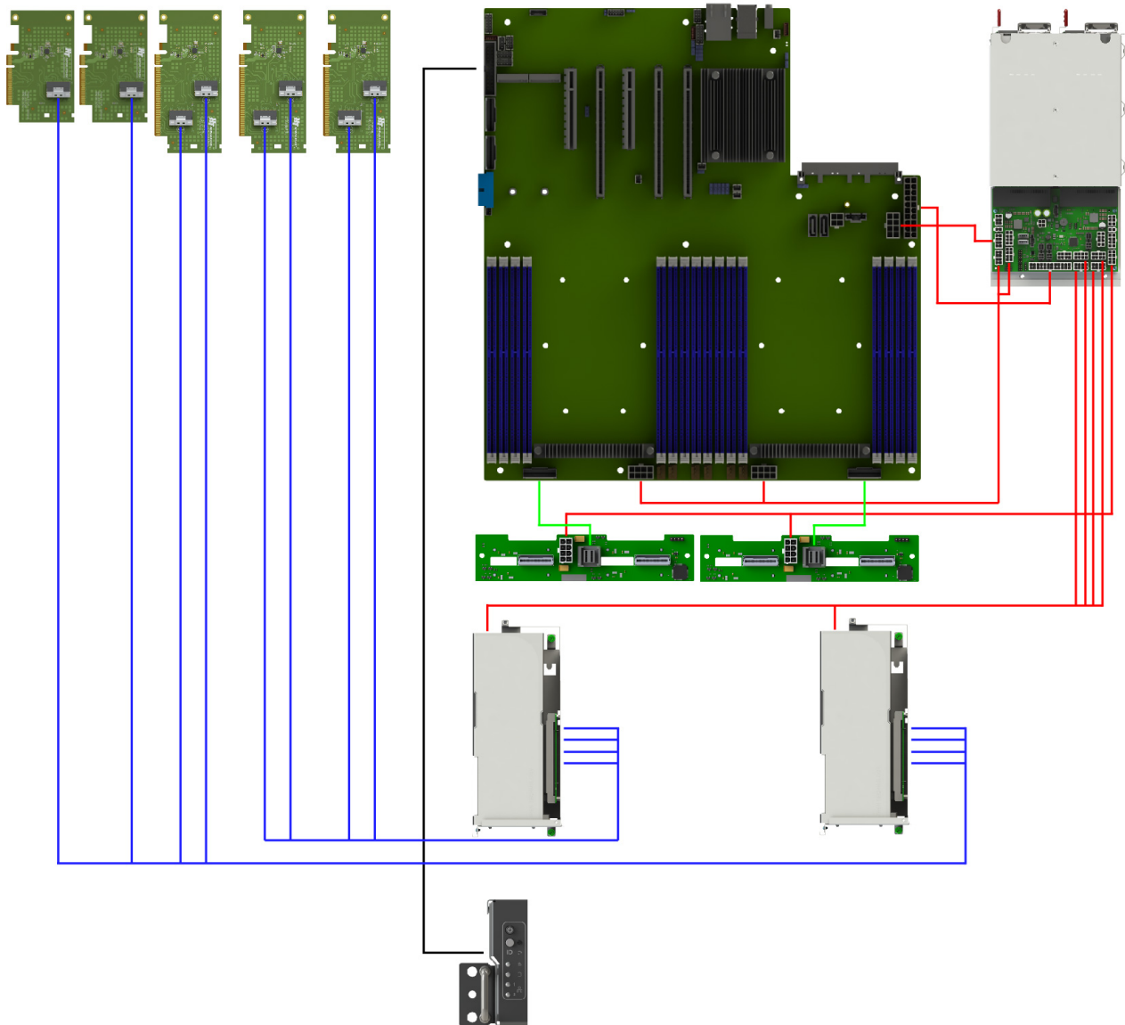
Рис. 31. Схема прокладки системных кабелей, кабелей питания, кабелей для подключения дисков SAS/SATA
