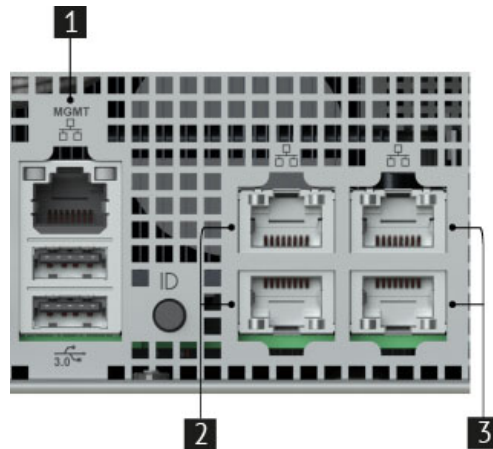
Рис. 6. Сетевые интерфейсы
