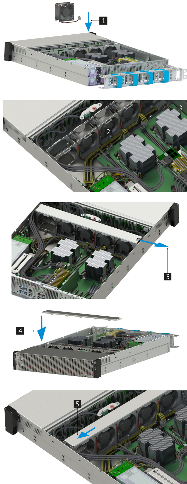
Рис. 27. Подключение вентилятора
