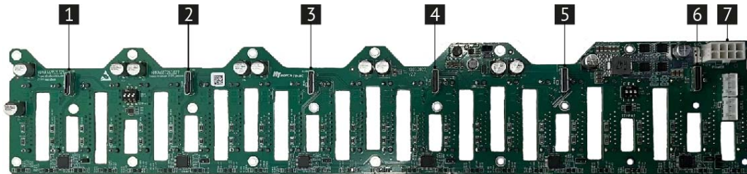
Рис. 10. Плата объединительная 24SFF пассивная (НИКА.469535.121)
