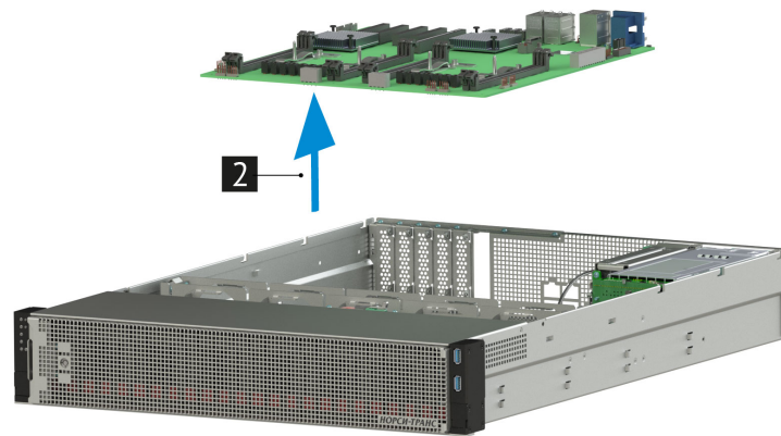
Рис. 36. Извлечение материнской платы из сервера
