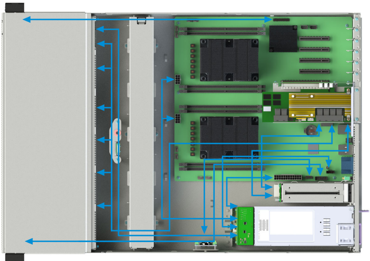
Рис. 24. Схема прокладки кабелей в сервере
