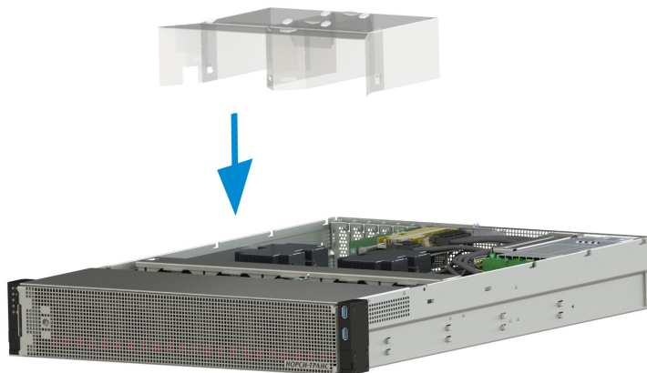
Рис. 23. Установка воздушного кожуха
