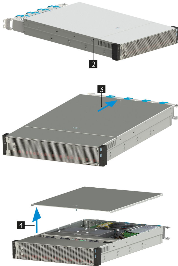
Рис. 20. Снятие верхней крышки сервера
