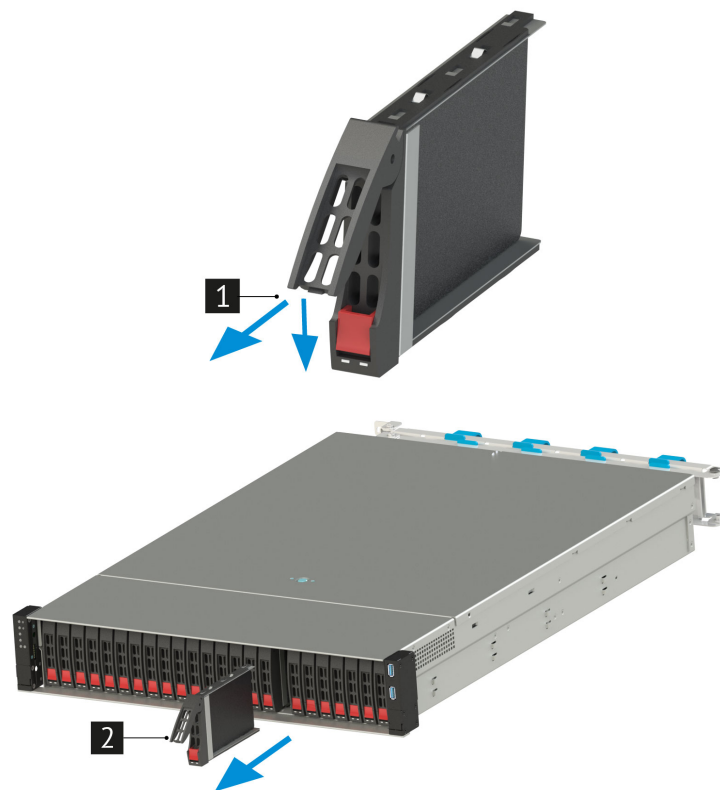
Рис. 38. Извлечение дисков
