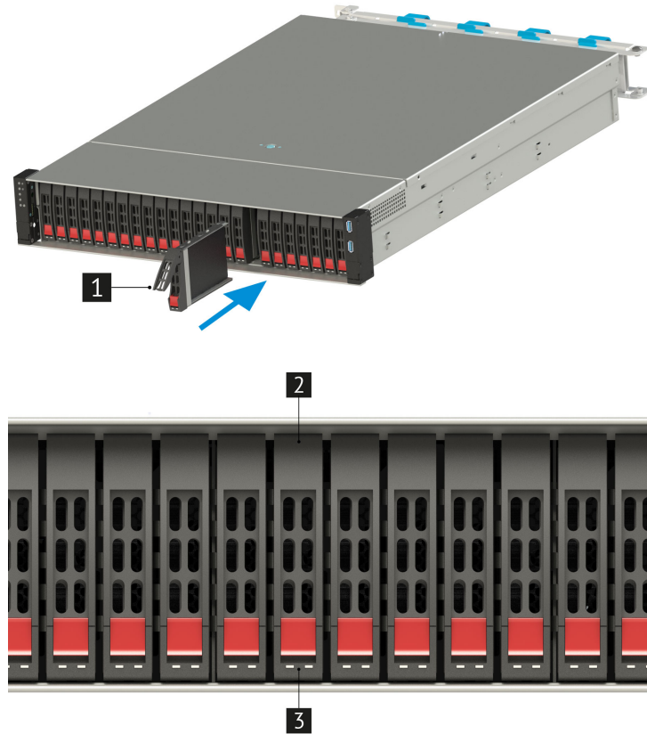
Рис. 39. Установка дисков
