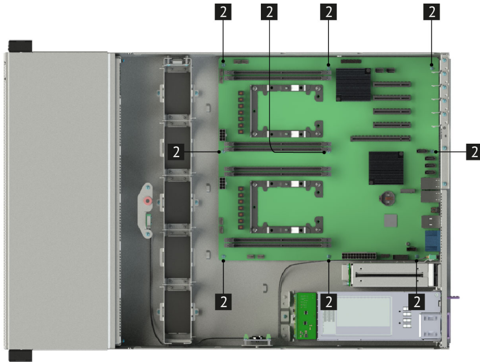
Рис. 37. Установка материнской платы в сервер
