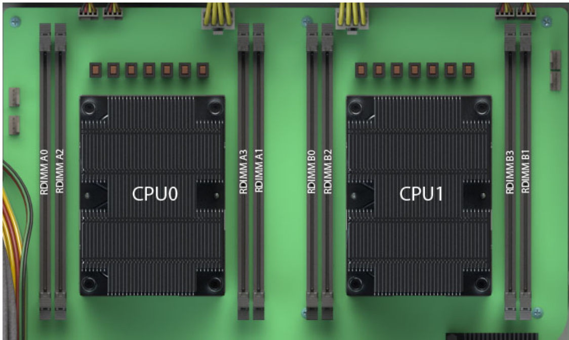
Рис. 28. Расположение разъемов
