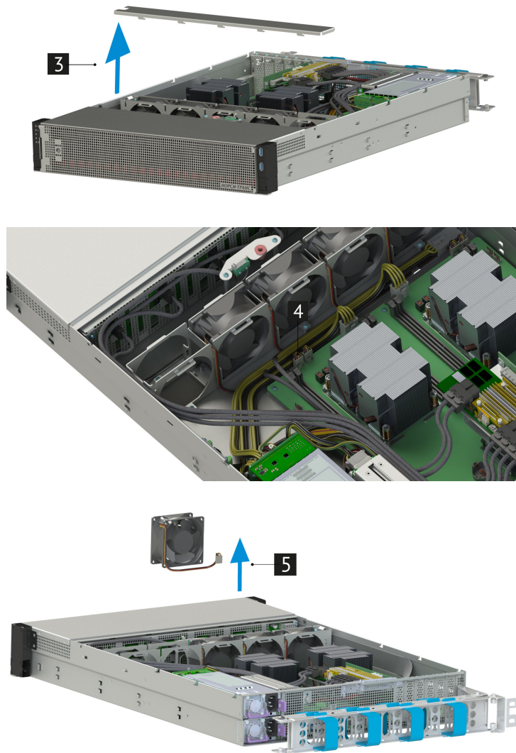
Рис. 26. Извлечение вентилятора из сервера
