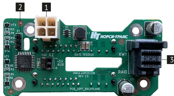
Рис. 12. Плата расширения 2SFF (НИКА.469535.038)
