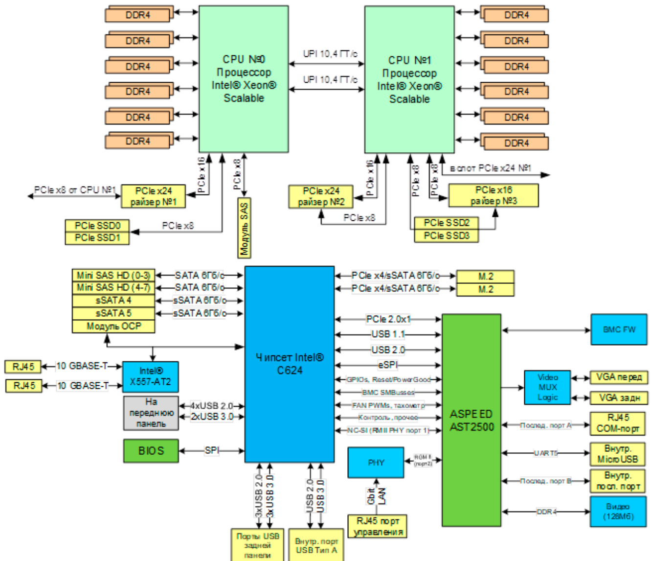
Рис. 1. Структурная схема материнской платы «НТ» НИКА.469555.001
