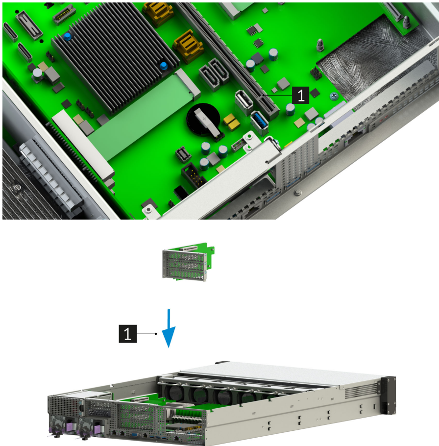
Рис. 50. Установка райзера PCIe 1x24-8-8-8
