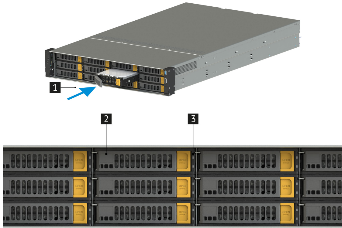
Рис. 46. Установка дисков
