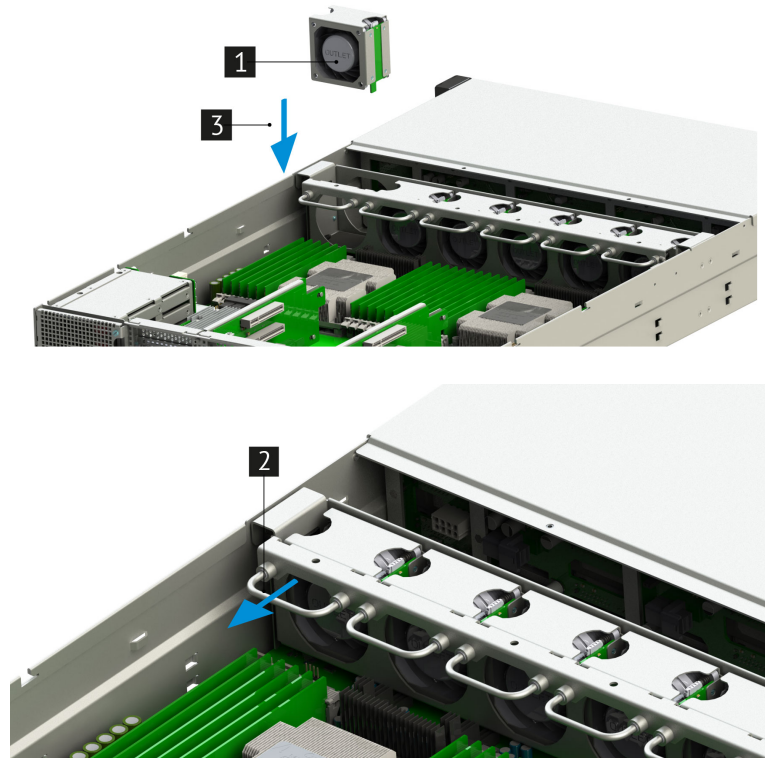
Рис. 32. Подключение вентилятора
