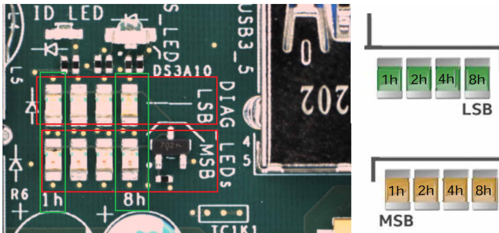
Рис. 6. Расположение и определение POST CODE LED
