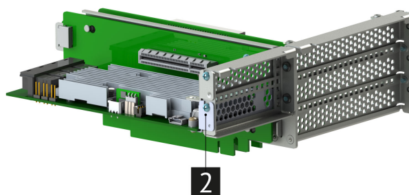
Рис. 54. Установка контроллера дискового MegaRAID 9361-16i
