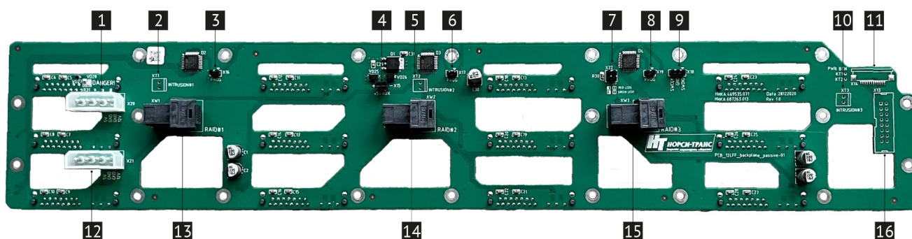
Рис. 11. Плата расширения 12LFF (НИКА.469535.071)
