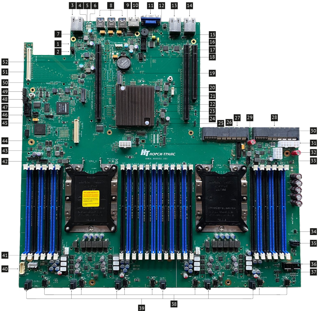
Рис. 12. Соединители и переключатели материнской платы
