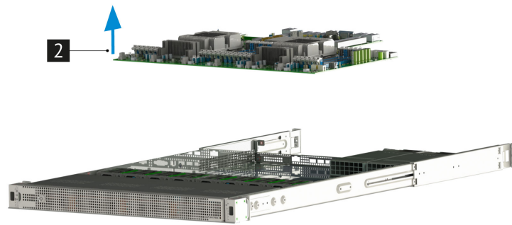
Рис. 38. Извлечение материнской платы
