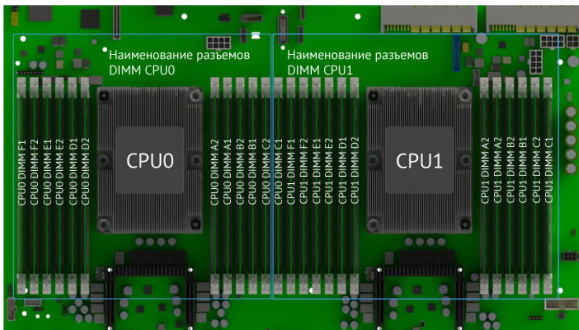
Рис. 30. Расположение разъемов
