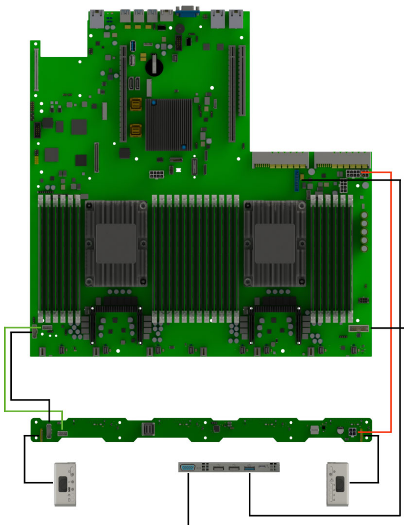
Рис. 25. Схема прокладки системных кабелей и кабелей питания
