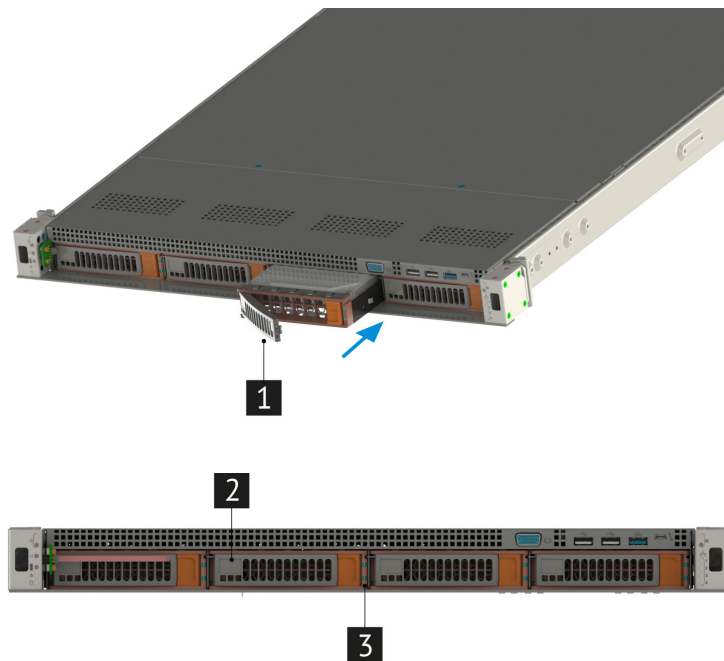
Рис. 42. Извлечение дисков
