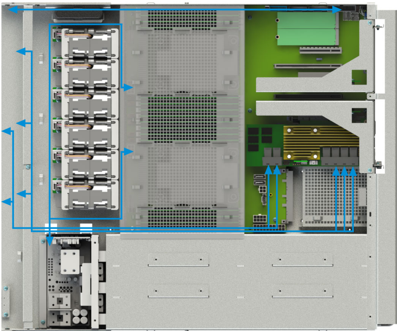
Рис. 26. Схема прокладки кабелей в модуле НИКА.467239.008 сервера
