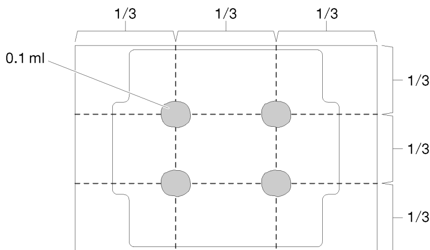
Рис. 40. Нанесение термопасты
