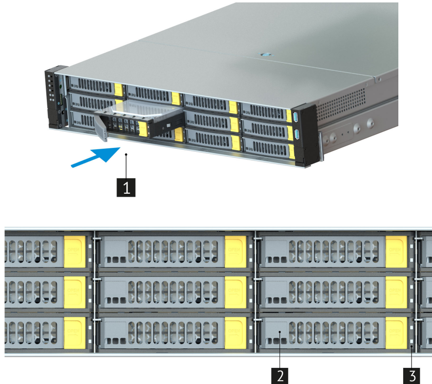
Рис. 51. Извлечение дисков
