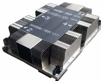
Рис. 41. 1U радиатор
