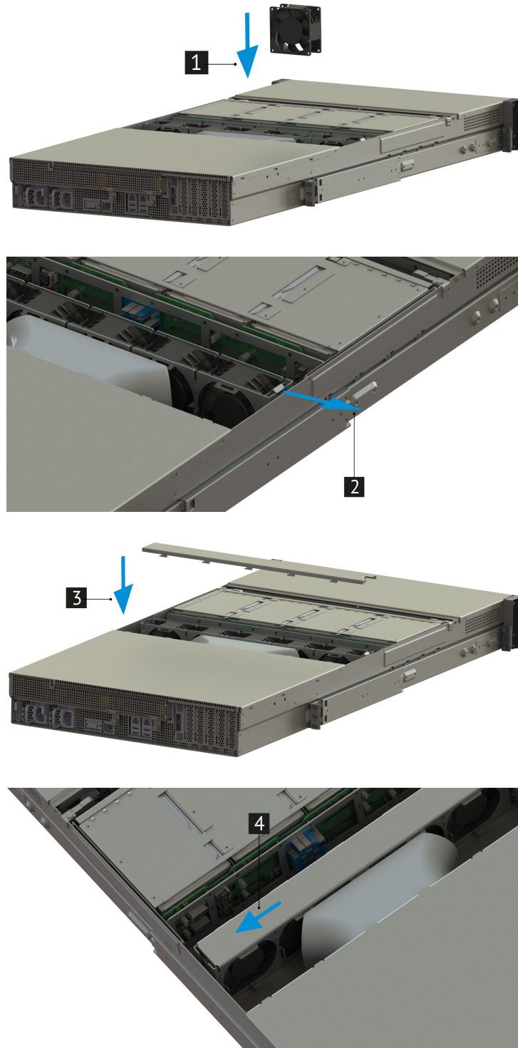
Рис. 36. Подключение вентилятора
