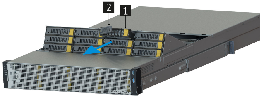
Рис. 52. Извлечение дисков
