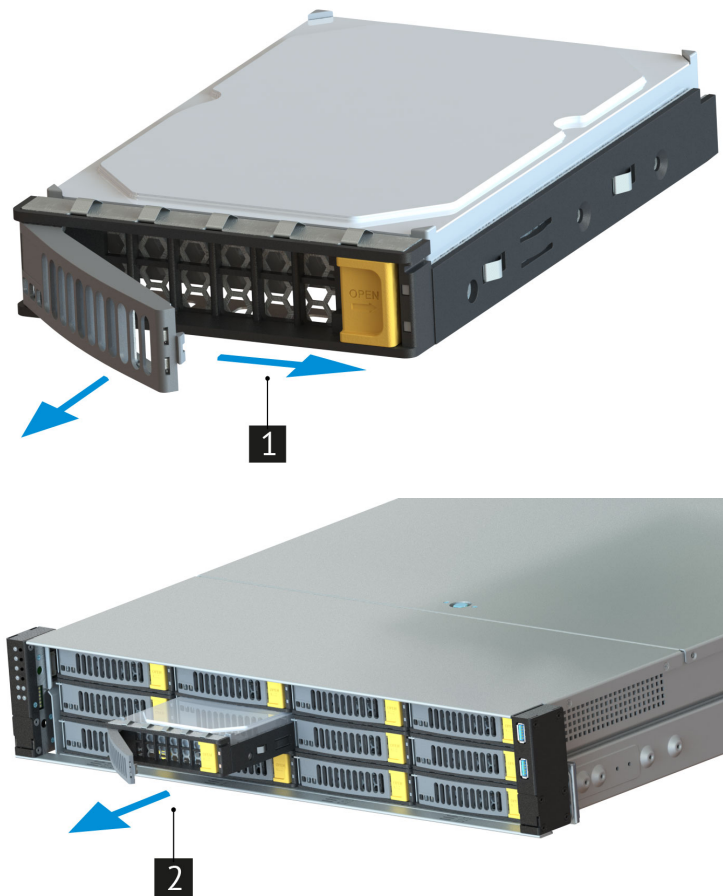
Рис. 50. Извлечение дисков
