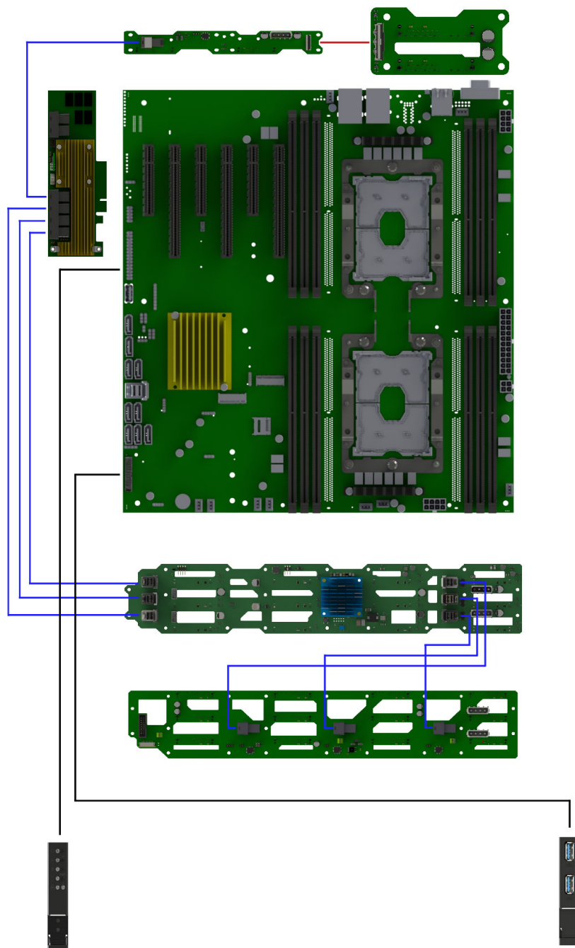
Рис. 34. Схема прокладки системных кабелей и кабелей питания
