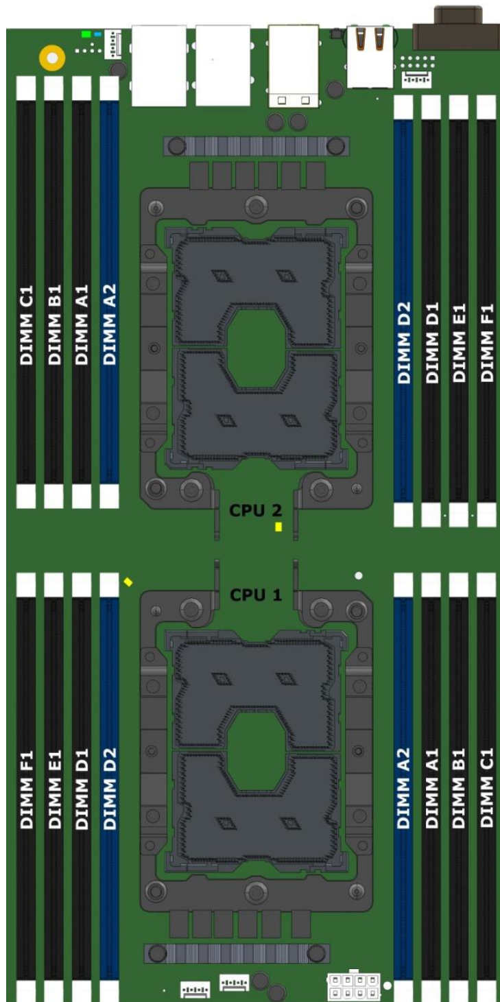
Рис. 37. Расположение разъемов
