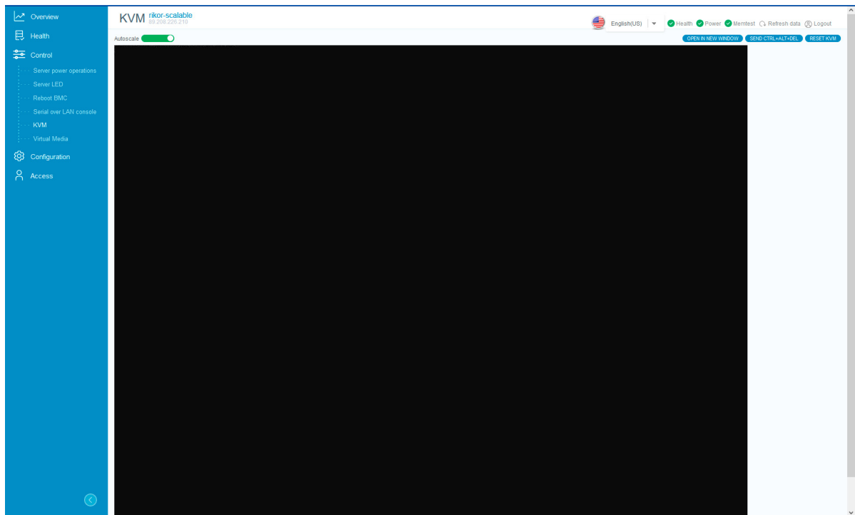
Рис. 86. Окно «KVM»
