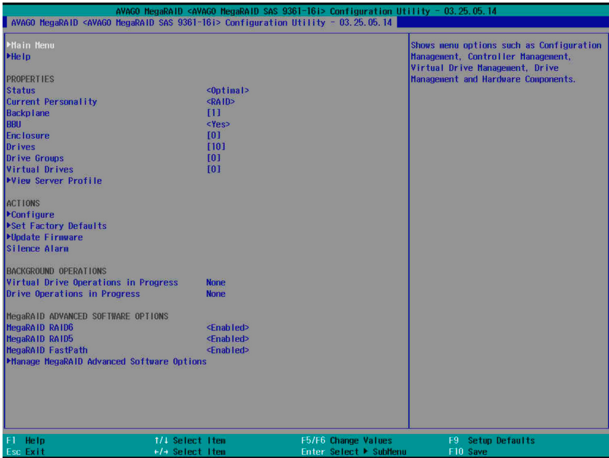
Рис. 77. Меню «AVAGO MegaRAID»
