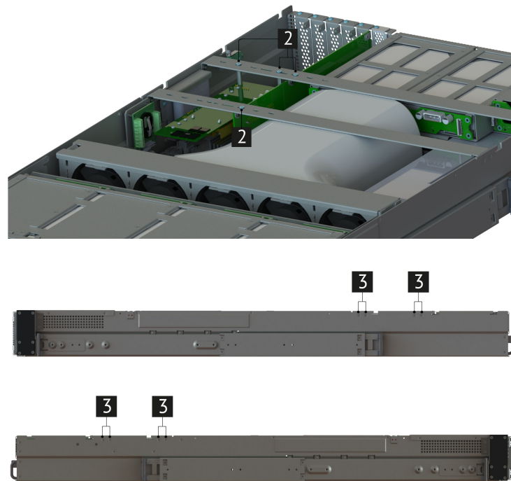
Рис. 28. Установка скоб
