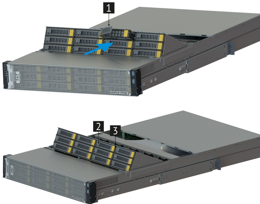
Рис. 53. Извлечение дисков
