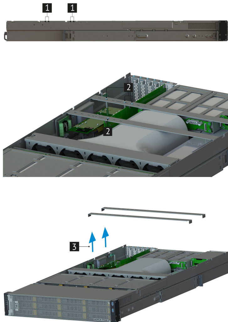
Рис. 27. Снятие скоб
