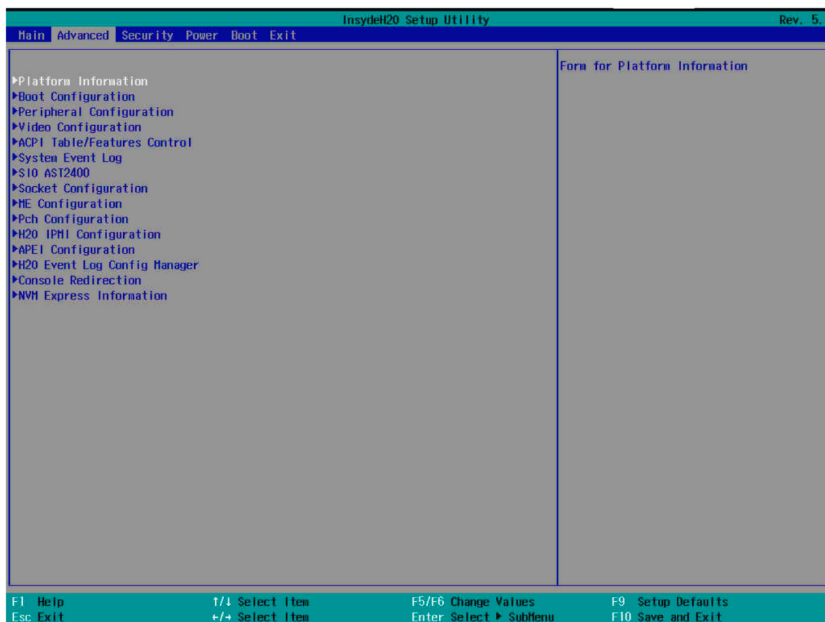
Рис. 63. Разделы меню «Advanced»
