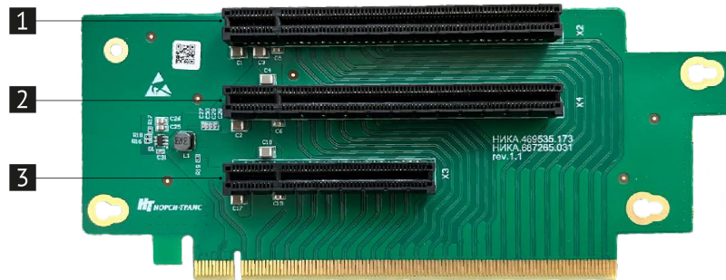
Рис. 15. Райзер 1x24-16-16-8 (НИКА.469535.173)
