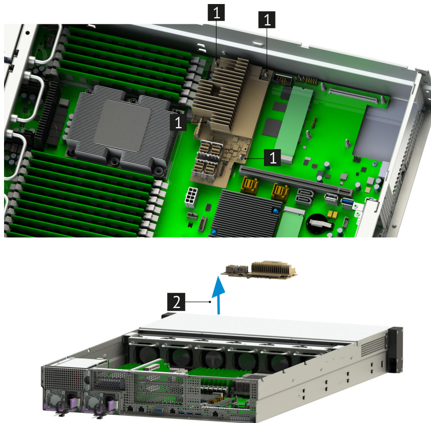
Рис. 55. Извлечение наплатного RAID-контроллера
