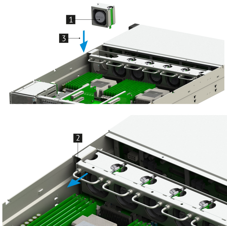
Рис. 32. Подключение вентилятора
