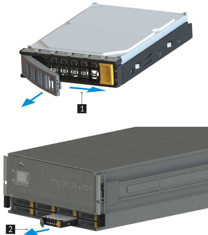
Рис. 42. Извлечение дисков
