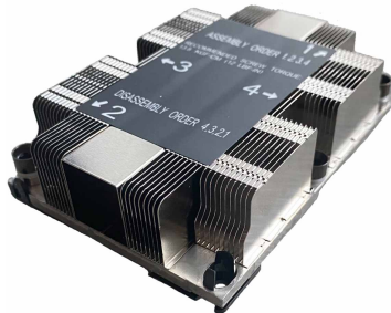
Рис. 34. 1U радиатор
