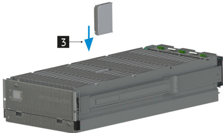
Рис. 45. Установка диска в массив дисков
