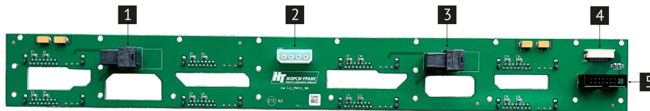
Рис. 10. Плата дискового массива А8 (НИКА.469535.013)
