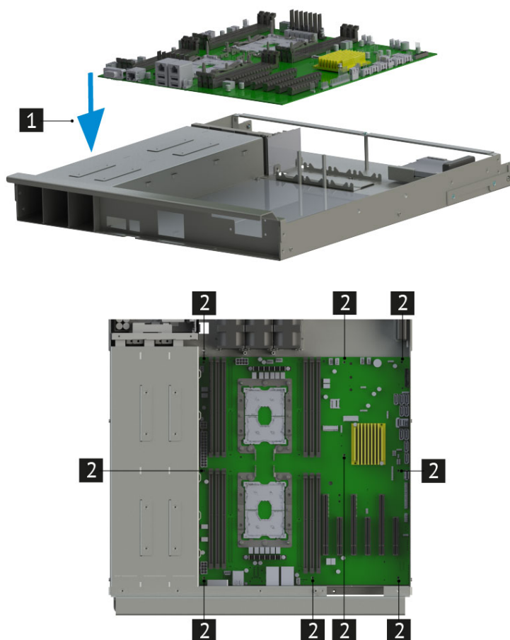
Рис. 41. Установка материнской платы
