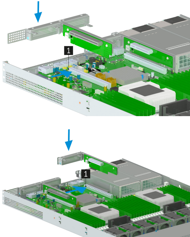
Рис. 46. Установка PCIe-райзера с основанием в корпус сервера
