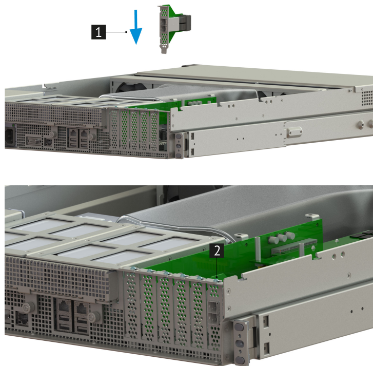
Рис. 49. Установка платы-переходника MiniSAS HD 8i-8e
