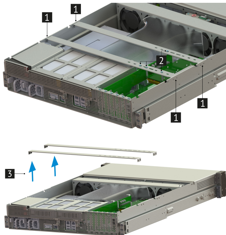
Рис. 22. Снятие скоб
