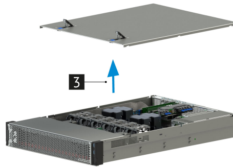
Рис. 22. Снятие верхней крышки сервера
