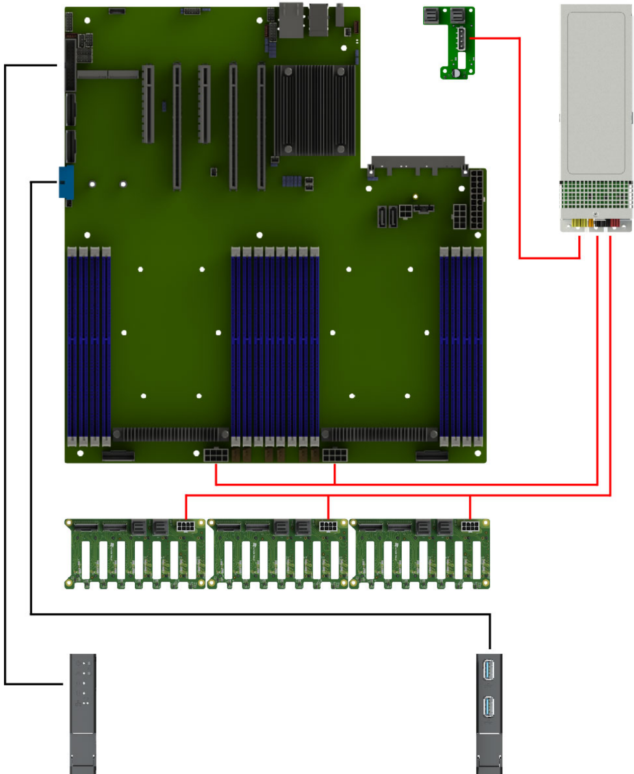
Рис. 26. Схема прокладки системных кабелей и кабелей питания при использовании платы расширения 2SF NVMe (НИКА.469535.220)
