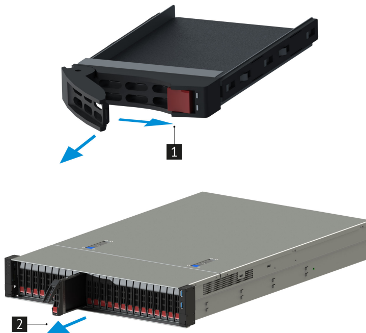
Рис. 45. Извлечение дисков
