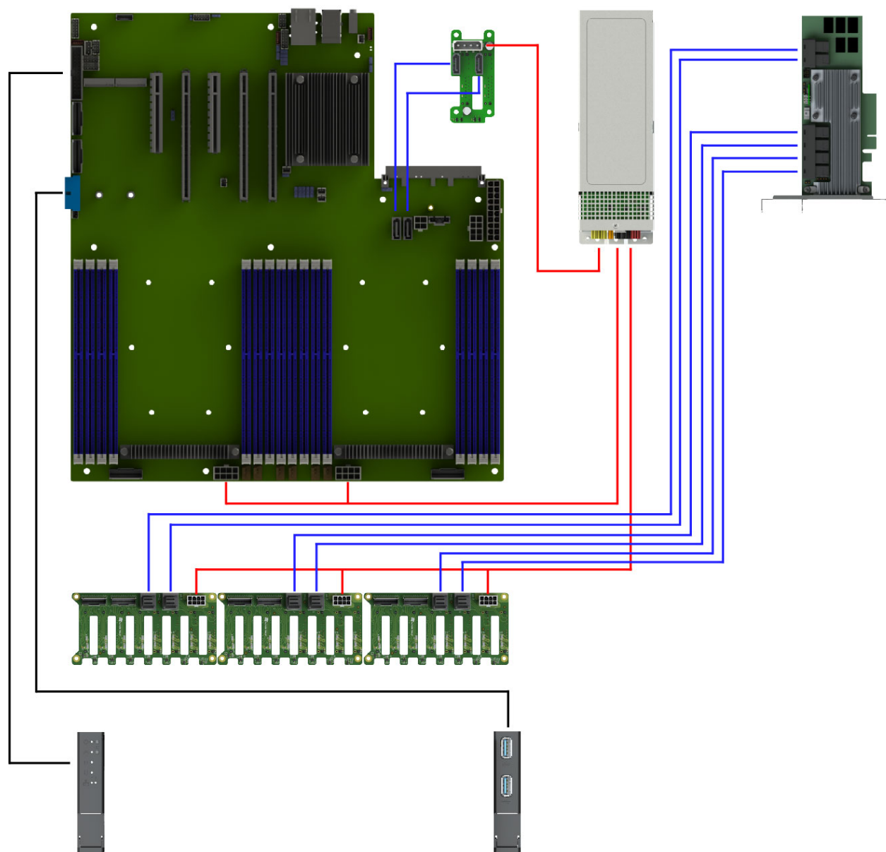
Рис. 28. Схема прокладки системных кабелей и кабелей питания с подключением PCIe RAID при использовании платы расширения 2SFf SATA (НИКА.469535.131)
