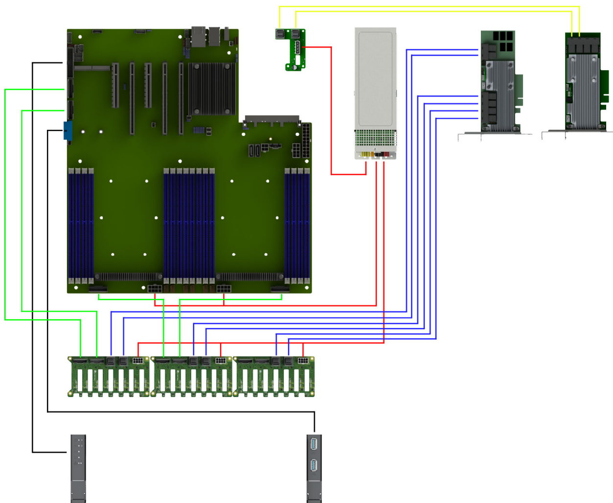
Рис. 31. Схема прокладки системных кабелей и кабелей Oculink-SLIMline X8-X8 с подключением PCIe RAID при использовании платы расширения 2SF NVMe (НИКА.469535.220)
