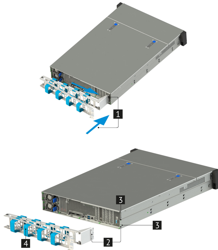
Рис. 17. Установка дополнительного кабельного органайзера.
