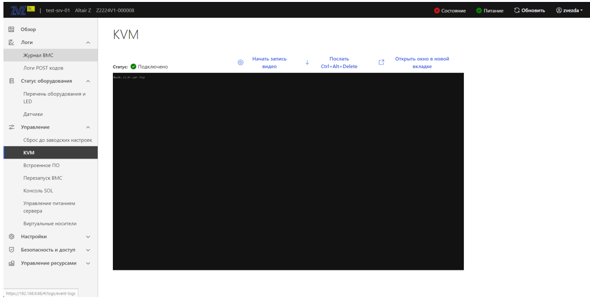
Рис. 81. Окно «KVM»
