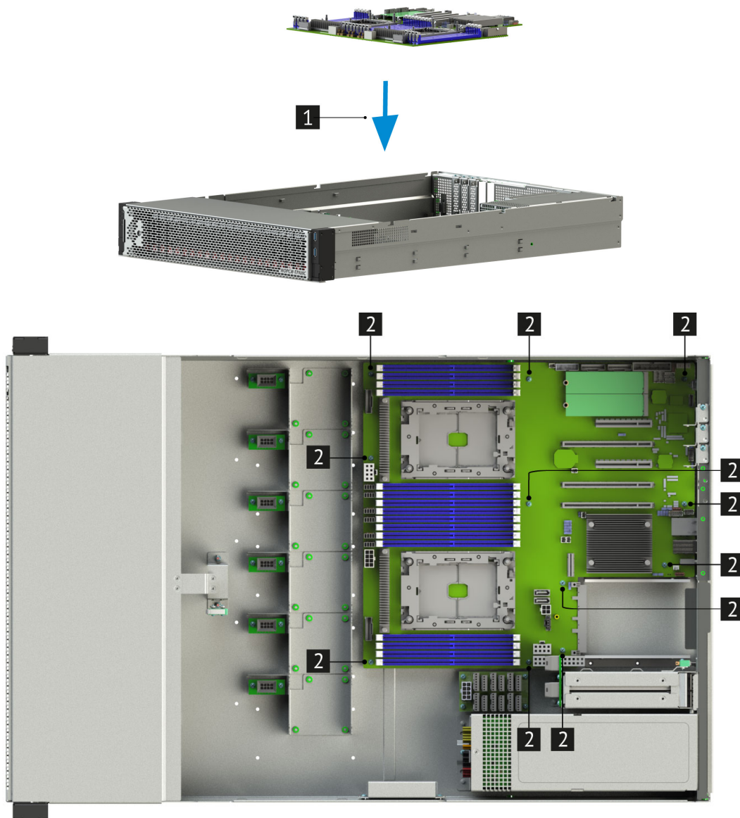
Рис. 44. Установка материнской платы в сервер
