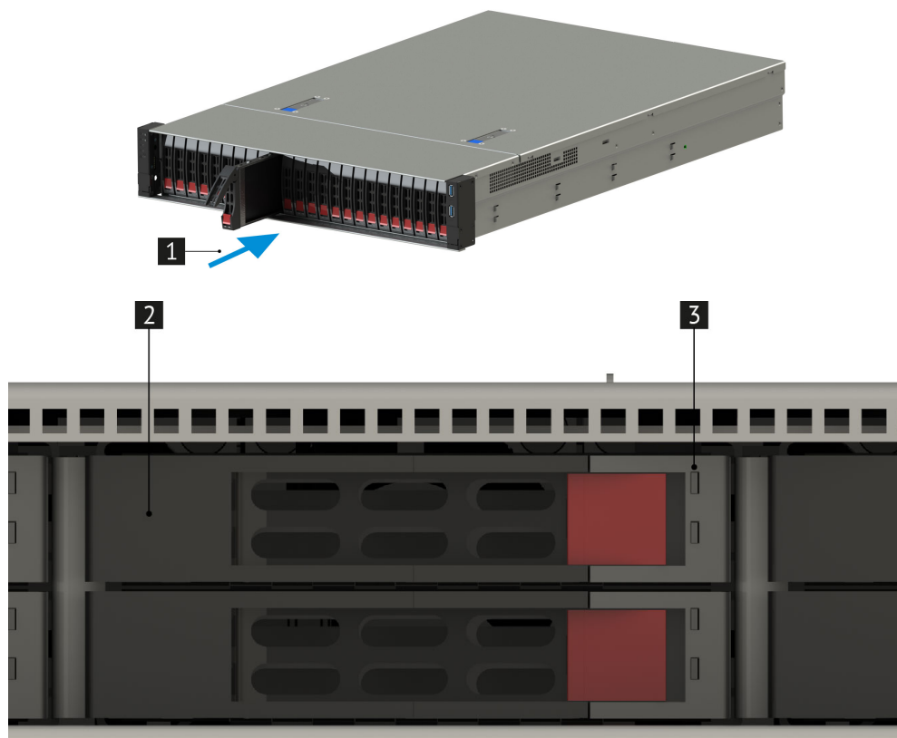
Рис. 46. Установка дисков
