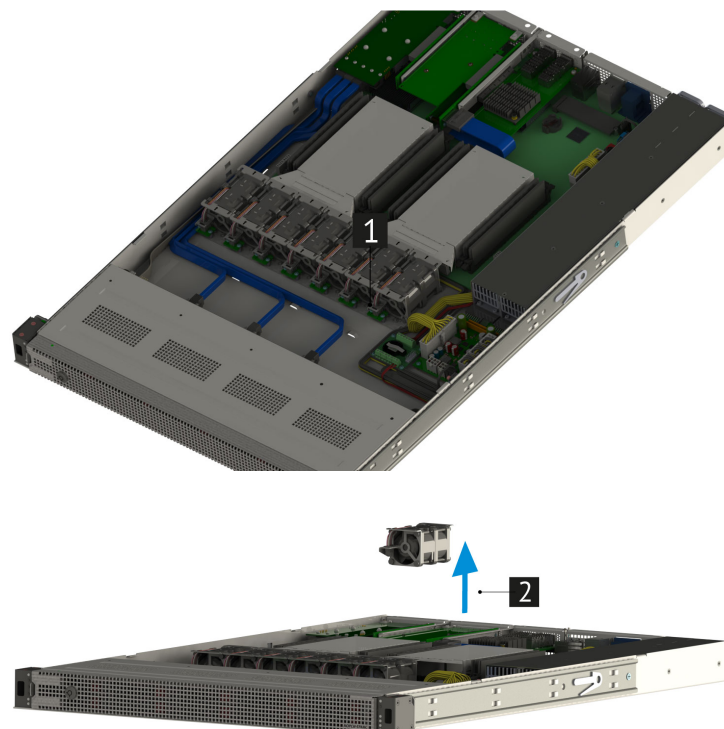
Рис. 26. Извлечение вентилятора из сервера
