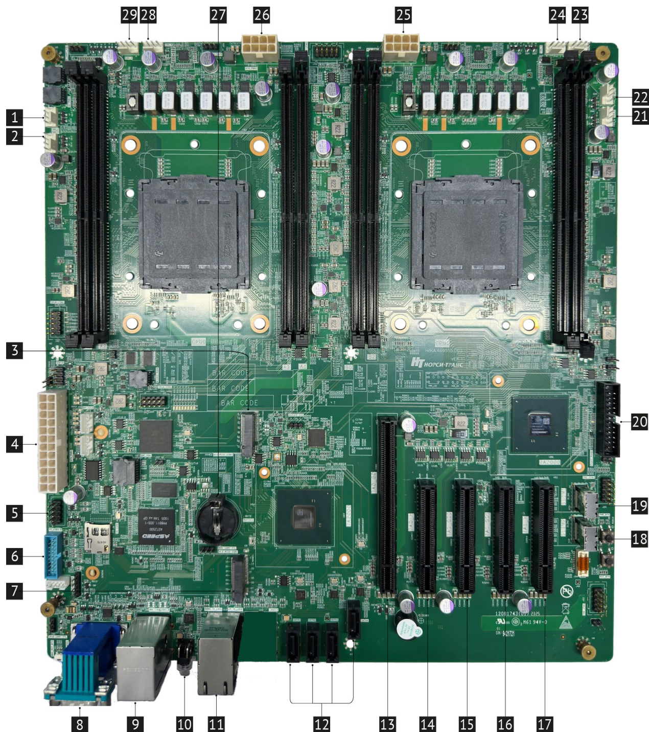
Рис. 10. Соединители и переключатели материнской платы
