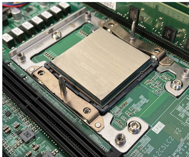
Рис. 32. Извлечение радиатора из сервера
