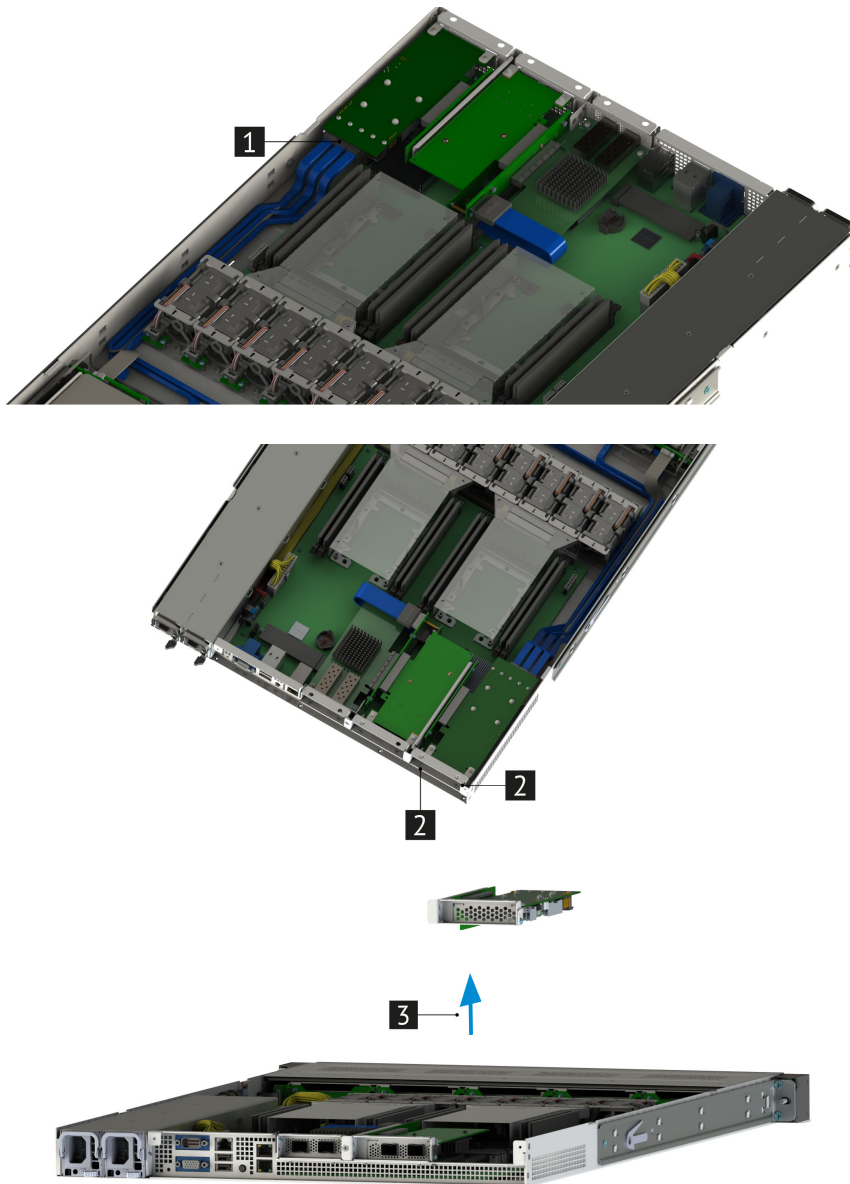
Рис. 41. Извлечение райзера PCIe 1U x8-x8
