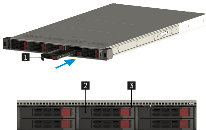
Рис. 39. Установка дисков
