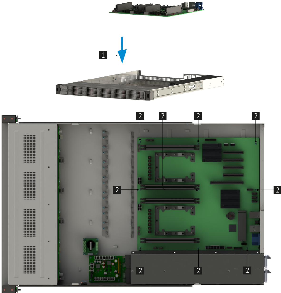
Рис. 37. Установка материнской платы в сервер
