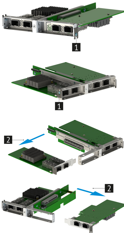
Рис. 47. Извлечение карт расширения
