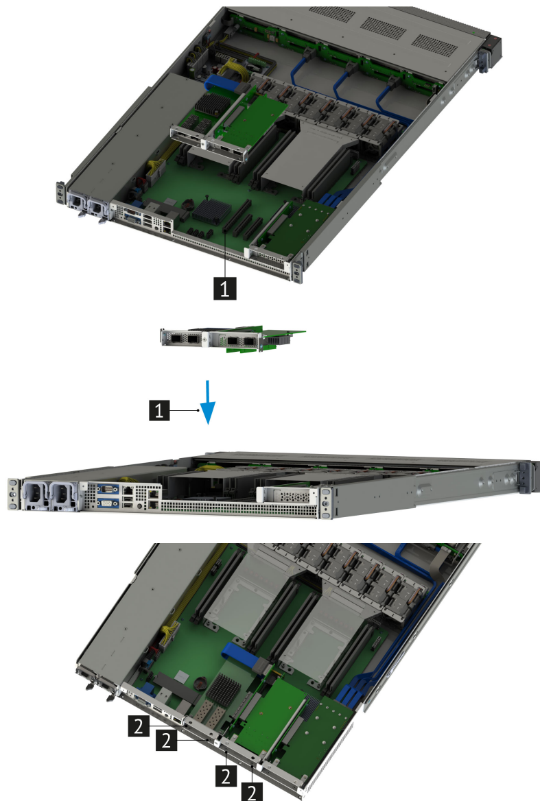
Рис. 44. Установка райзера PCIe 1U x16-x8-x8-Ос
