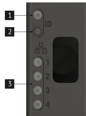
Рис. 4. Правая панель управления
