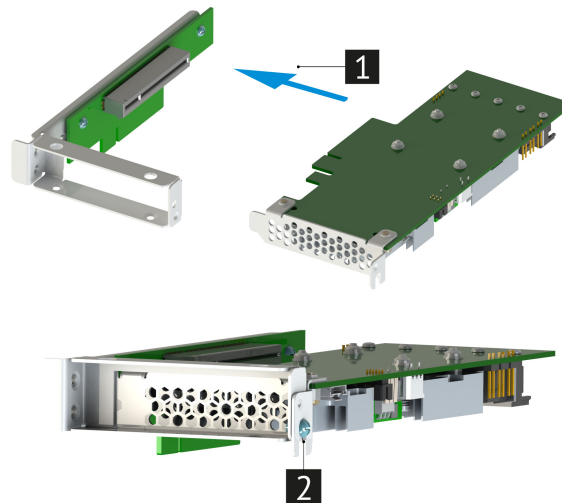
Рис. 46. Установка контроллера дискового MegaRAID 9361-16i
