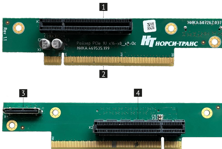
Рис. 13. Райзер PCIe 1U x16-x8-x8-0c (НИКА.469535.199)
