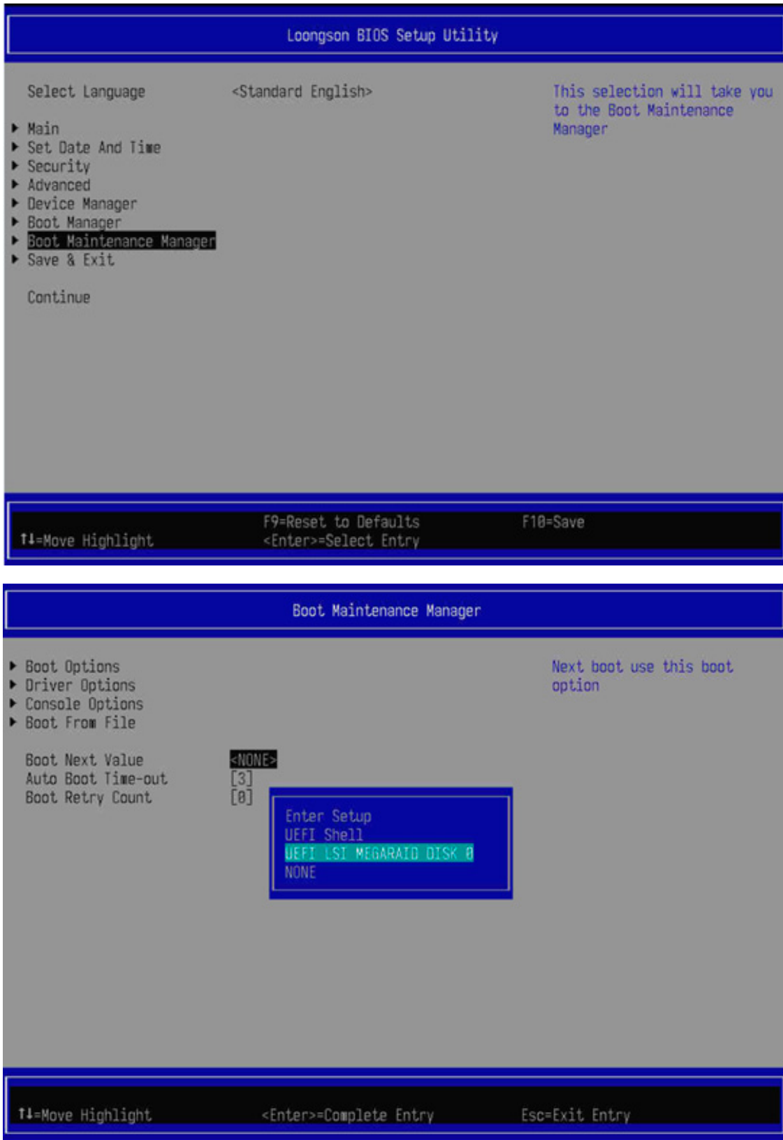
Рис. 90. Выбор RAID-массива как основного boot загрузчика
