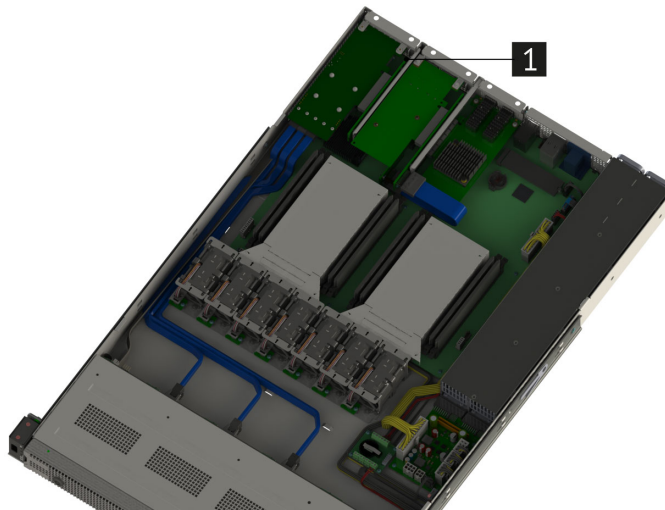
Рис. 40. Расположение райзера PCIe 1U x8-x8 в сервере
