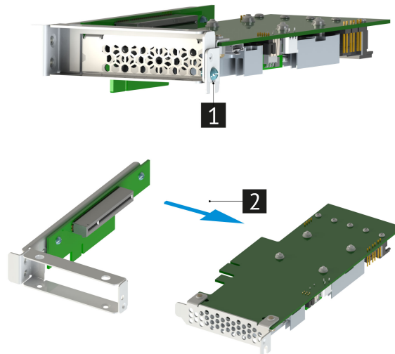
Рис. 45. Извлечение контроллера дискового MegaRAID 9361-16i
