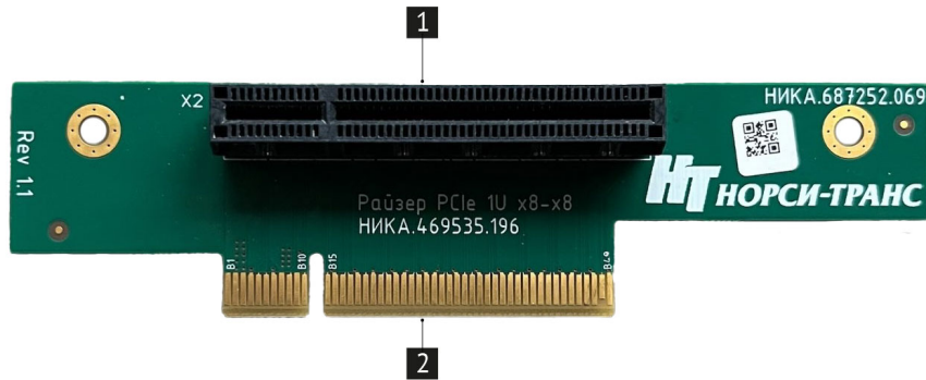
Рис. 12. Райзер PCIe 1U x8-x8 (НИКА.469535.196)
