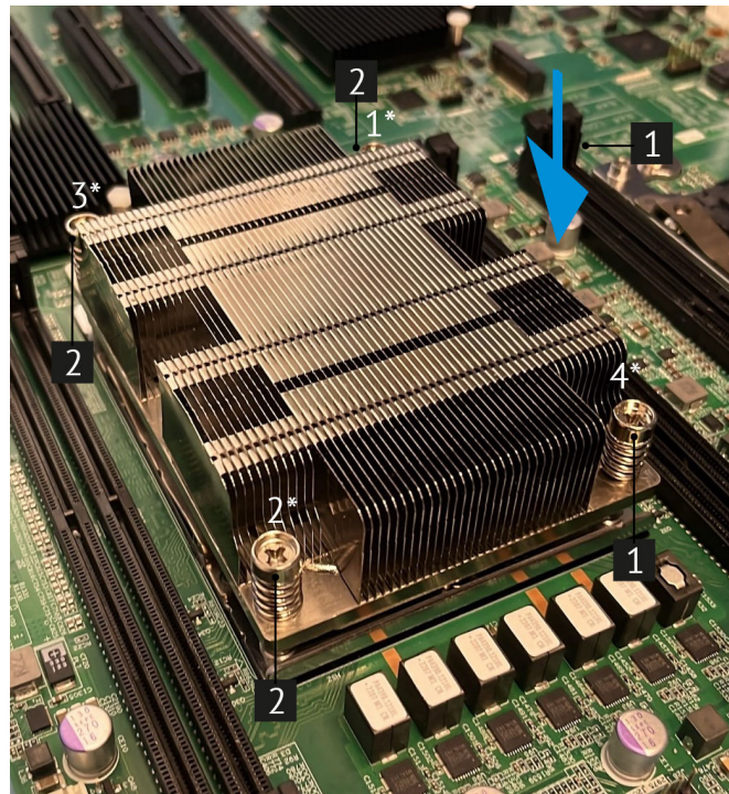
Рис. 33. Установка радиатора
