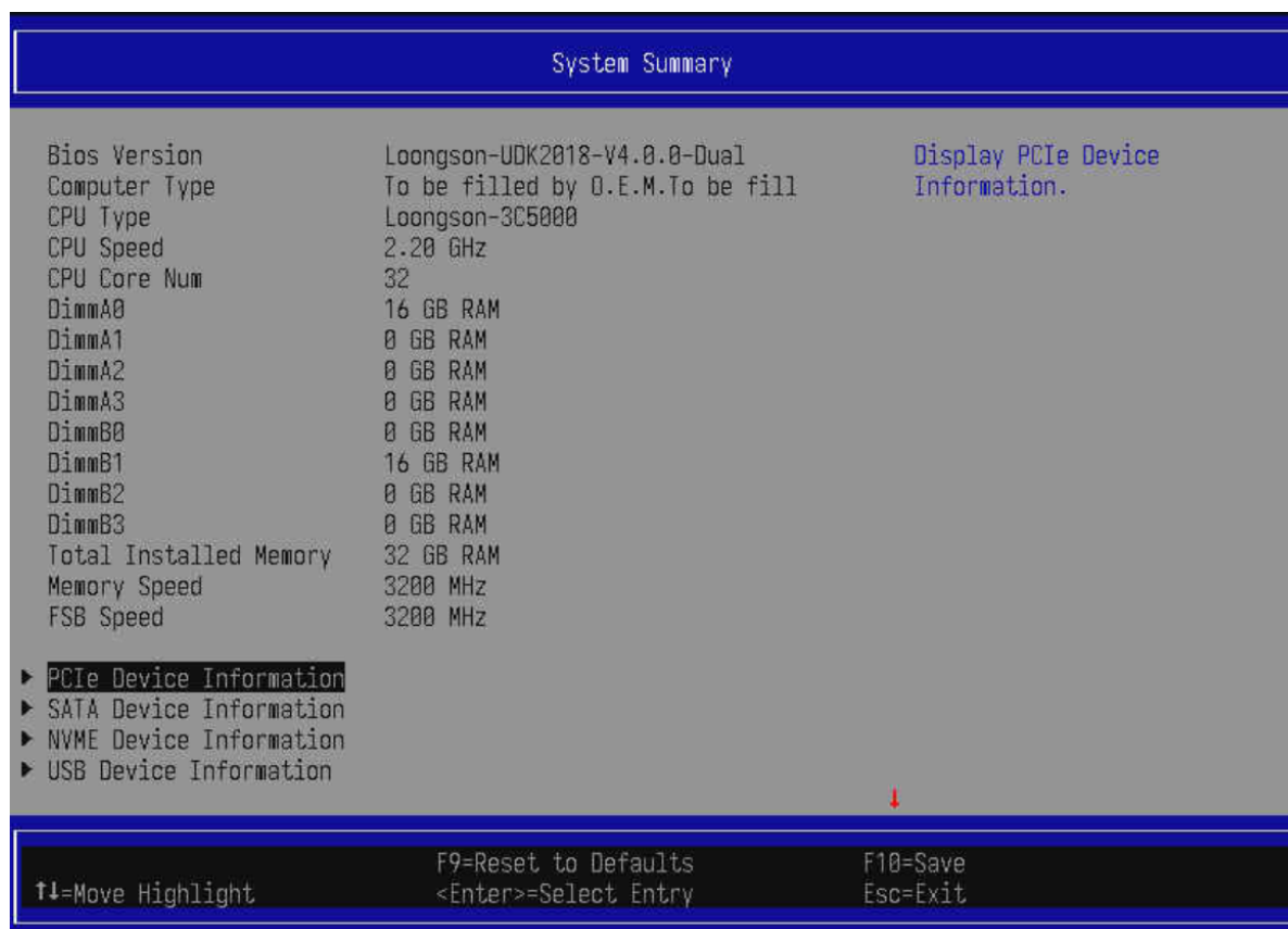
Рис. 57. Разделы меню «Main»
