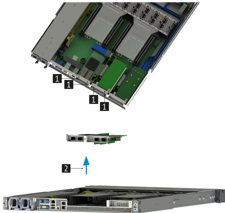
Рис. 43. Извлечение райзера PCIe 1U x16-x8-x8-0c
