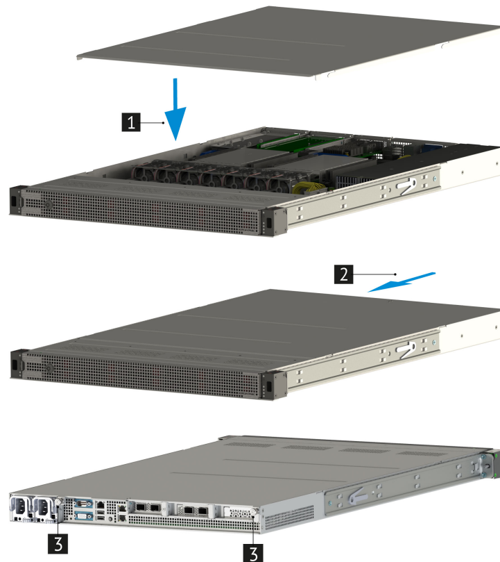
Рис. 21. Установка верхней крышки сервера
