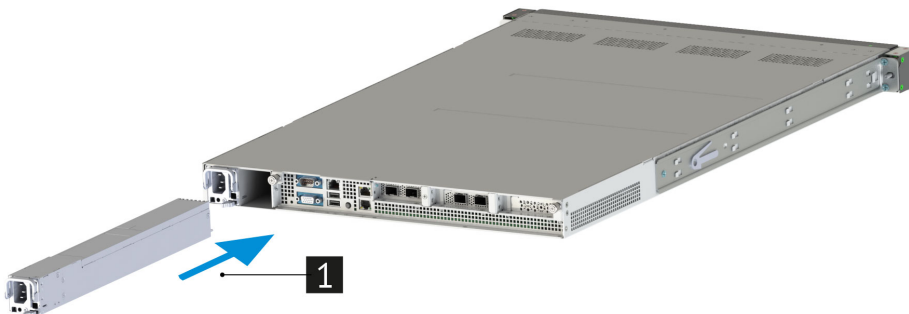
Рис. 53. Установка блока питания сервера
