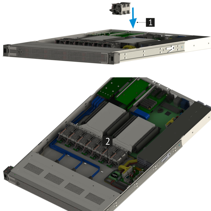
Рис. 27. Подключение вентилятора
