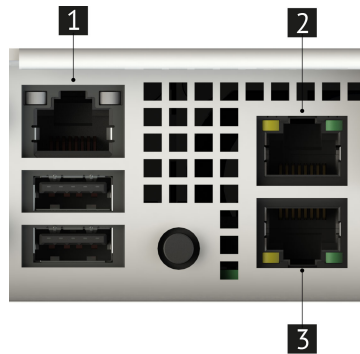
Рис. 7. Сетевые интерфейсы
