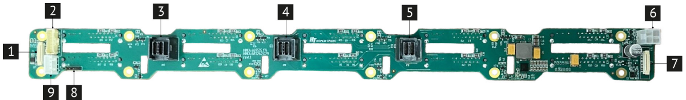
Рис. 11. Плата расширения 10SFF SAS (НИКА.469535.174)
