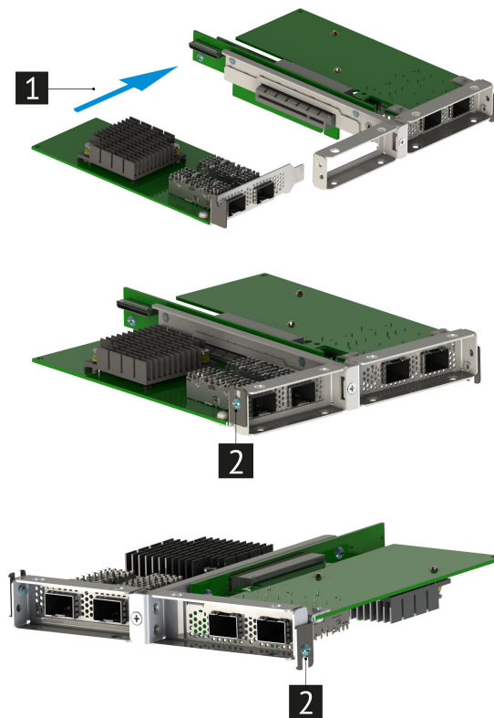
Рис. 48. Установка карт расширения
