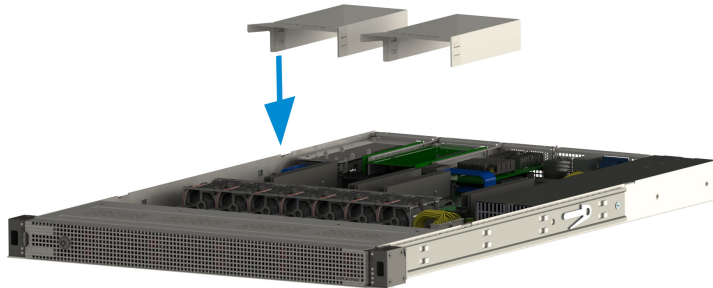
Рис. 23. Установка воздушного кожуха
