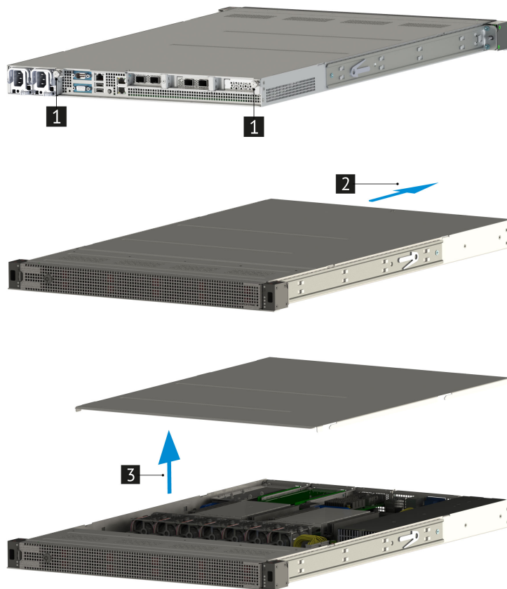
Рис. 20. Снятие верхней крышки сервера
