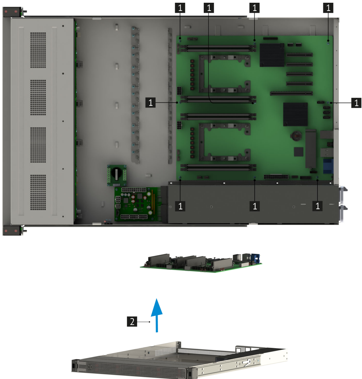
Рис. 36. Извлечение материнской платы из сервера
