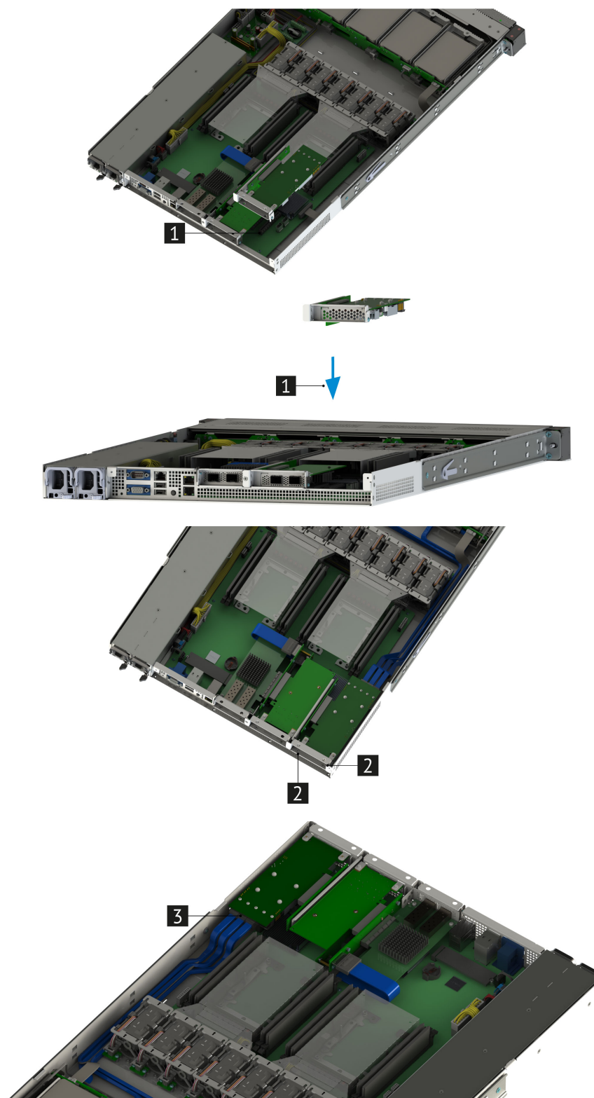
Рис. 42. Установка райзера PCIe 1U x8-x8
