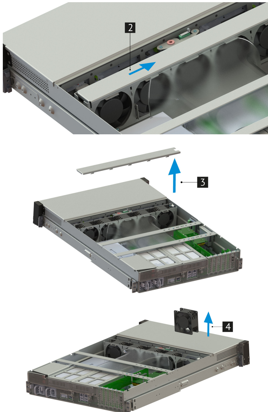
Рис. 30. Извлечение вентилятора
