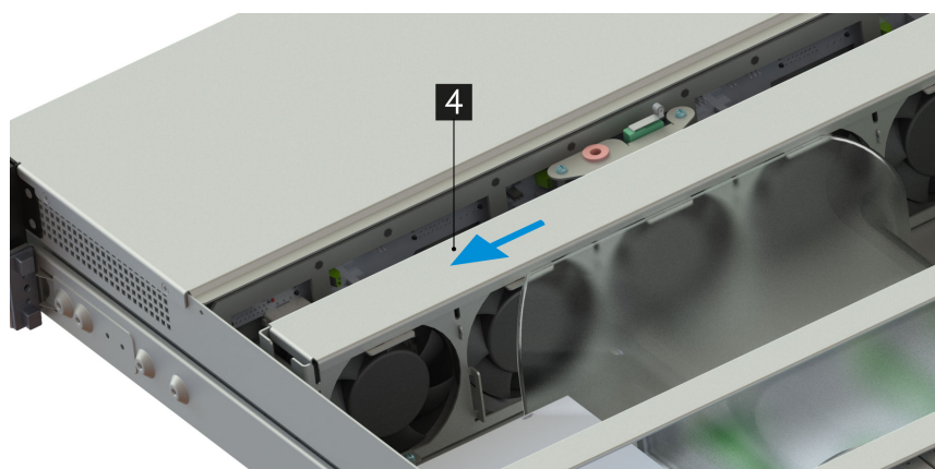
Рис. 31. Подключение вентилятора
