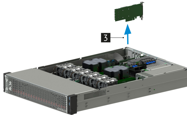
Рис. 56. Извлечение контроллера дискового MegaRAID 9361-16i
