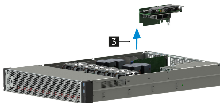
Рис. 52. Извлечение райзера PCIe x16-x16
