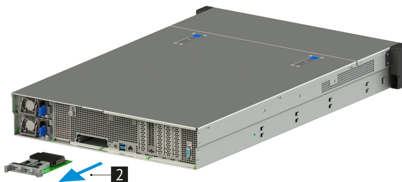
Рис. 58. Извлечение карты OCP 3.0 PCIe x16
