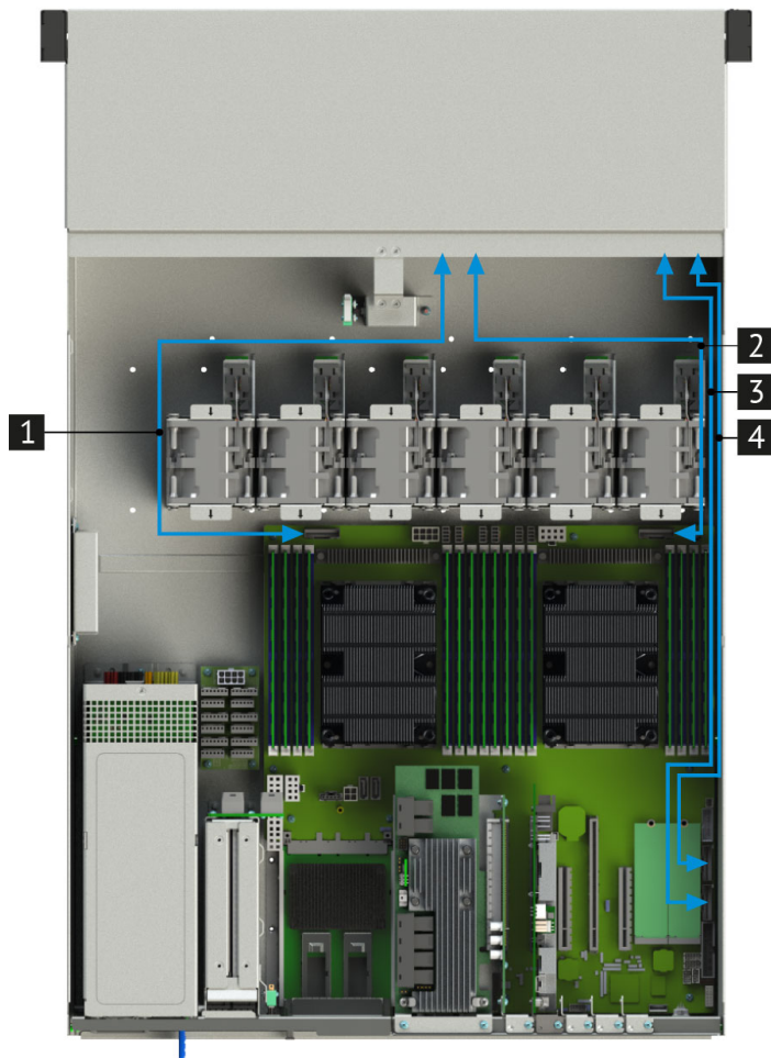
Рис. 48. Схема прокладки кабелей SlimSAS-SLIMline X8-X8
