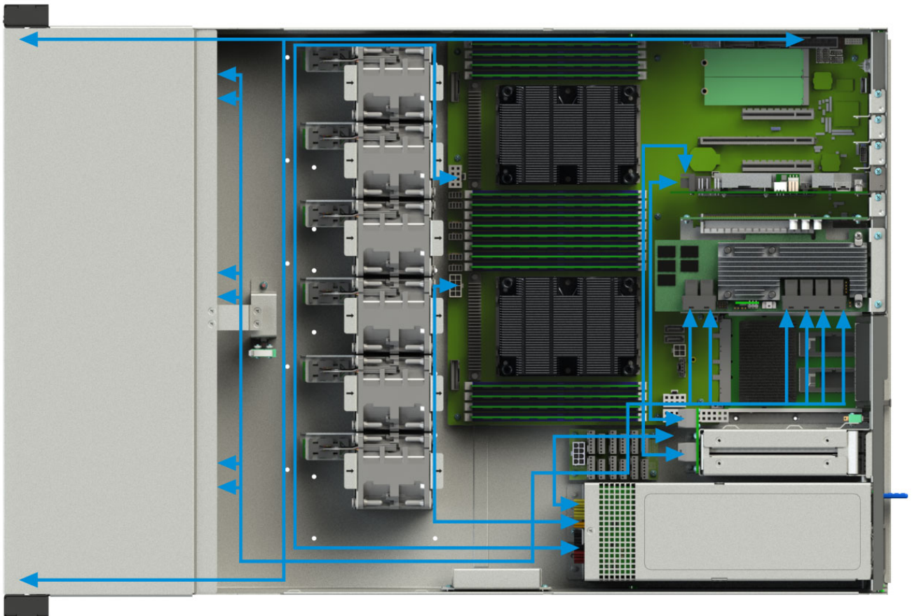
Рис. 24. Схема прокладки кабелей в сервере
