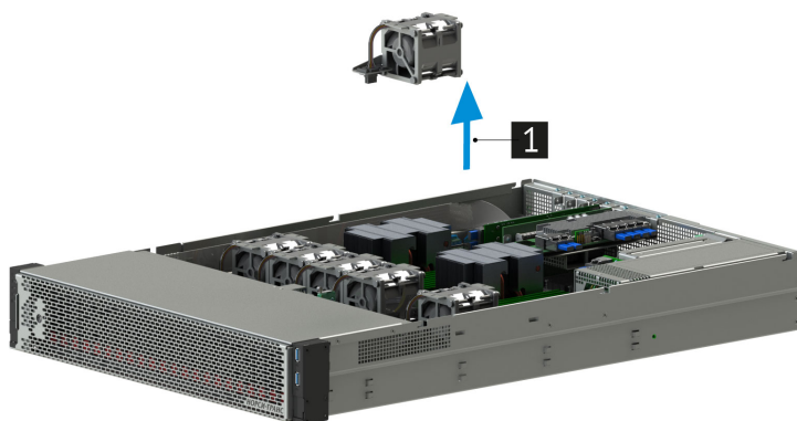
Рис. 33. Извлечение вентилятора из сервера
