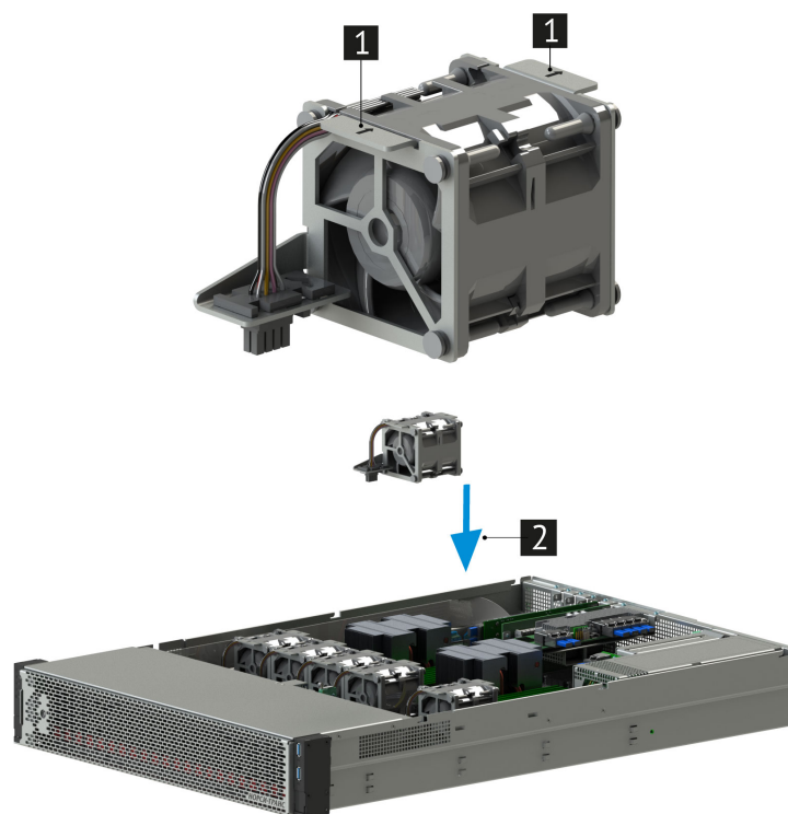
Рис. 34. Подключение вентилятора
