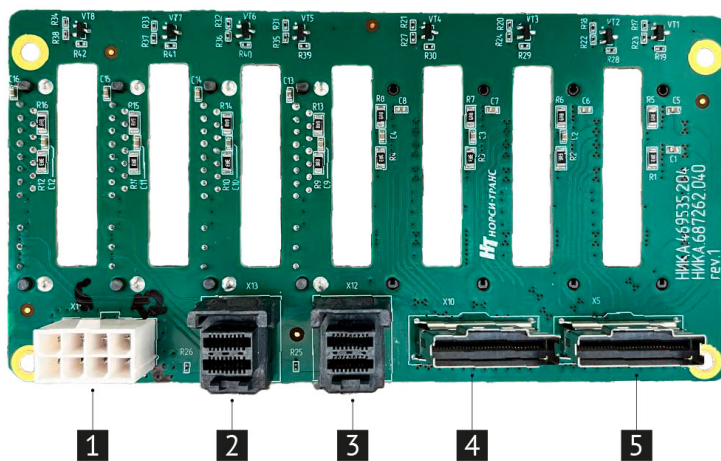
Рис. 10. Плата расширения 8SFF (НИКА.469535.204)
