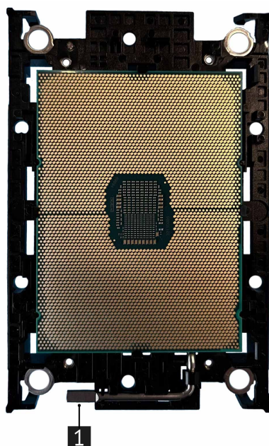
Рис. 41. Снятие процессора с радиатора
