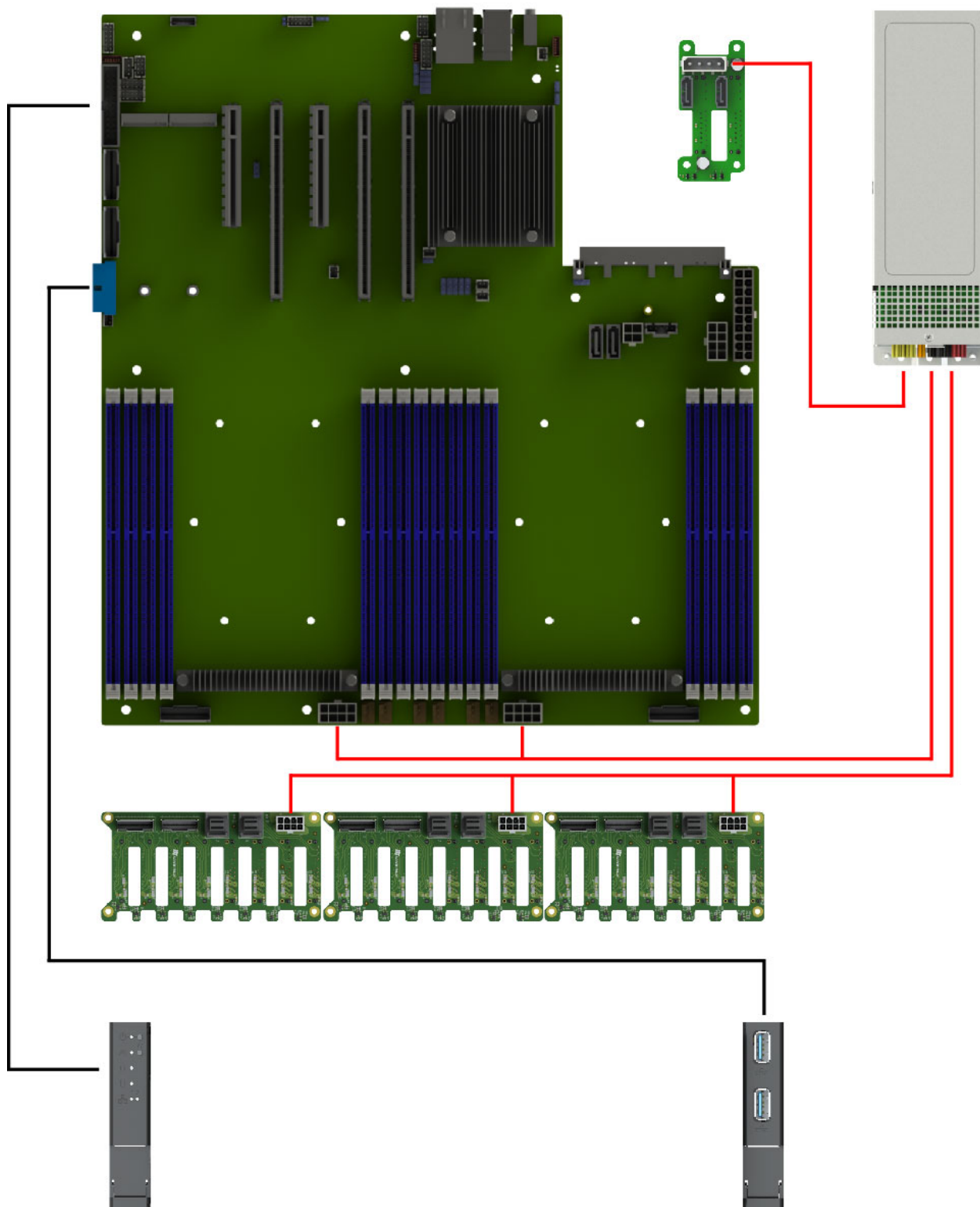
Рис. 25. Схема прокладки системных кабелей и кабелей питания при использовании платы расширения 2SFF SATA (НИКА.469535.131)
