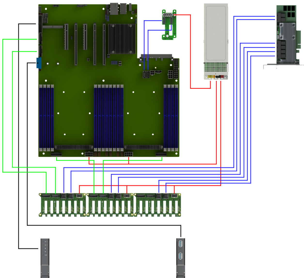
Рис. 32. Схема прокладки системных кабелей и кабелей Oculink-SLIMline X8-X8 с подключением PCIe RAID при использовании платы расширения 2SFF SATA (НИКА.469535.131)
