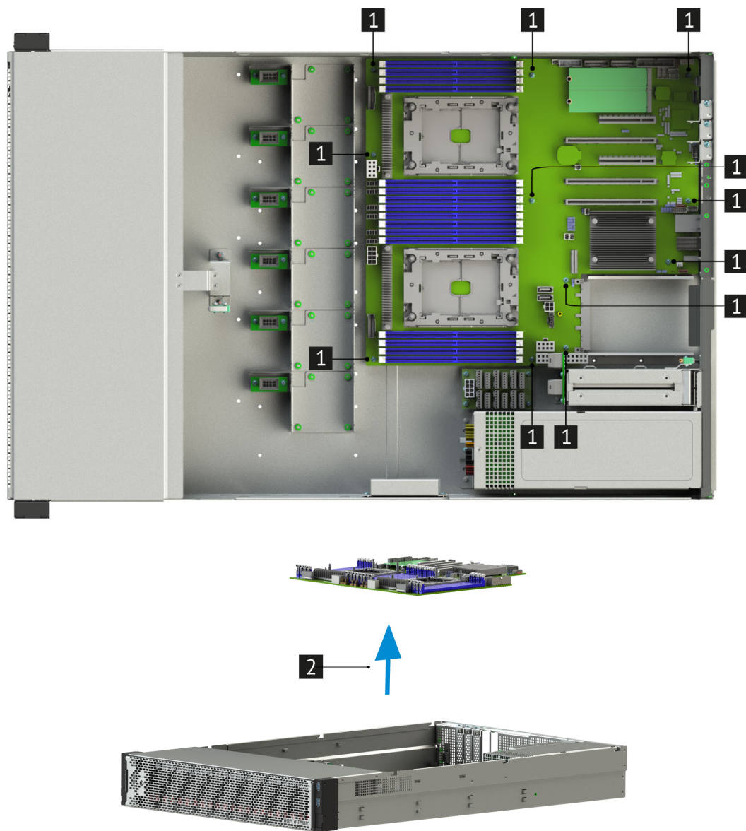
Рис. 43. Извлечение материнской платы из сервера
