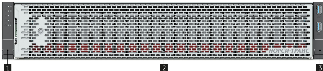
Рис. 2. Вид сервера спереди с защитной передней панелью
