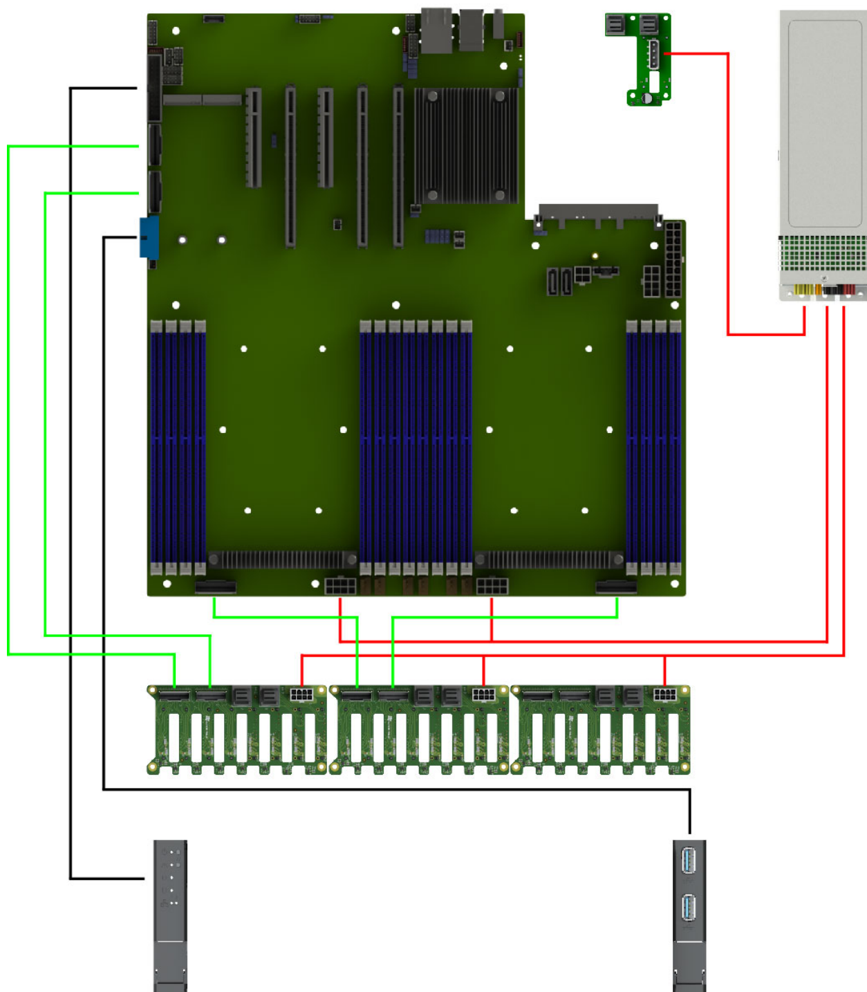
Рис. 29. Схема прокладки системных кабелей и кабелей SlimSAS-SlimSAS X8-X8 при использовании платы расширения 2SFF NVMe (НИКА.469535.220)
