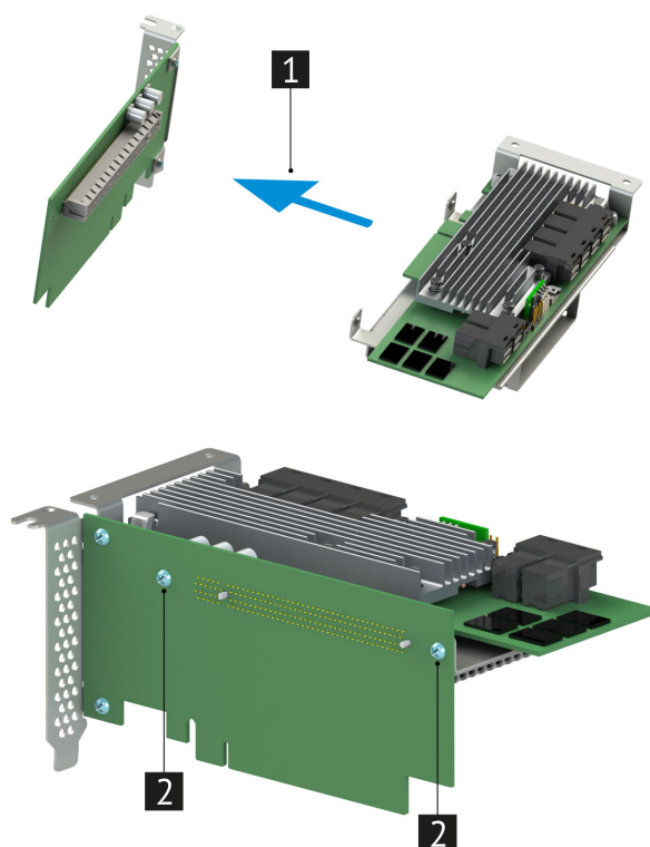
Рис. 55. Установка контроллера дискового MegaRAID 9361-24i
