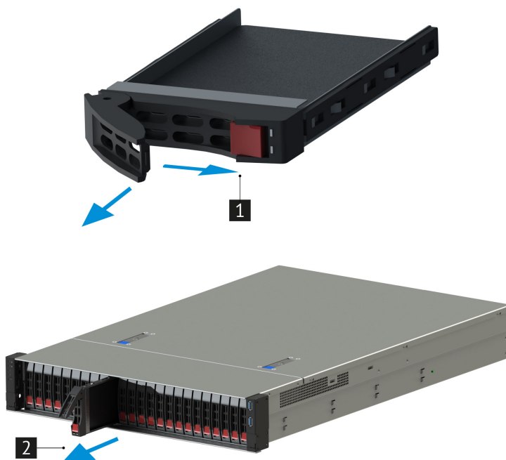
Рис. 45. Извлечение дисков
