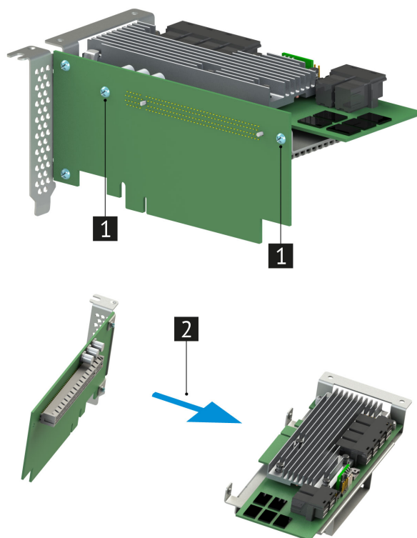
Рис. 54. Извлечение контроллера дискового MegaRAID 9361-24i
