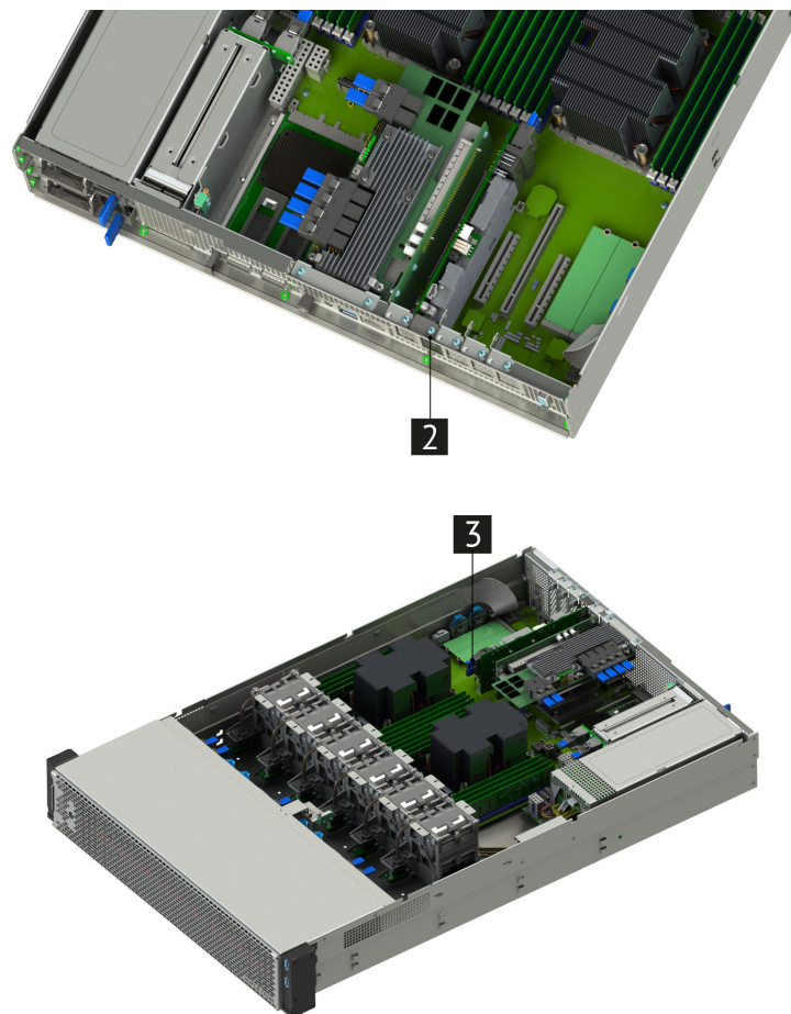
Рис. 57. Установка контроллера дискового MegaRAID 9361-16i
