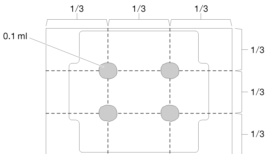
Рис. 42. Нанесение термопасты
