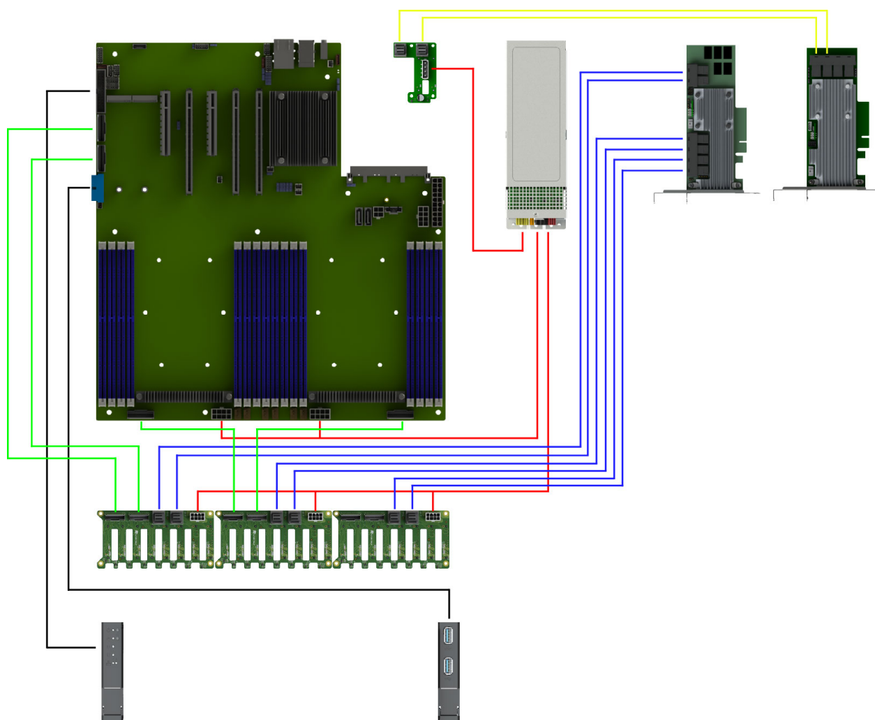
Рис. 31. Схема прокладки системных кабелей и кабелей Oculink-SLIMline X8-X8 с подключением PCIe RAID при использовании платы расширения 2SFF NVMe (НИКА.469535.220)
