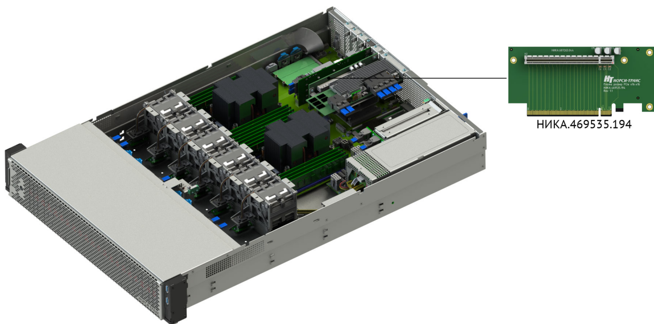
Рис. 13. Расположение PCIe-райзеров в сервере
