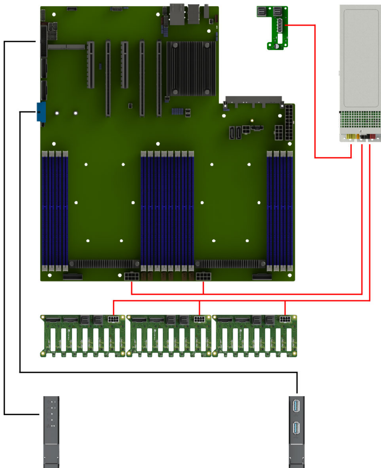
Рис. 26. Схема прокладки системных кабелей и кабелей питания при использовании платы расширения 2SFF NVMe (НИКА.469535.220)
