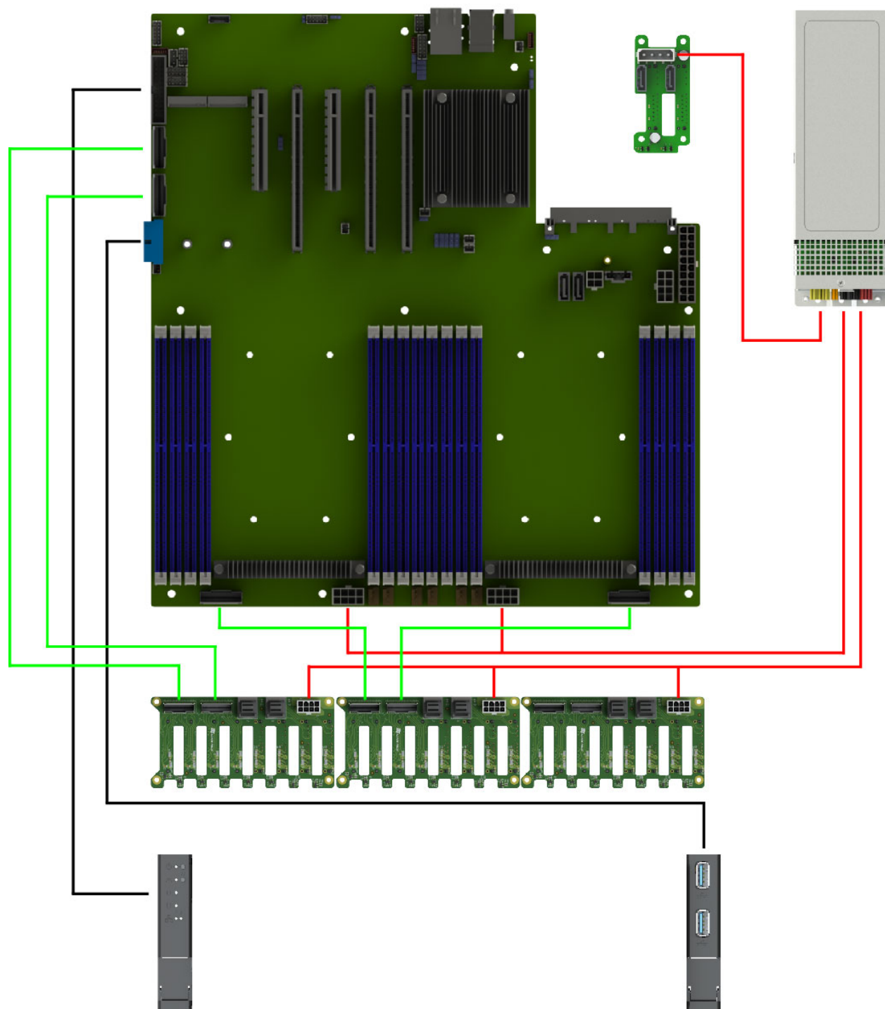
Рис. 30. Схема прокладки системных кабелей и кабелей SlimSAS-SlimSAS X8-X8 при использовании платы расширения 2SFF SATA (НИКА.469535.131)
