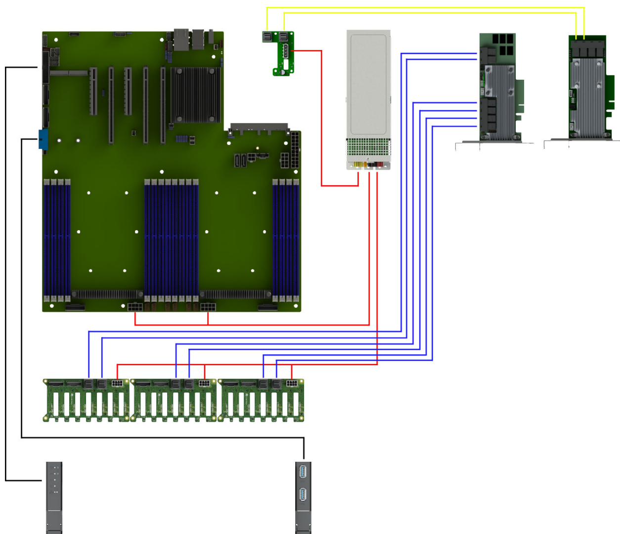
Рис. 27. Схема прокладки системных кабелей и кабелей питания с подключением PCIe RAID при использовании платы расширения 2SFF NVMe (НИКА.469535.220)
