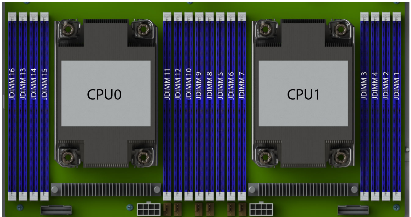
Рис. 35. Расположение разъемов
