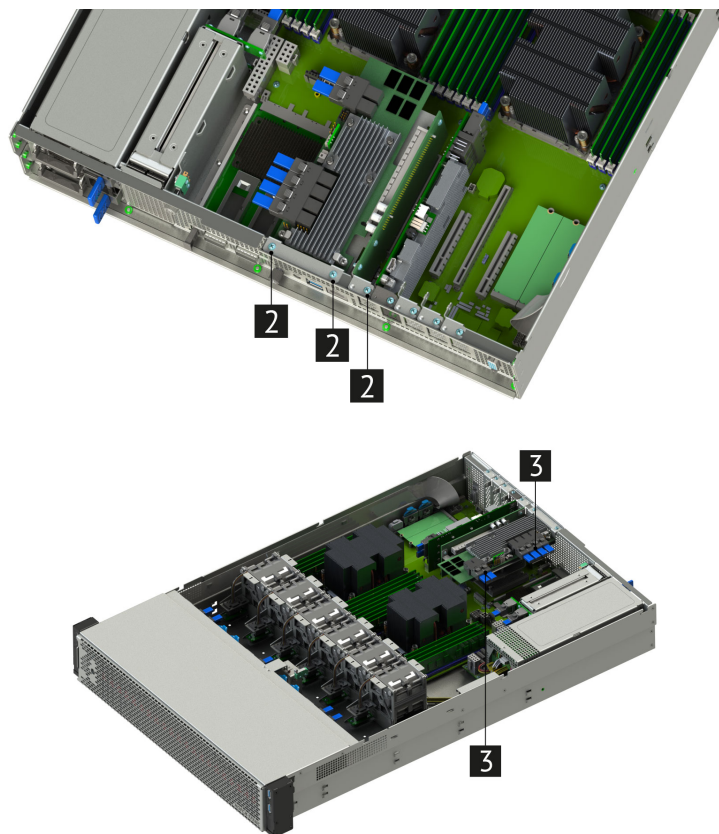
Рис. 53. Установка райзера PCIe x16-x16
