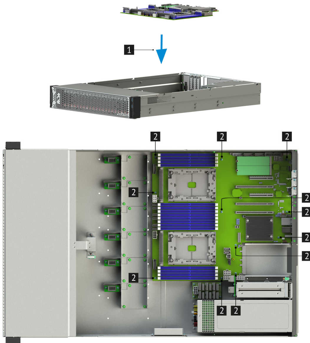
Рис. 44. Установка материнской платы в сервер
