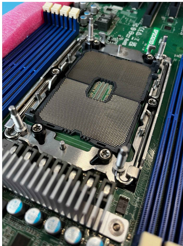
Рис. 39. Снятие модуля процессора с радиатором
