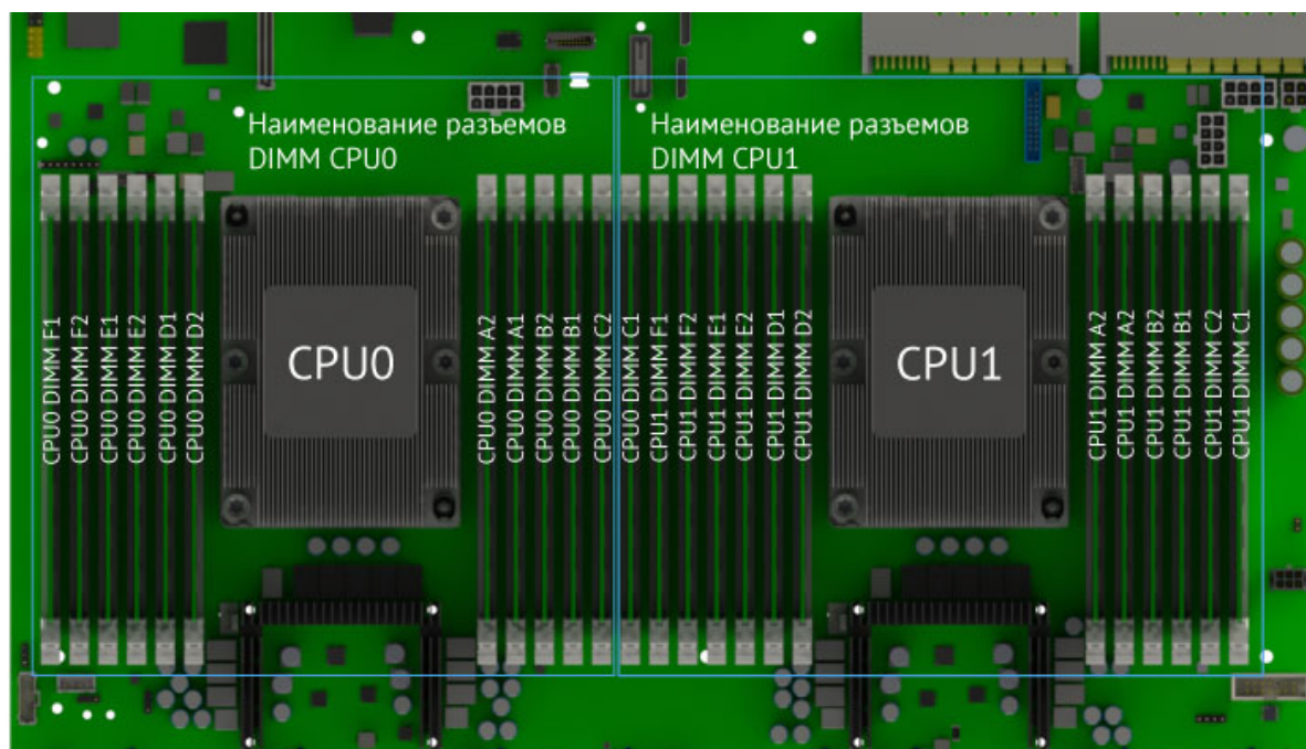
Рис. 30. Расположение разъемов
