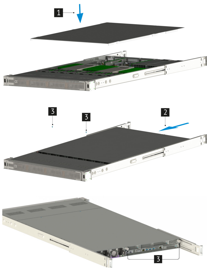
Рис. 21. Установка верхней крышки платформы
