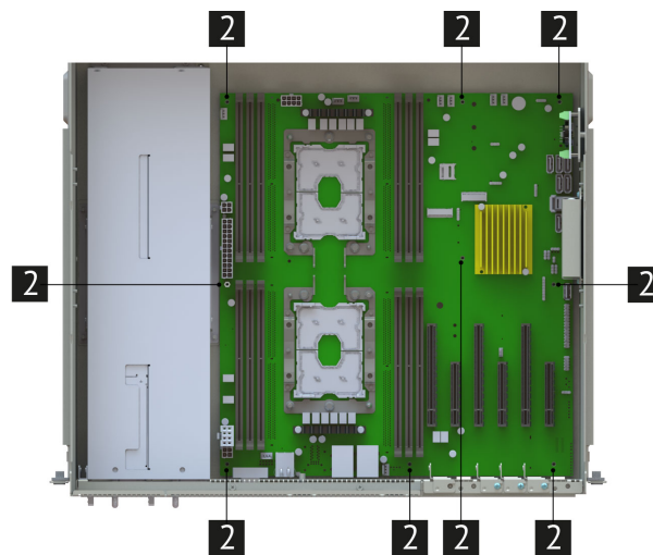
Рис. 44. Установка материнской платы
